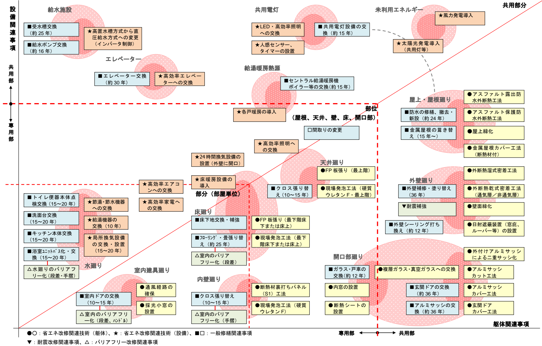
図 集合住宅における一般的な維持・修繕工事に関連する省エネ改修工事項目の例
