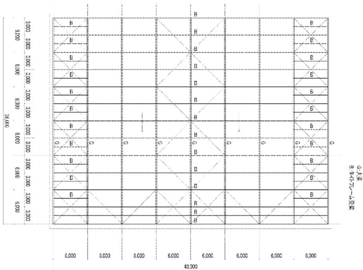
図 A3.1 設計対象の架構
