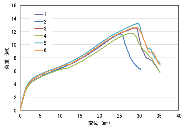
(b) ねじ留め位置が 20mm の場合
