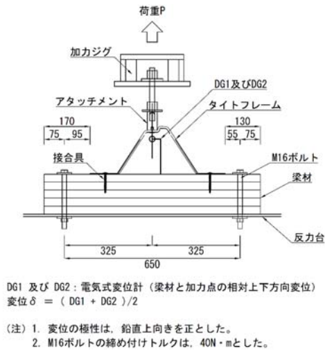
図 4.1 試験方法
