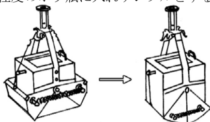
[エクマンバージ型採泥器]
