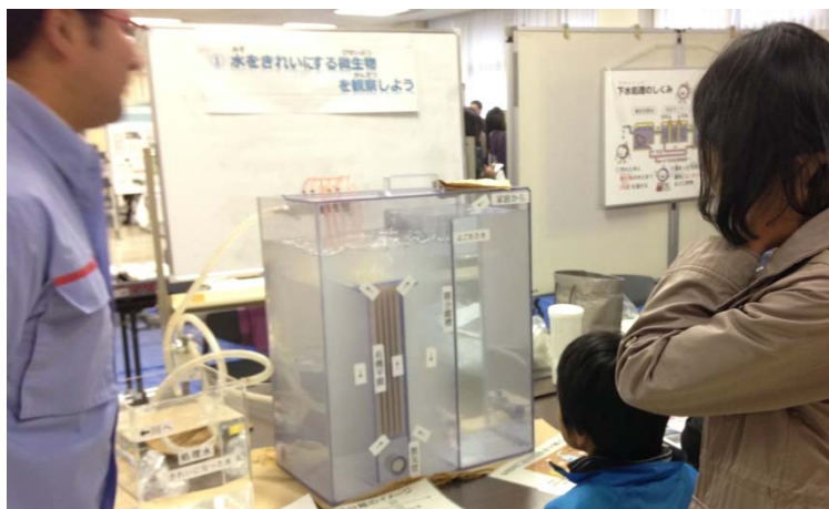
模型による膜分離活性汚泥法のデモンストレーション
