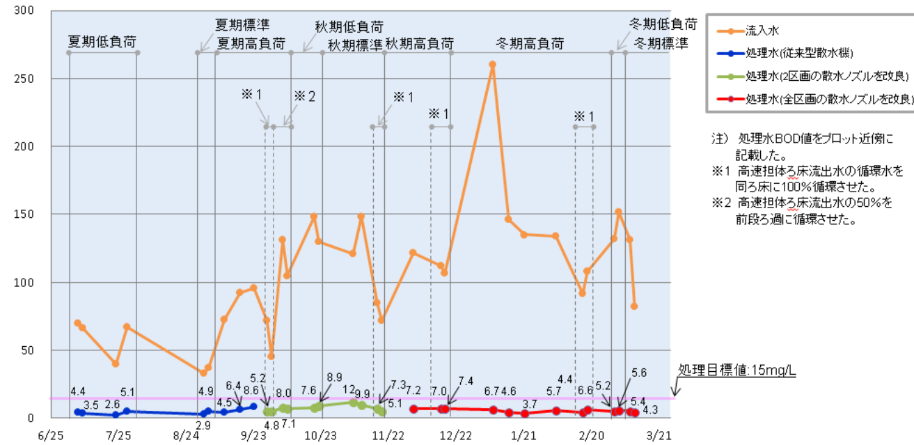
流入下水および処理水BODの経日変化
