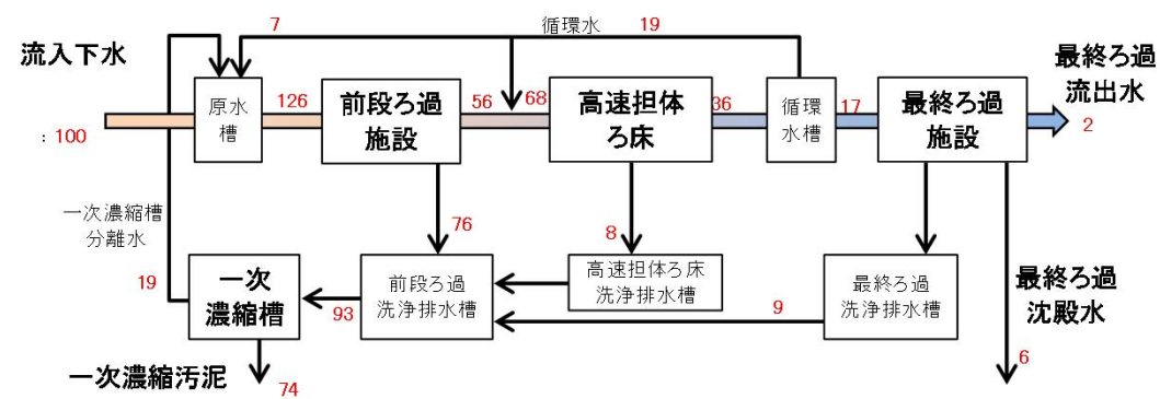
固形物収支 (実測値平均)
