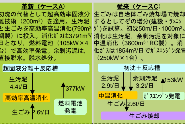
都市ガス併用で消化ガス100%利用可能で発電効率は40%以上
