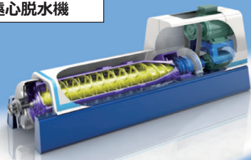
機内二液調質型 遠心脱水機
