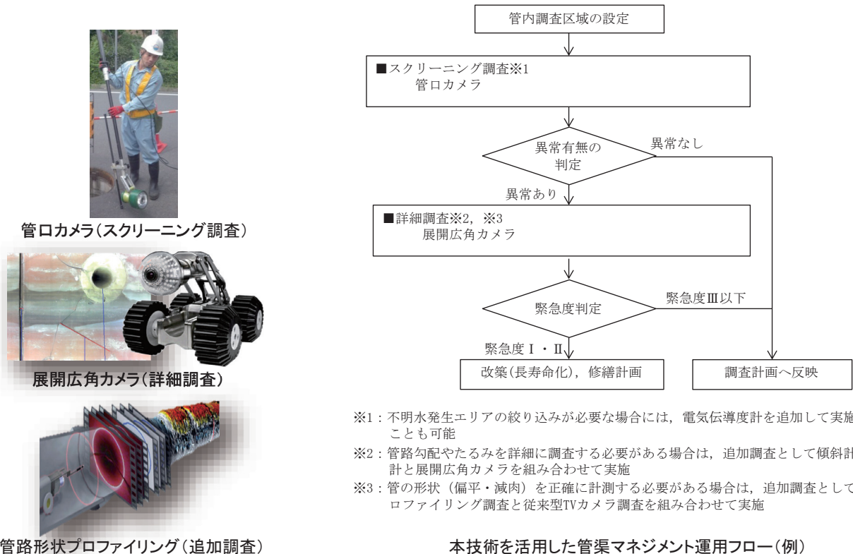
本技術を活用した管渠マネジメント運用フロー(例)
