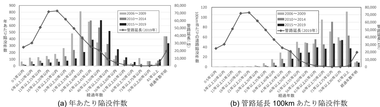
図 1 1 道路陥没件数と布設からの経過年数の関係
