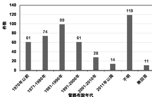
図5 被災した下水道管路の布設年代
