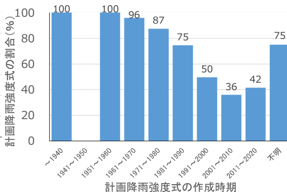
図 1 4 降雨資料期間が 40 年未満の割合
