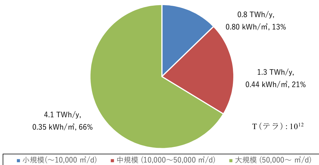
図 4-1 全国の下水处理場の年間消費電力量（規模別、平成 28 年度版下水道統計を整理）
