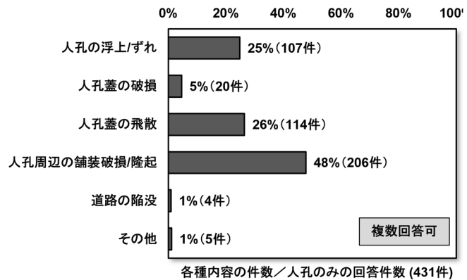
図7 人孔とその周辺の被害の状況
