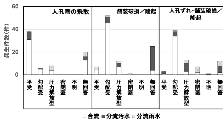
(a) 人孔蓋の飛散 (b) 舗装破損/隆起 (c) 人孔ずれ・舗装破損/隆起
