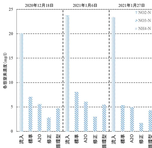
図1 各態窒素濃度
