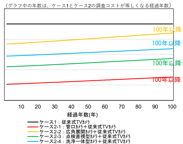
(c) 塩ビ管 (左：詳細調査に対する組合せ調査のコスト比、右：コスト縮減額・リスク顕在化費用)
