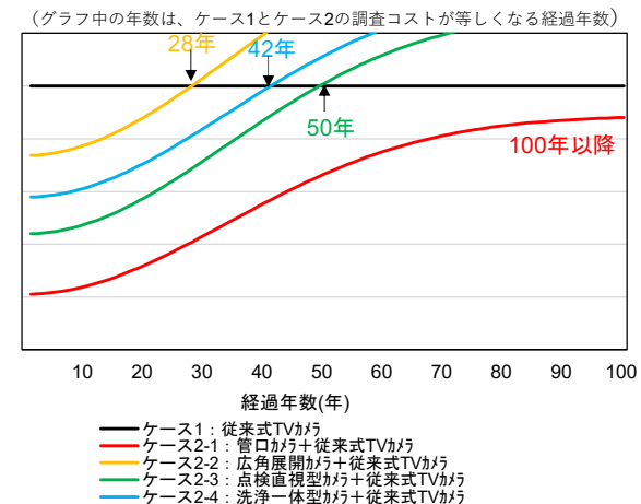
(b) 陶管 (左：詳細調査に対する組合せ調査のコスト比、右：コスト縮減額・リスク顕在化費用)
