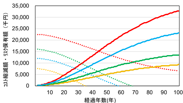
(a) コンクリート管 (左：詳細調査に対する組合せ調査のコスト比、右：コスト縮減額・リスク顕在化費用)
