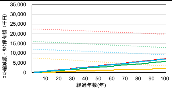
(c) 塩ビ管 (左：詳細調査に対する組合せ調査のコスト比、右：コスト縮減額・リスク顕在化費用)
