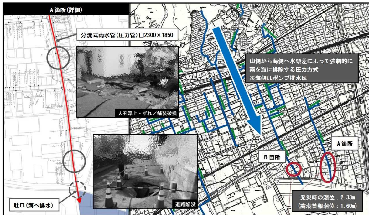
図 1 4 被害場所の詳細 (B 市)
