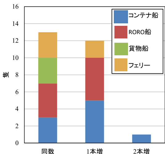
図-2.4(b) 船種別の係留索最大本数の増加数 (平時から津波来襲時)
