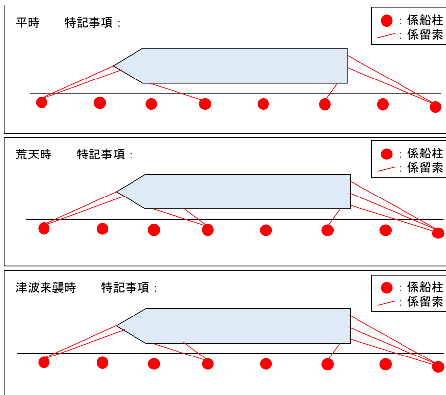
図-2.1 係船柱と係留索の平面的な掛け方に関する回答例（コンテナ船，10,000GT）
