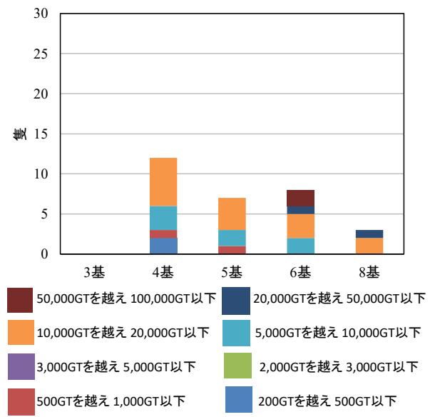
図-A. 2(b) 船型別の係船柱利用数 (荒天時)
