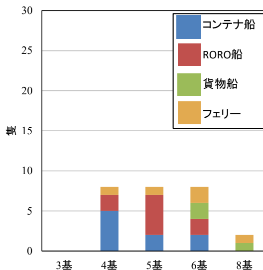
図-A.1(c) 船種別の係船柱利用数 (津波来襲時)
