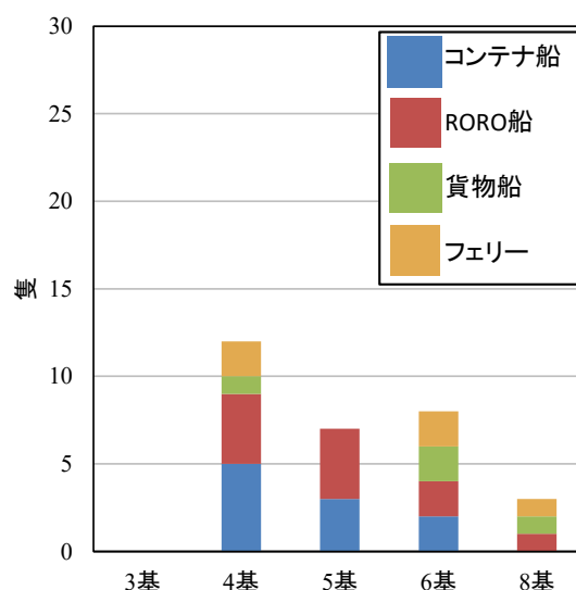
図-A.1(b) 船種別の係船柱利用数 (荒天時)
