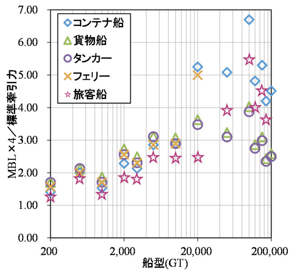
図-4.4 概算牽引力 (係留索4本) と標準牽引力の比較 (標準牽引力を1.0とした場合)
