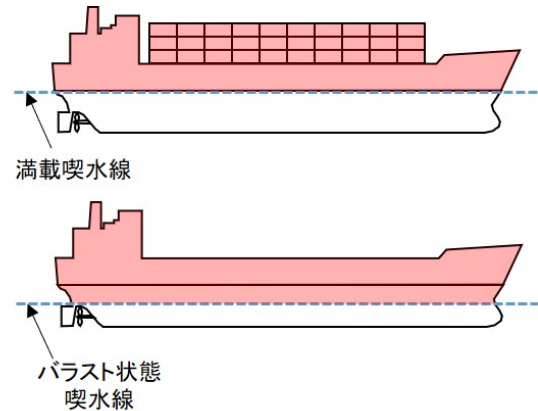
図-3.2 船側投影面積 A_1 を算定する際の範囲 (概念図)
