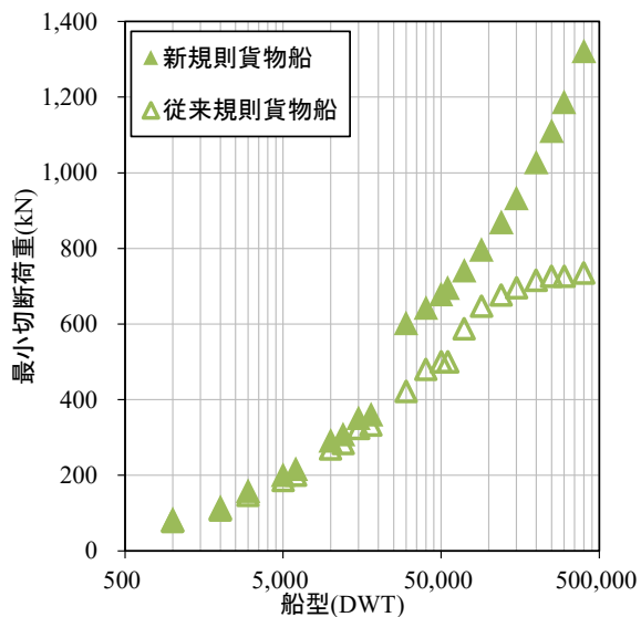
図-3.3(b) 貨物船の従来規則と新規規則による最小切断荷重の比較
