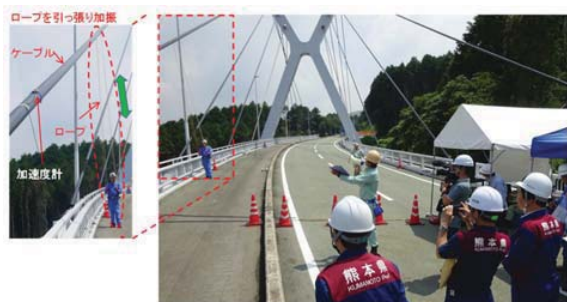
写真 ケーブル張力の確認試験状況
