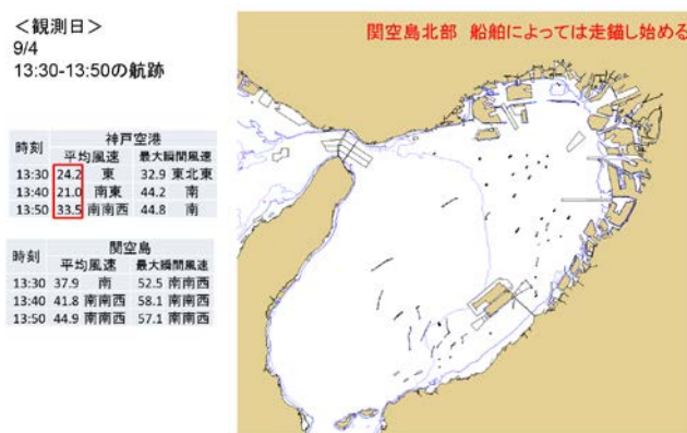
図-5.8 2018年9月4日13:30～13:50の船舶の航跡
