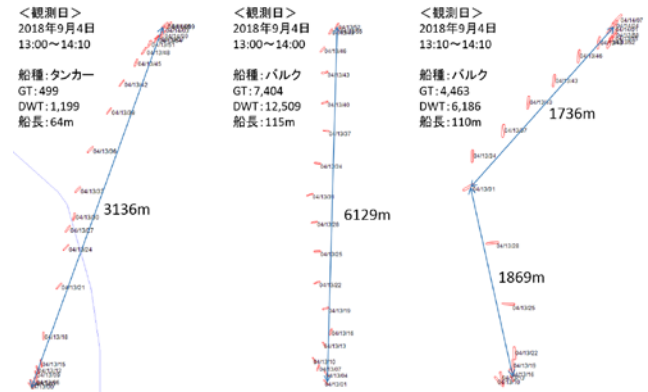
図-5.3 走錨距離の計測例
