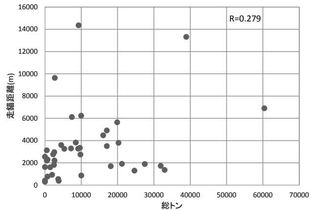
図-5.4 走錨した船舶の総トンと走錨距離の関係
