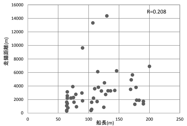
図-5.5 走錨した船舶の船長と走錨距離との関係
