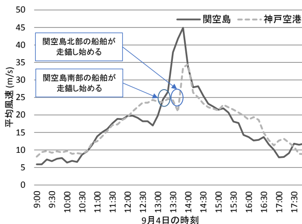
図-5.9 台風21号大阪湾通過前後の風速データ
