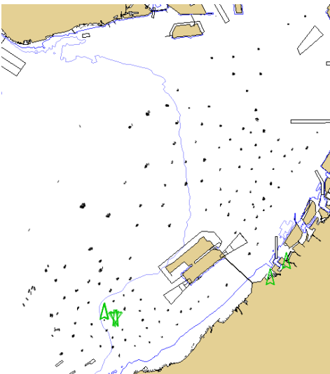
図-5.2 2017年台風18号最接近時の船舶の航跡 (2017年9月17日20:10~21:10)
