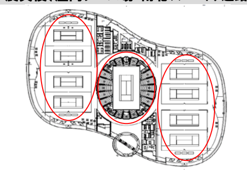
図. 参-13 部隊中継基地としての利用状況平面図
