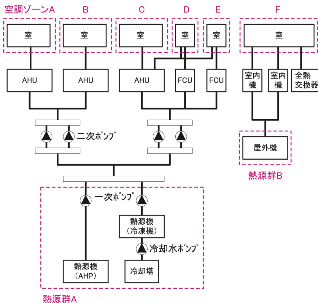
図 2-5-1 熱源群の例
