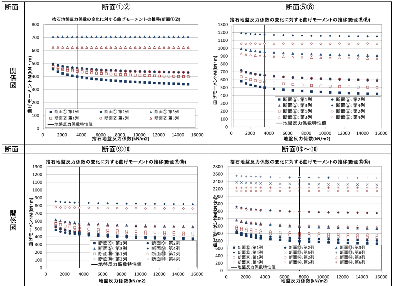
付表 B-16 捨石の地盤反力係数の変化に対する曲げモーメントの推移
