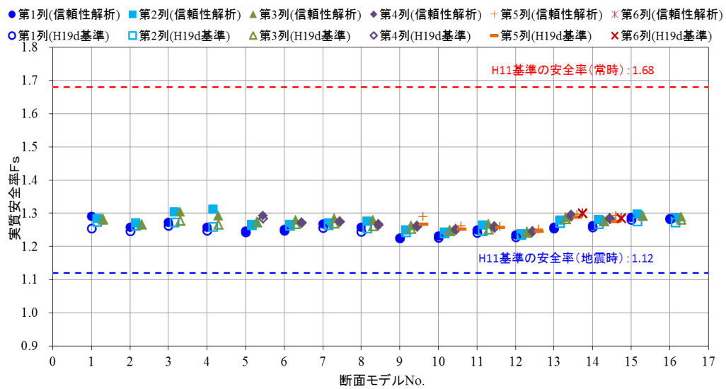
付図 F-5 各検討断面の実質安全率(設定 A)
