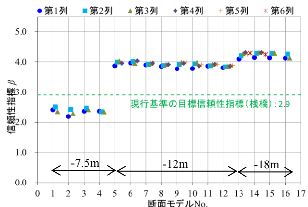
図-37 現行港湾基準を満たす断面の信頼性指標
