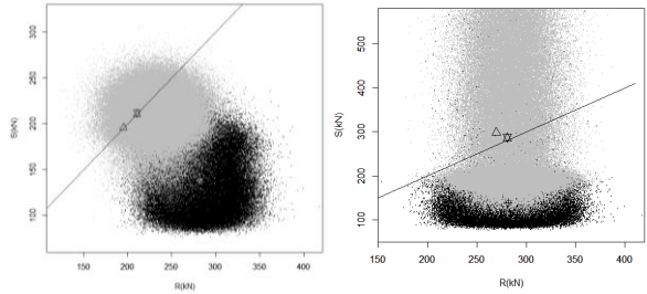
付図 F-16 限界圧縮率以降の防舷材反力の設定方法による破壊点の変化(例：断面⑤第1列)
