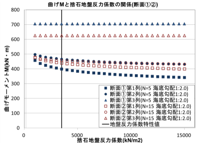
付図 B-4 曲げモーメントと捨石地盤反力係数の関係
