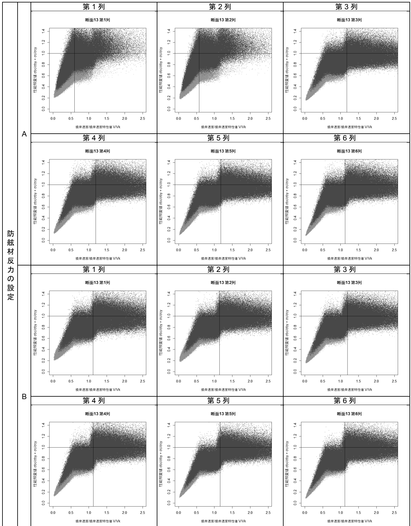
付表 F-68 接岸速度-性能照査値分布図(断面⑬ 設定 A および設定 B)
