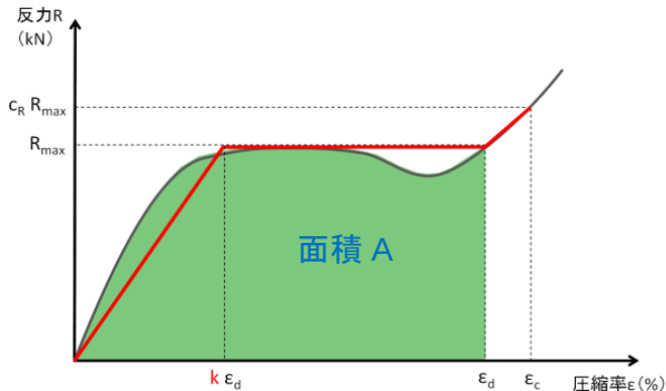
図-26 性能曲線面積 A
