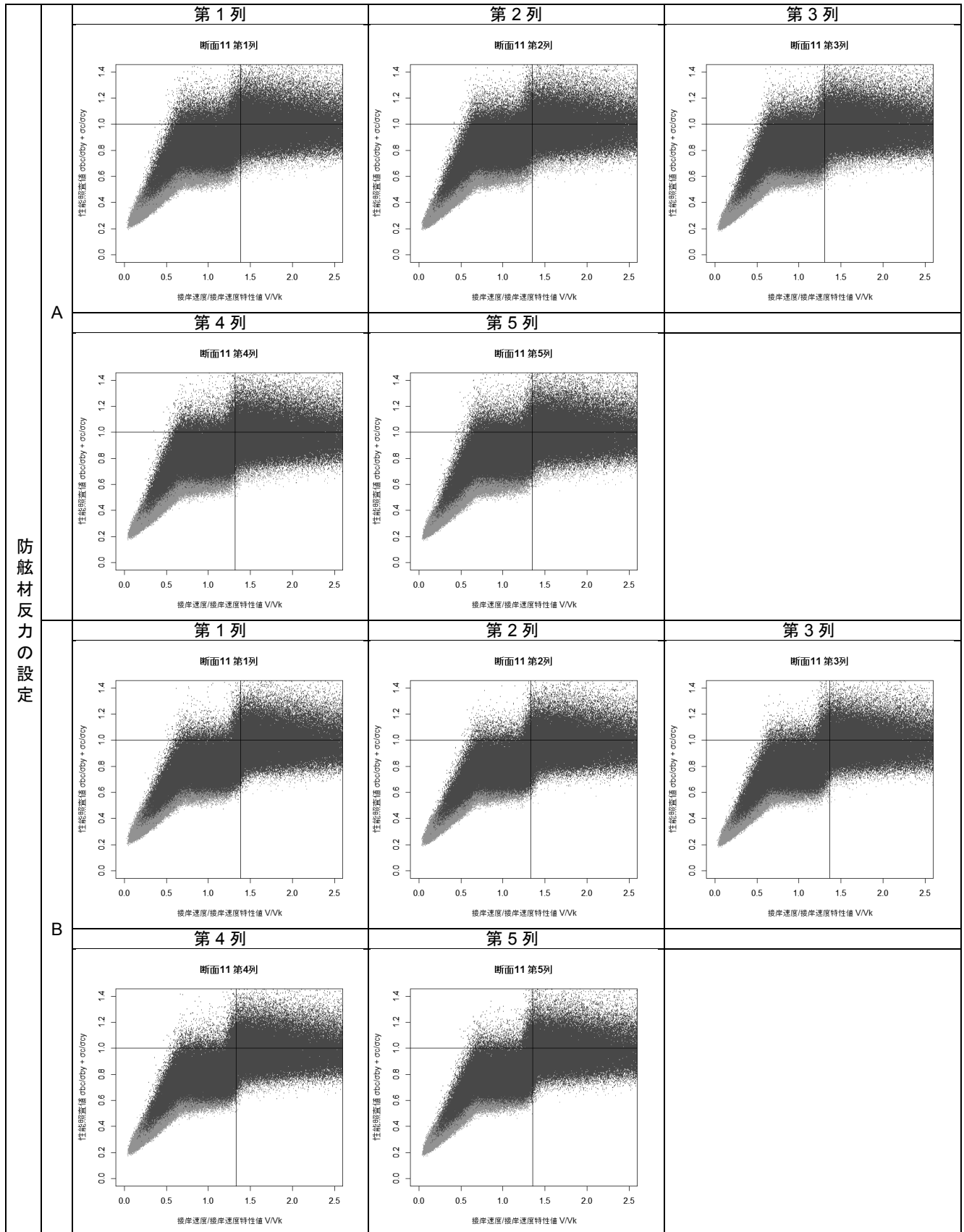
付表 F-64 接岸速度-性能照査値分布図(断面⑪ 設定 A および設定 B)
