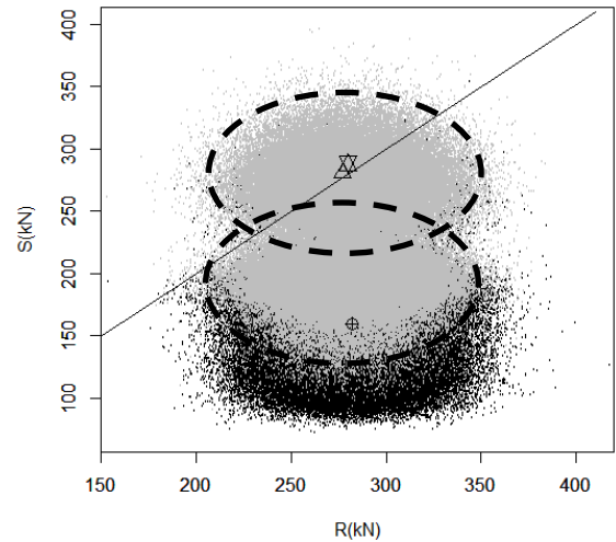
図-33 信頼性解析におけるサンプリング結果の二極分布
