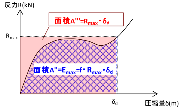
図-24 エネルギー吸収効率を示す係数 f
