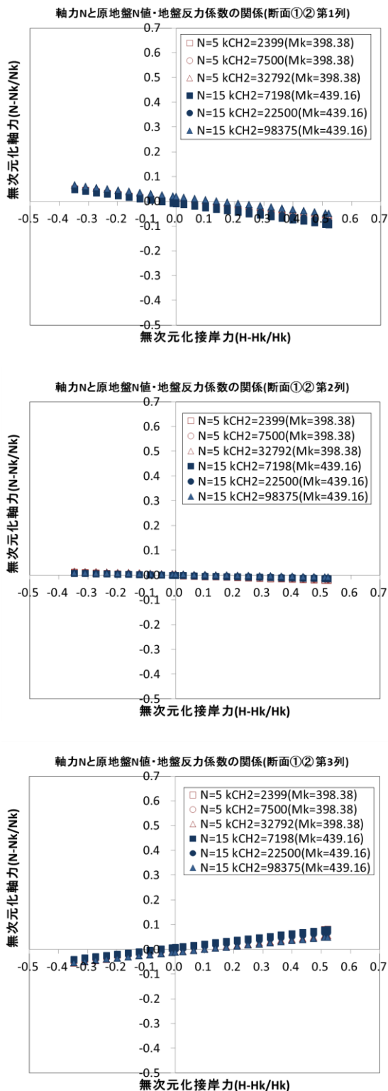
図-8 無次元化した軸力と原地盤 N 値，および地盤反力係数の関係(断面①②)
