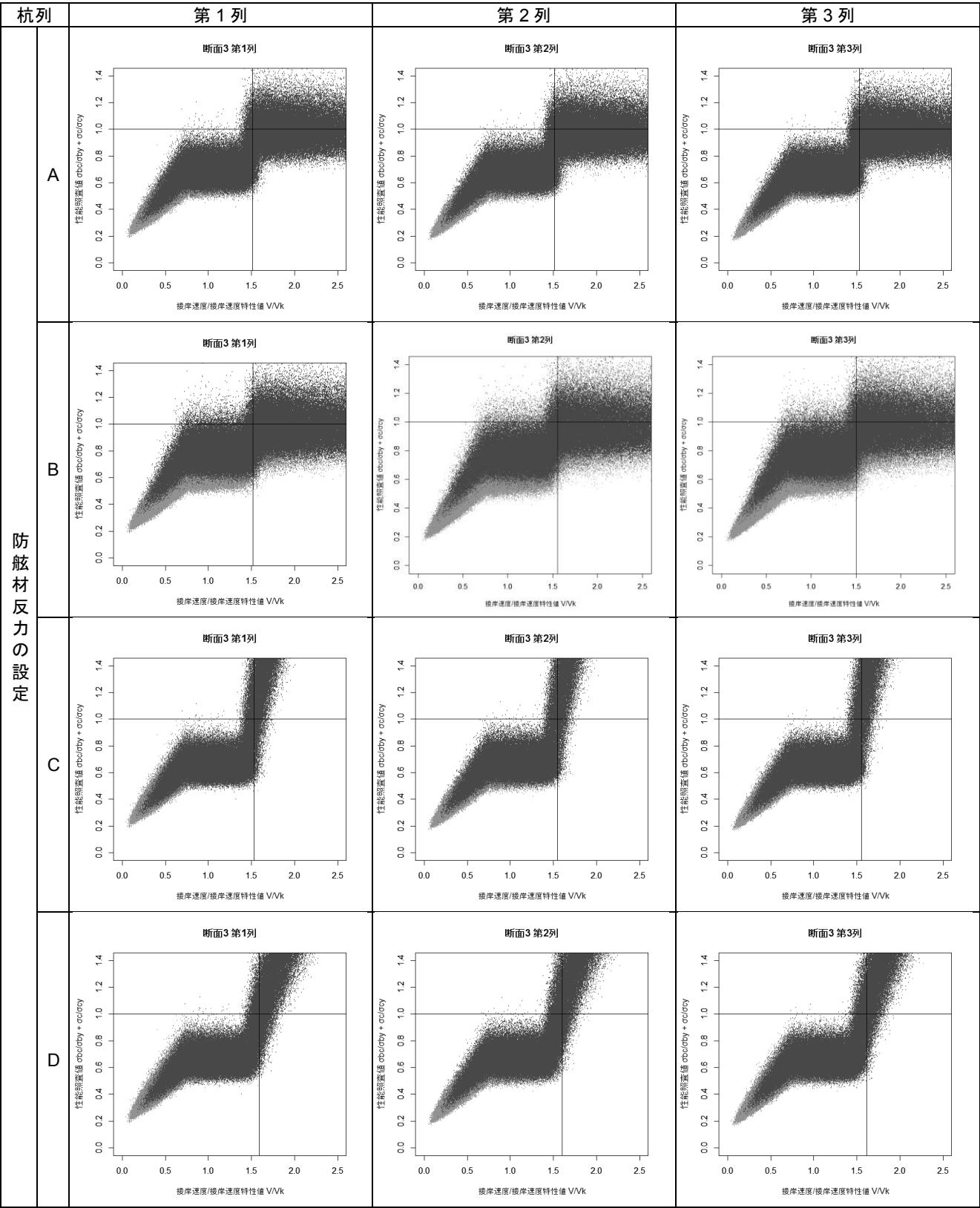
付表 F-54 接岸速度-性能照査値分布図(断面③)
