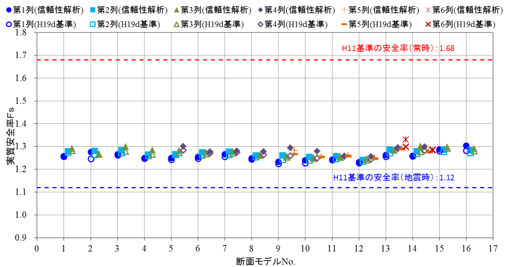
付図 F-8 各検討断面の実質安全率(設定 B)
