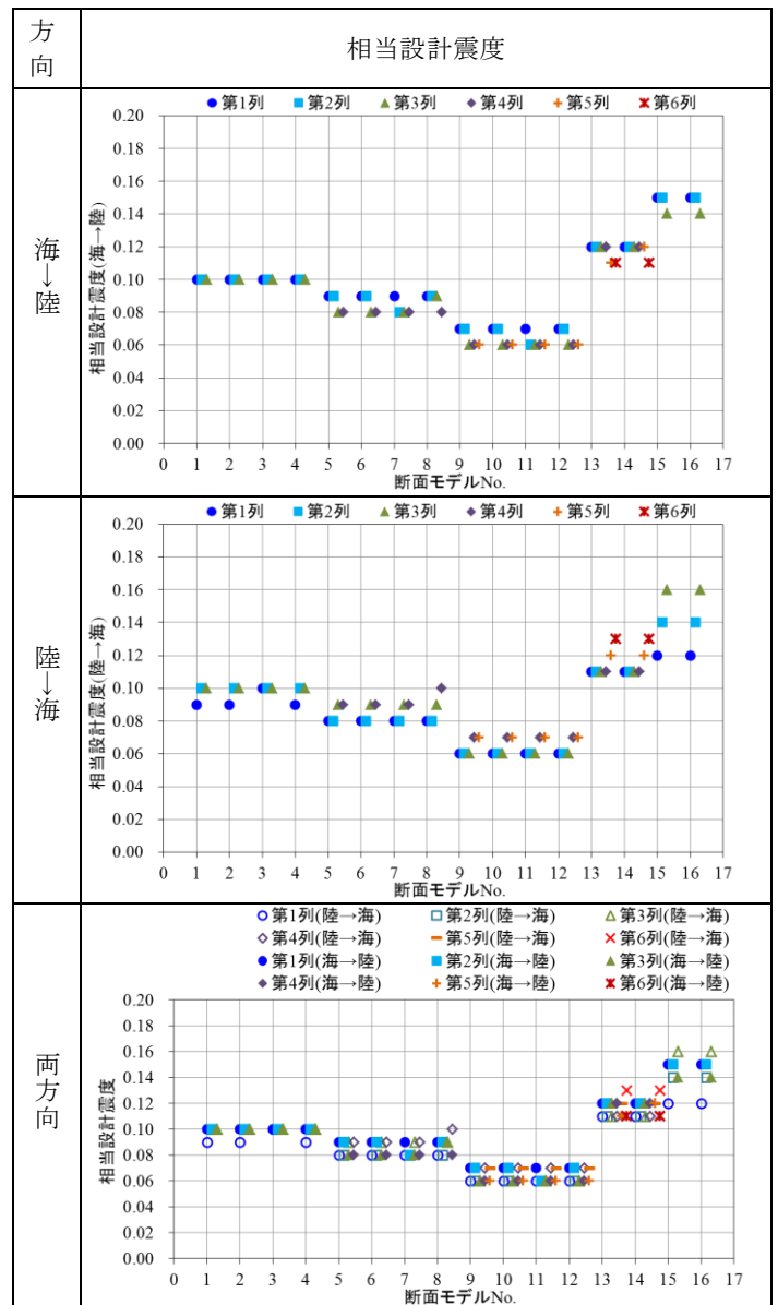
付表 I-3 相当設計震度
