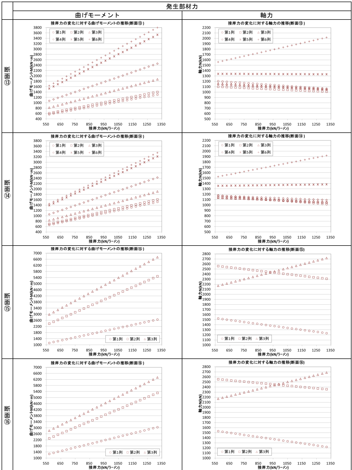
付表 B-14 接岸力の変化に対する近似式出力値の推移(断面⑬～⑯)
