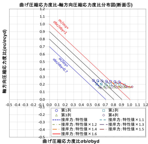
付図 C-5 曲げ圧縮・軸方向圧縮応力度比分布図(設計水深 12m : 断面⑤(杭列数 4), 断面⑨(杭列数 5))
