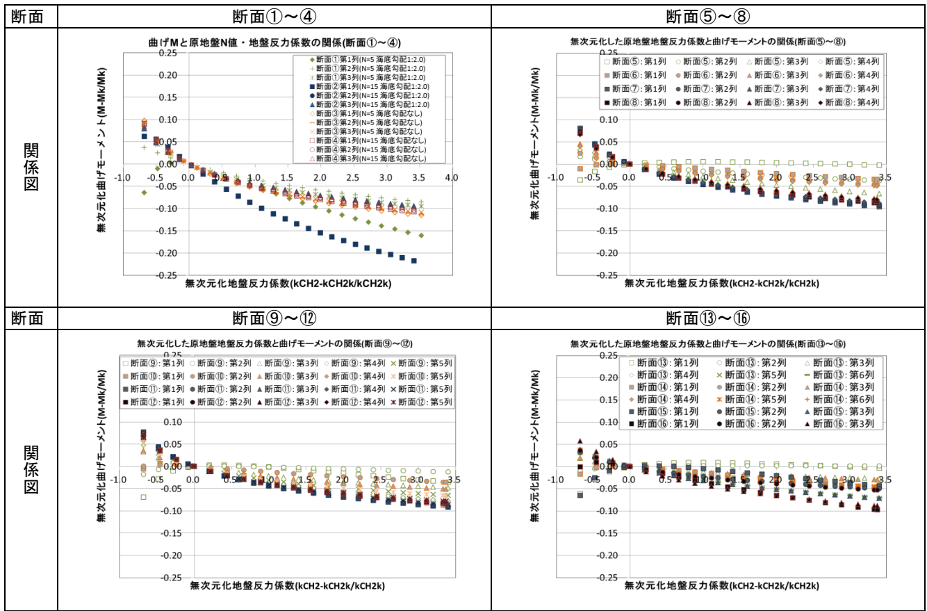
付表 B-21 無次元化した原地盤の地盤反力係数と曲げモーメントの関係
