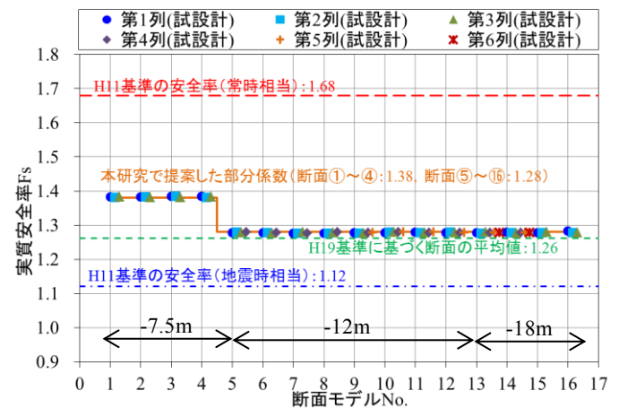
図-48 試設計断面の実質安全率
