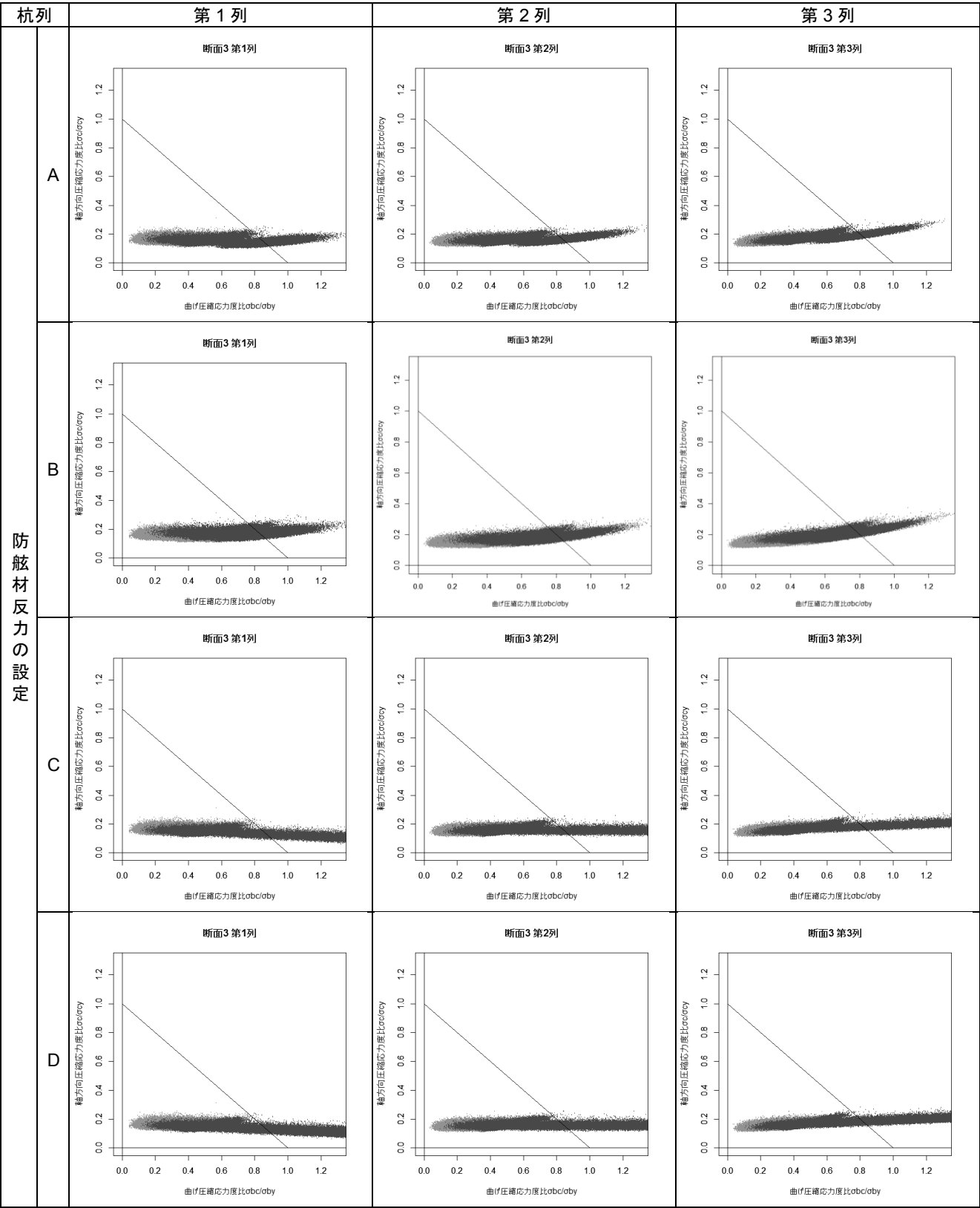
付表 F-32 杭列毎の曲げ圧縮応力度比-軸方向圧縮応力度比分布図(断面③)
