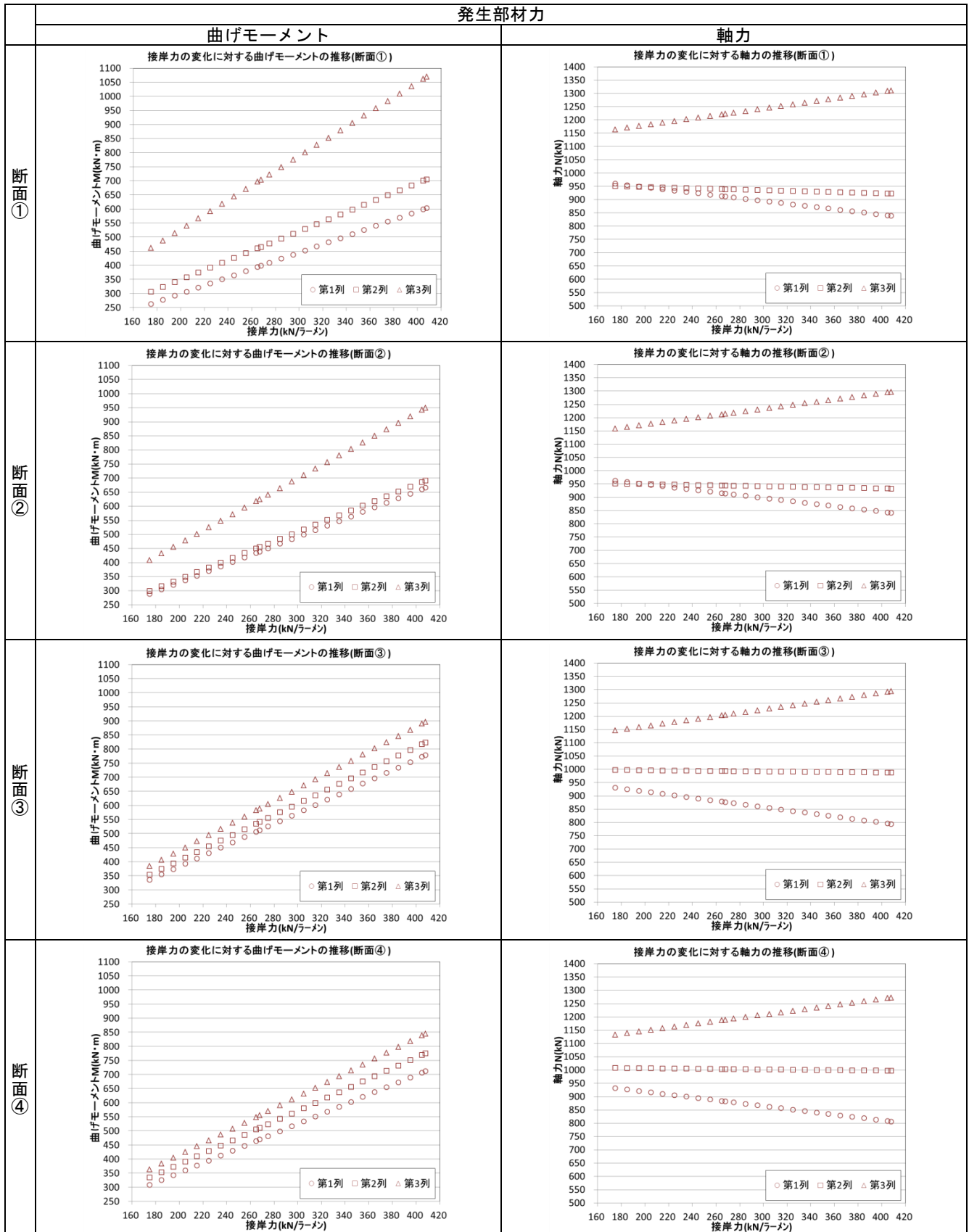
付表 B-11 接岸力の変化に対する近似式出力値の推移(断面①～④)
