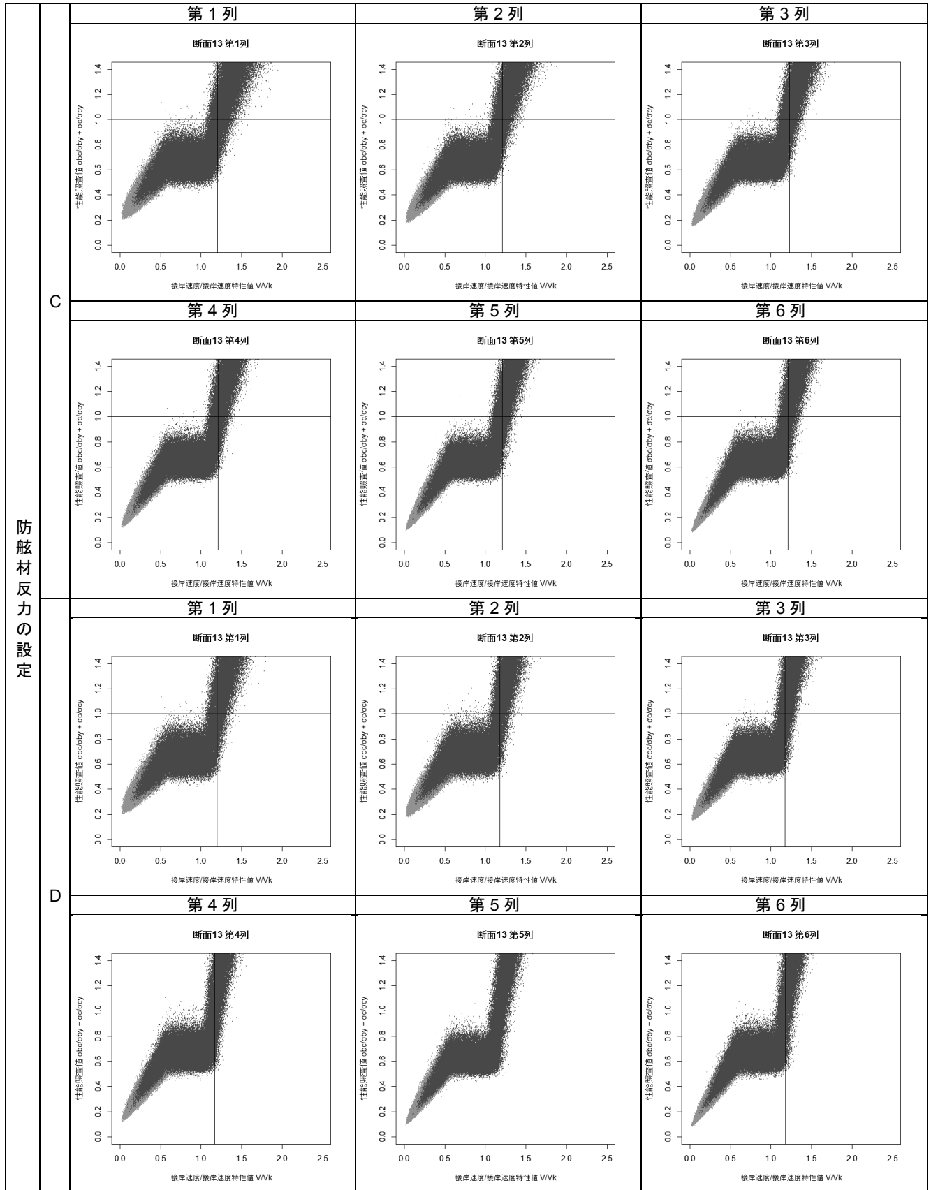
付表 F-69 接岸速度-性能照査値分布図(断面⑬ 設定 C および設定 D)
