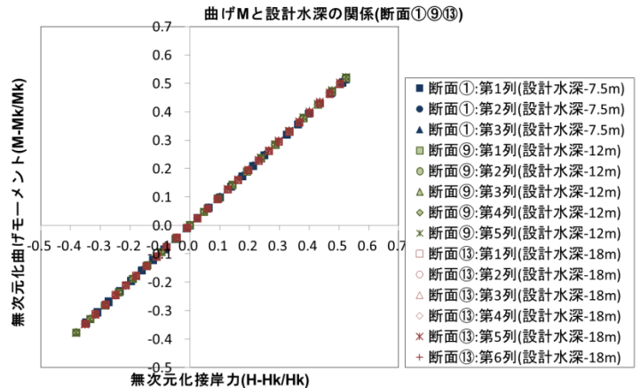
付図 B-9 無次元化した接岸力の変化に対する曲げモーメントと設計水深の関係
