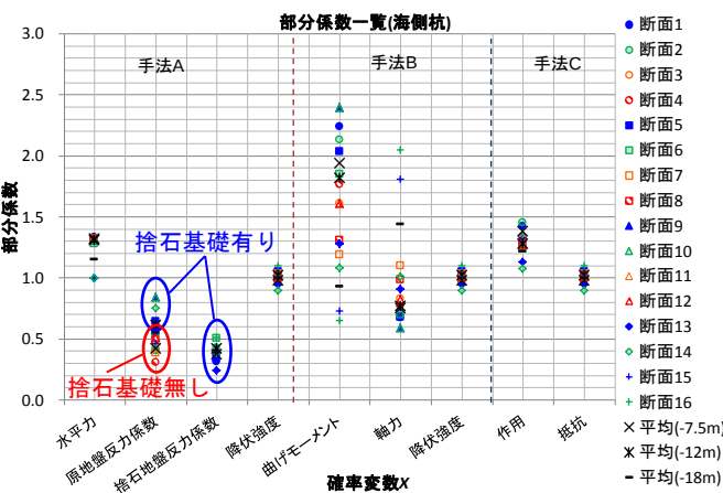
図-41 手法 A における部分係数のバラツキ (目標破壊確率 1.52 \times 10^{-4} 、ターゲット設計水深-12m)
