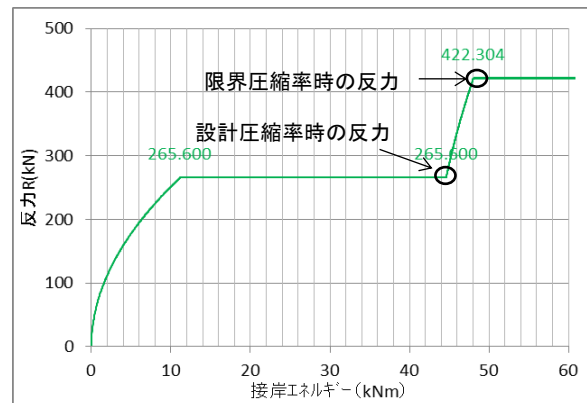
図-34 モデル防舷材の接岸エネルギー-反力関係式
