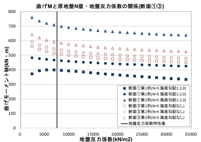
付図 B-1 原地盤の地盤反力係数の変化に対する曲げモーメントの推移(断面①③, N=5)
