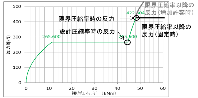
付図 F-15 モデル防舷材の接岸エネルギー-反力関係式
