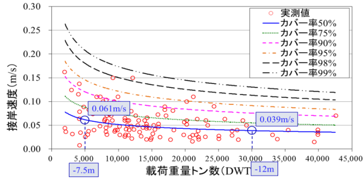
図-12 カバー率別の接岸速度と船型の関係（貨物船）
