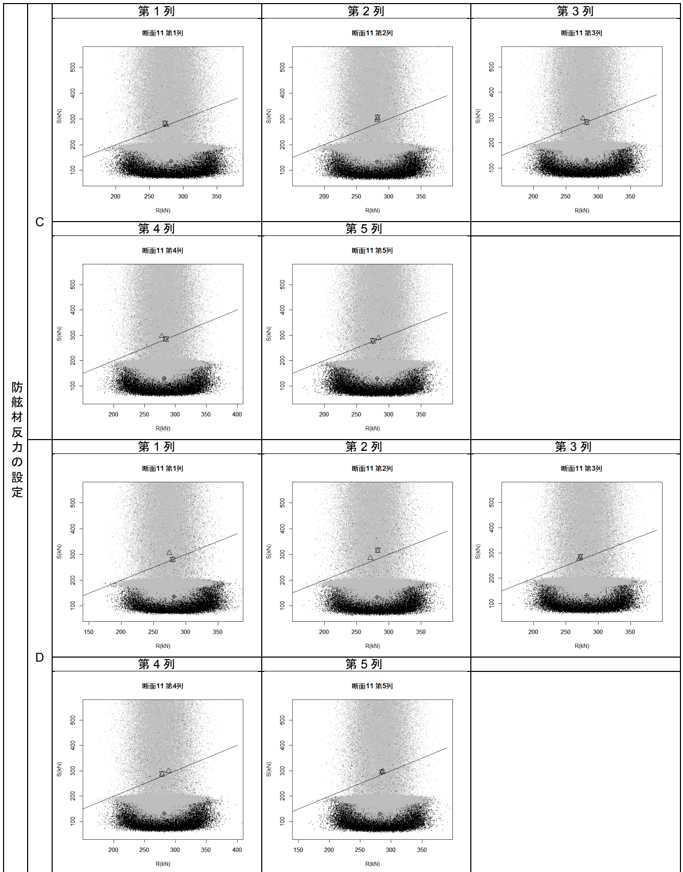
付表 F-21 杭列毎の抵抗-作用分布図(断面⑪ 設定 C および設定 D)
