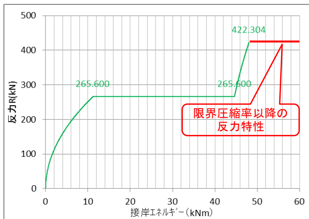
図-32 限界圧縮率以降の反力特性の設定
