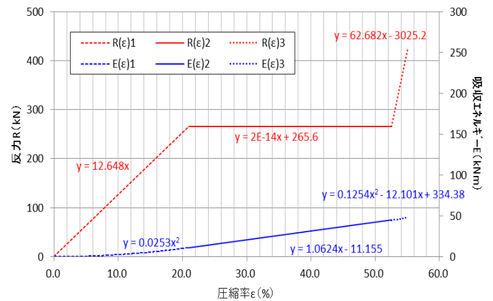
図-30 モデル化後の性能曲線図
