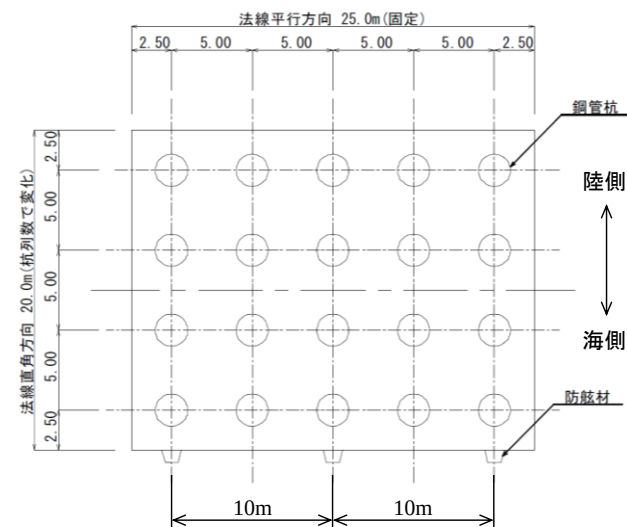
図-15 上部工形状（例：断面モデル⑤, ⑥, ⑦, ⑧）
