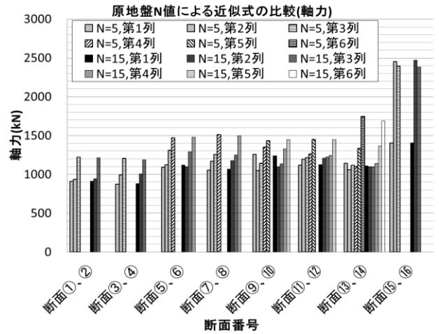
付図 A-2 N 値に対する軸力の比較
