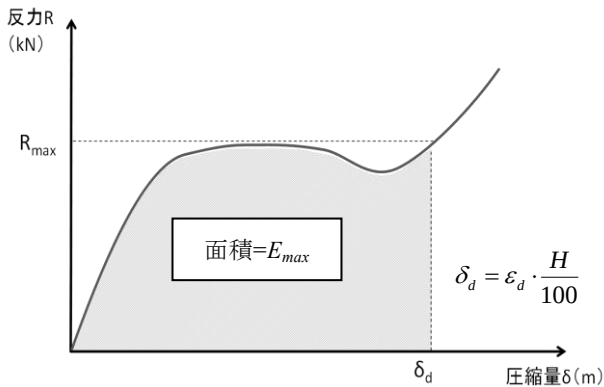
図-25 反力 R -圧縮量 \delta 曲線と吸収エネルギーの関係
