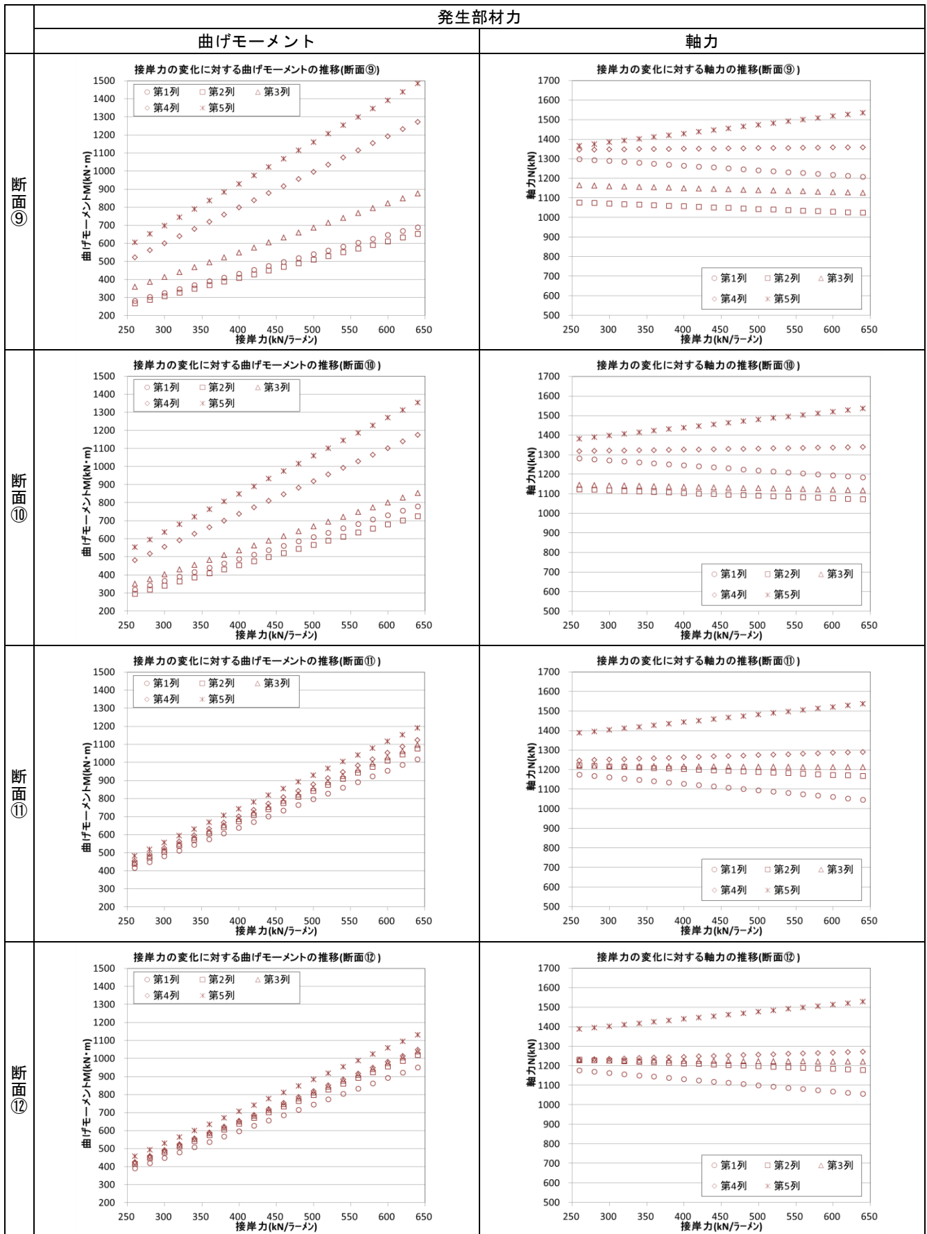
付表 B-13 接岸力の変化に対する近似式出力値の推移(断面⑨～⑫)
