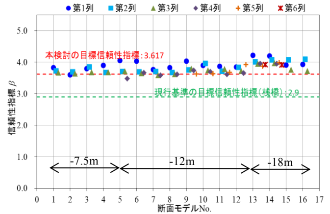
図-47 試設計断面の信頼性指標
