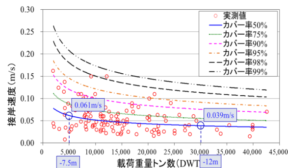
図-43 カバー率別の接岸速度と船型の関係 (貨物船)
