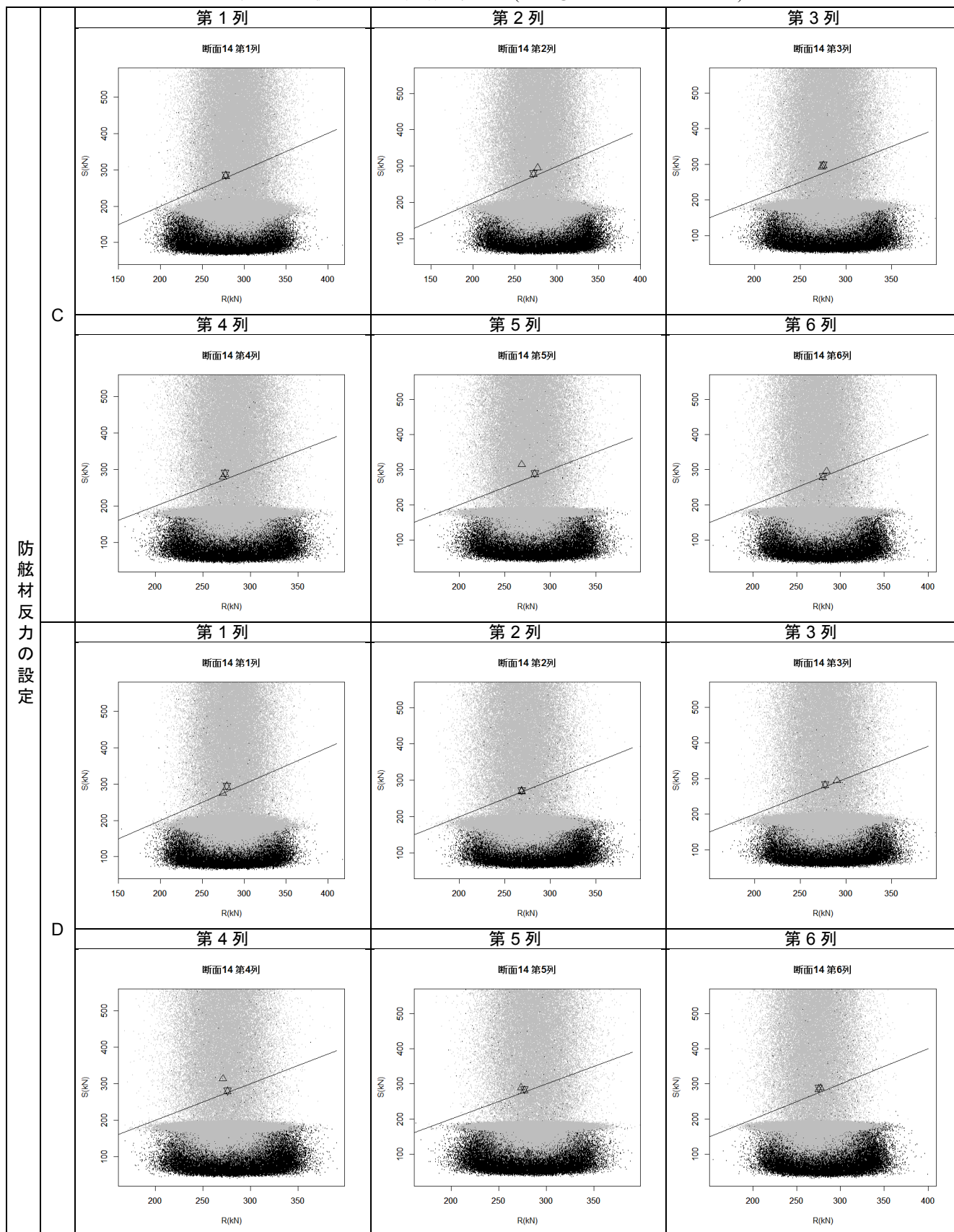
付表 F-27 杭列毎の抵抗-作用分布図(断面⑭ 設定 C および設定 D)
