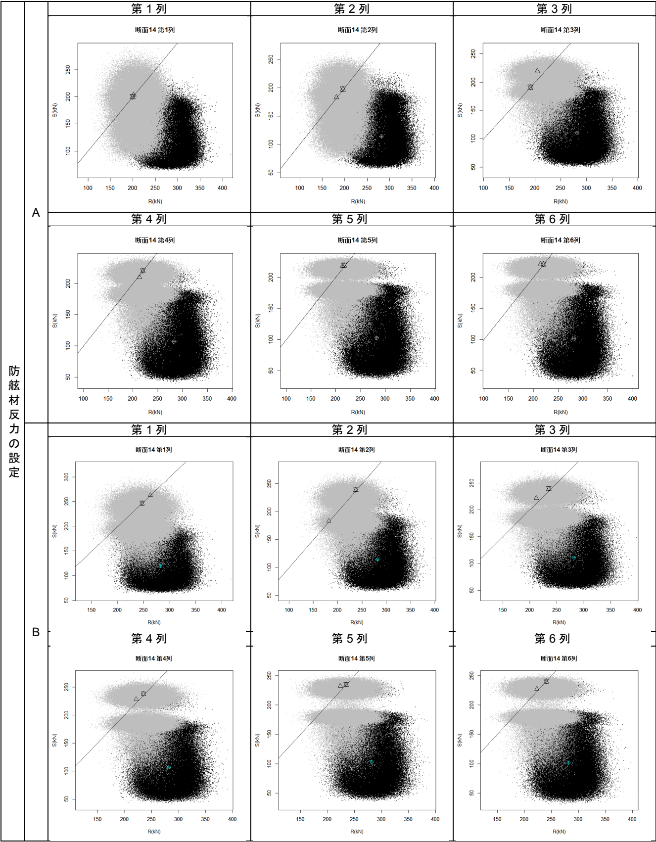
付表 F-26 杭列毎の抵抗-作用分布図(断面⑭ 設定 A および設定 B)
