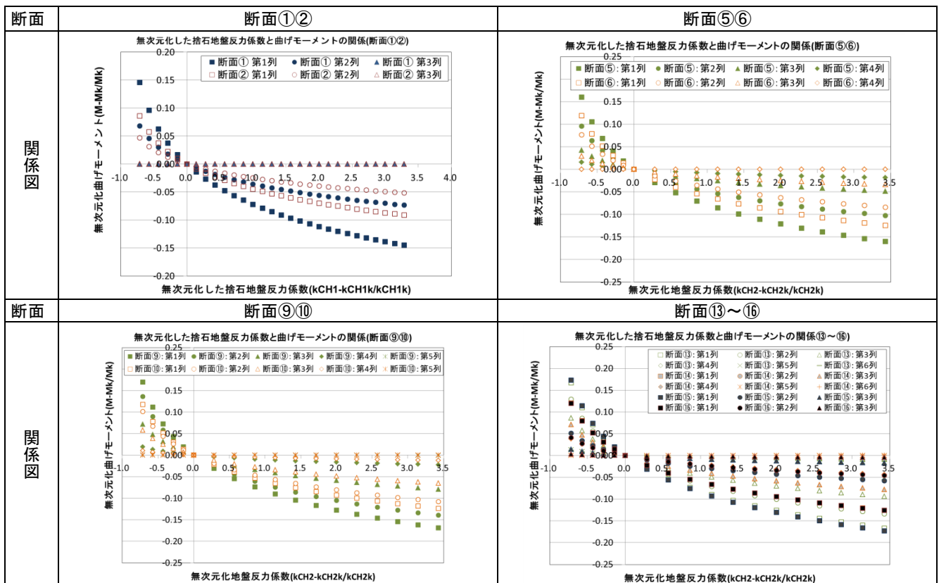
付表 B- 22 無次元化した捨石の地盤反力係数と曲げモーメントの関係
