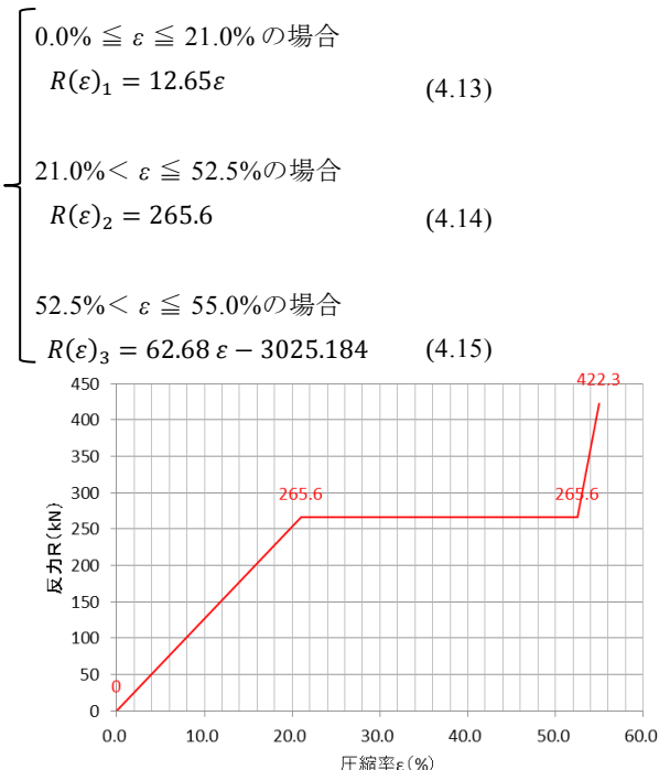
図-28 直線化した反力 R - 圧縮率 \varepsilon の関係式 R(\varepsilon)
