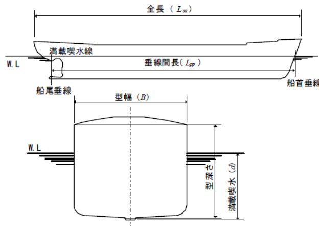
付図 D-5 船舶寸法の名称
