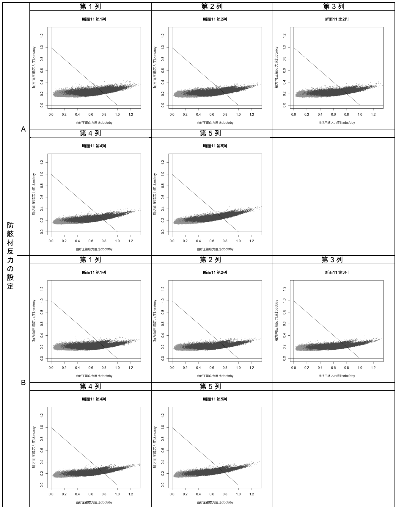
付表 F-42 杭列毎の曲げ圧縮応力度比-軸方向圧縮応力度比分布図(断面⑪ 設定 A および設定 B)
