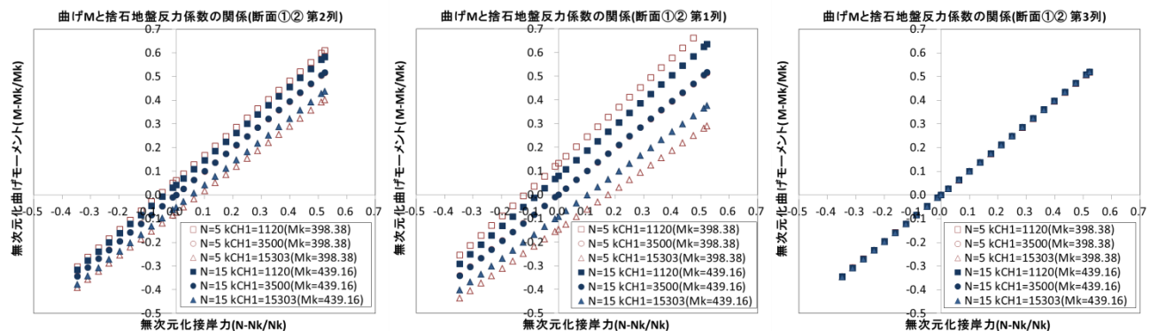
付図 B-6 接岸力の変化に対する無次元化した曲げモーメントと捨石地盤反力係数の関係(断面①②)
