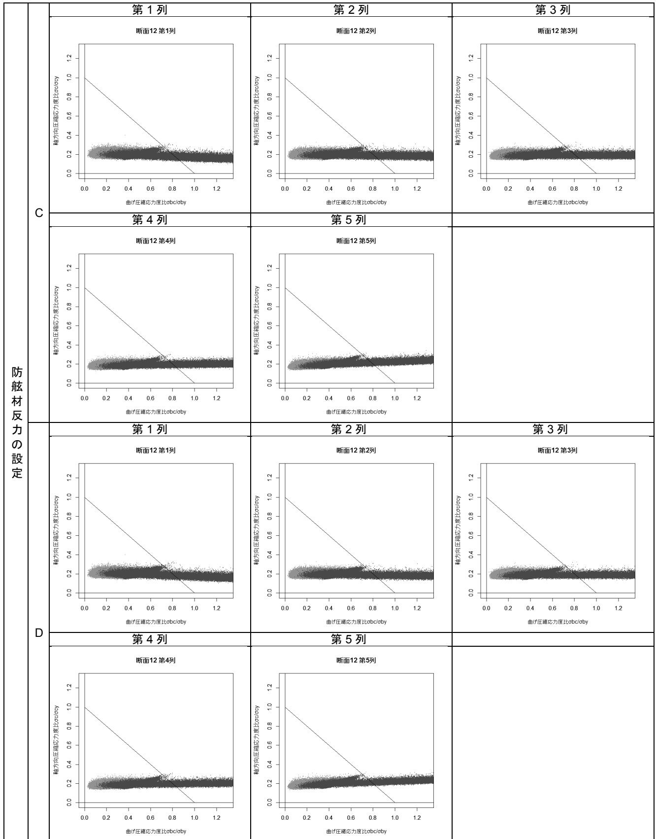
付表 F-45 杭列毎の曲げ圧縮応力度比-軸方向圧縮応力度比分布図(断面⑫ 設定 C および 設定 D)
