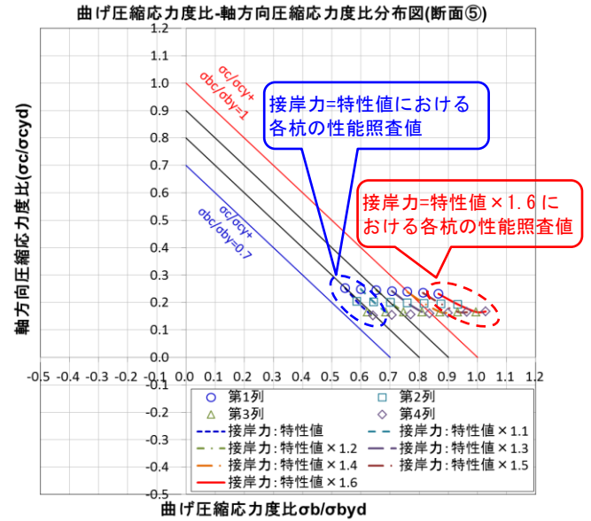
図-9 曲げ圧縮応力度比-軸方向圧縮応力度比分布図
