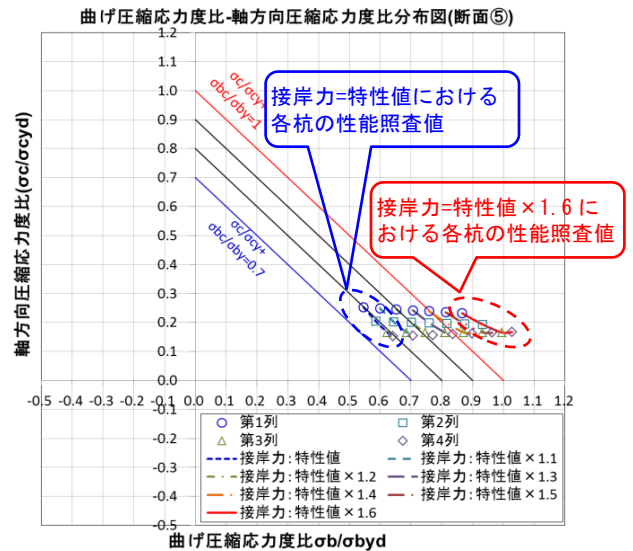
付図 C-1 圧縮応力度比分布図(断面⑤：海底勾配有り)
