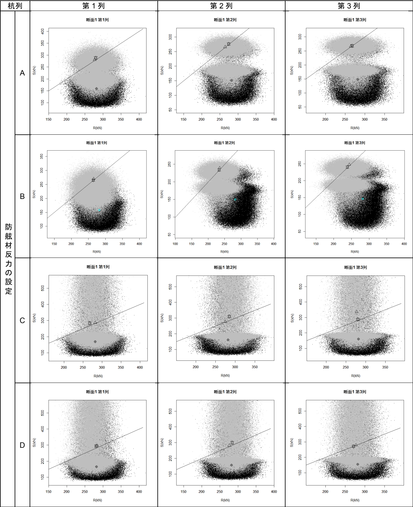
付表 F-8 杭列毎の抵抗-作用分布図(断面①)
