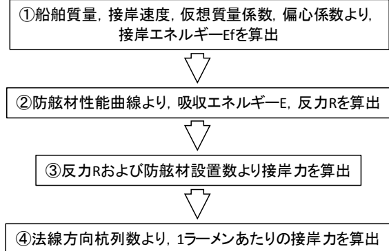
図-13 接岸力の算出過程
