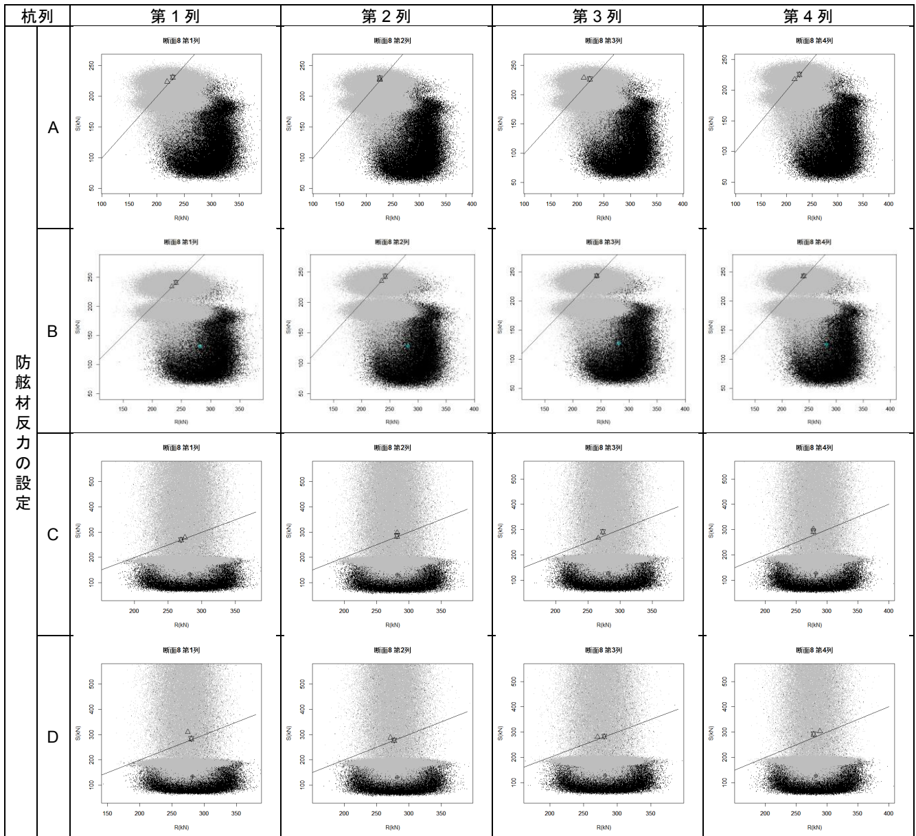
付表 F-15 杭列毎の抵抗-作用分布図(断面⑧)
