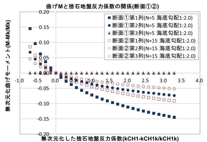
付図 B-5 無次元化した捨石地盤反力係数の変化に対する曲げモーメントの推移(断面①②)
