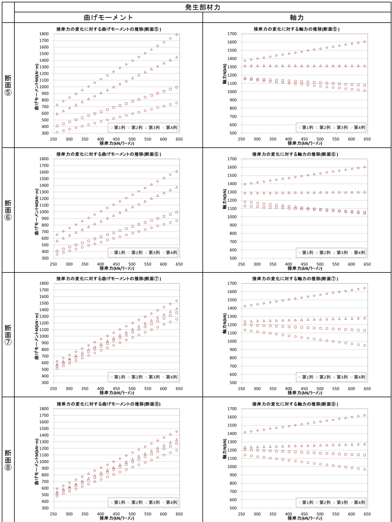
付表 B-12 接岸力の変化に対する近似式出力値の推移(断面⑤～⑧)
