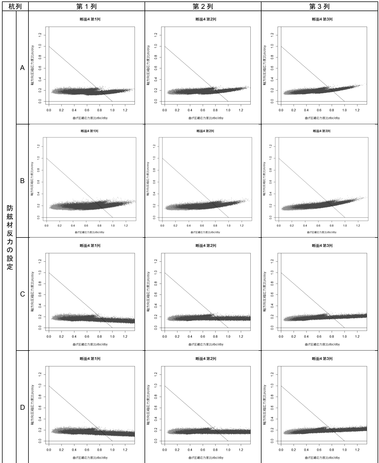
付表 F-33 杭列毎の曲げ圧縮応力度比-軸方向圧縮応力度比分布図(断面④)
