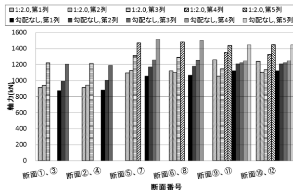
付図 A-4 海底勾配に対する軸力の比較
