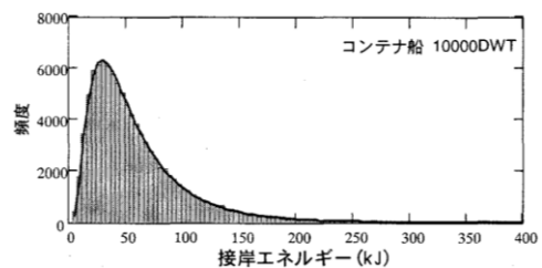
付図 D-1 MCS による接岸エネルギーの確率分布
