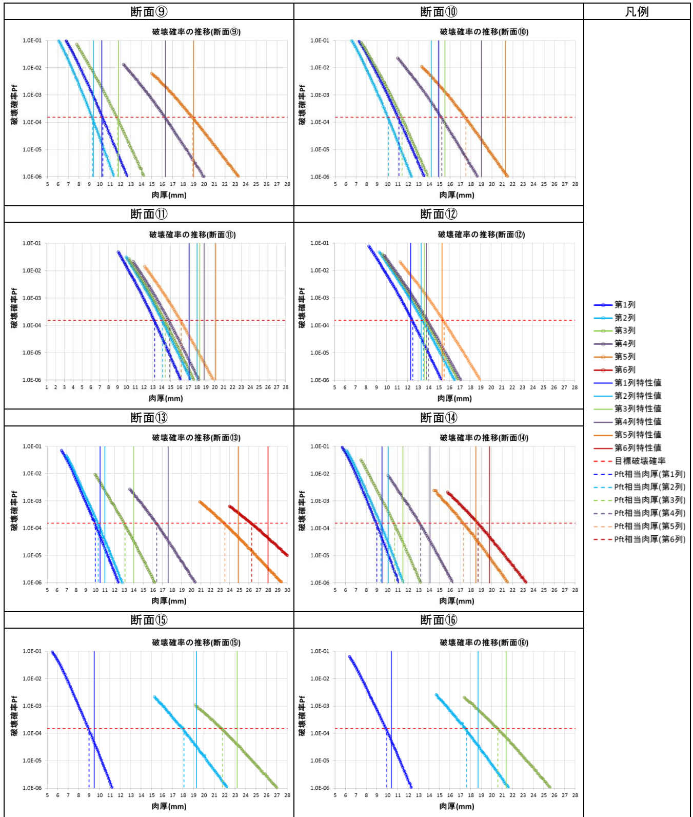
付表 G-5 肉厚ごとの破壊確率の推移と目標破壊確率相当の肉厚(断面⑨～⑯)
