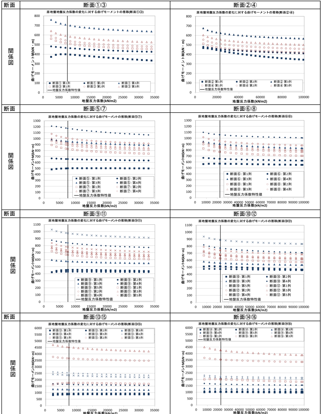
付表 B-15 原地盤の地盤反力係数の変化に対する曲げモーメントの推移
