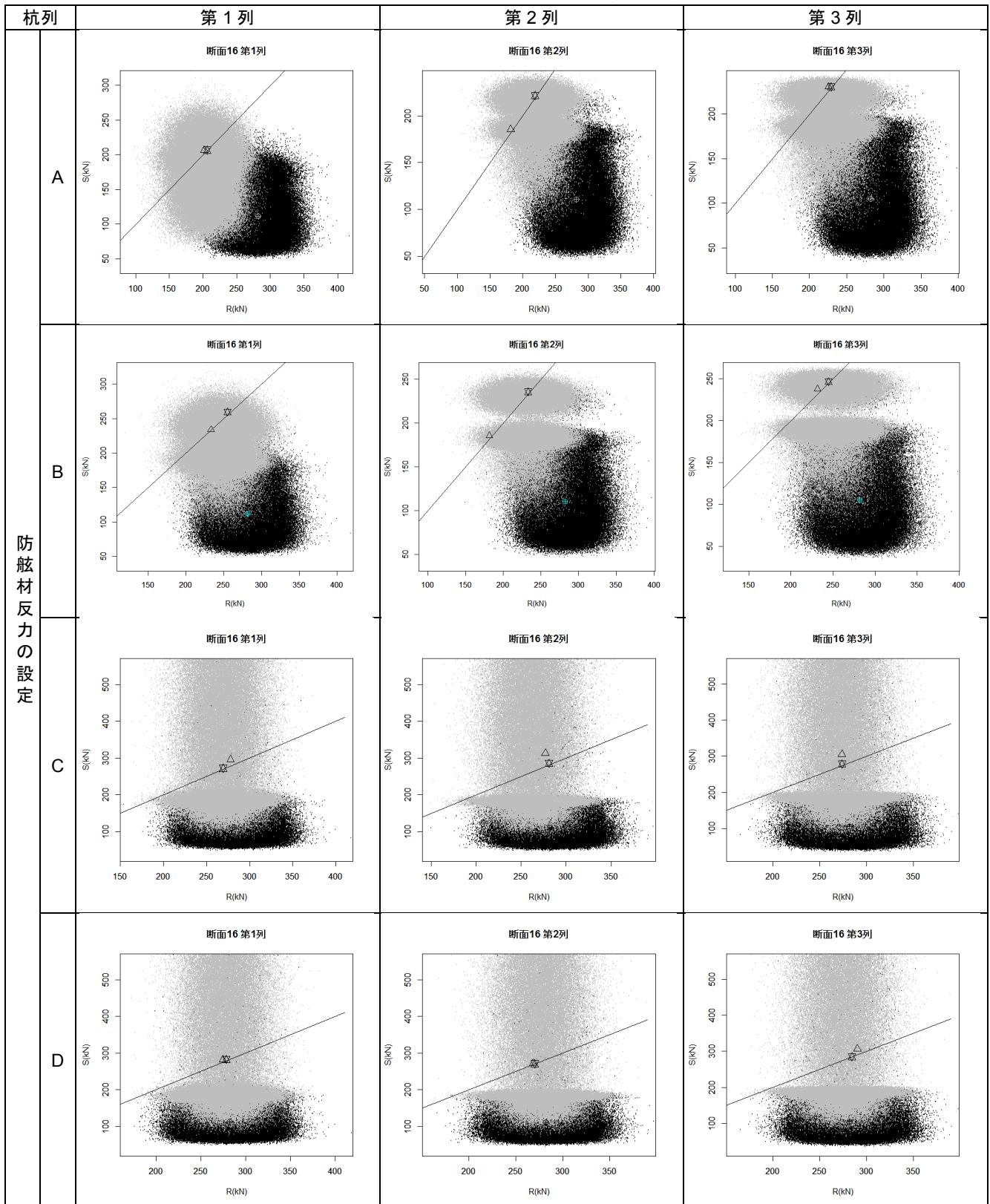
付表 F-29 杭列毎の抵抗-作用分布図(断面⑩)
