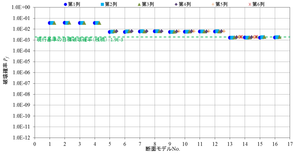
付図 F-9 各検討断面の破壊確率(設定 C)
