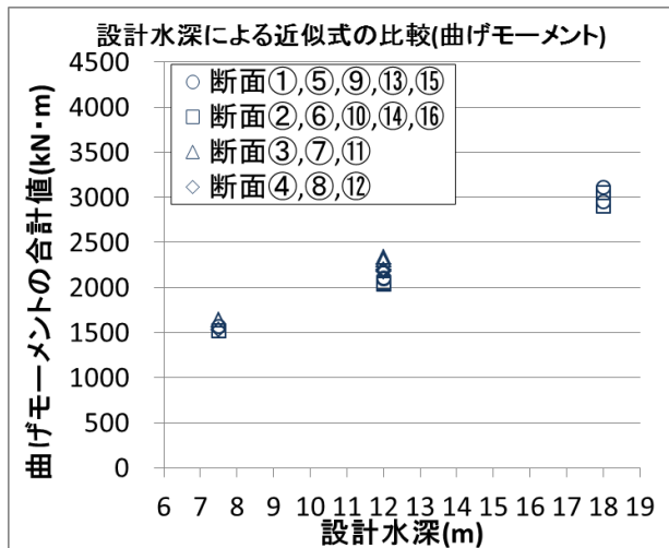
付図 A-7 設計水深に対する曲げモーメント合計値の比較
