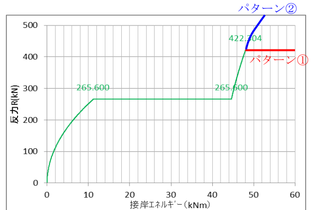
付図 F-2 限界圧縮率以降の反力特性の設定パターン
