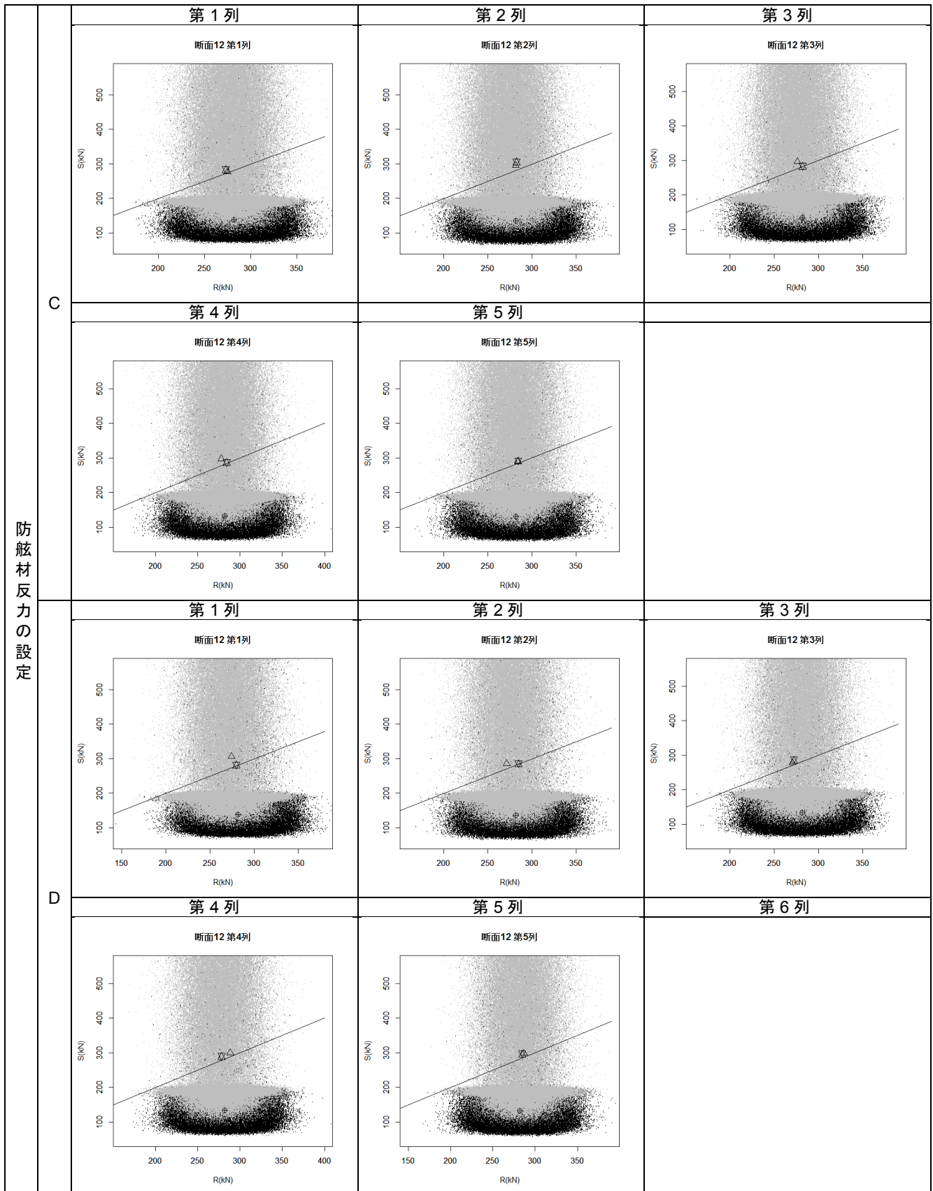
付表 F-23 杭列毎の抵抗-作用分布図(断面⑫ 設定 C および設定 D)
