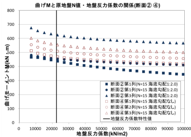
付図 B-2 原地盤の地盤反力係数の変化に対する 曲げモーメントの推移(断面②④, N=15)
