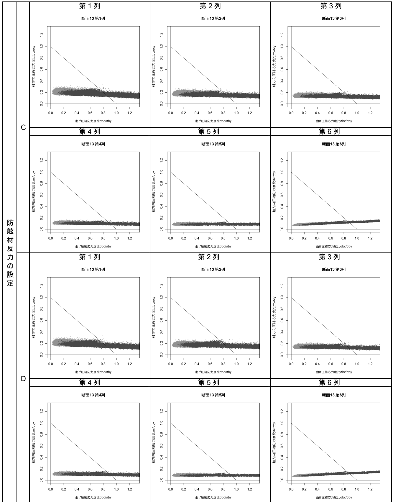
付表 F-47 杭列毎の曲げ圧縮応力度比-軸方向圧縮応力度比分布図(断面⑬ 設定 C および設定 D)
