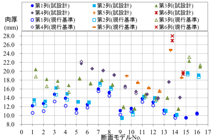
図-45 試設計および現行港湾基準での杭肉厚
