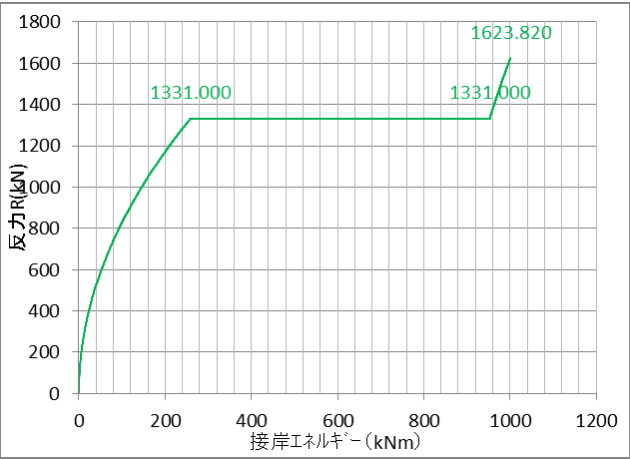
付図 E-6 モデル防舷材の接岸エネルギーと反力の関係
