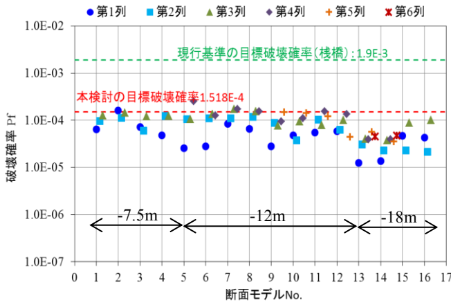
図-46 試設計断面の破壊確率
