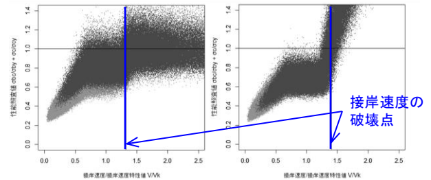
付図 F-17 接岸速度破壊点の変化(例：断面⑤第1列)
