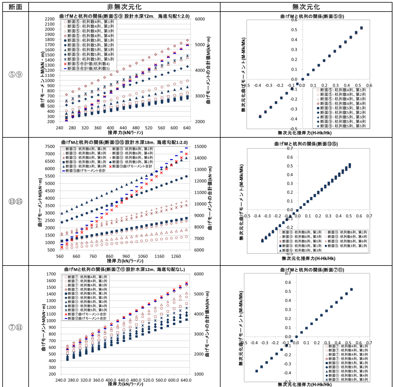
付表B-7 接岸力の変化に対する曲げモーメントと杭列の関係
