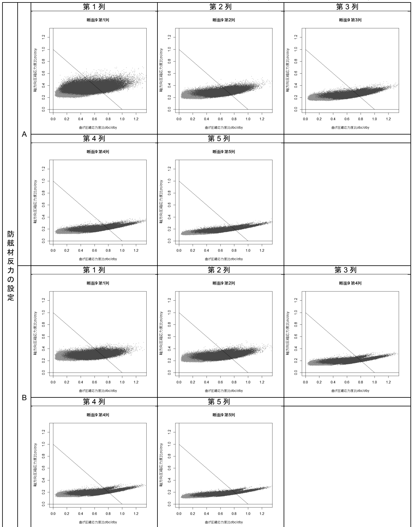
付表 F-38 杭列毎の曲げ圧縮応力度比-軸方向圧縮応力度比分布図(断面⑨ 設定 A および設定 B)
