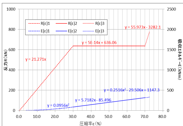
付図 E-3 モデル防舷材の性能曲線
