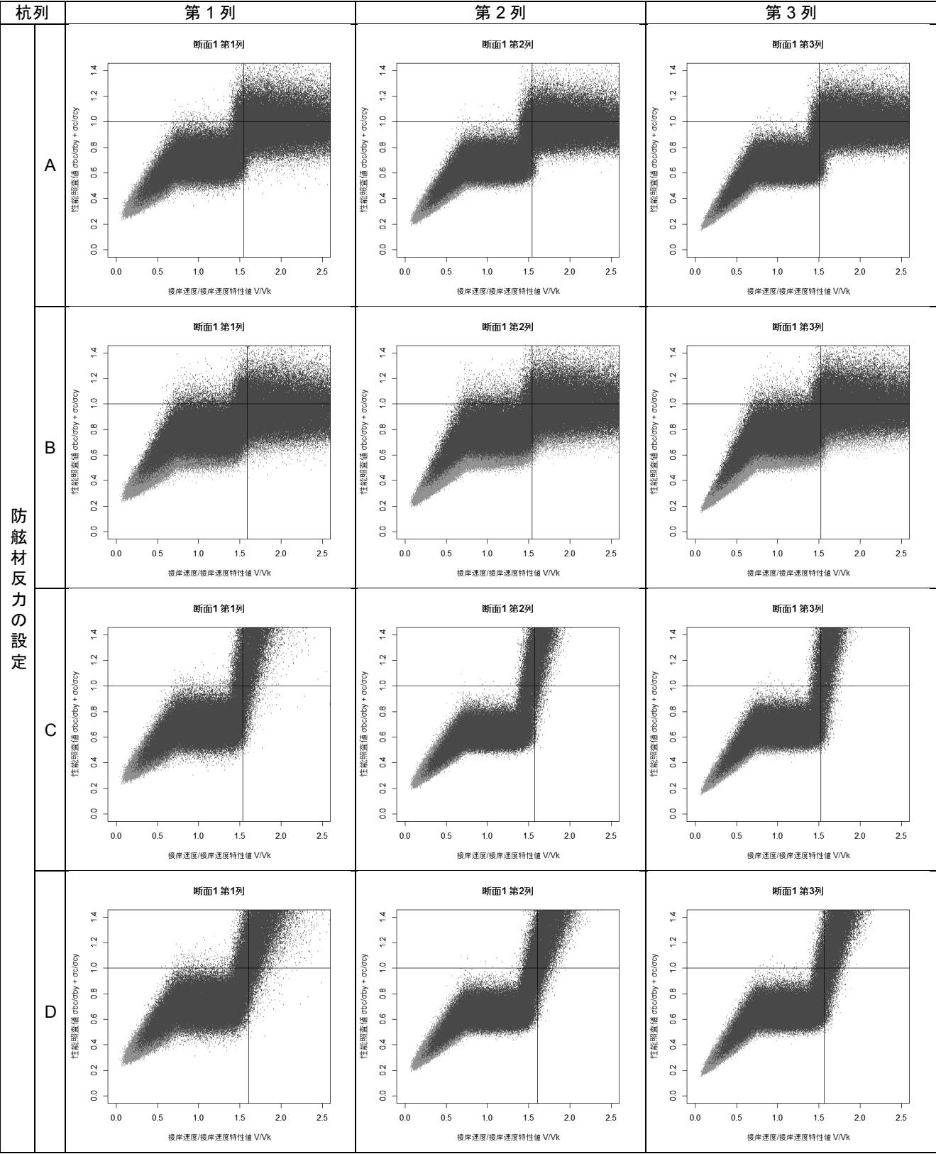
付表 F-52 接岸速度-性能照査値分布図(断面①)
