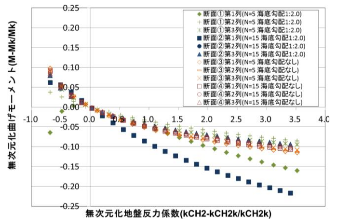
図-6 無次元化した原地盤の地盤反力係数の変化に対する曲げモーメントの推移(断面①～④)
