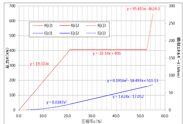
付図 E-1 モデル防舷材の性能曲線
