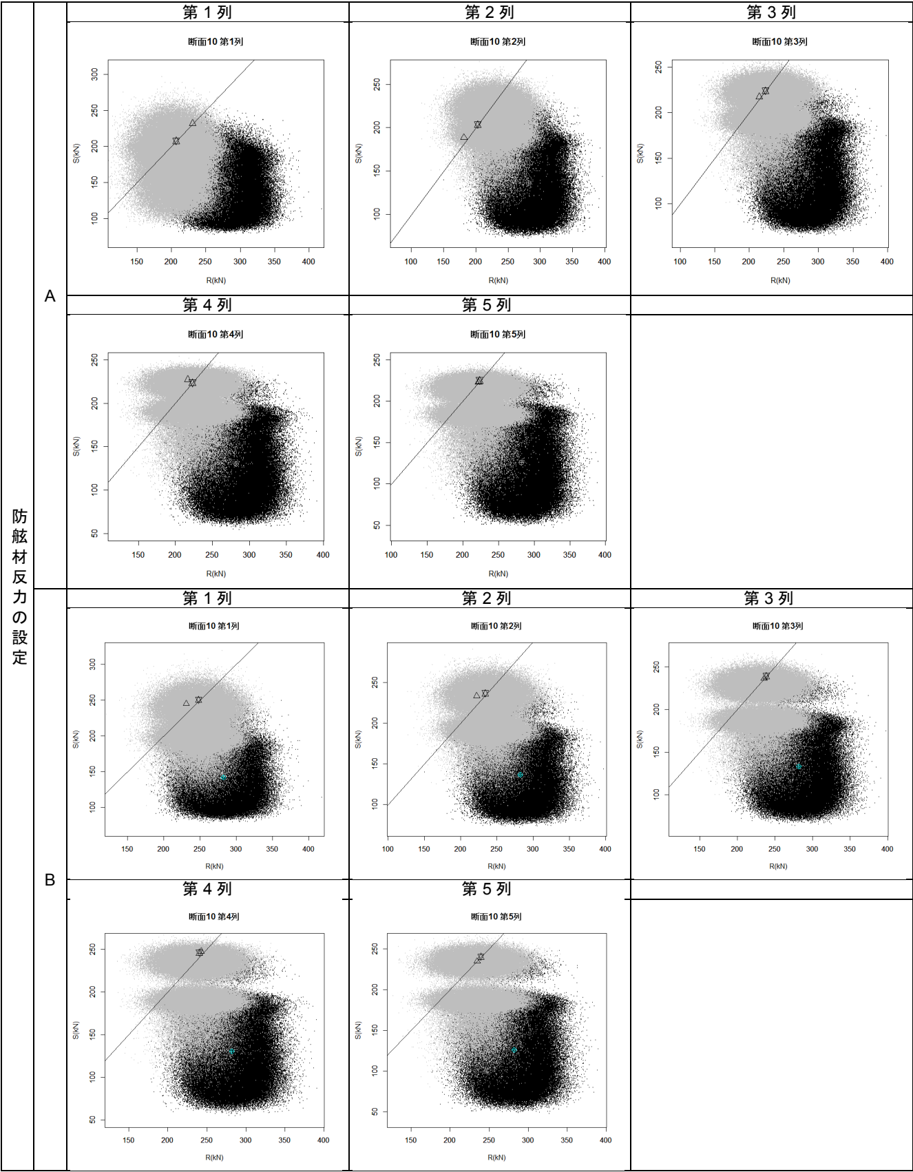
付表 F-18 杭列毎の抵抗-作用分布図(断面⑩ 設定 A および設定 B)
