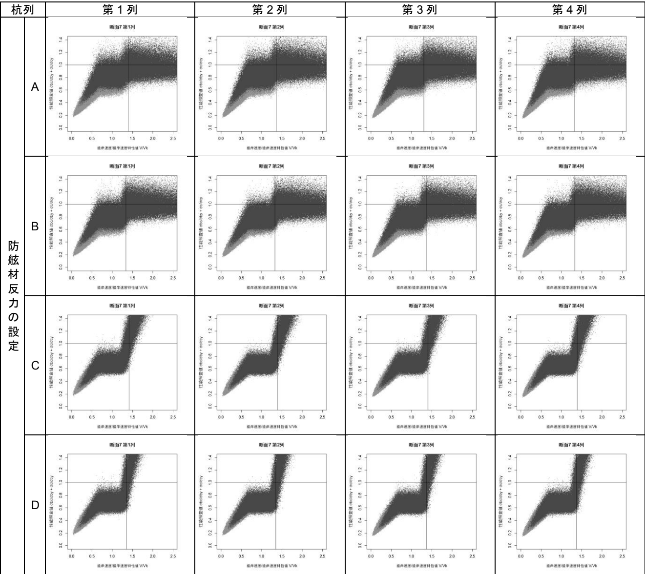
付表 F-58 接岸速度-性能照査値分布図(断面⑦)
