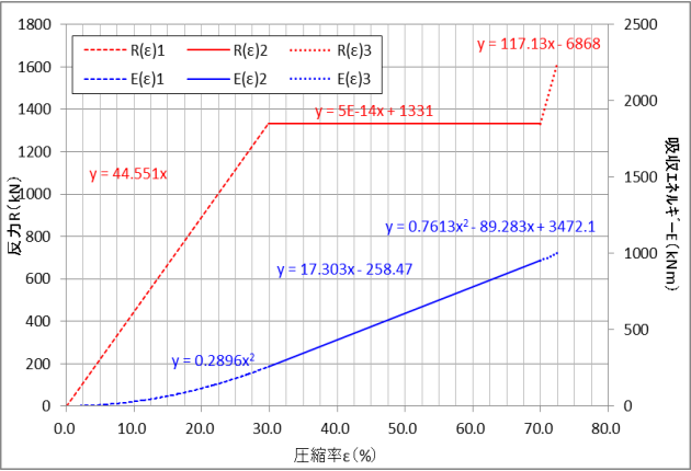
付図 E-5 モデル防舷材の性能曲線
