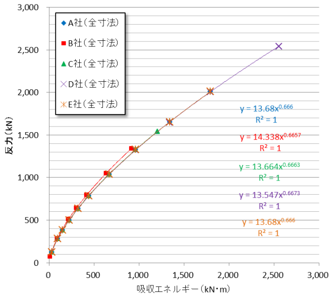
図-21 吸収エネルギーと反力の関係
