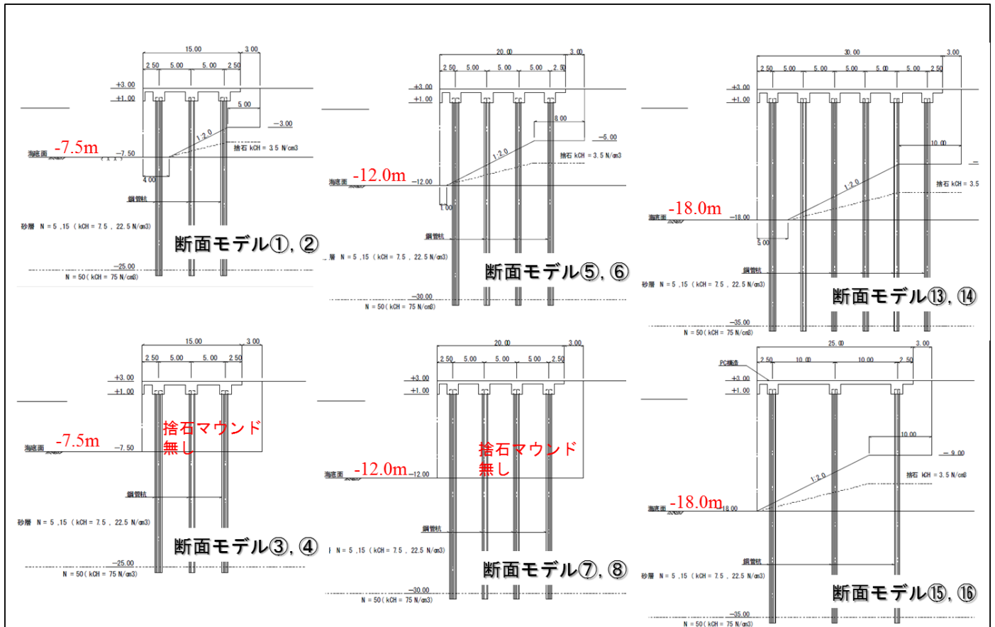
図-3 検討断面図
