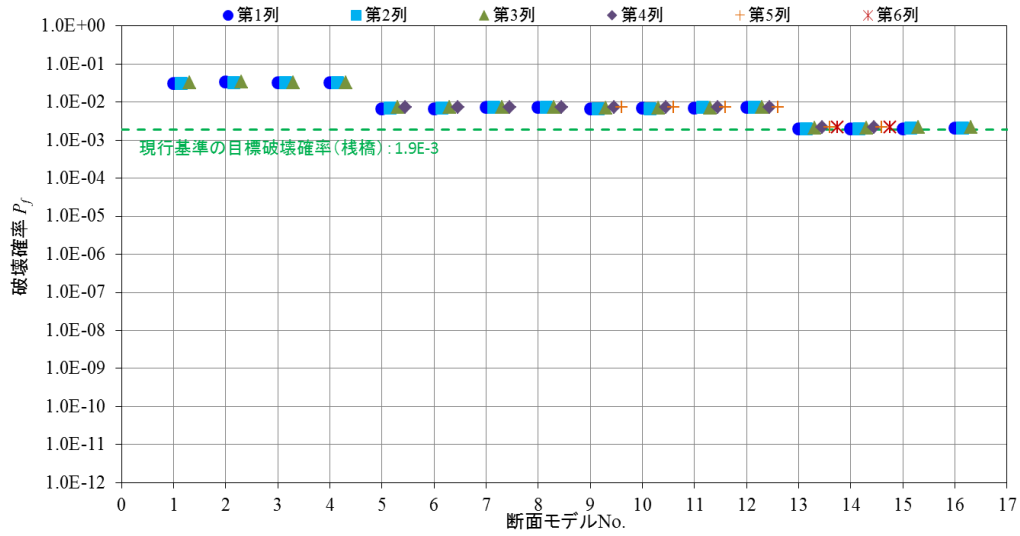
付図 F-12 各検討断面の破壊確率(設定 D)
