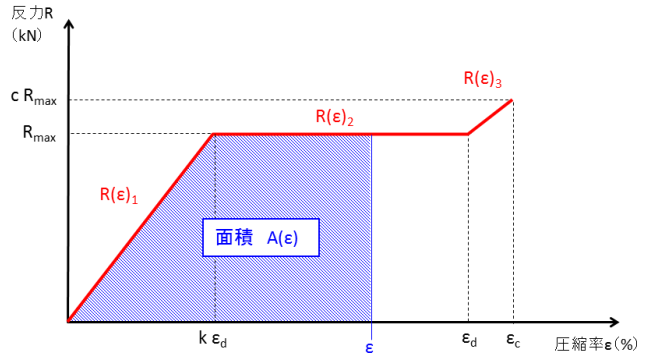
図-29 圧縮率 \varepsilon と面積 A(\varepsilon) の関係
