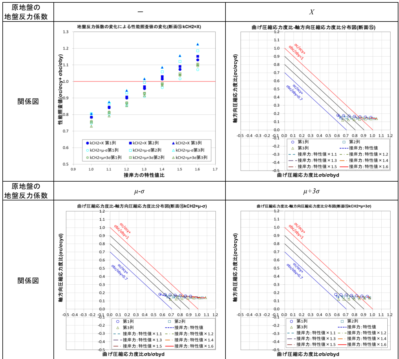
付表 C-9 接岸力および原地盤反力係数を変化させた際の曲げ圧縮・軸方向圧縮応力度比分布図(断面⑮)
