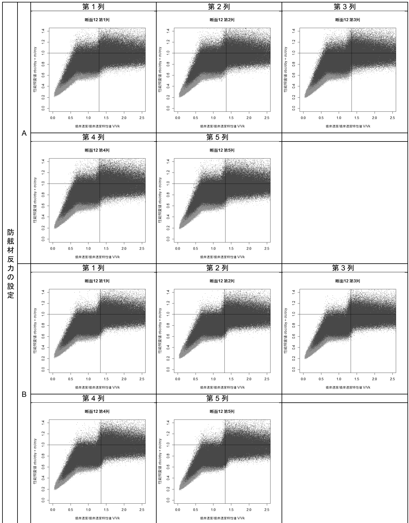
付表 F-66 接岸速度-性能照査値分布図(断面⑫ 設定 A および設定 B)
