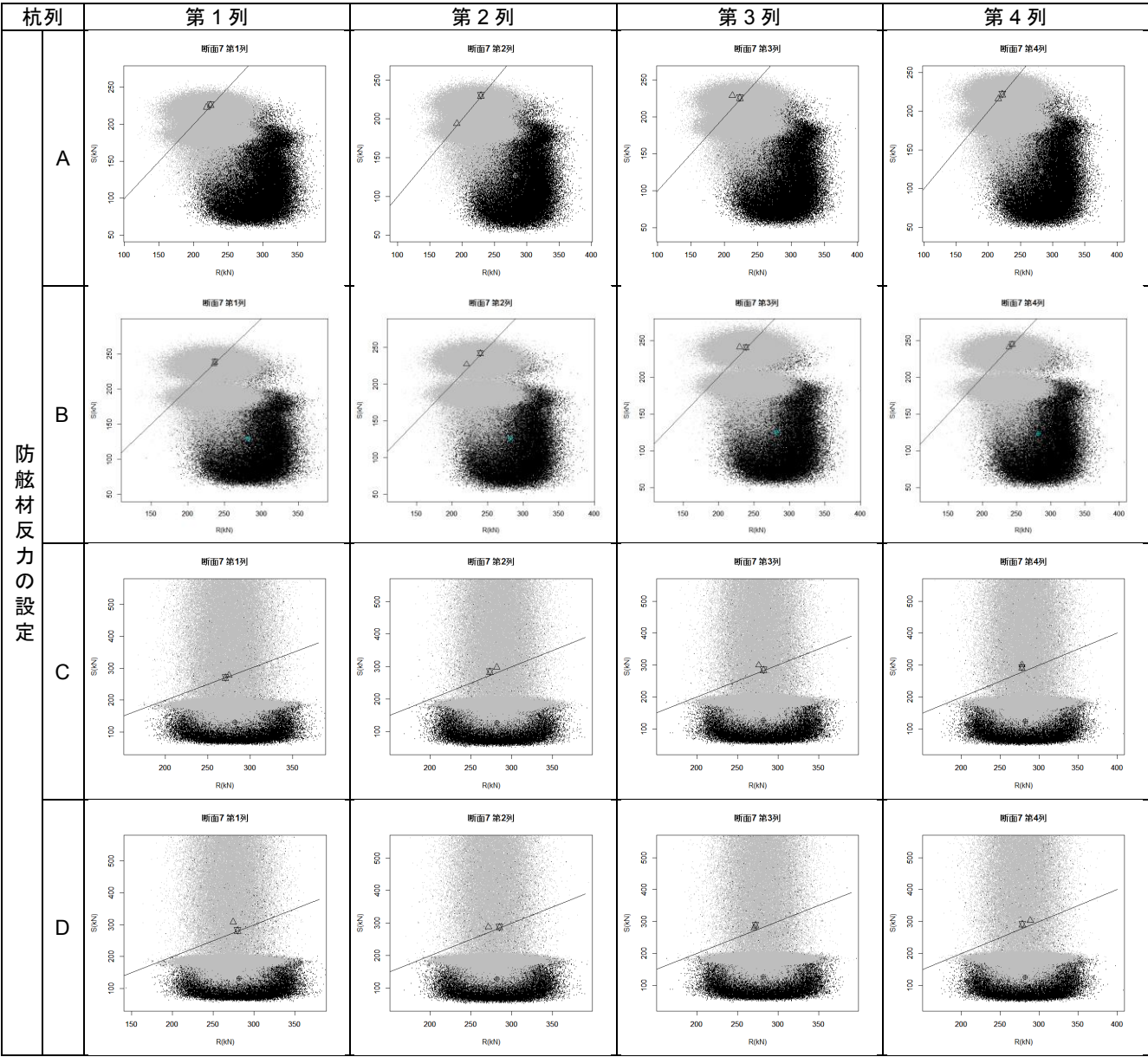
付表F-14 杭列毎の抵抗-作用分布図(断面⑦)
