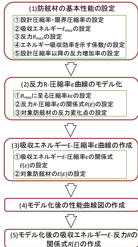
図-23 モデル防舷材の設定手順
