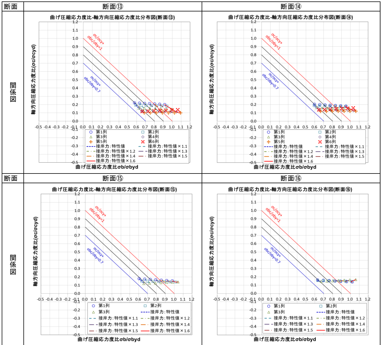
付表 C-8 接岸力を変化させた際の曲げ圧縮・軸方向圧縮応力度比分布図(断面⑬～⑯)
