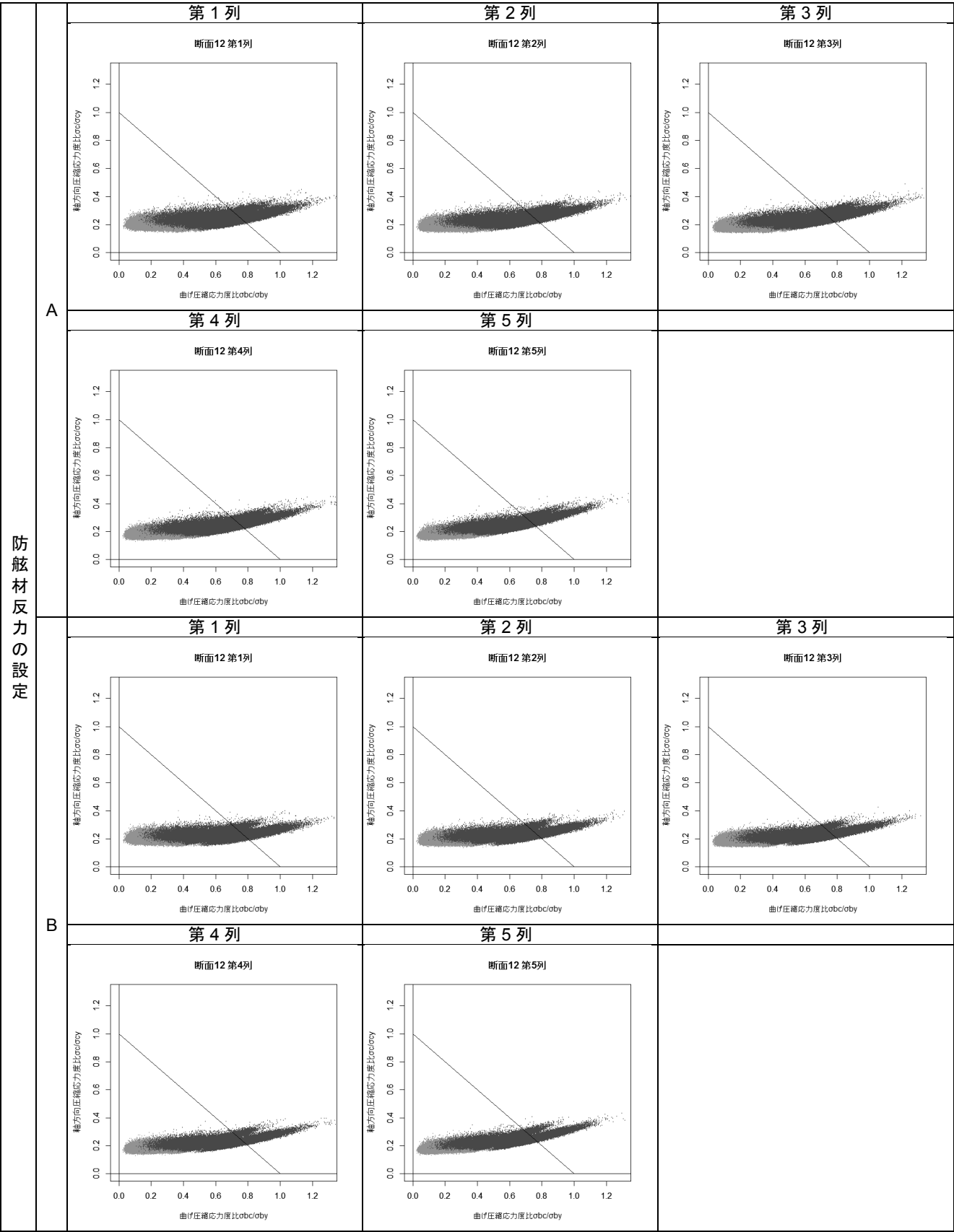
付表 F-44 杭列毎の曲げ圧縮応力度比-軸方向圧縮応力度比分布図(断面⑫ 設定 A および設定 B)
