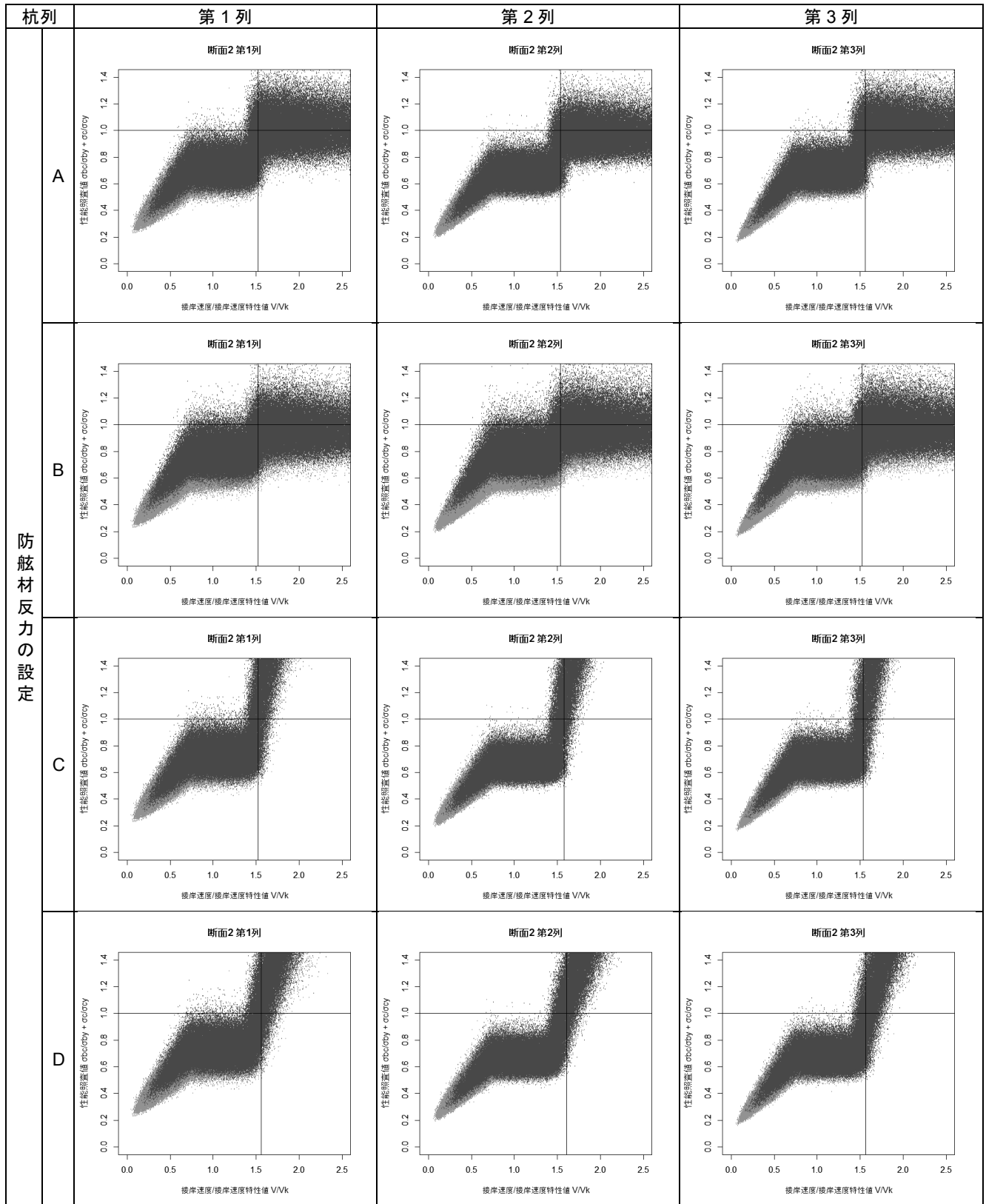
付表 F-53 接岸速度-性能照査値分布図(断面②)
