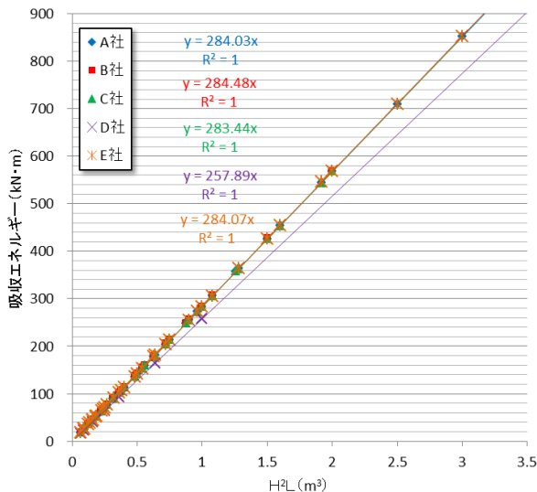
図-16 防舷材寸法ごとの吸収エネルギー(公表値)
