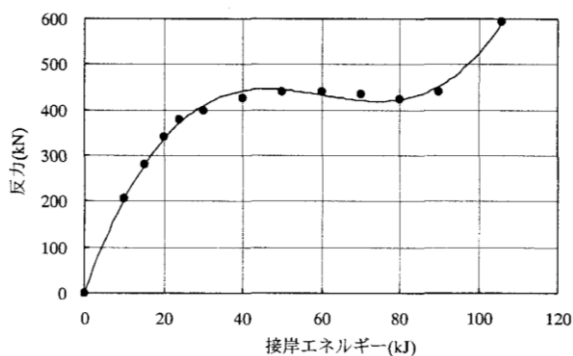
図-39 現行港湾基準検討時の防舷材反力特性
