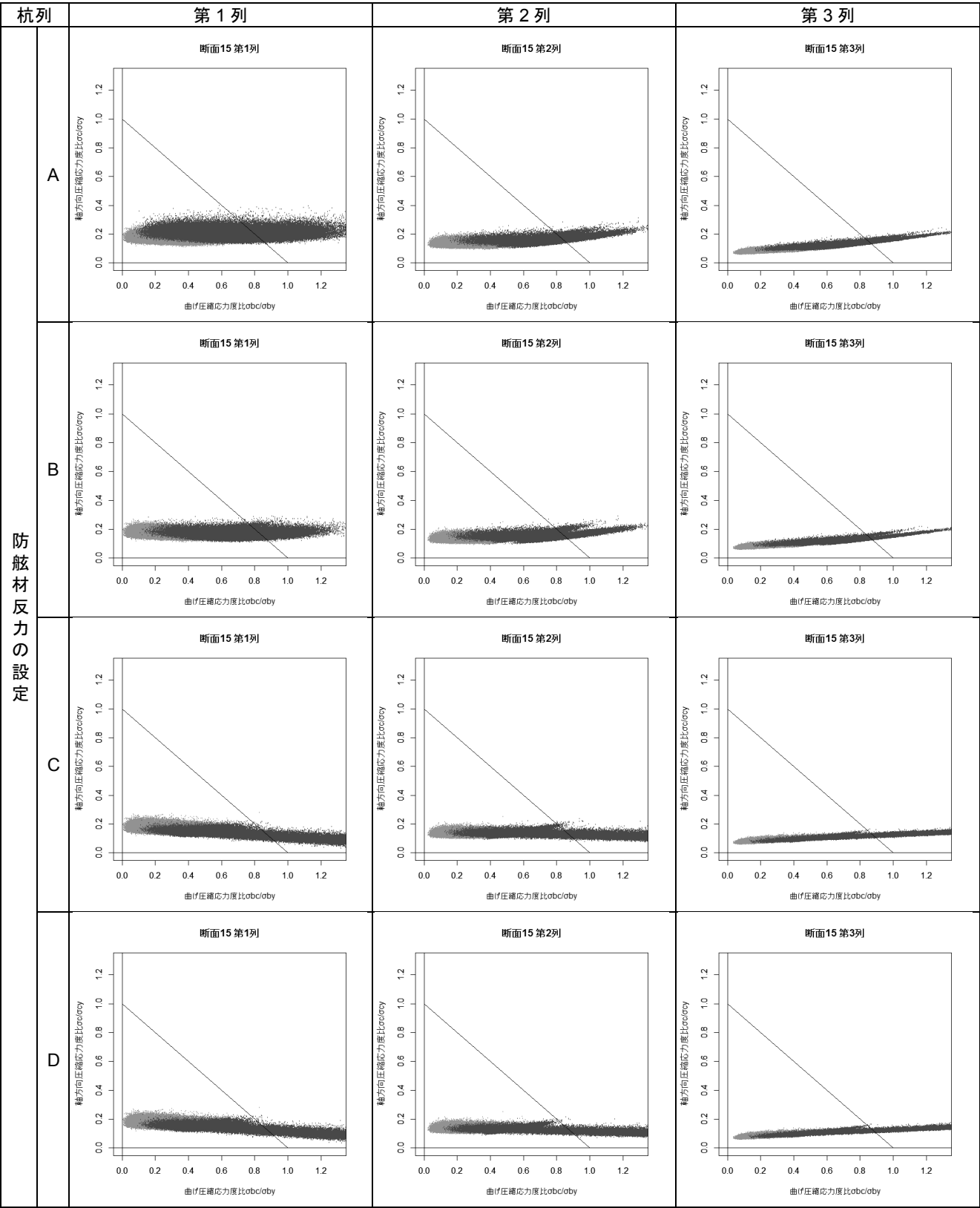
付表 F-50 杭列毎の曲げ圧縮応力度比-軸方向圧縮応力度比分布図(断面⑮)
