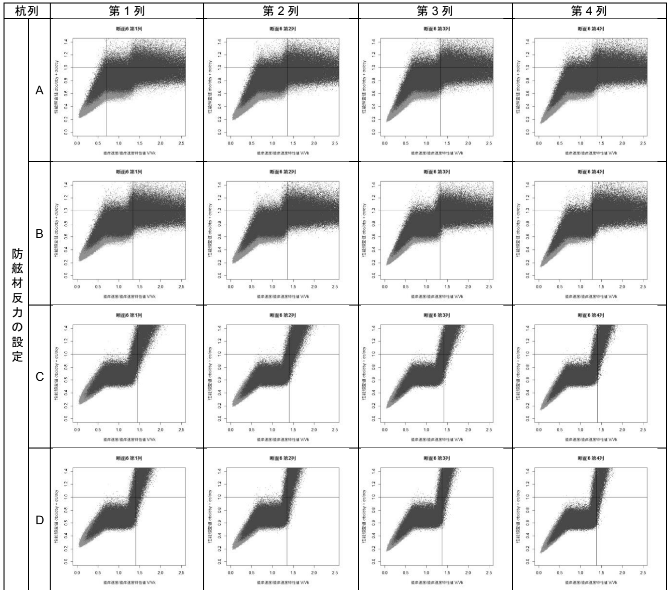
付表F-57 接岸速度-性能照査値分布図(断面⑥)
