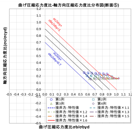
付図C-3 圧縮応力度比分布図(断面⑤：N=5)
