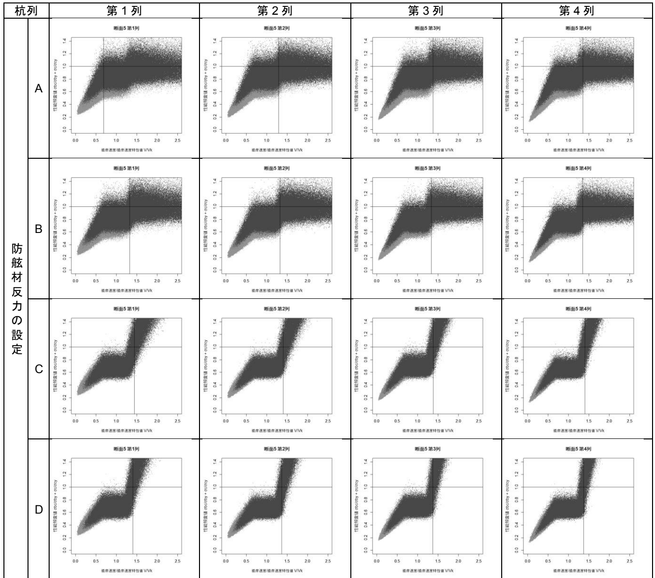
付表 F-56 接岸速度-性能照査値分布図(断面⑤)
