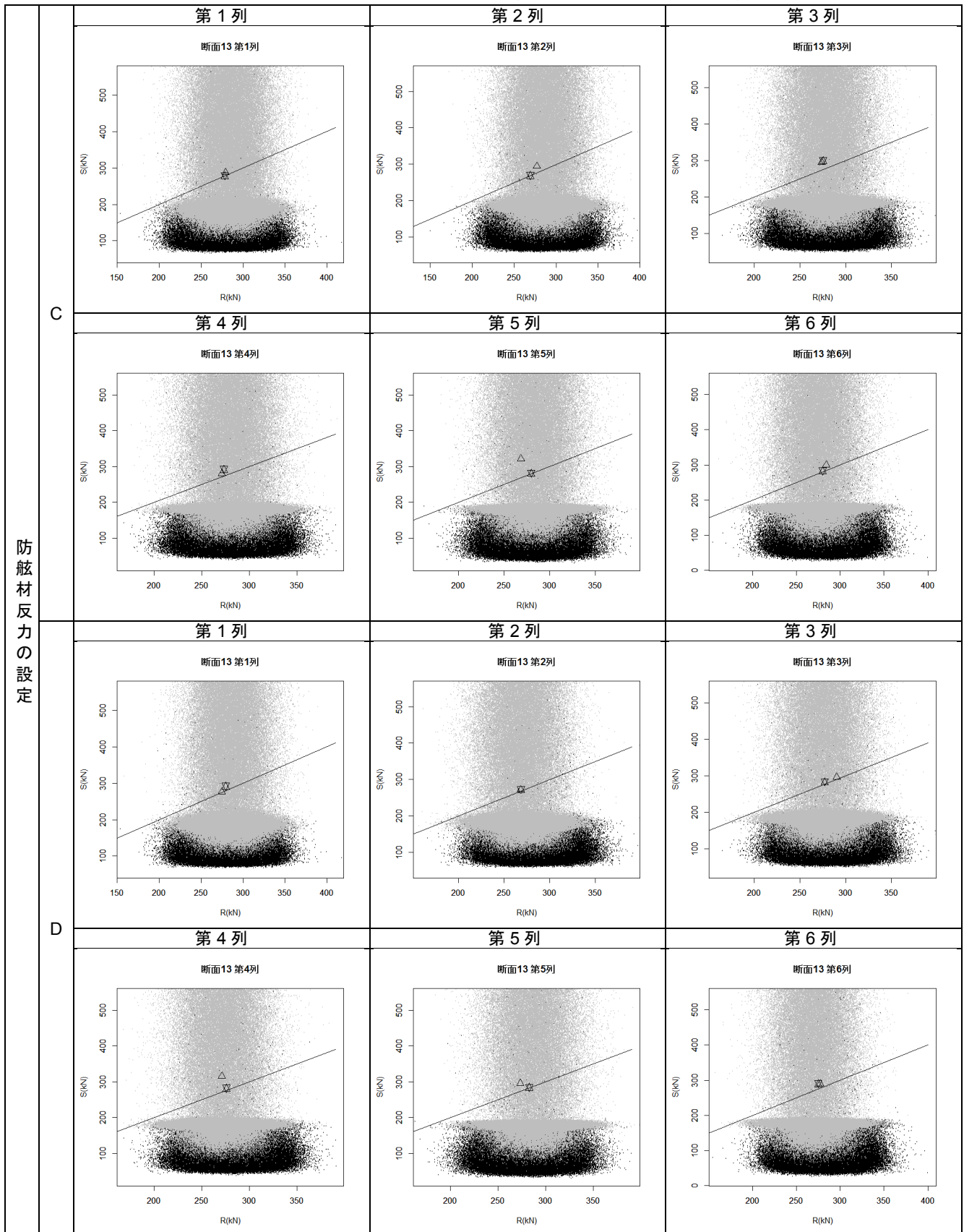
付表 F-25 杭列毎の抵抗-作用分布図(断面⑬ 設定 C および設定 D)
