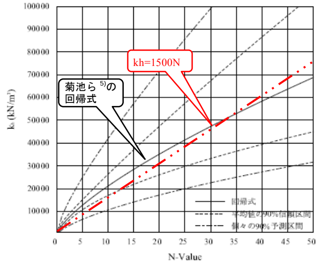
図-11 kh と N 値の回帰分析結果
