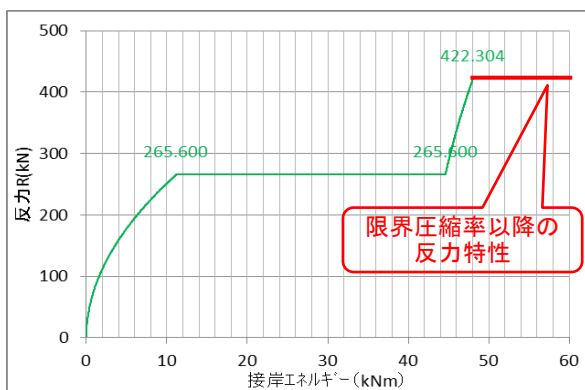
付図 F-1 限界圧縮率以降の反力特性の設定(本稿本文)
