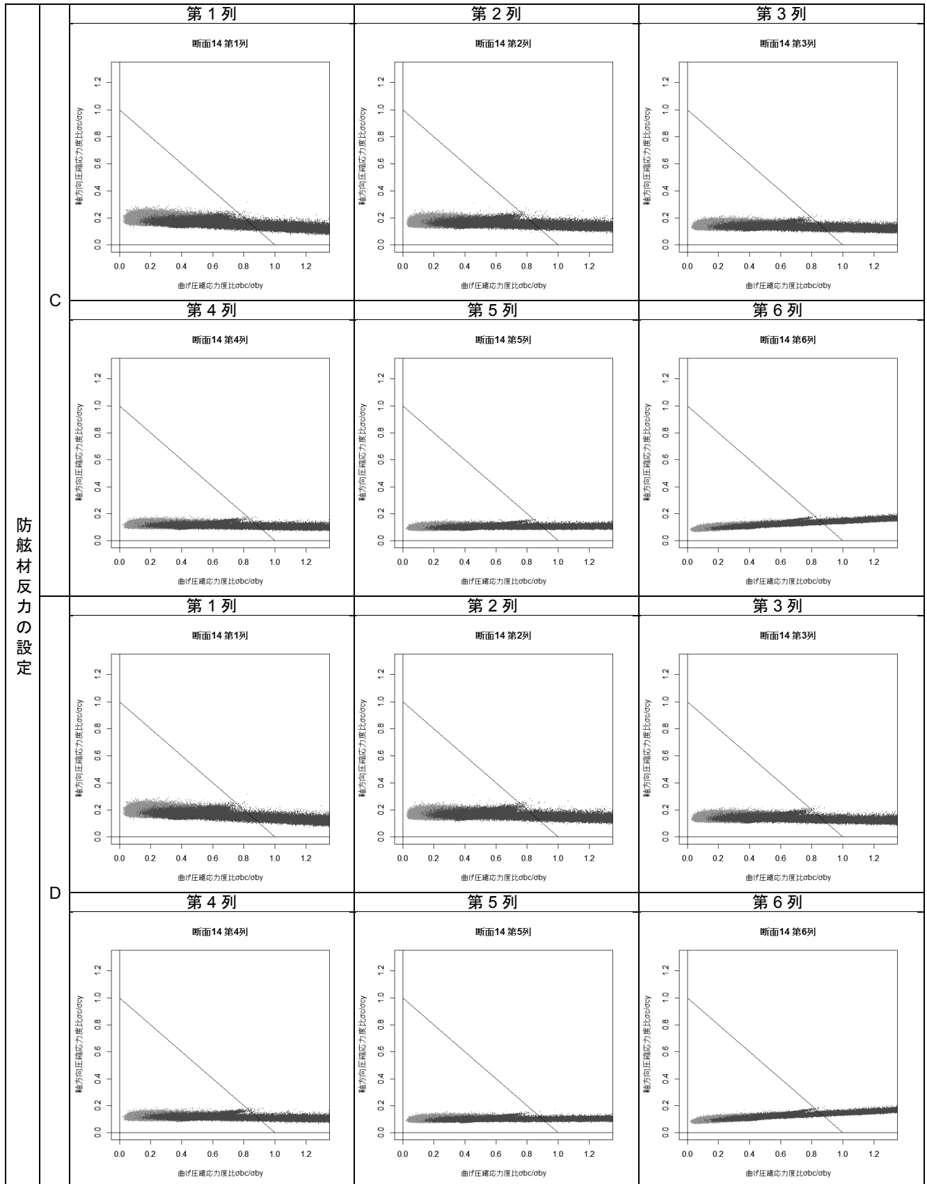
付表 F-49 杭列毎の曲げ圧縮応力度比-軸方向圧縮応力度比分布図(断面⑭ 設定 C および設定 D)
