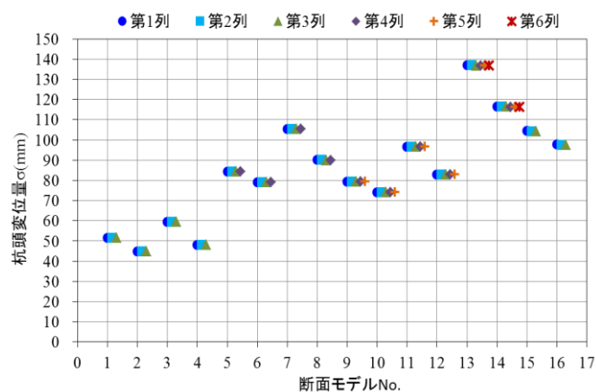
付図Ⅰ-1 試設計断面の杭頭変位量(船舶接岸時)
