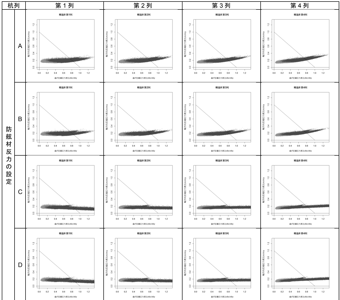
付表 F-37 杭列毎の曲げ圧縮応力度比-軸方向圧縮応力度比分布図(断面⑧)
