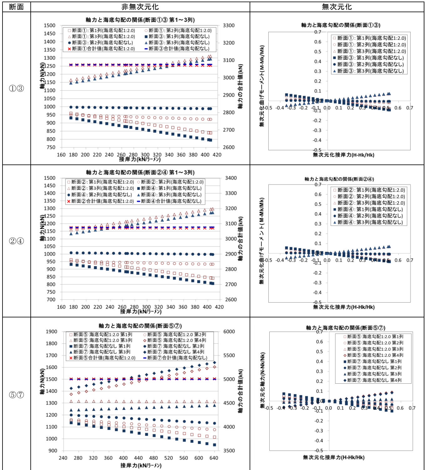
付表 B-6 接岸力の変化に対する軸力と海底勾配の関係
