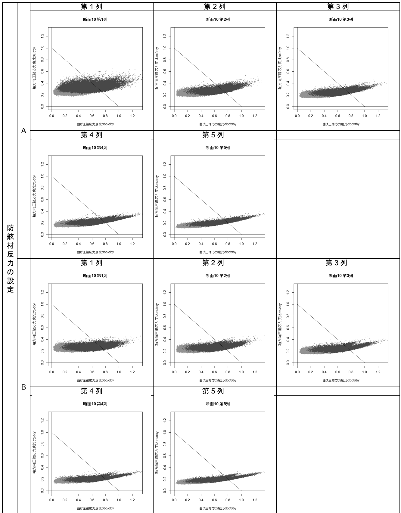
付表 F-40 杭列毎の曲げ圧縮応力度比-軸方向圧縮応力度比分布図(断面⑩ 設定 A および設定 B)
