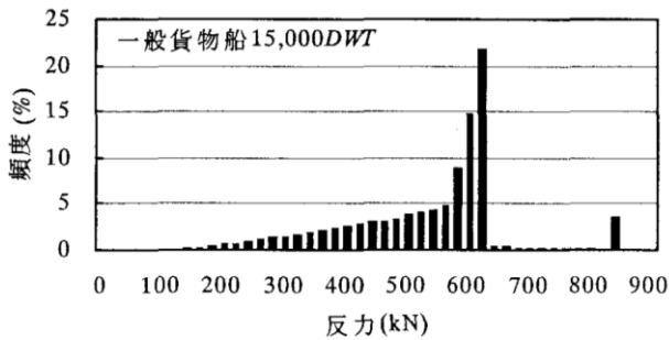
付図 D-2 防舷材反力の確率分布(貨物船, 15,000DWT)
