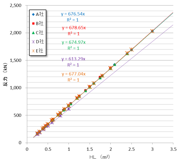
図-17 防舷材寸法ごとの反力(公表値)
