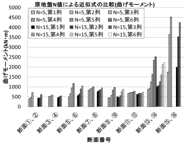
付図 A-1 N 値に対する曲げモーメントの比較
