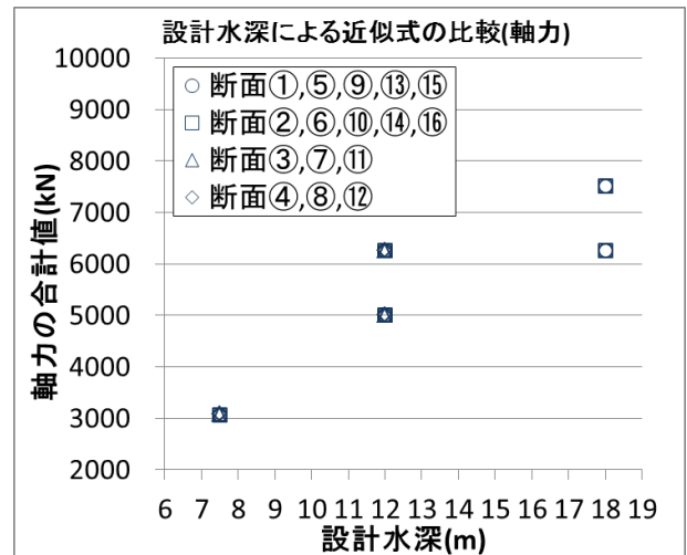
付図 A-8 設計水深に対する軸力合計値の比較
