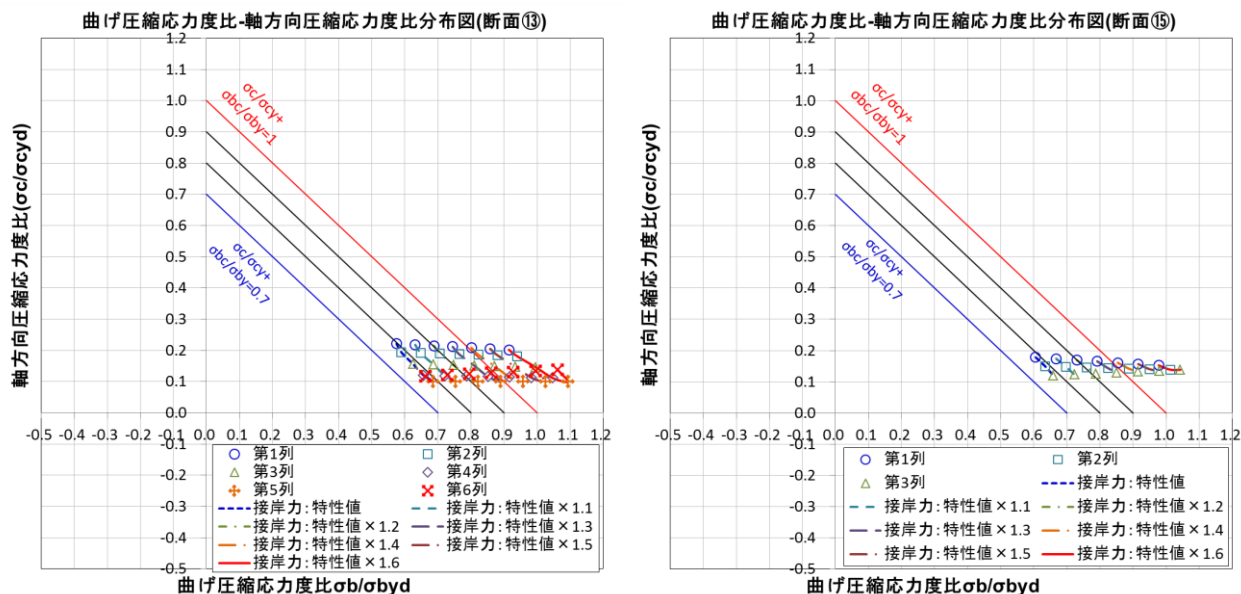
付図 C-6 曲げ圧縮・軸方向圧縮応力度比分布図(設計水深 18m：断面⑬(杭列数 6)，断面⑮(杭列数 3))
