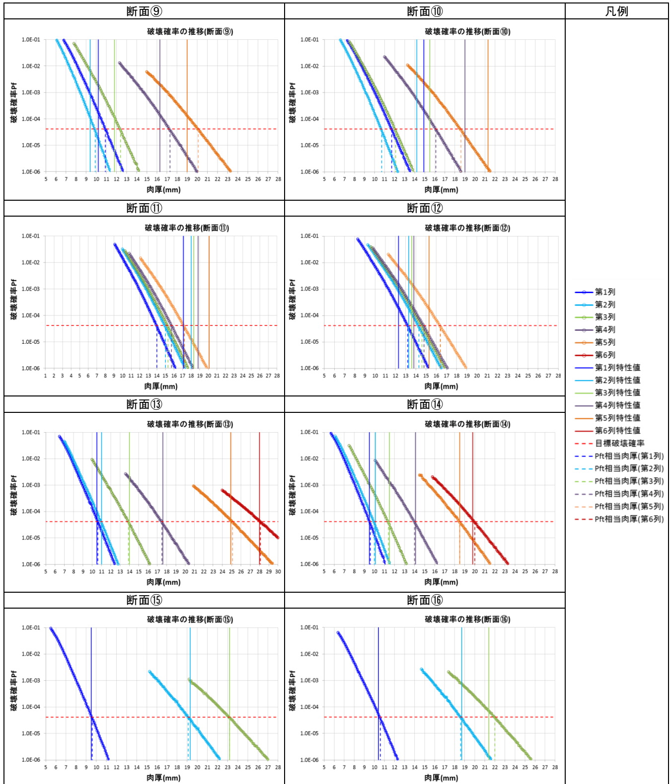
付表 G-7 肉厚ごとの破壊確率の推移と目標破壊確率相当の肉厚(断面⑨～⑯)
