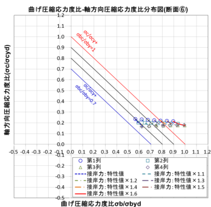
付図C-4 圧縮応力度比分布図(断面⑥：N=15)
