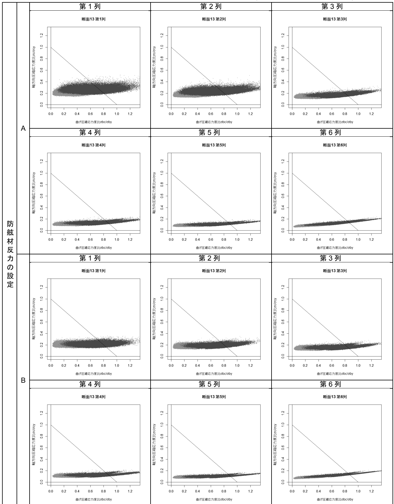
付表 F-46 杭列毎の曲げ圧縮応力度比-軸方向圧縮応力度比分布図(断面⑬ 設定 A および設定 B)
