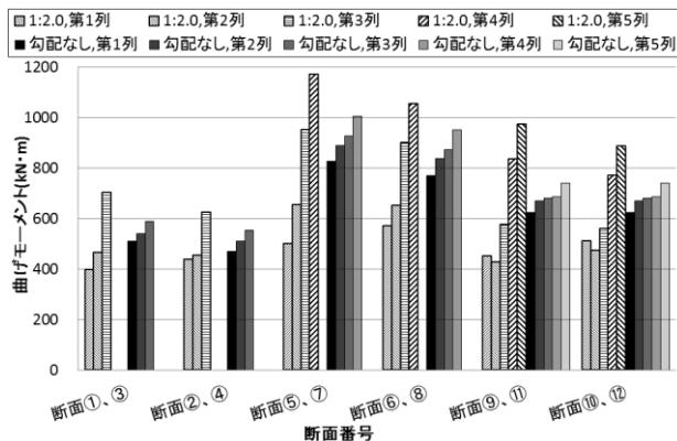
付図 A-3 海底勾配に対する曲げモーメントの比較
