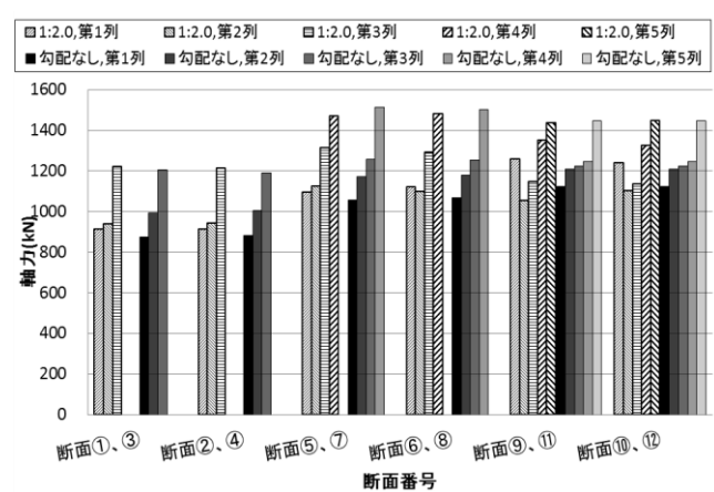
図-5 海底勾配に対する軸力の比較
