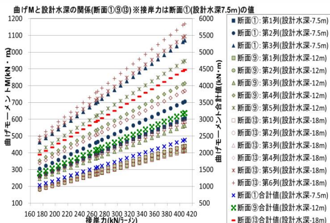
付図 B-8 接岸力の変化に対する曲げモーメントと設計水深の関係
