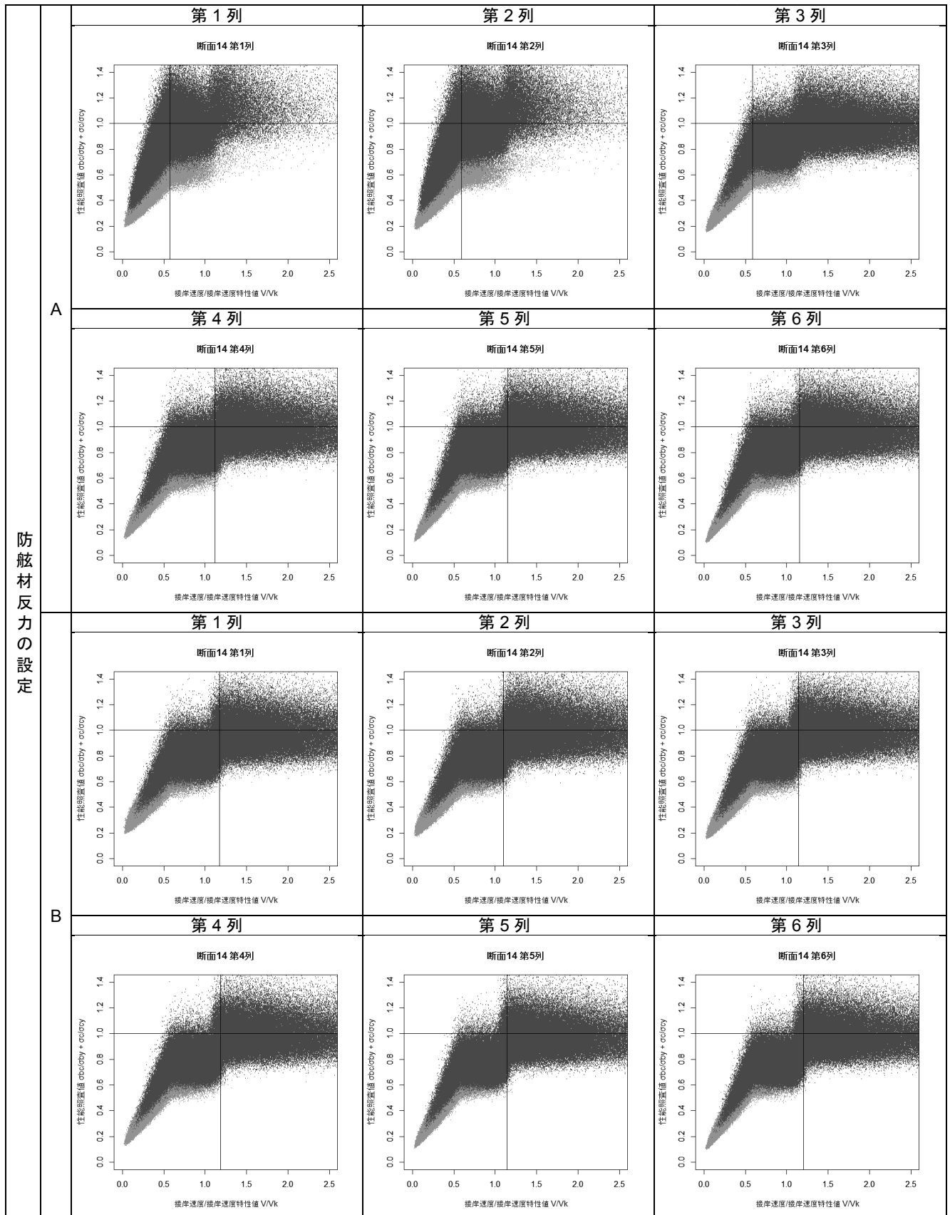
付表 F-70 接岸速度-性能照査値分布図(断面⑭ 設定 A および設定 B)
