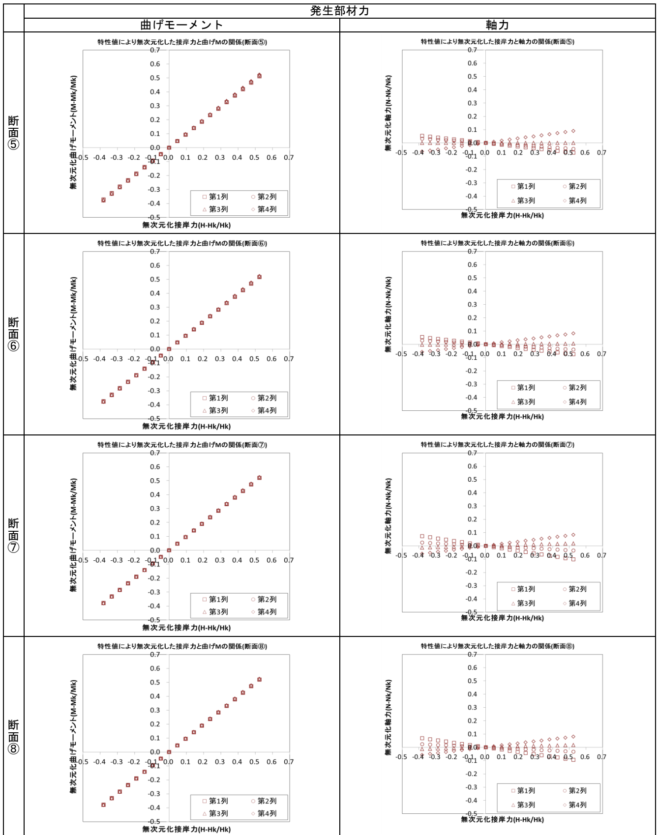
付表 B-18 無次元化した接岸力と出力値の関係(断面⑤～⑧)
