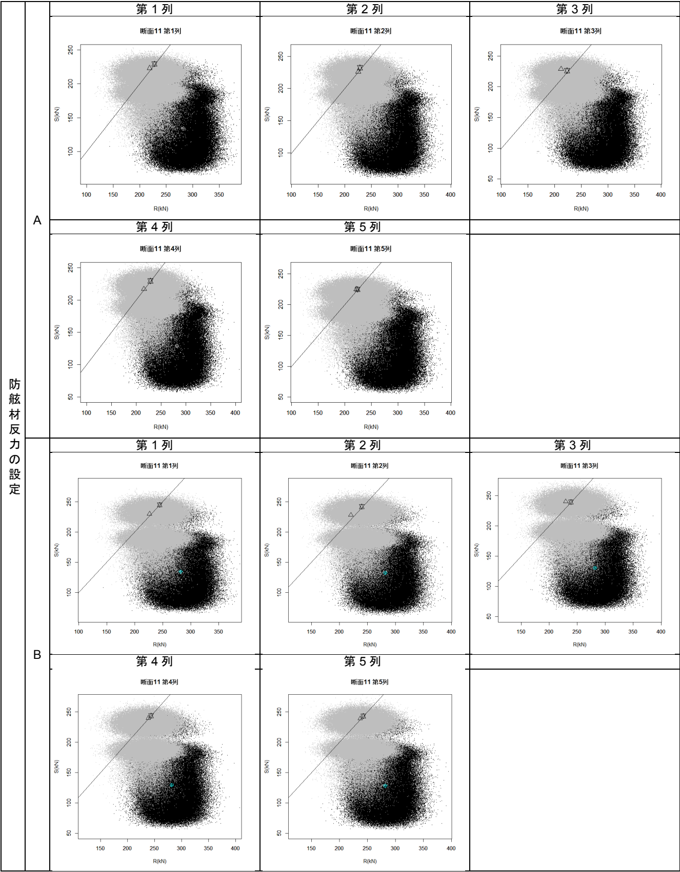
付表 F-20 杭列毎の抵抗-作用分布図(断面⑪ 設定 A および設定 B)
