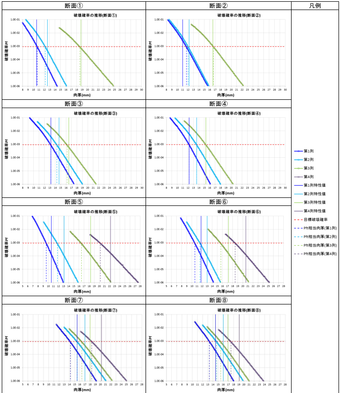
付表 G-2 肉厚ごとの破壊確率の推移と目標破壊確率相当の肉厚(断面①～⑧)
