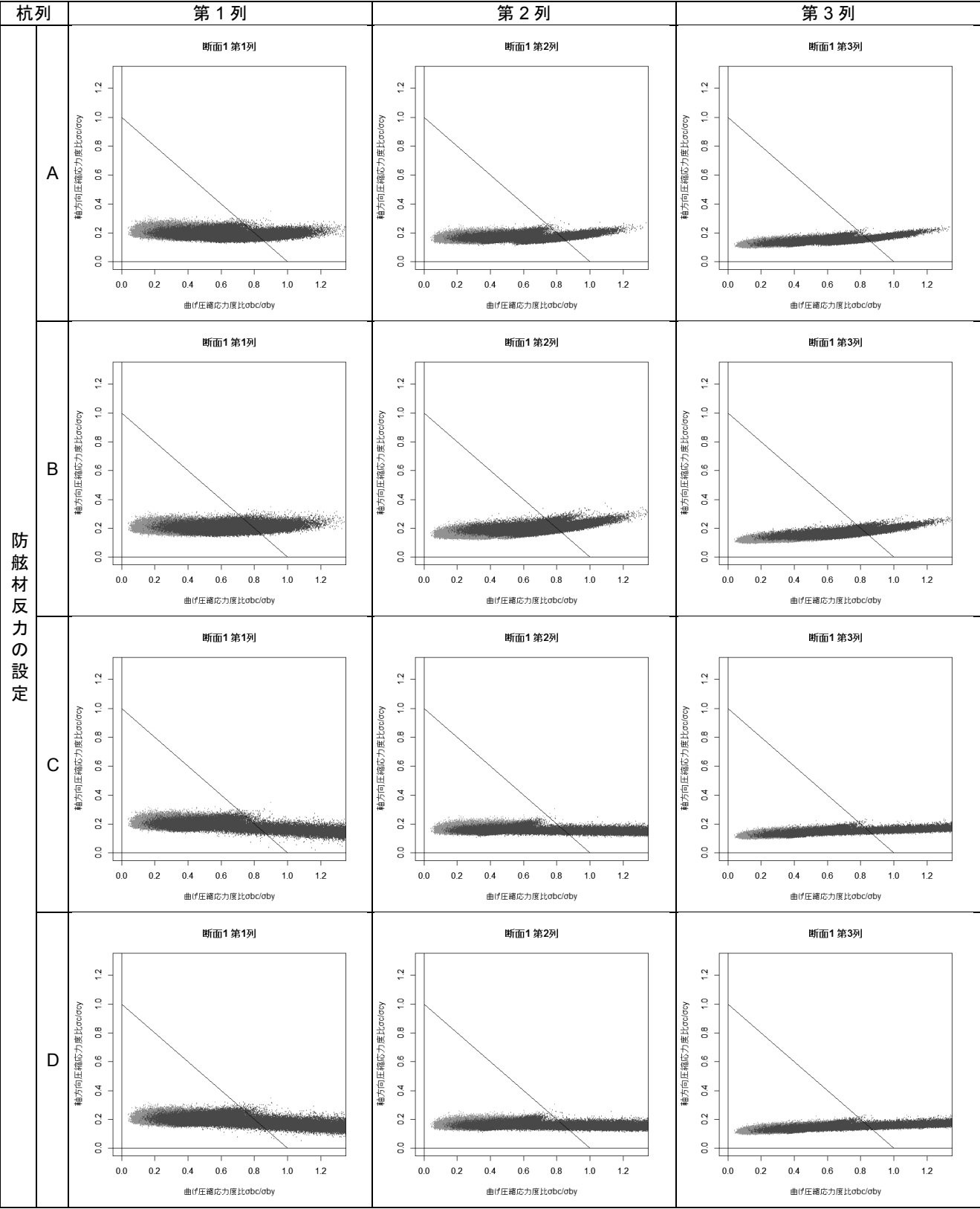
付表 F-30 杭列毎の曲げ圧縮応力度比-軸方向圧縮応力度比分布図(断面①)
