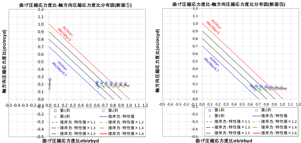
付図 C-7 曲げ圧縮・軸方向圧縮応力度比分布図(断面①：設計水深 7.5m，断面⑮：設計水深 18m)
