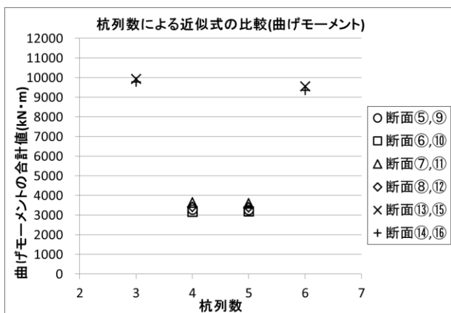
付図 A-5 杭列数に対する曲げモーメントの比較 (曲げモーメントの合計値)
