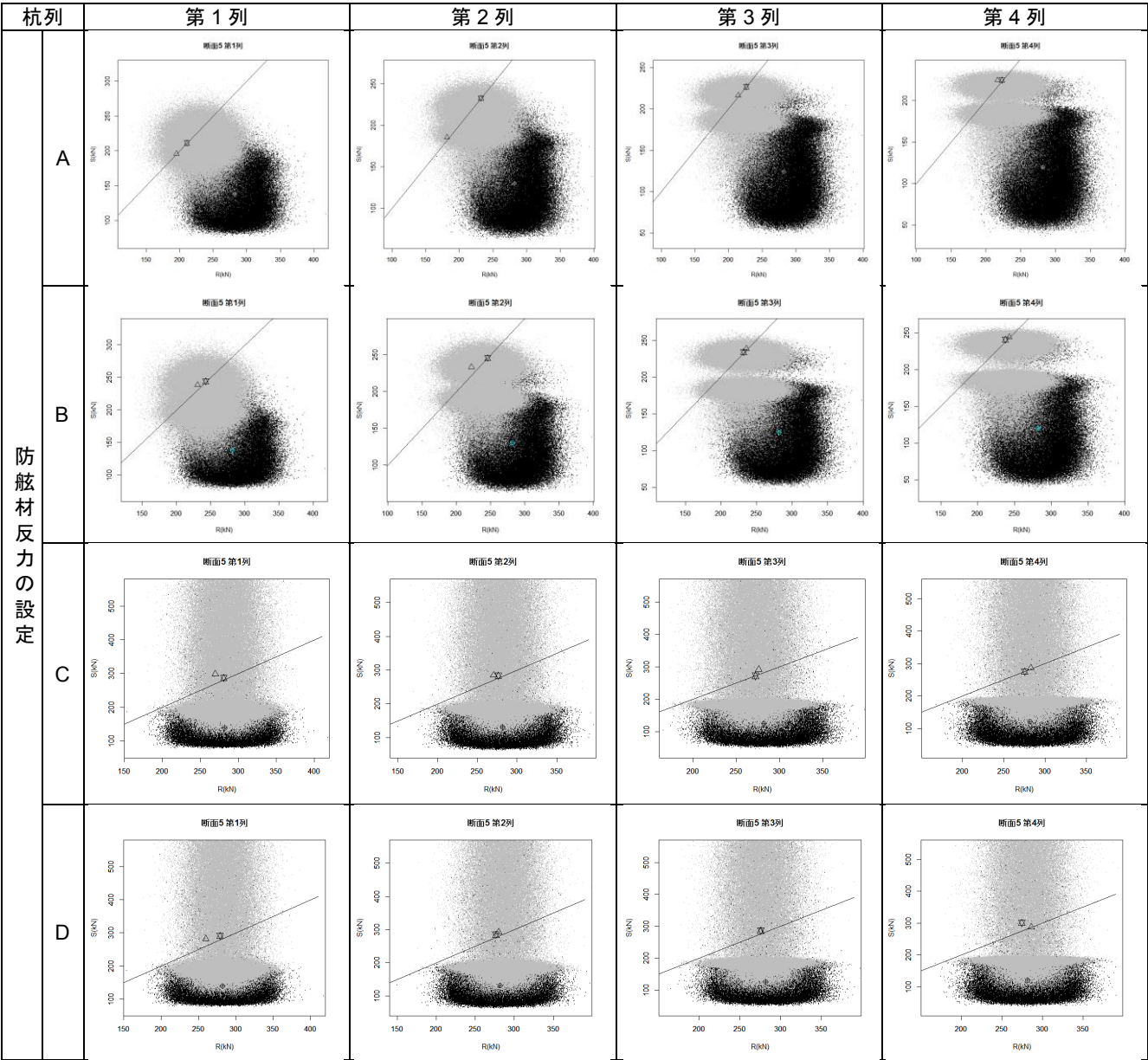
付表F-12 杭列毎の抵抗-作用分布図(断面⑤)
