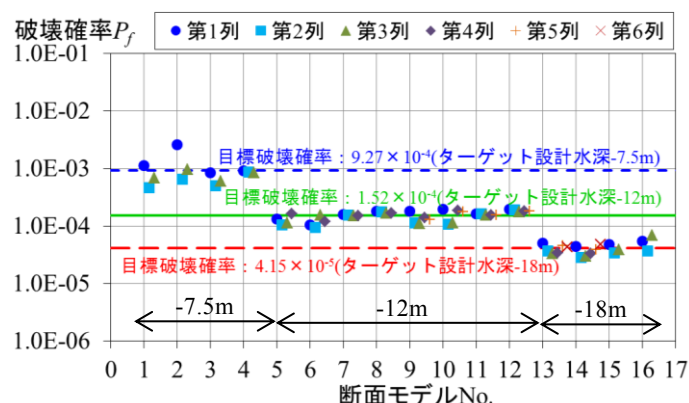
図-40 ターゲット設計水深と目標破壊確率
