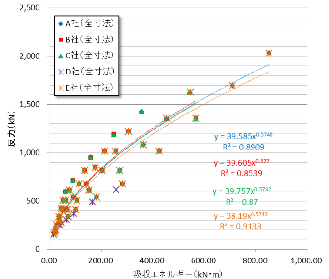
図-18 吸収エネルギーと反力の関係
