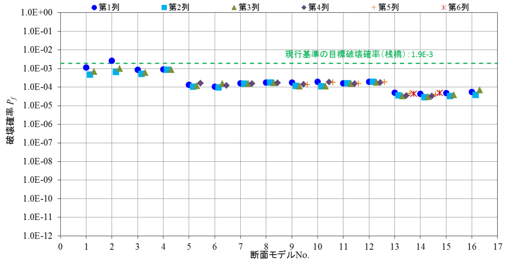
付図 F-6 各検討断面の破壊確率(設定 B)
