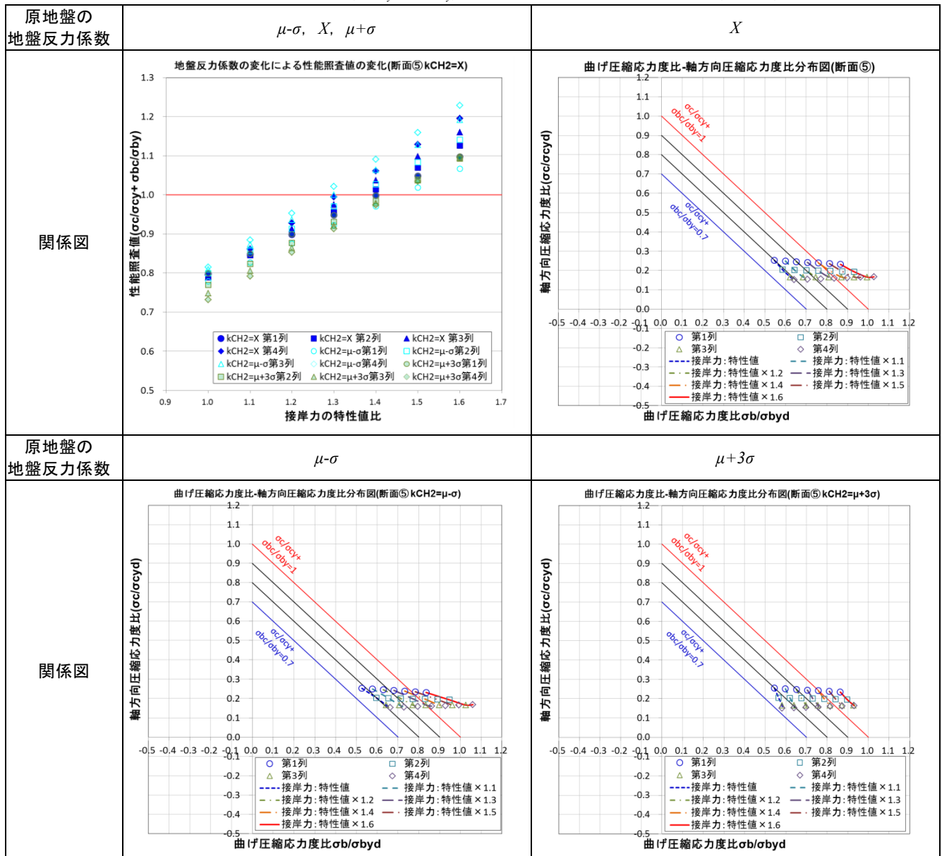
付表 C-3 性能照査値( \sigma_c/\sigma_{cy} + \sigma_{bc}/\sigma_{by} )と原地盤の地盤反力係数との関係(断面⑤)
