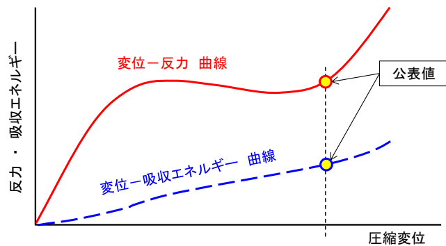
図-14 ゴム防舷材の性能曲線
