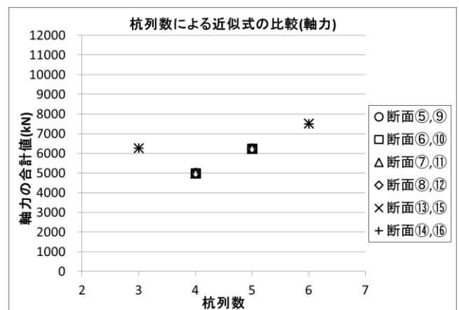
付図 A-6 杭列数に対する軸力の比較(軸力の合計値)
