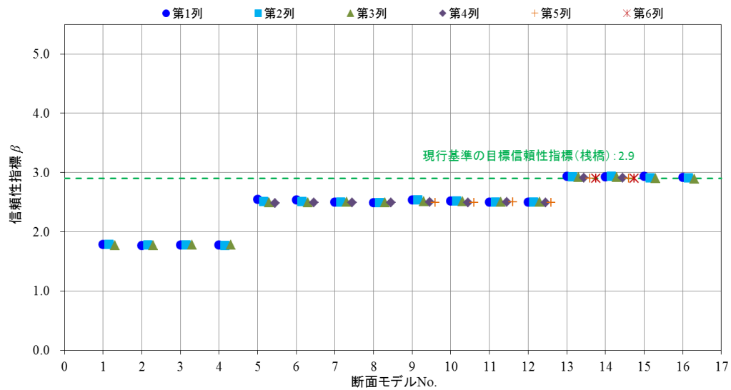
付図 F-10 各検討断面の信頼性指標(設定 C)
