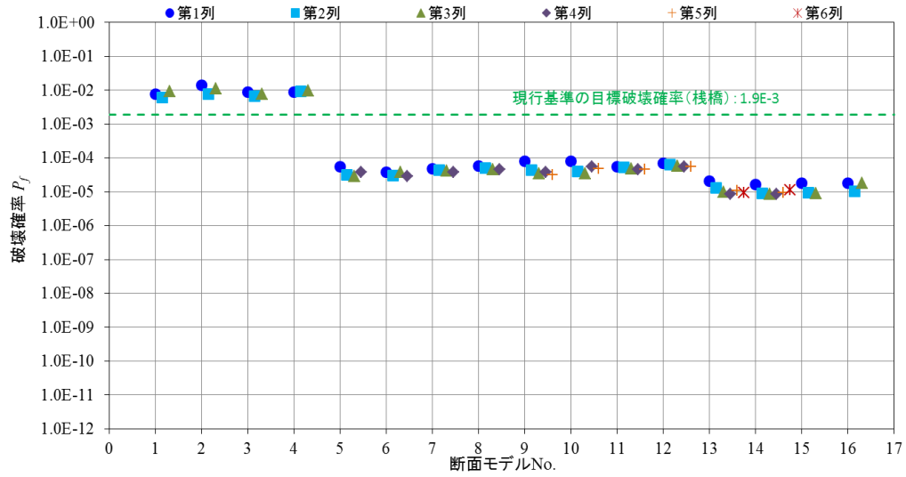
付図 F-3 各検討断面の破壊確率(設定 A)
