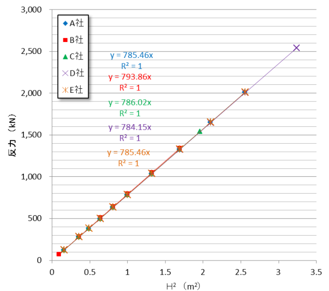
図-20 防舷材寸法ごとの反力(公表値)
