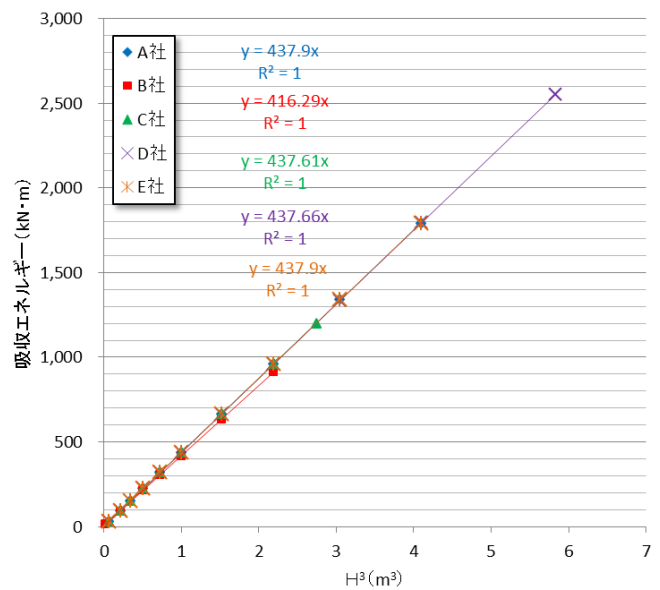
図-19 防舷材寸法ごとの吸収エネルギー(公表値)
