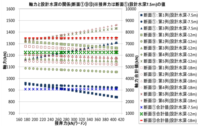
付図 B-10 接岸力の変化に対する軸力と設計水深の関係
