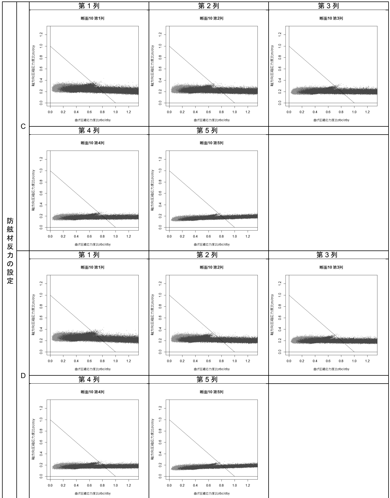
付表 F-41 杭列毎の曲げ圧縮応力度比-軸方向圧縮応力度比分布図(断面⑩ 設定 C および設定 D)
