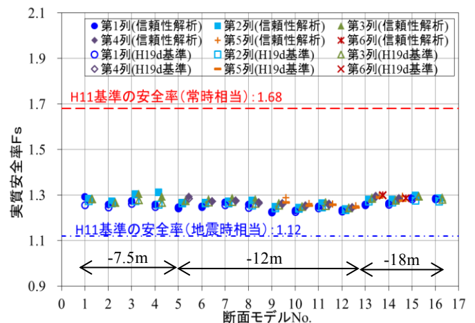
図-38 破壊点における実質安全率と現行港湾基準に基づく断面の実質安全率
