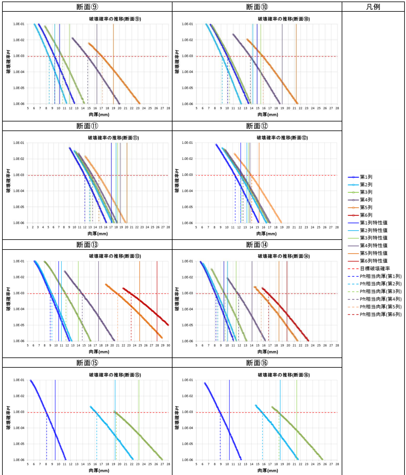
付表 G-3 肉厚ごとの破壊確率の推移と目標破壊確率相当の肉厚(断面⑨～⑯)
