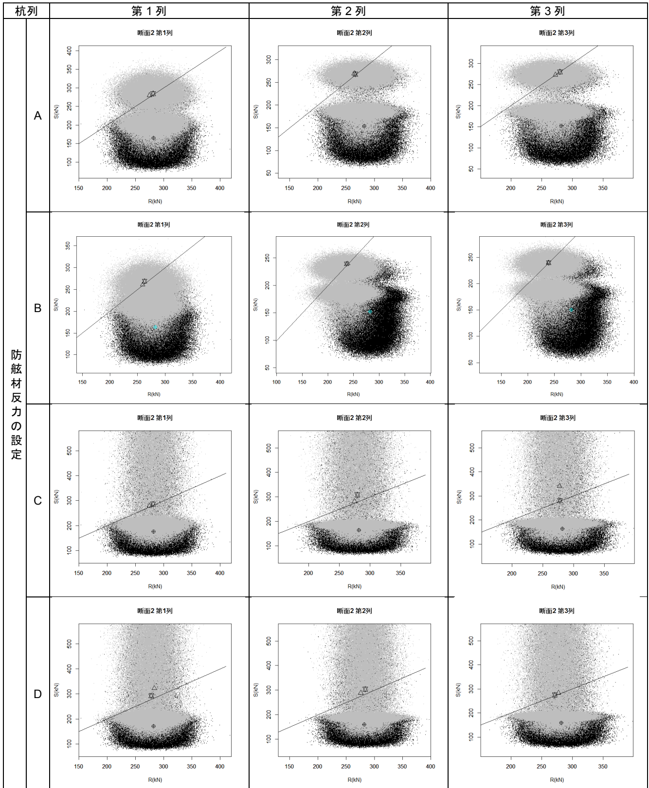
付表 F-9 杭列毎の抵抗-作用分布図(断面②)
