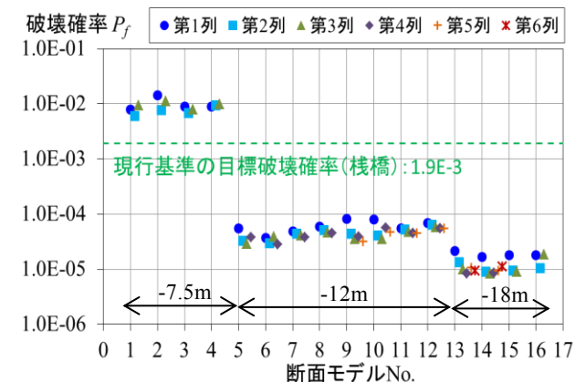
図-36 現行港湾基準を満たす断面の破壊確率
