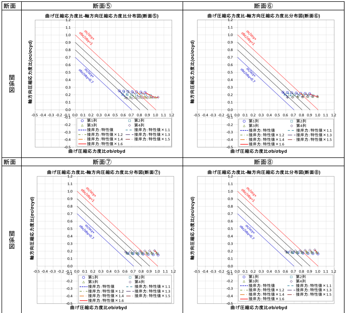
付表 C-6 接岸力を変化させた際の曲げ圧縮・軸方向圧縮応力度比分布図(断面⑤～⑧)
