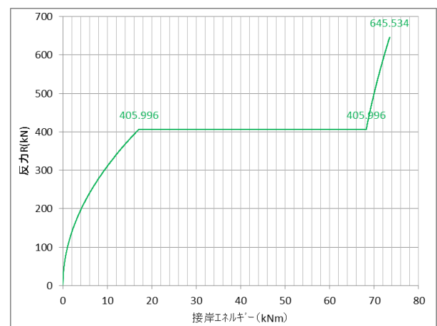
付図 E-2 モデル防舷材の接岸エネルギーと反力の関係
