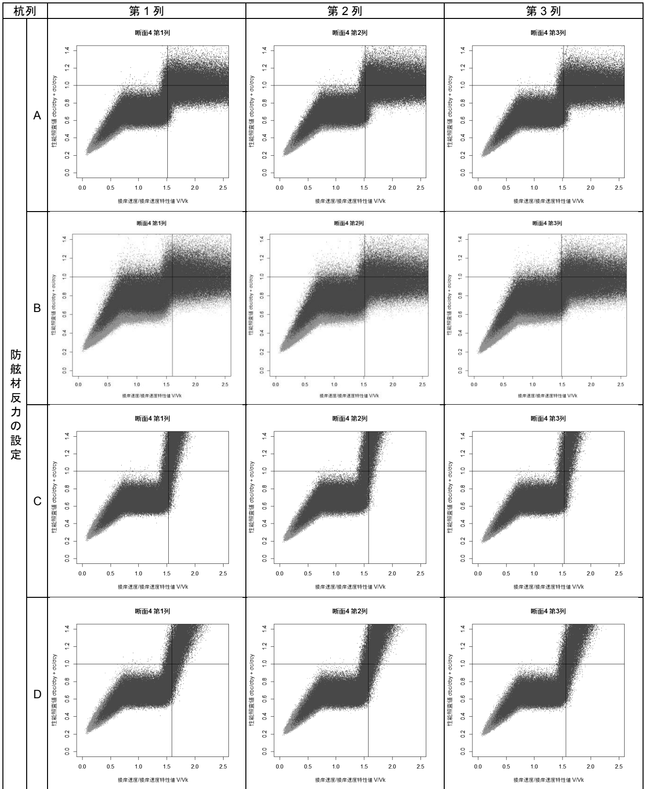
付表 F-55 接岸速度-性能照査値分布図(断面④)
