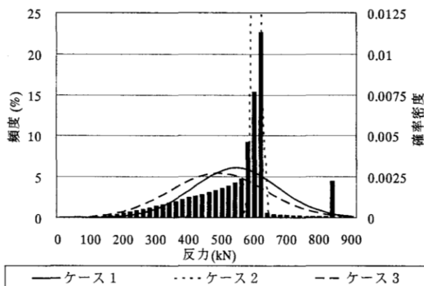
付図 D-3 防舷材反力の確率分布と正規分布化の検討ケース
