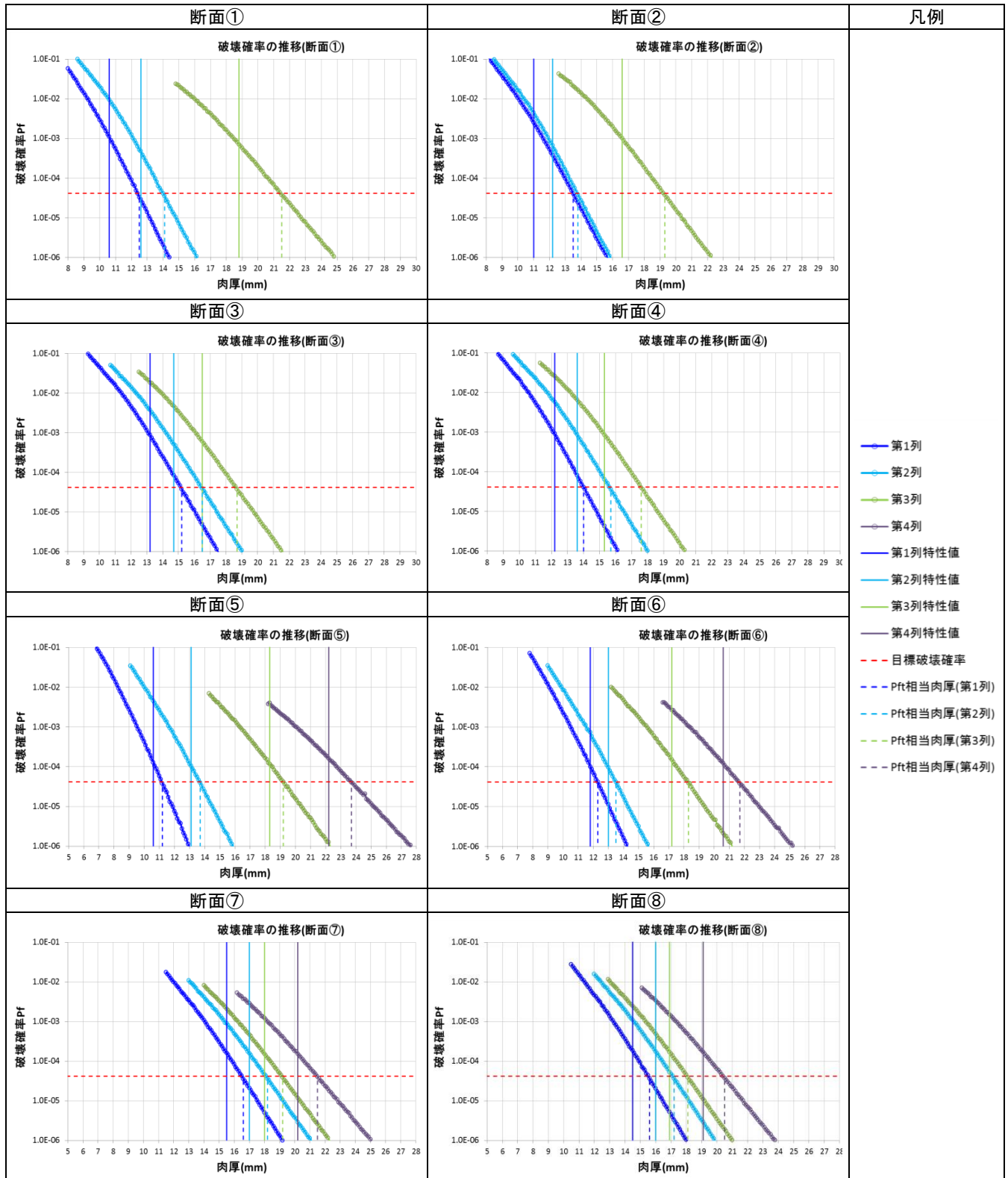
付表 G-6 肉厚ごとの破壊確率の推移と目標破壊確率相当の肉厚(断面①～⑧)
