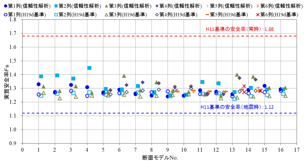
付図 F-11 各検討断面の実質安全率(設定 C)
