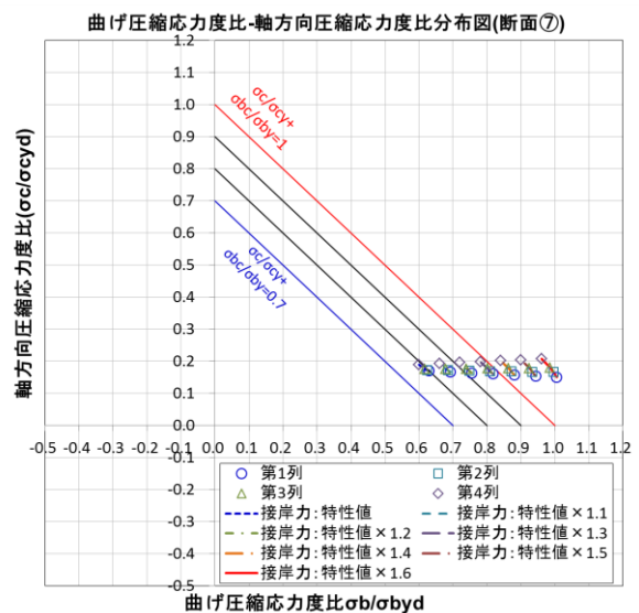
付図 C-2 圧縮応力度比分布図(断面⑦：海底勾配なし)
