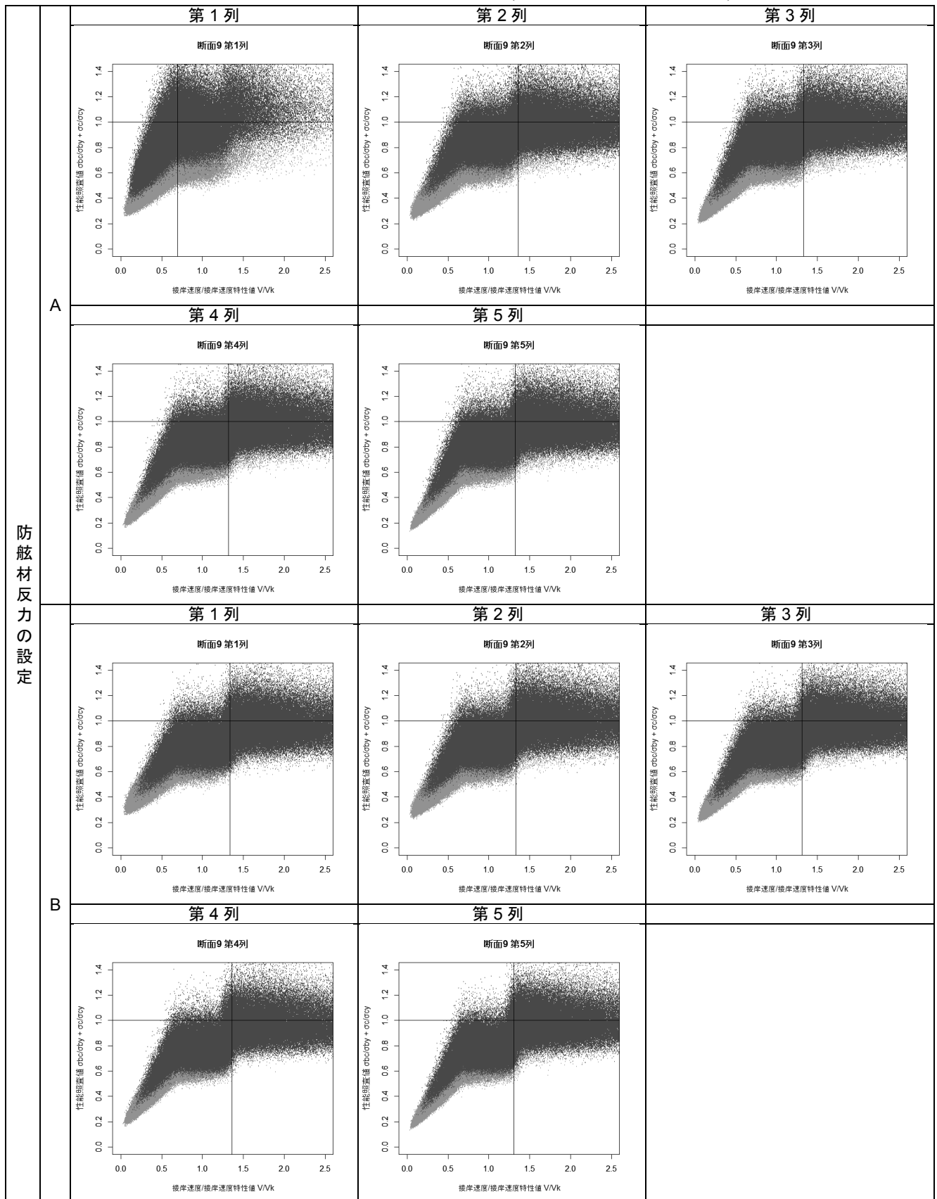
付表 F-60 接岸速度-性能照査値分布図(断面⑨ 設定 A および設定 B)
