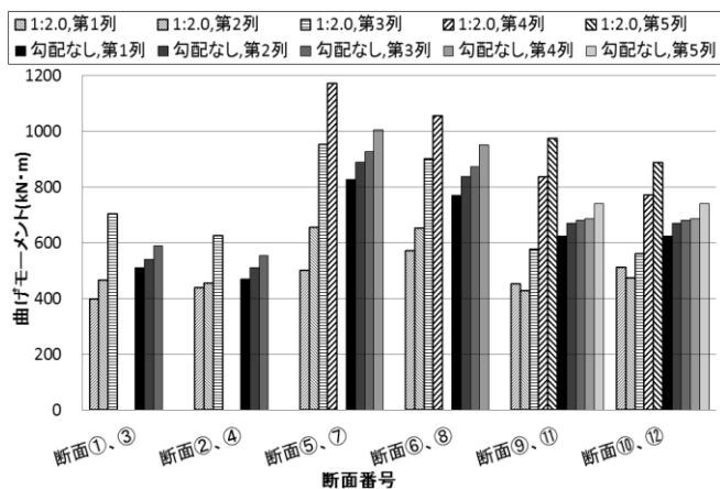
図-4 海底勾配に対する曲げモーメントの比較
