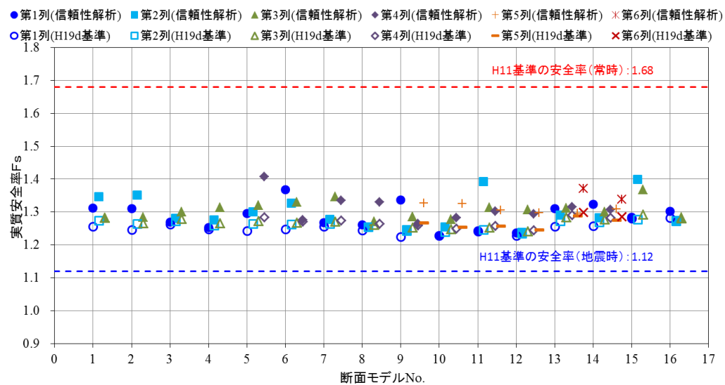
付図 F-14 各検討断面の実質安全率(設定 D)
