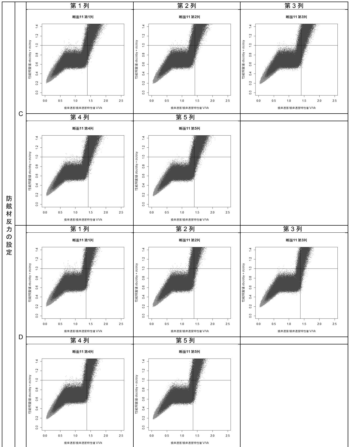
付表 F-65 接岸速度-性能照査値分布図(断面⑪ 設定 C および設定 D)
