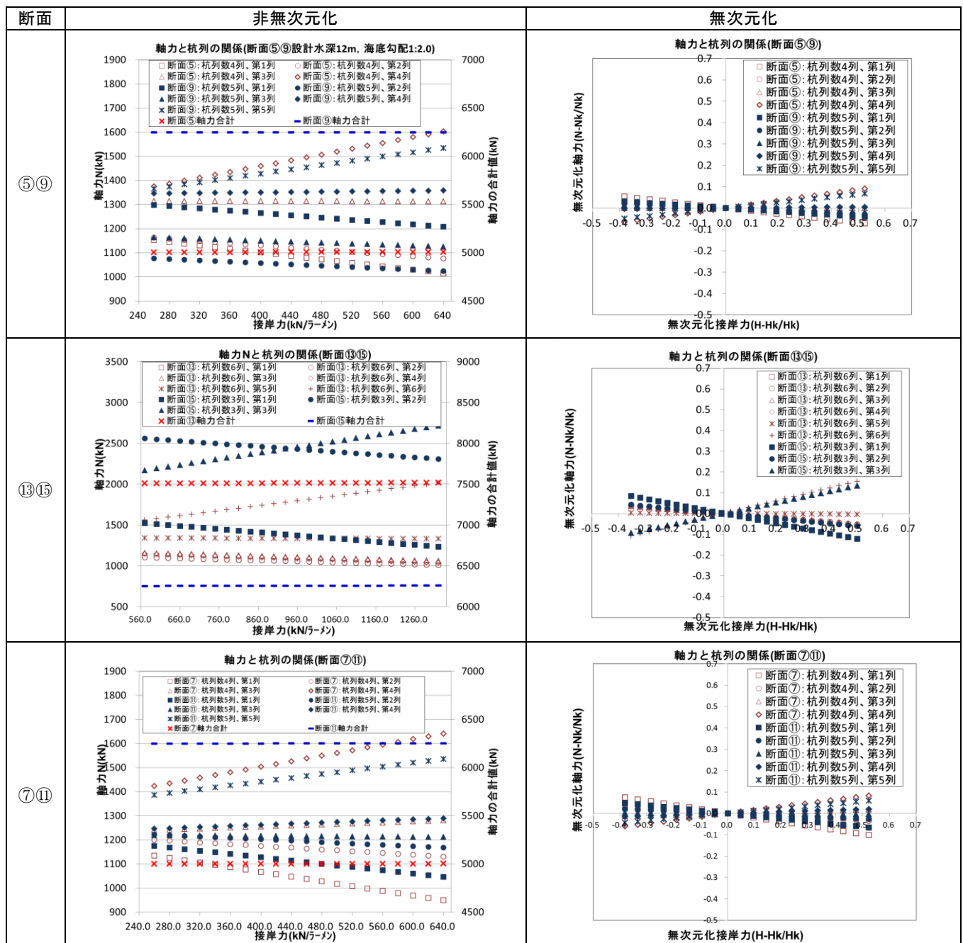
付表 B-8 接岸力の変化に対する軸力と杭列の関係
