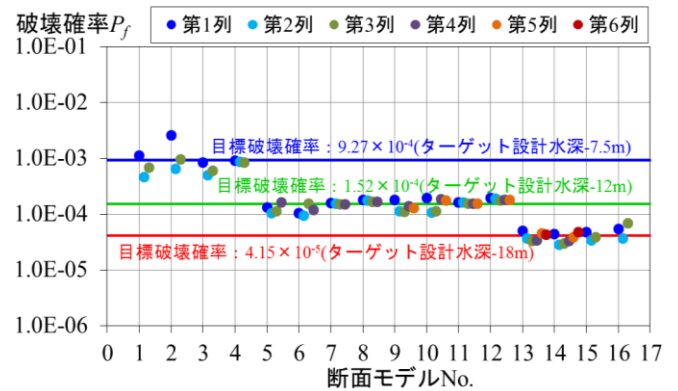
付図 G-1 ターゲット設計水深と目標破壊確率
