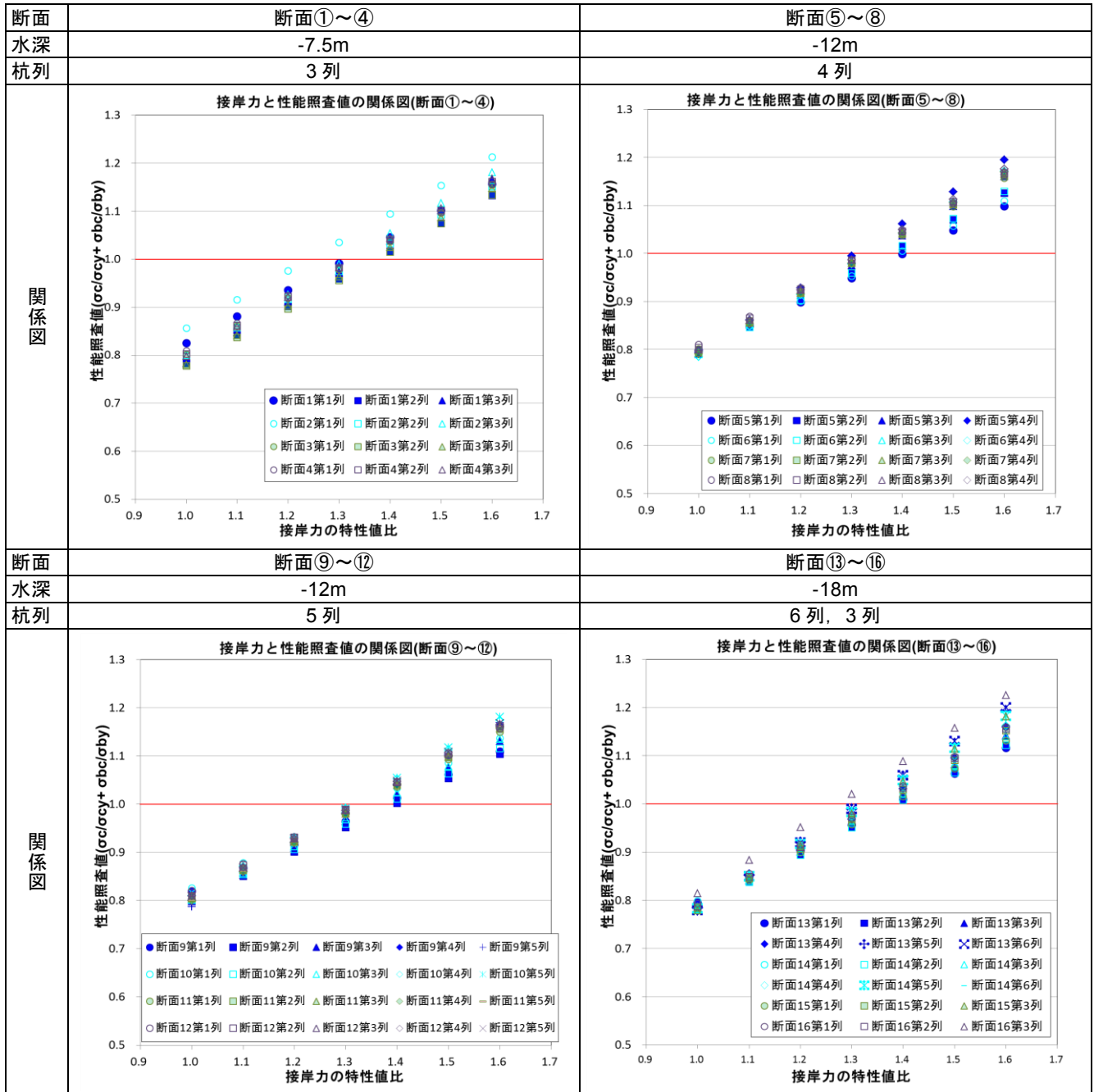
付表 C-4 接岸力と性能照査値の関係図
