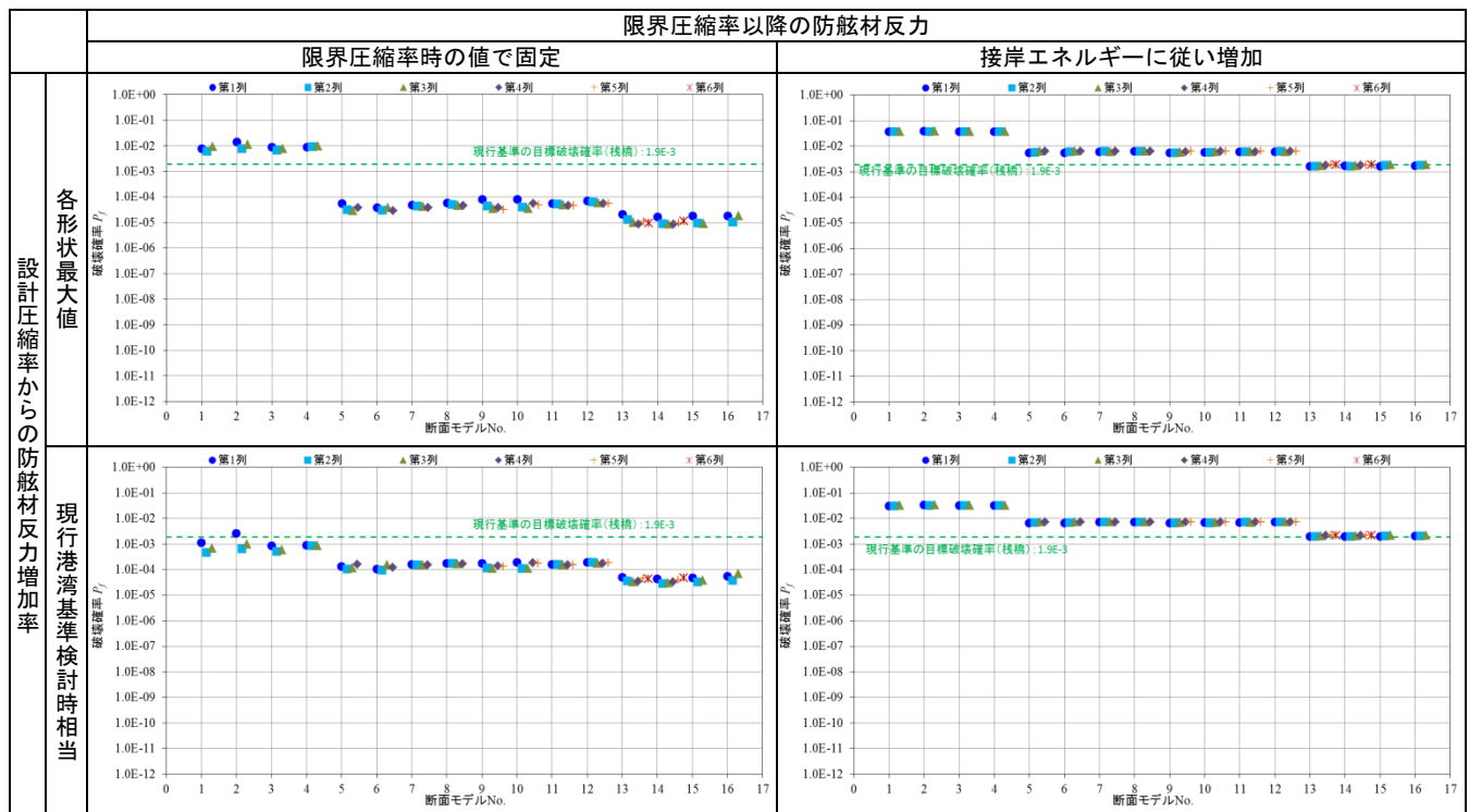
付表 F-78 各杭の破壊確率
