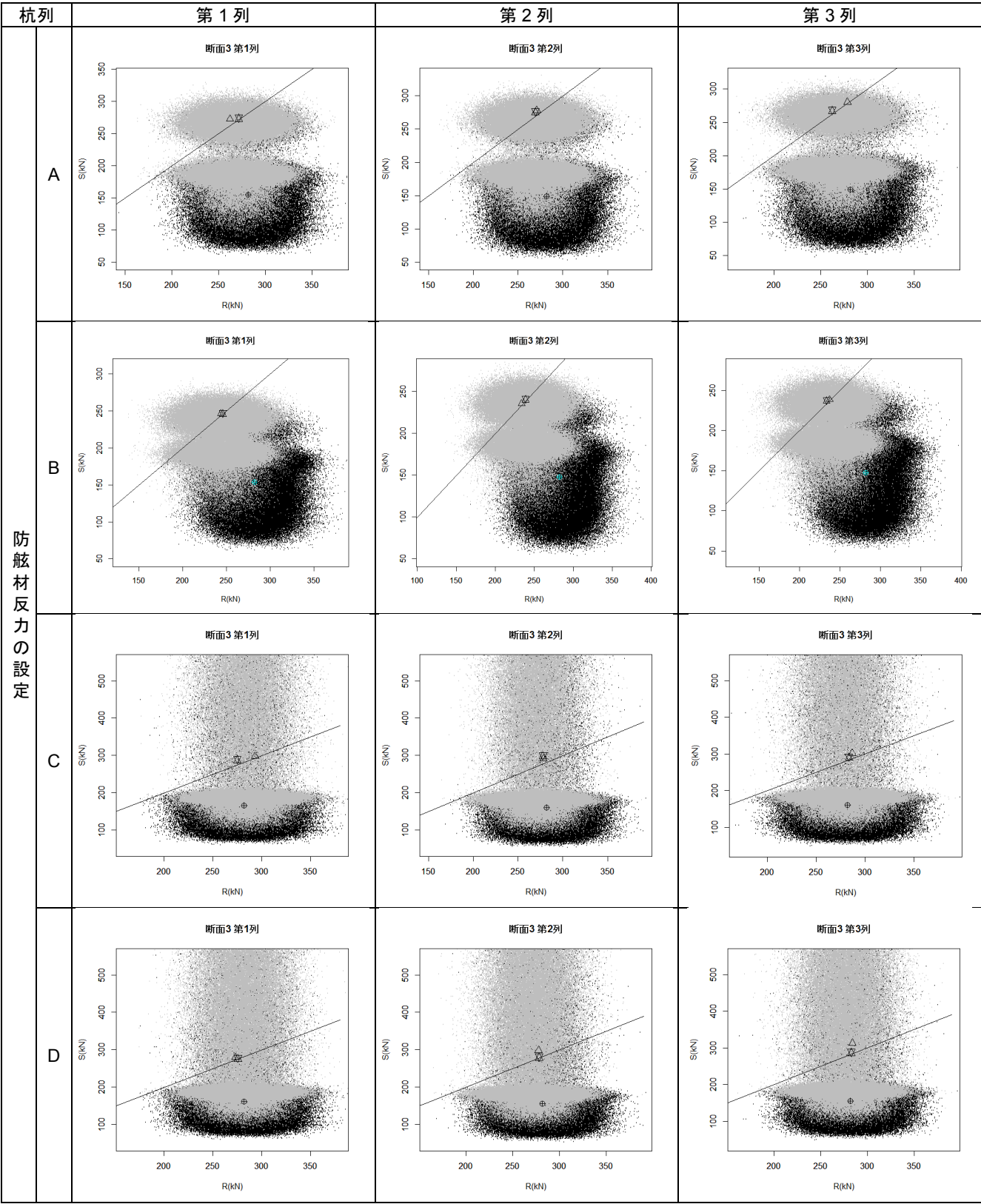
付表 F-10 杭列毎の抵抗-作用分布図(断面③)
