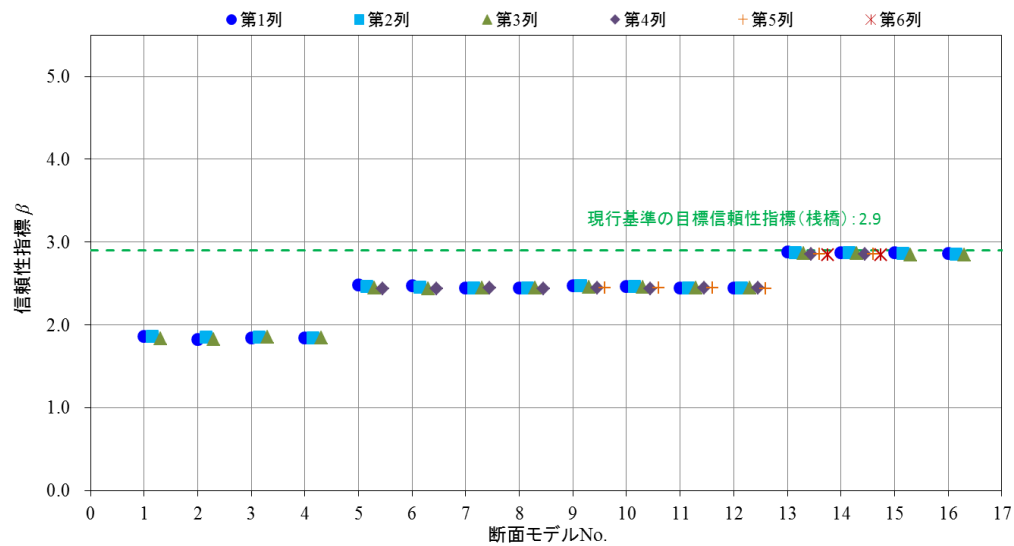
付図 F-13 各検討断面の信頼性指標(設定 D)
