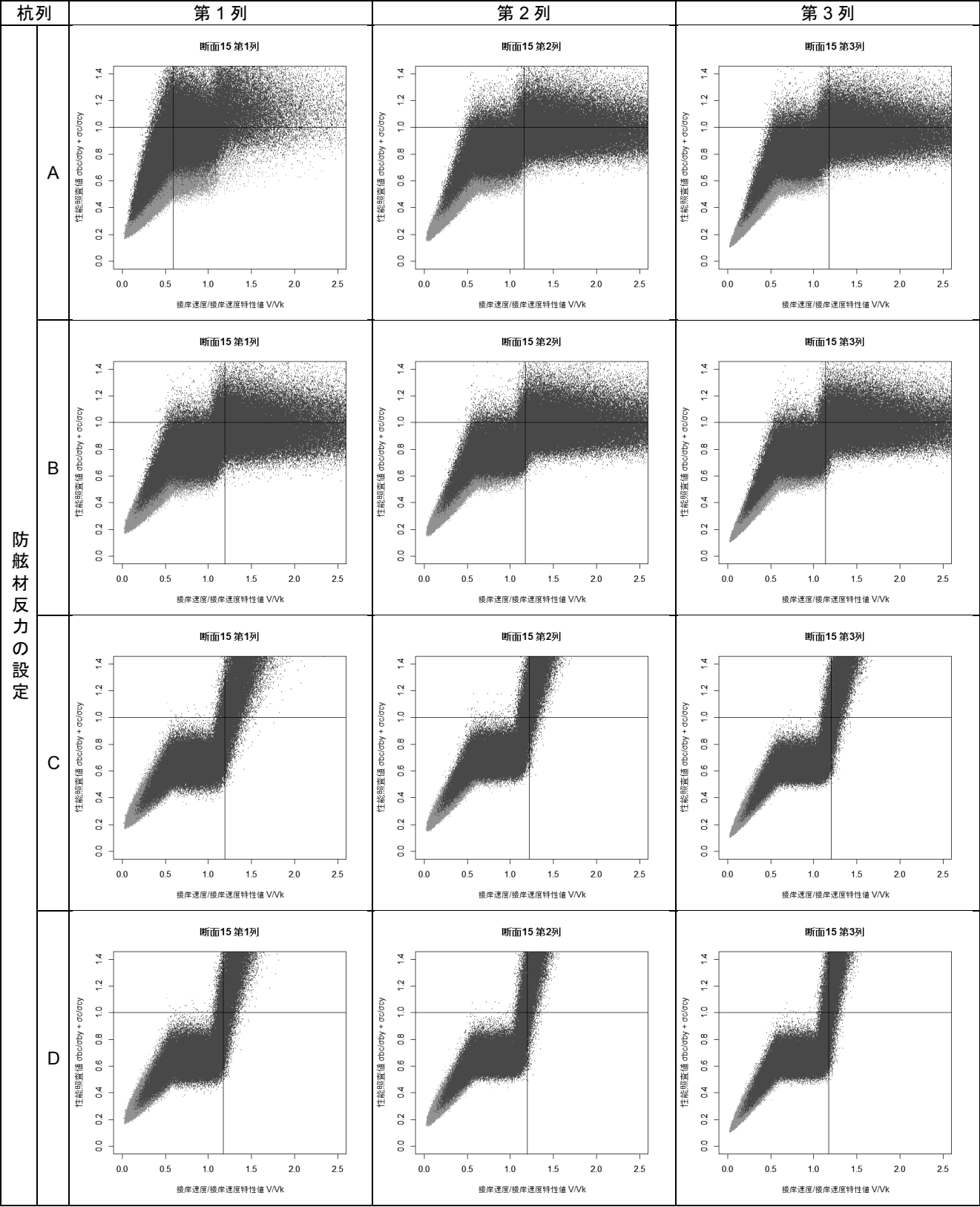
付表 F-72 接岸速度-性能照査値分布図(断面⑮)
