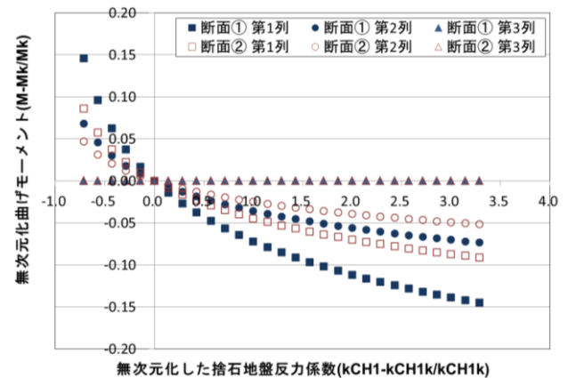
図-7 無次元化した捨石地盤反力係数の変化に対する曲げモーメントの推移(断面①②)
