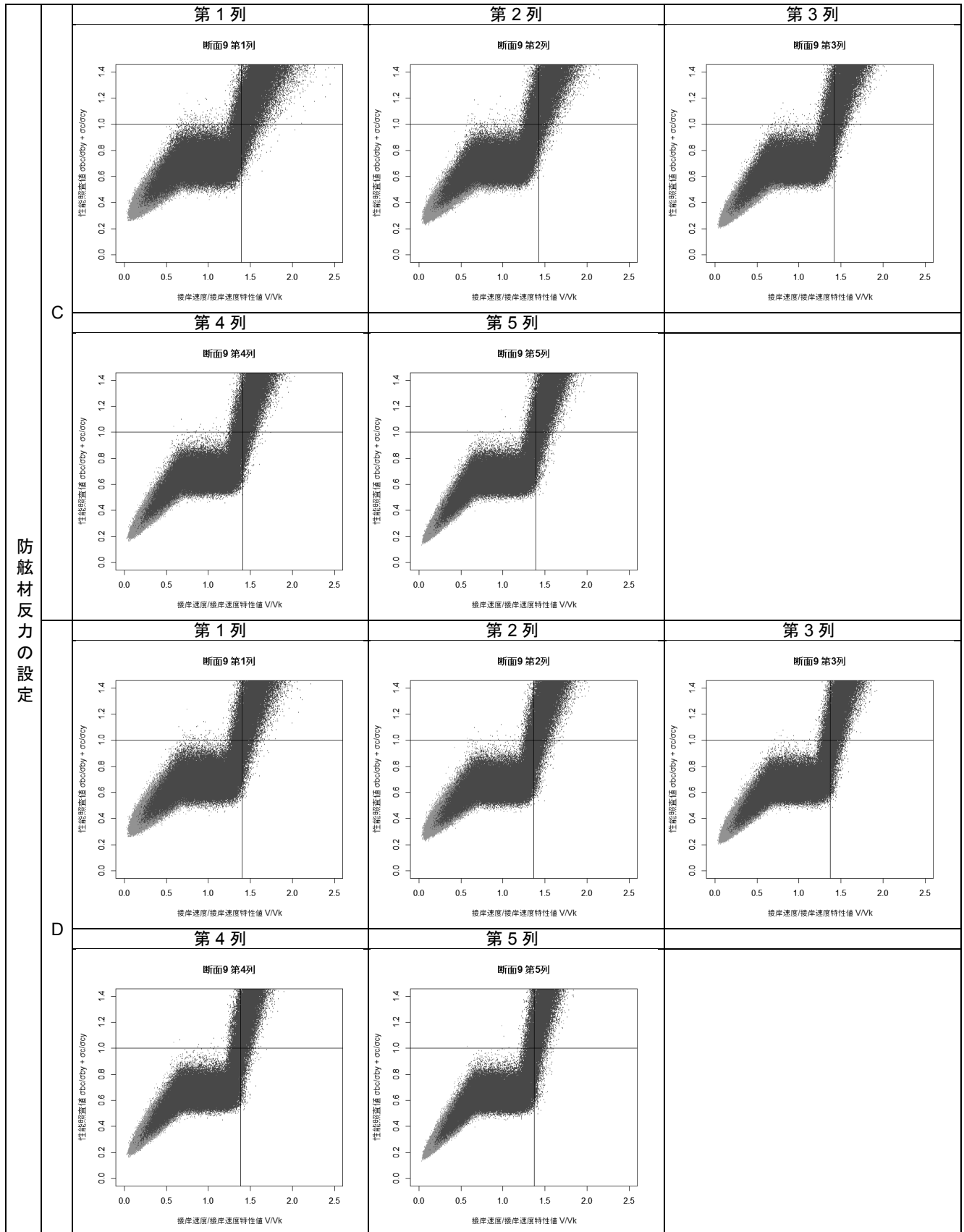
付表 F-61 接岸速度-性能照査値分布図(断面⑨ 設定 C および設定 D)
