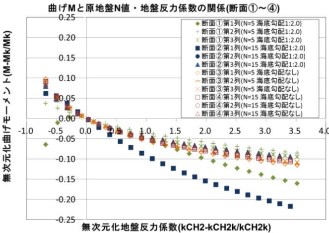
付図 B-3 無次元化した原地盤の地盤反力係数の変化に 対する曲げモーメントの推移
