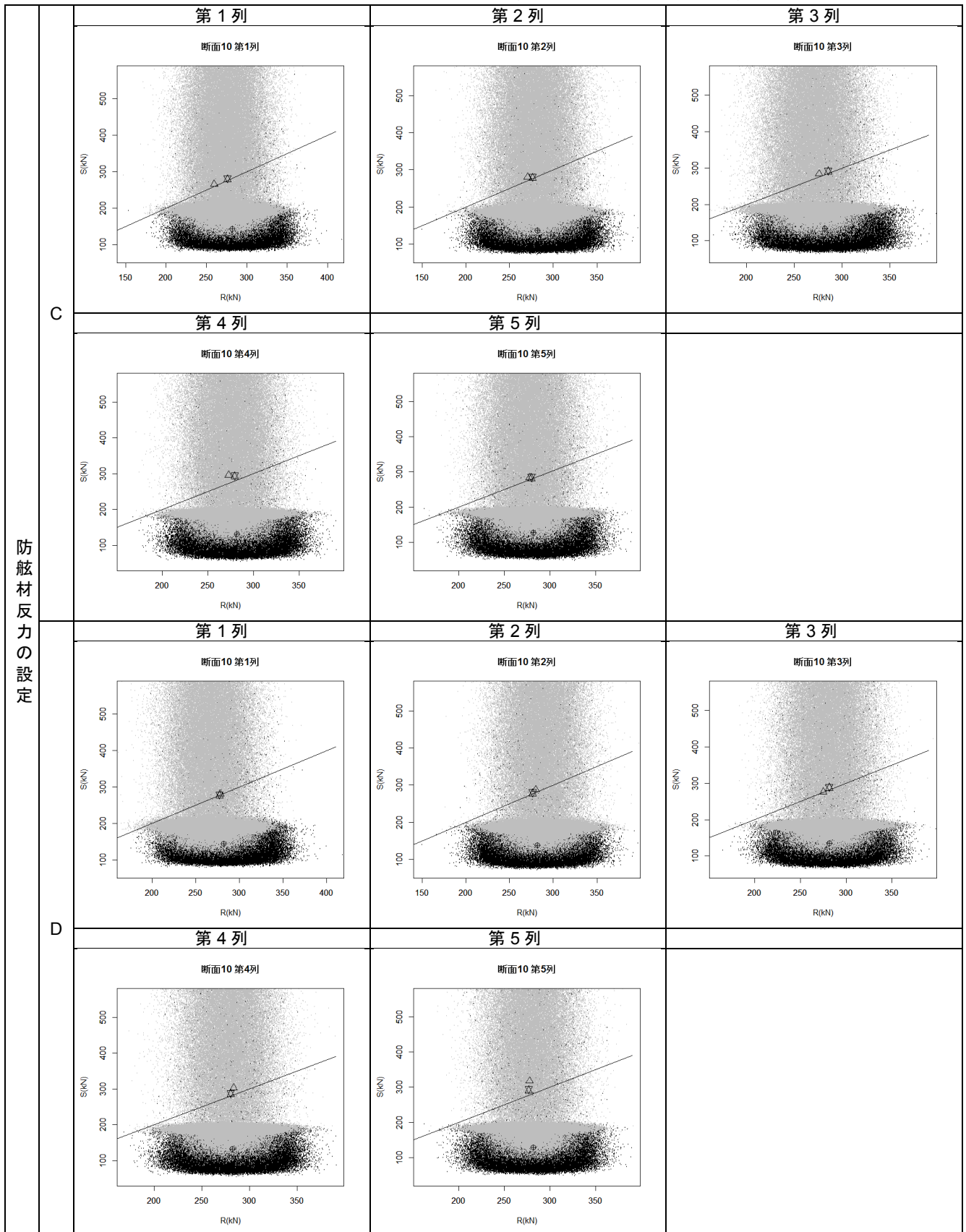
付表 F-19 杭列毎の抵抗-作用分布図(断面⑩ 設定 C および設定 D)
