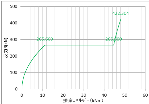
図-31 モデル化後の接岸エネルギー E_f と反力 R の関係
