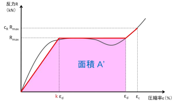
図-27 直線モデル面積 A'
