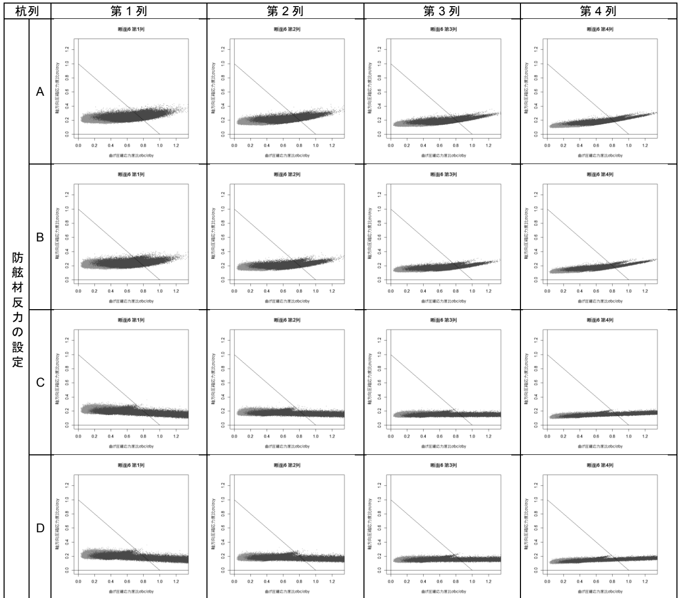
付表 F-35 杭列毎の曲げ圧縮応力度比-軸方向圧縮応力度比分布図(断面⑥)
