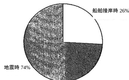
図-42 杭の断面応力度の決定条件
