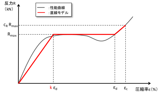
図-22 性能曲線の直線モデル化
