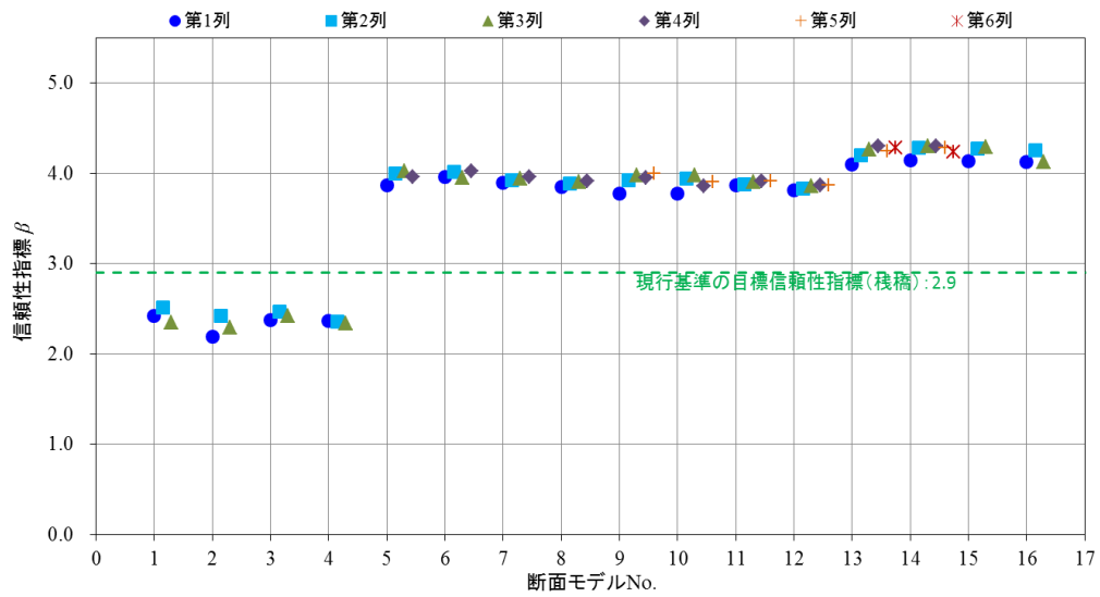
付図 F-4 各検討断面の信頼性指標(設定 A)
