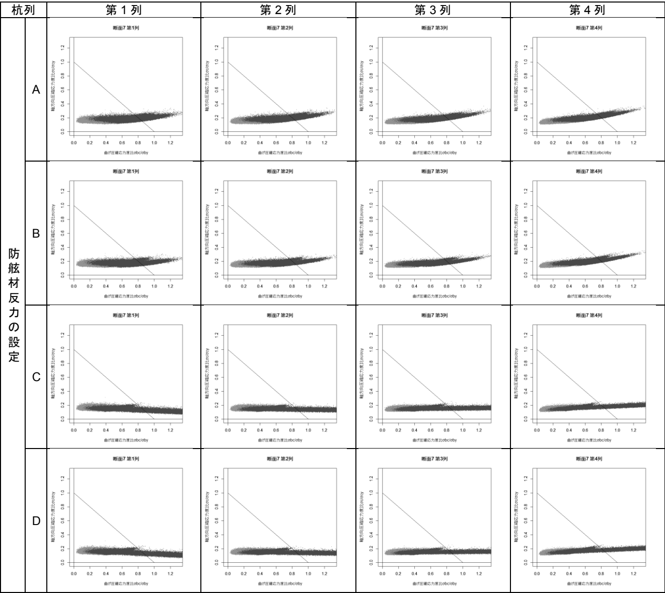
付表 F-36 杭列毎の曲げ圧縮応力度比-軸方向圧縮応力度比分布図(断面⑦)
