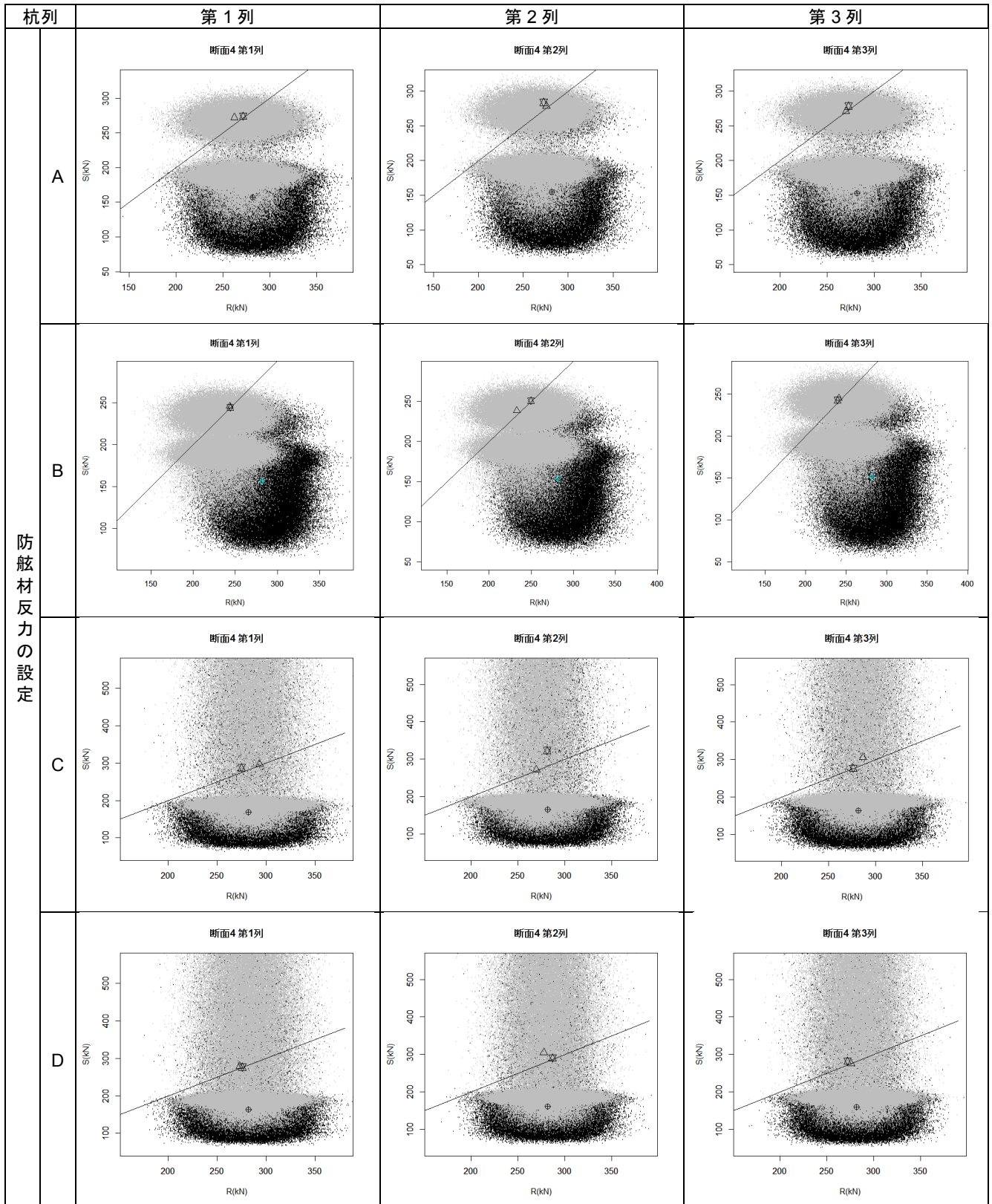
付表F-11 杭列毎の抵抗-作用分布図(断面④)
