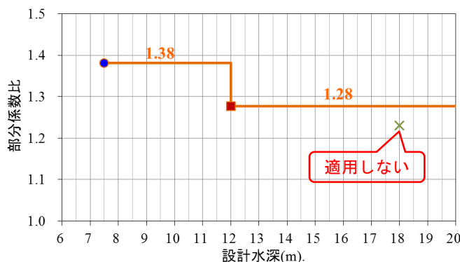
図-44 部分係数の適用範囲
