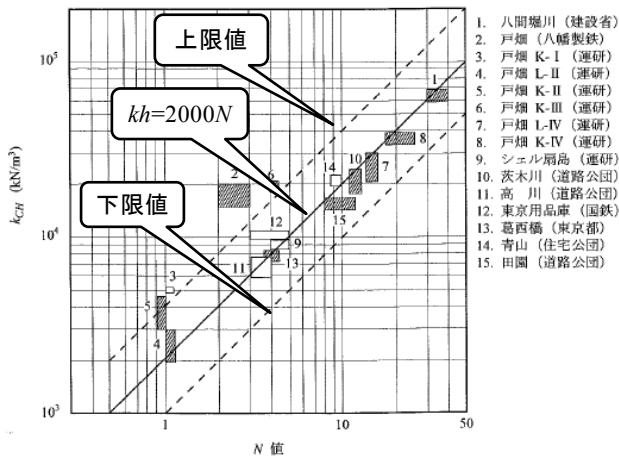
図-10 横山の関係図
