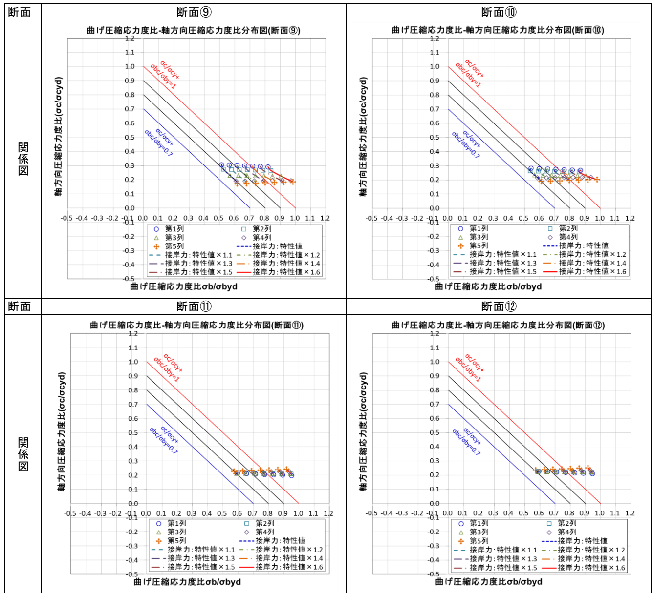
付表 C-7 接岸力を変化させた際の曲げ圧縮・軸方向圧縮応力度比分布図(断面⑨～⑫)
