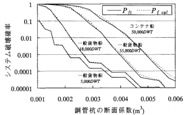
付図 D-4 システム破壊確率の比較(正規分布化ケース 1)
