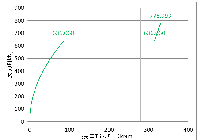
付図 E-4 モデル防舷材の接岸エネルギーと反力の関係
