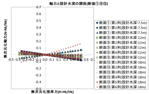
付図 B-11 無次元化した接岸力の変化に対する軸力と設計水深の関係
