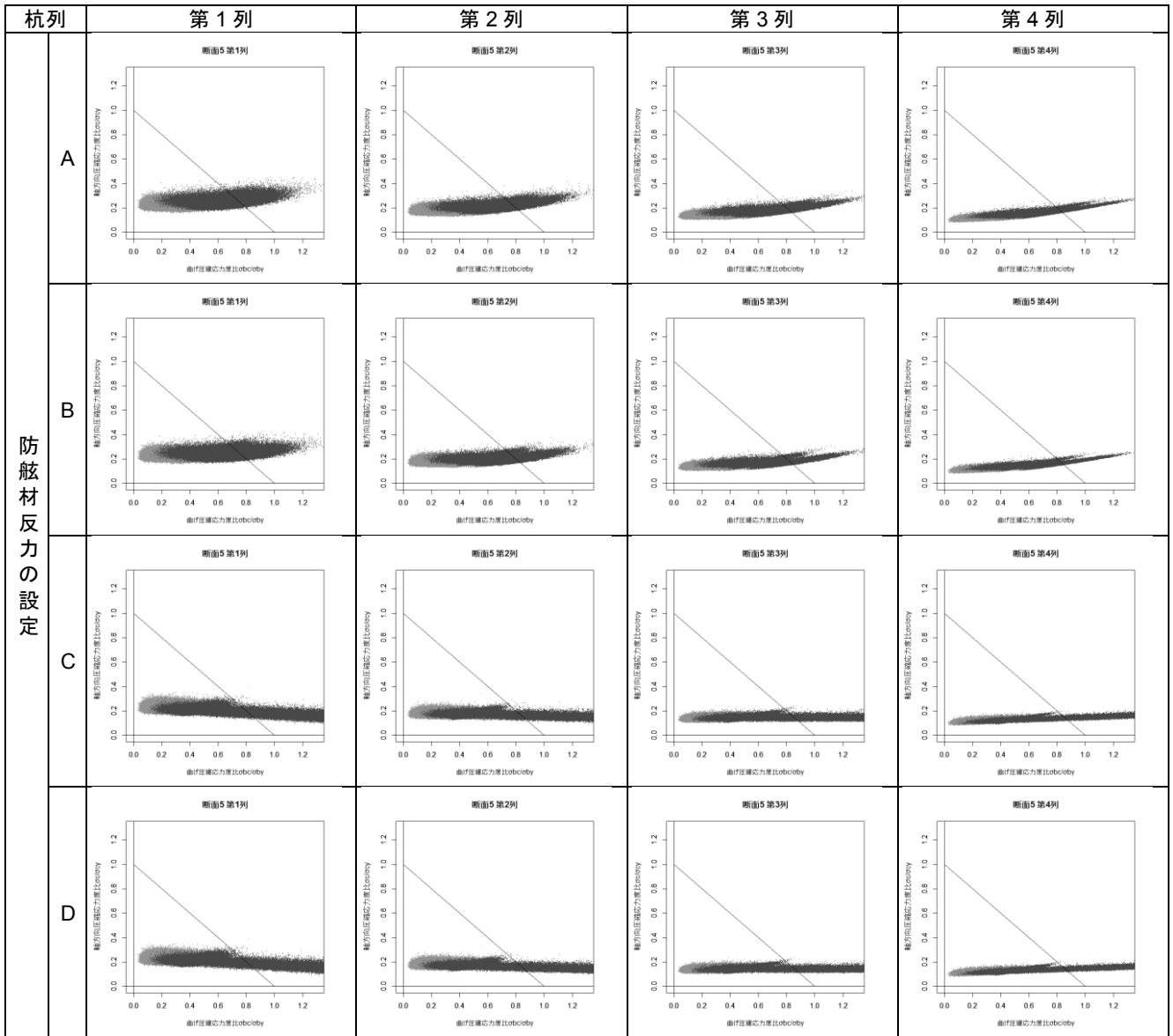
付表 F-34 杭列毎の曲げ圧縮応力度比-軸方向圧縮応力度比分布図(断面⑤)
