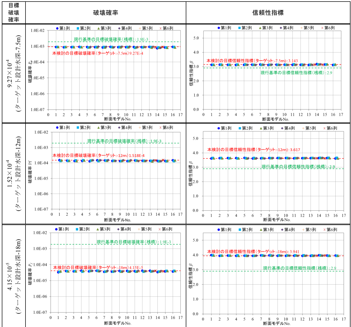
付表 H-4 目標破壊確率における各断面の破壊確率・信頼性指標
