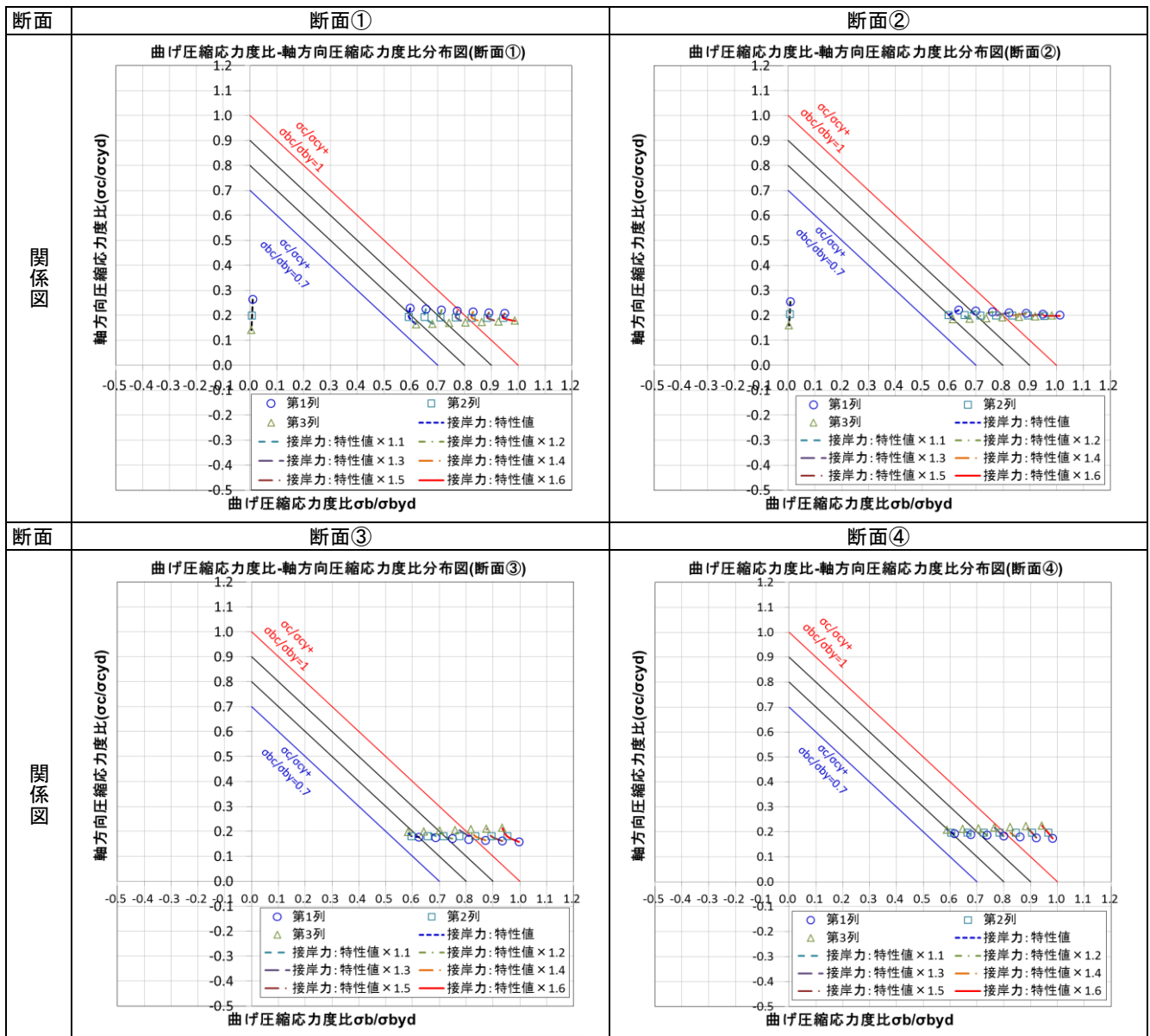
付表 C-5 接岸力を変化させた際の曲げ圧縮・軸方向圧縮応力度比分布図(断面①～④)
