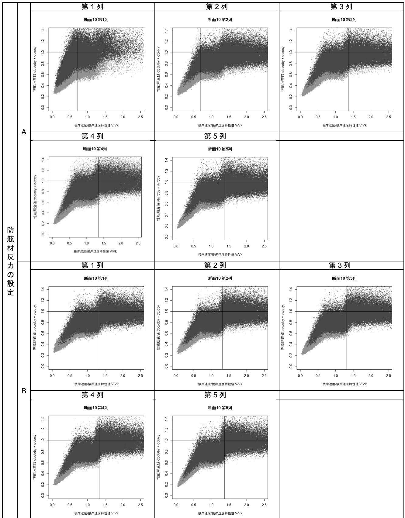
付表 F-62 接岸速度-性能照査値分布図(断面⑩ 設定 A および設定 B)
