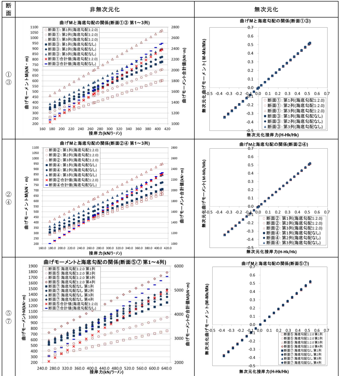
付表 B-5 接岸力の変化に対する曲げモーメントと海底勾配の関係
