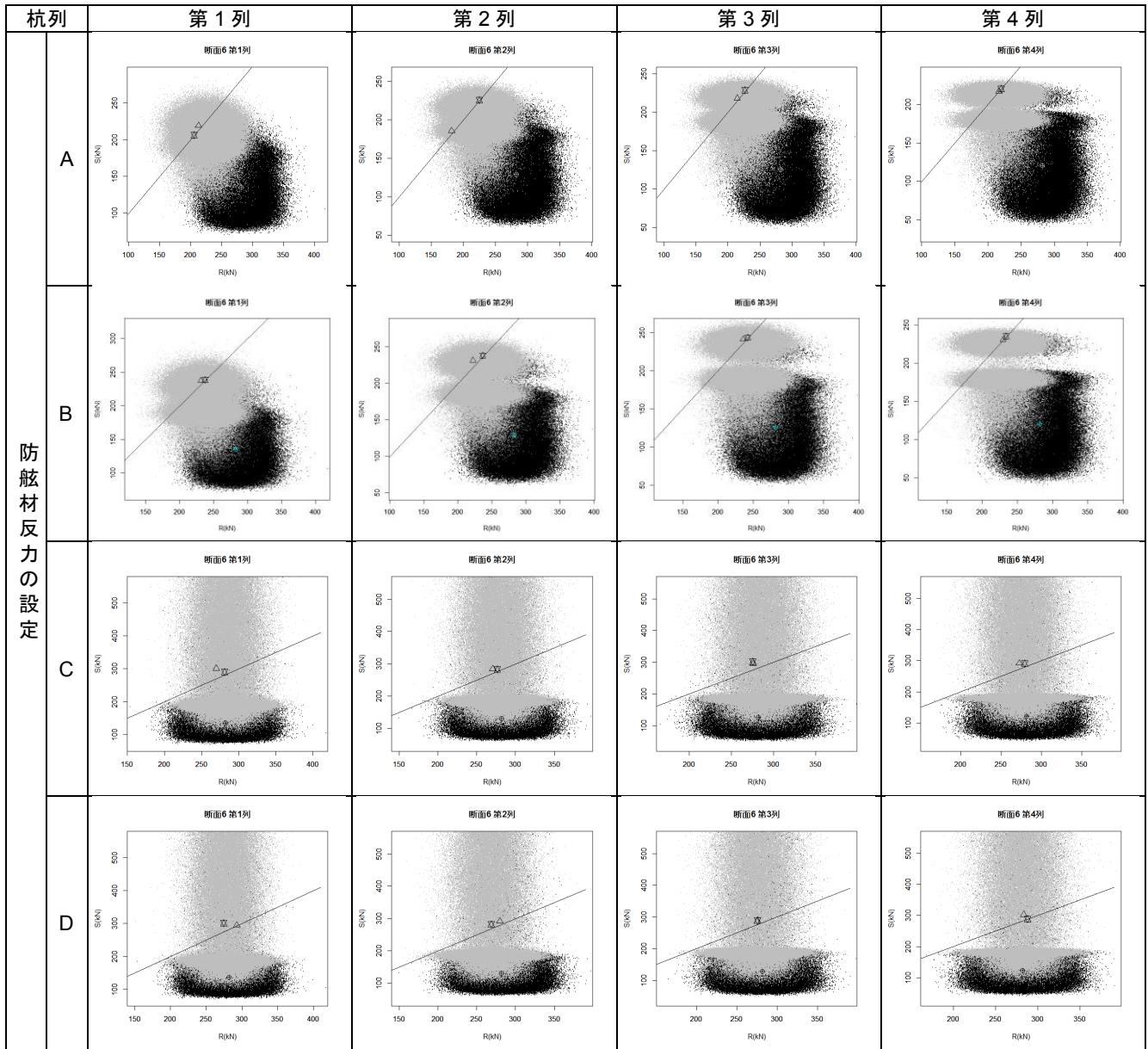
付表F-13 杭列毎の抵抗-作用分布図(断面⑥)
