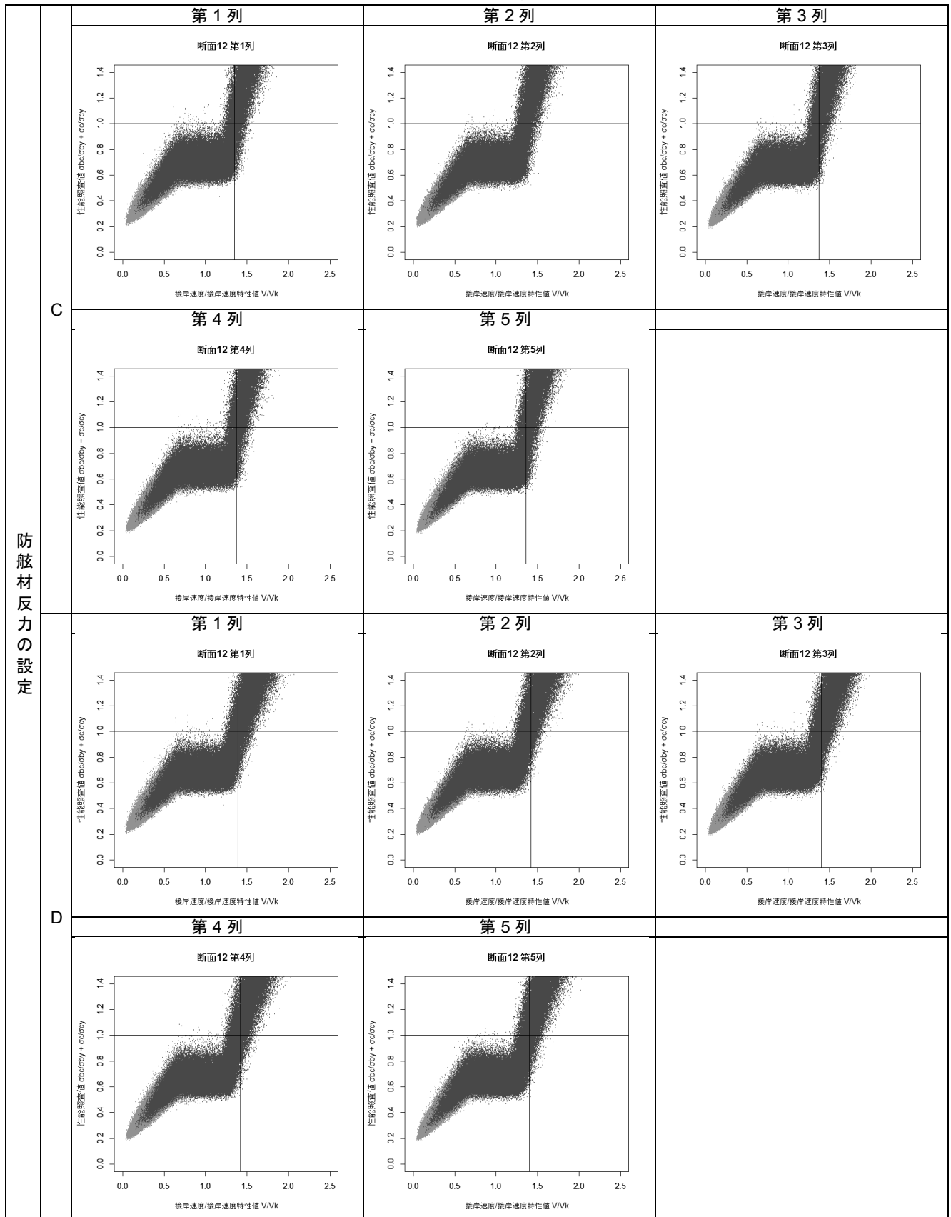
付表 F-67 接岸速度-性能照査値分布図(断面⑫ 設定 C および設定 D)
