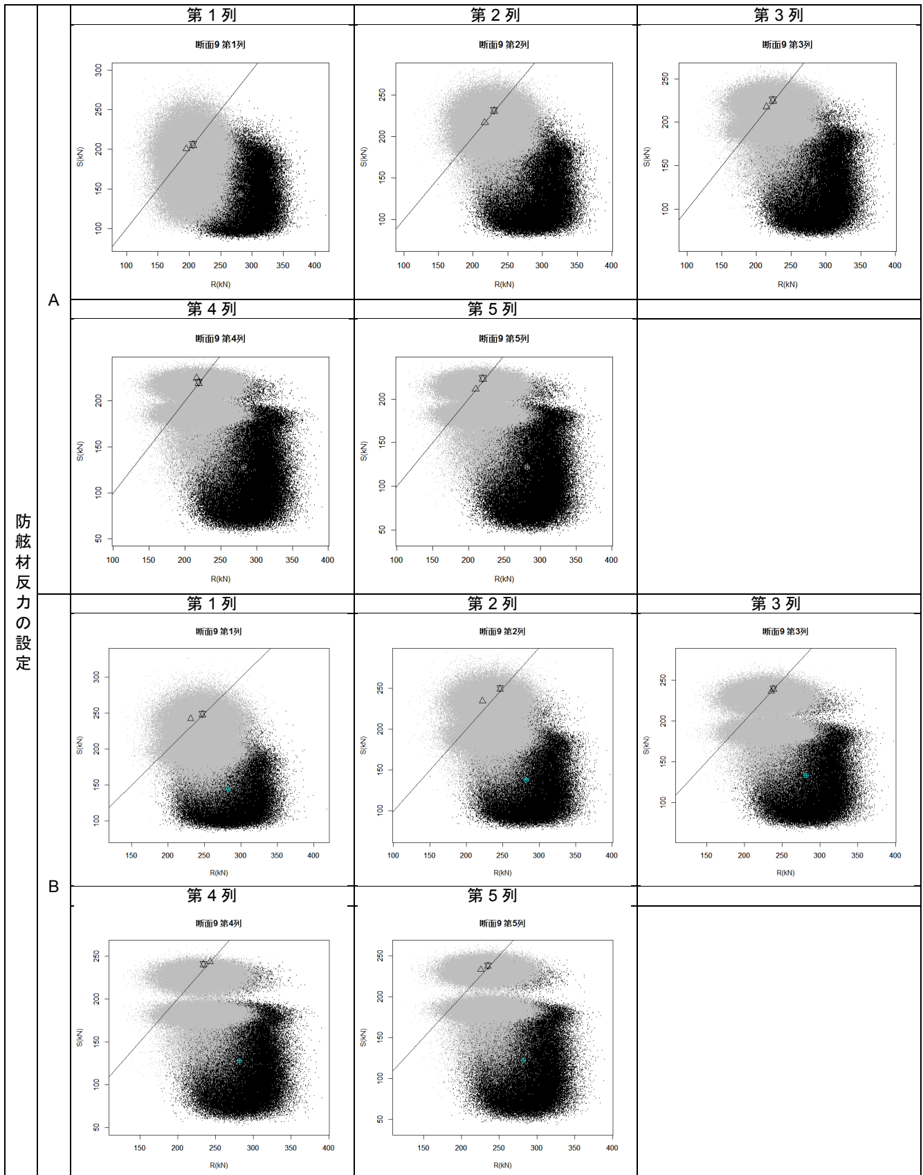
付表 F-16 杭列毎の抵抗-作用分布図(断面⑨ 設定 A および設定 B)
