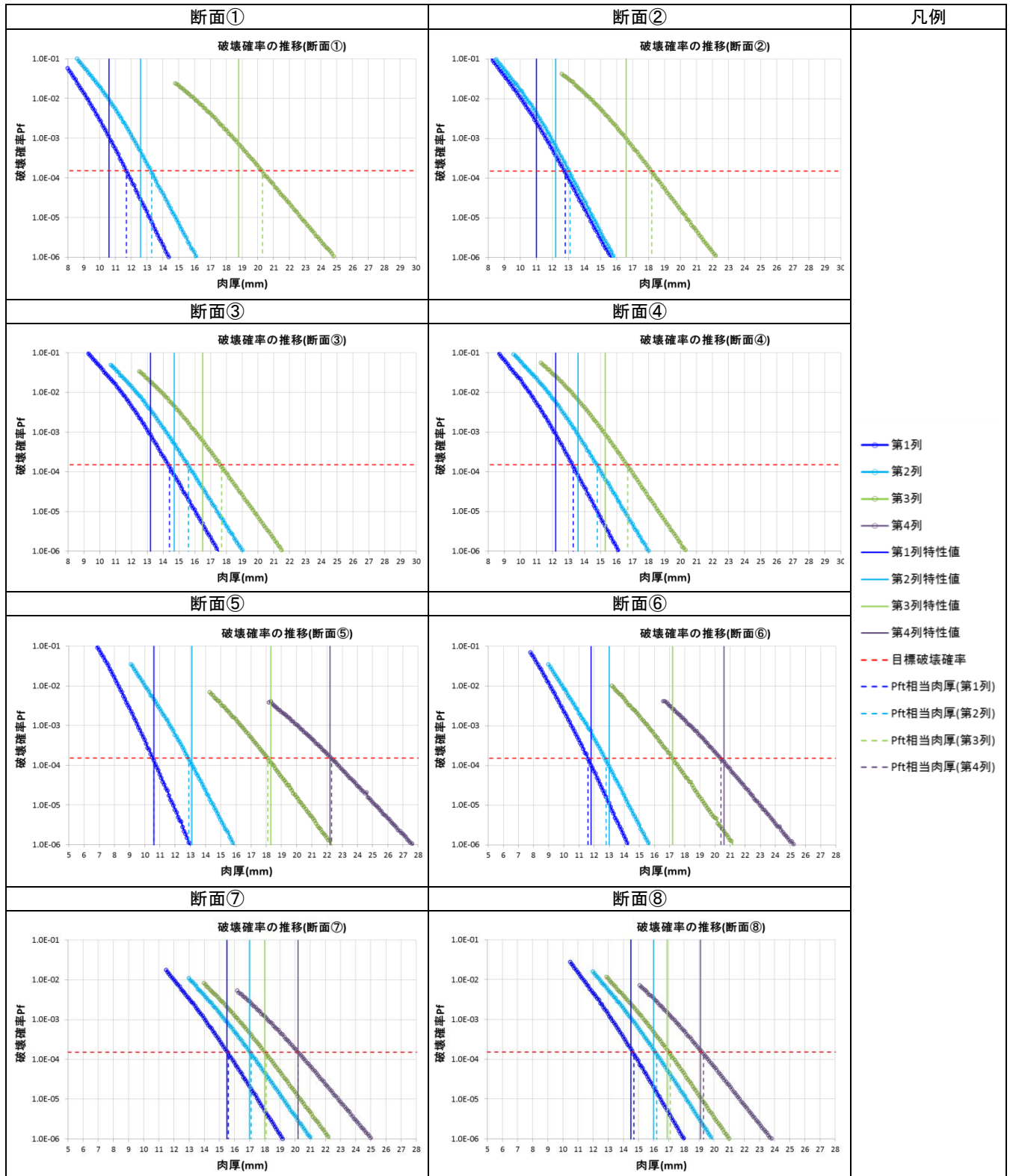
付表 G-4 肉厚ごとの破壊確率の推移と目標破壊確率相当の肉厚(断面①～⑧)
