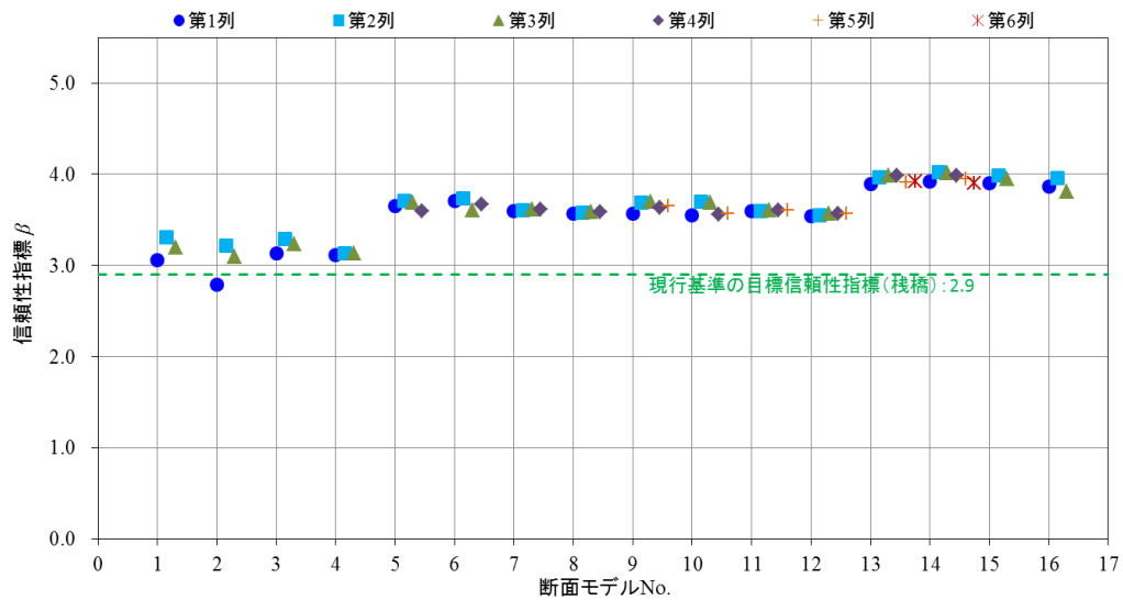
付図 F-7 各検討断面の信頼性指標(設定 B)
