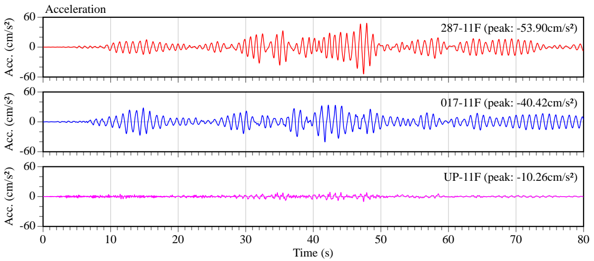
図 4.4-22 広島第2 合同庁舎11 階(11F)の加速度波形
