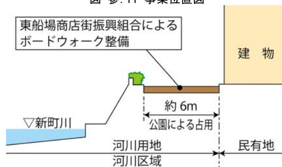
図-参. 12 ボードウォーク整備の横断イメージ図
