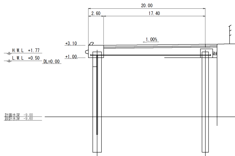
図-A. 12. 299 No. 21 塩釜港区_貞山ふ頭 2 号岸壁の断面図 (被災前)
