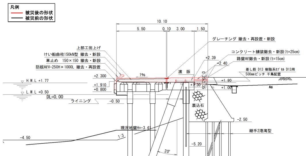
図-A. 12. 285 No. 16 塩釜港区_中ふ頭西側さん橋の断面図（復旧後）
