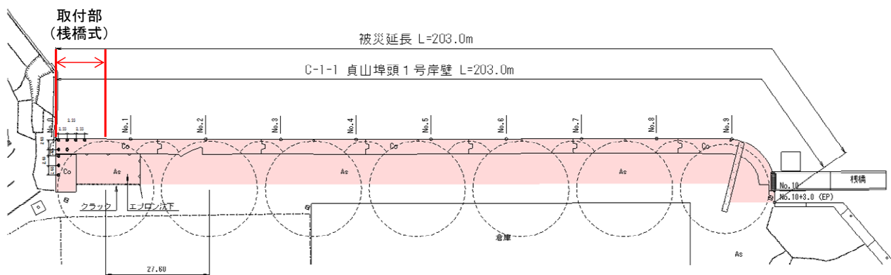
図一A.12.296 No. 20 塩釜港区_貞山ふ頭 1号岸壁の平面図 (被災後)
