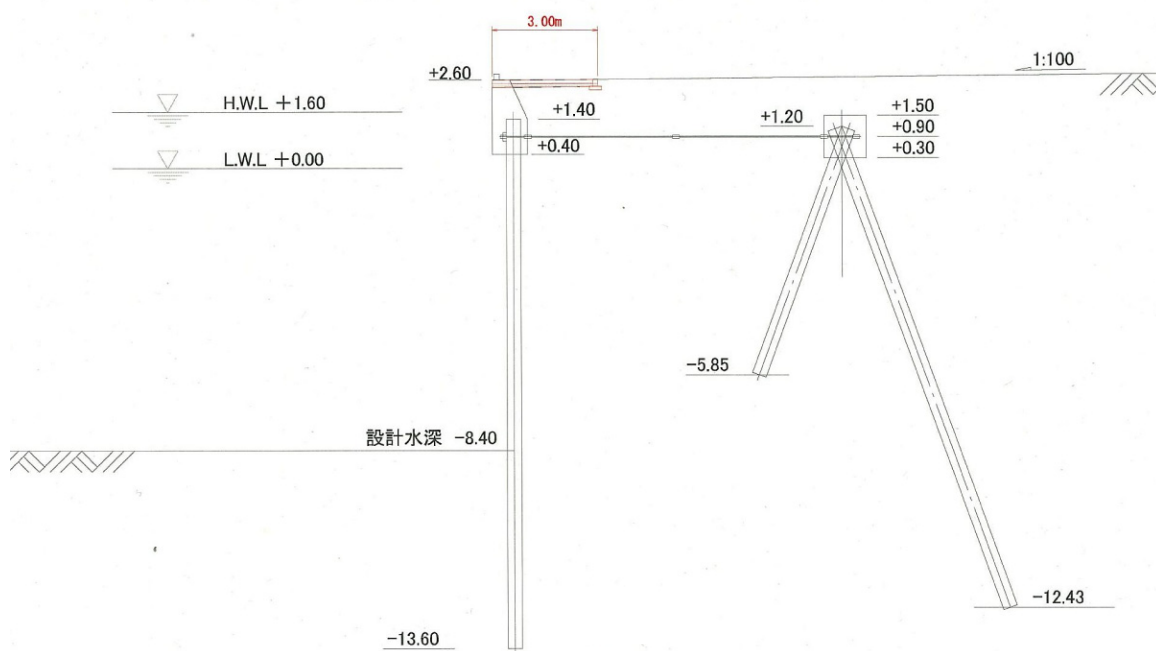
図-A. 12. 64 No. 5 仙台港区_中野地区_護岸Ⅱの断面図（復旧後）
