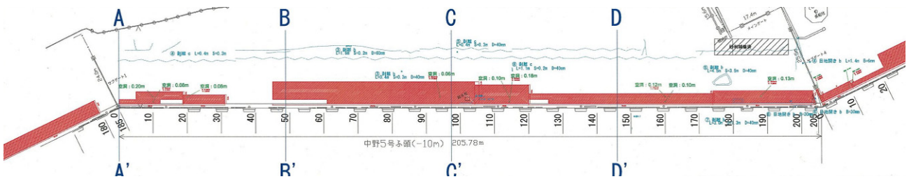
図-A.12.231 No.6 仙台港区_中野地区_5号岸壁 (-10m) の平面図 (被災後)
