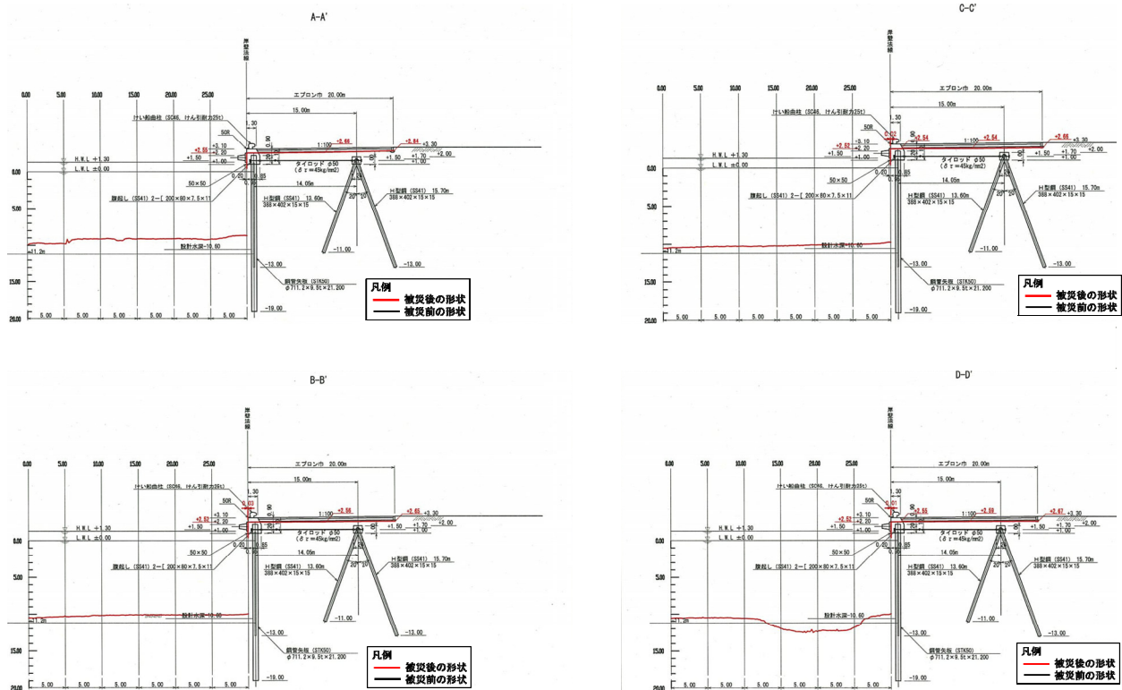
図-A.12.236 No.6 仙台港区_中野地区_6号岸壁 (-10m) の断面図 (被災後)
