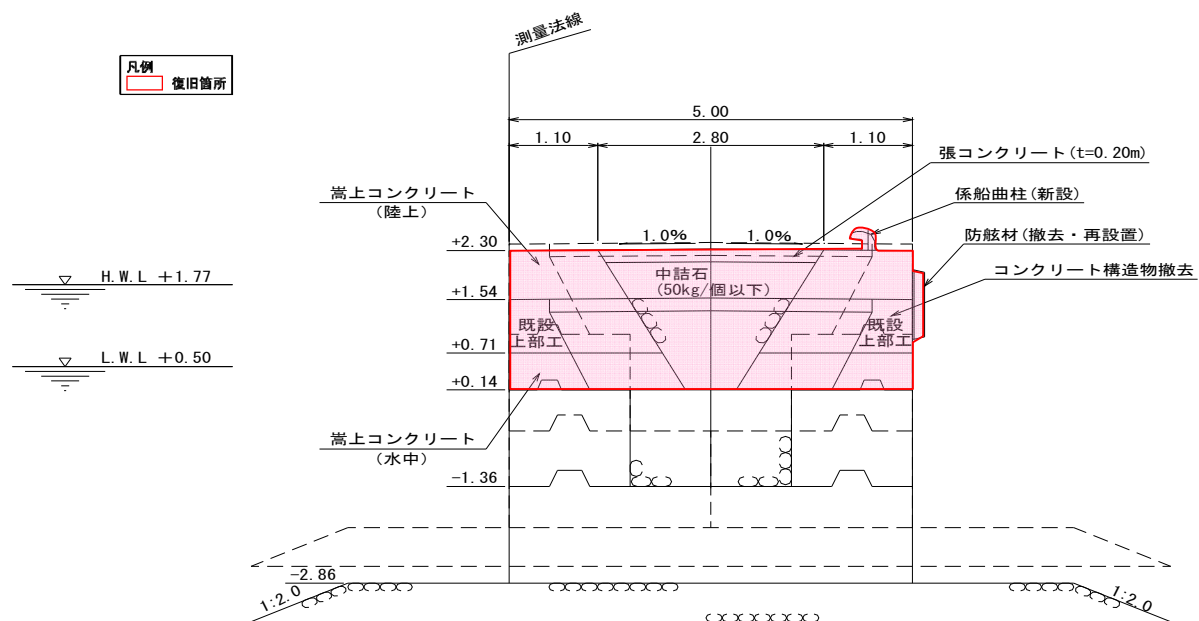
図-A.12.256 No.4 塩釜港区_石浜 (B) 物揚場の断面図 (復旧後)
