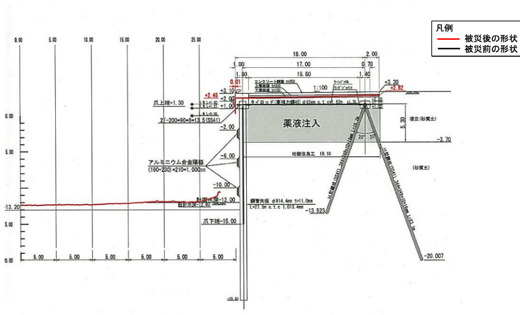
図-A. 12. 182 No.3 仙台区_中野地区_高松木材埠頭岸壁（-12m）の断面図 B-B'（被災後）
