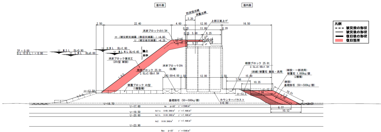
図-A.12.122 No.16 仙台区_新北防波堤の断面図 No.14 地点 (被災前・後_復旧後)
