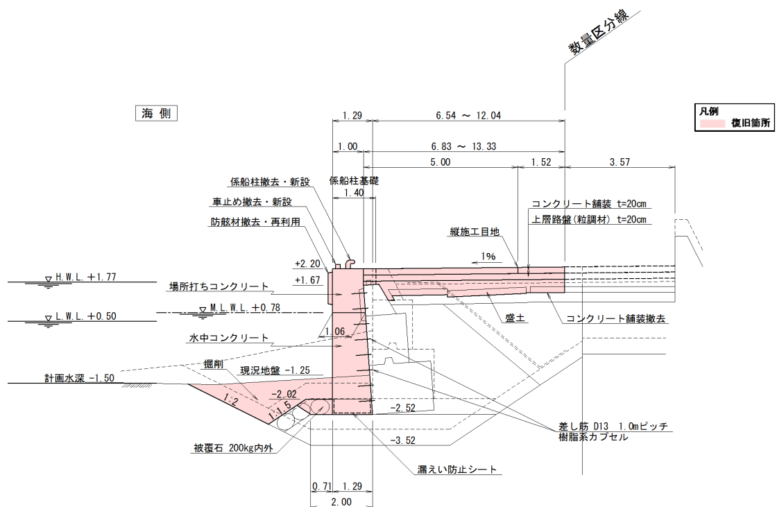
図-A.12.258 No.5 塩釜港区_代ヶ崎 (A) 物揚場の断面図 No.2 地点 (復旧後)
