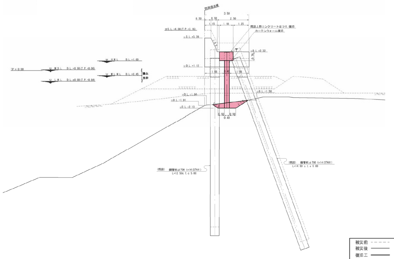
図-A. 12. 130 No. 17 仙台港区_高砂防波堤の断面図④ (被災後)
