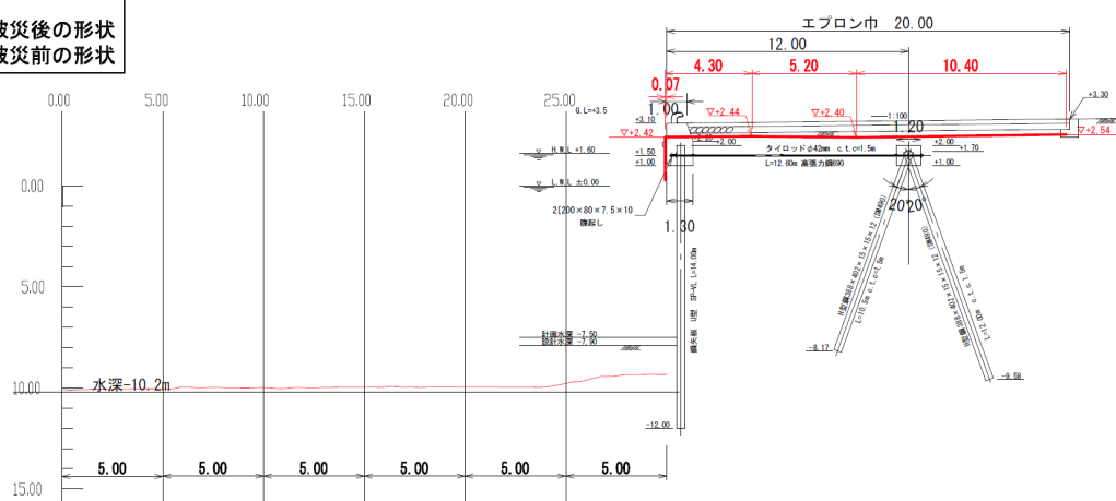
図-A.12.197 No.4 仙台港区_中野地区_岸壁 (-7.5m) の断面図 D-D' (被災後)
