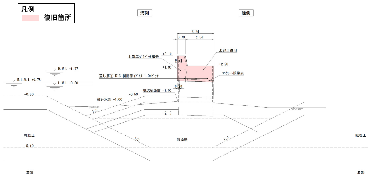
図－A.12.101 No.11 塩釜港区_東宮浜西側防波護岸の断面図No.2+4.66（復旧後）
