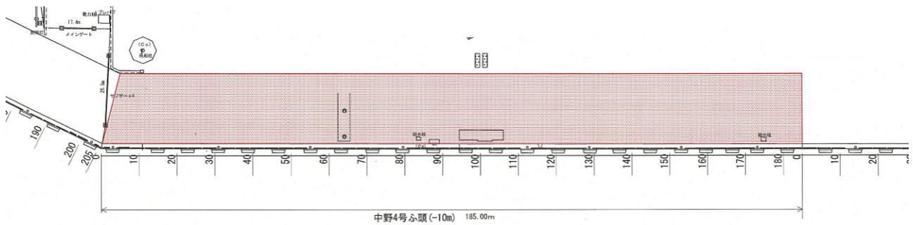
図-A. 12. 241 No.6 仙台港区_中野地区_4号岸壁 (-10m) の平面図 (復旧後)
