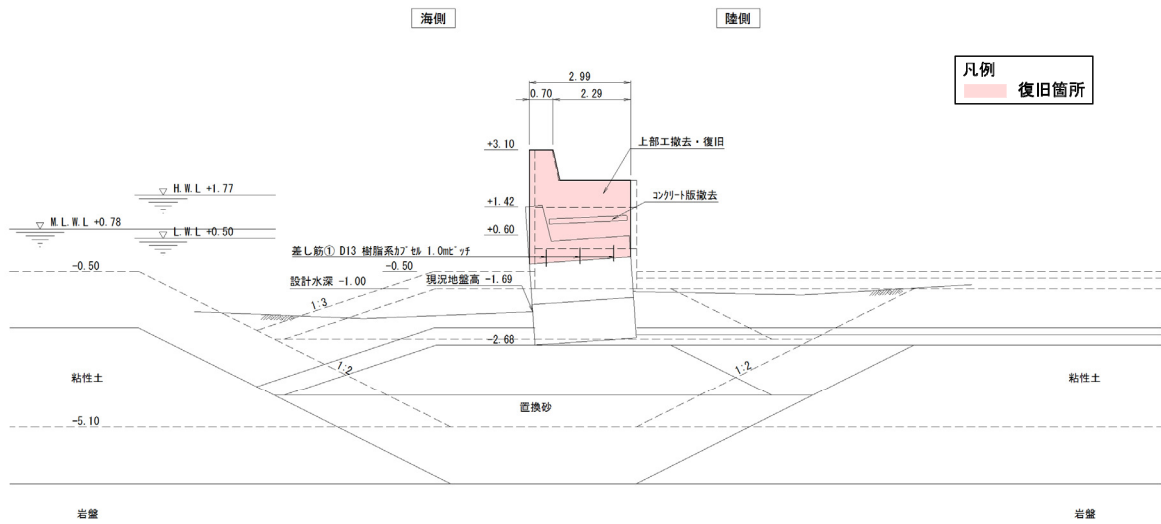
図-A.12.111 No. 14 塩釜港区_東宮浜東側防波護岸の断面図 No. 0 地点（復旧後）
