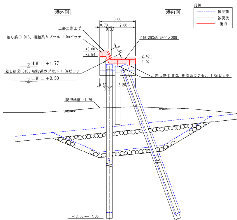
図-A.12.114 No. 15 塩釜港区_要害 (A) (B) 防波堤の断面図 (復旧後)
