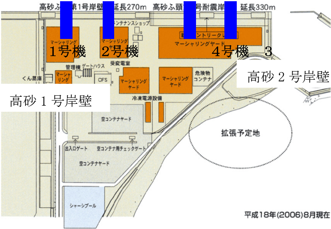
図－A. 12. 347 ガントリークレーンの設置位置
