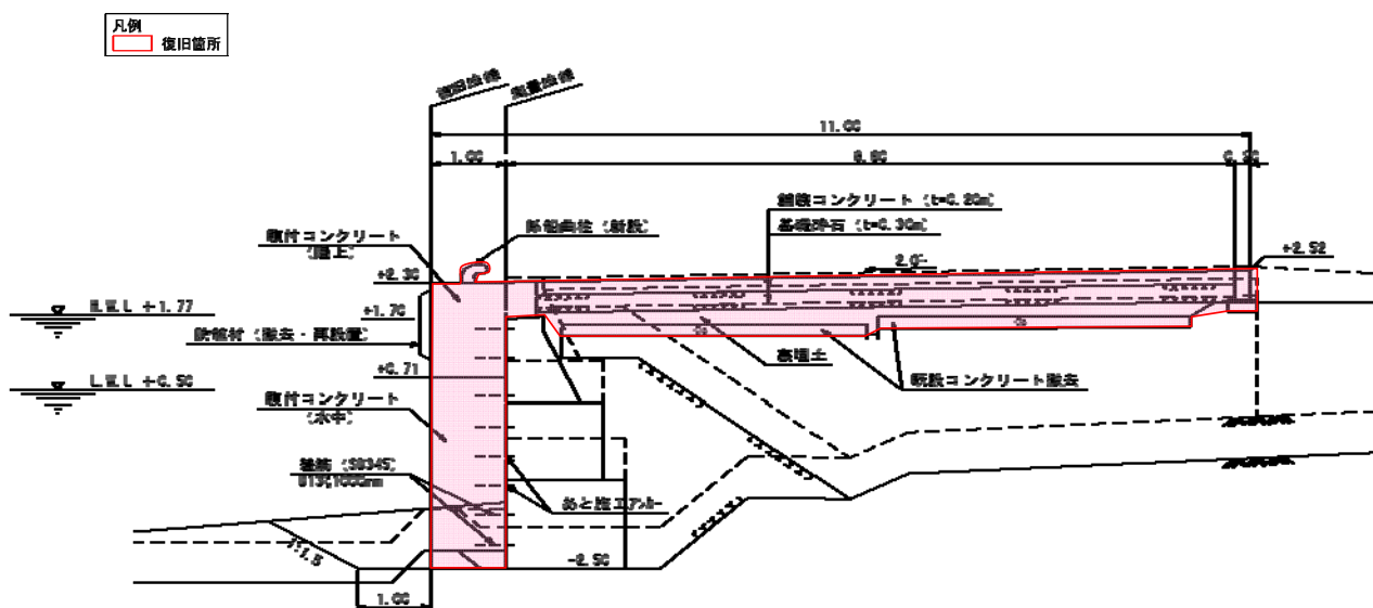
図－A.12.254 No.3 塩釜港区_石浜 (A) 物揚場の断面図（復旧後）
