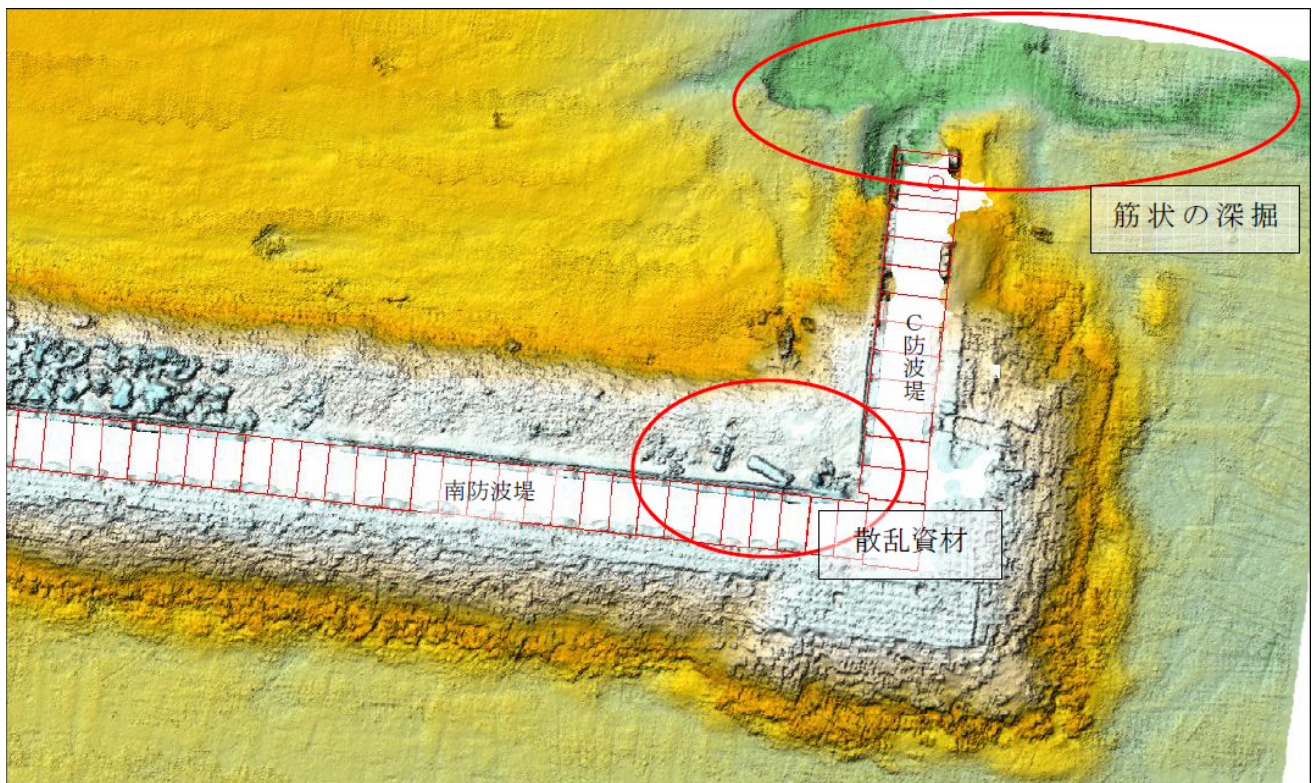
図-A. 12. 19 No. 2 仙台港区_外港地区_南防波堤の平面図（被災後）
