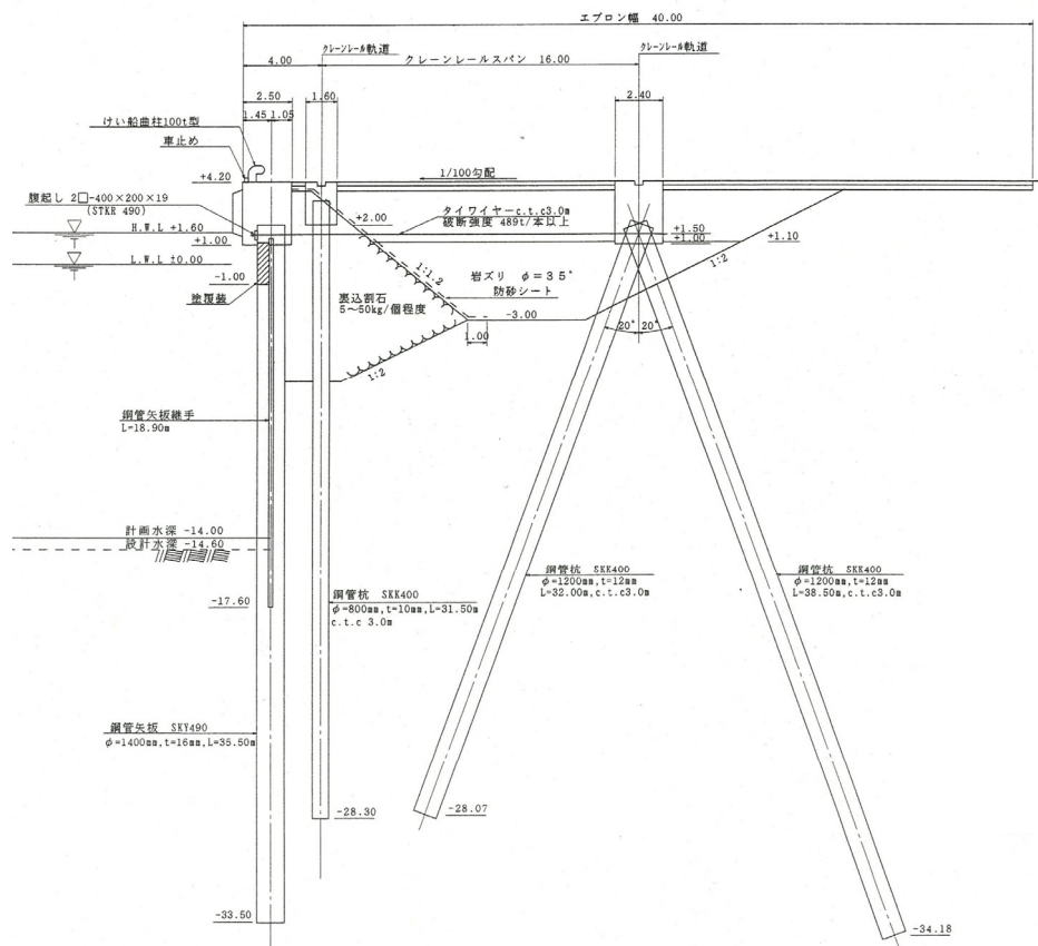
図-A.12.169 No.2 仙台港区_向洋地区_岸壁 (-14m) の断面図 (1区) (被災前)
