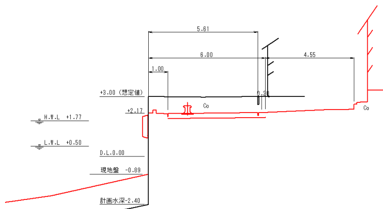
図-A. 12. 309 No. 23 塩釜港区_東ふ頭・中ふ頭間物揚場の断面図 (被災後)
