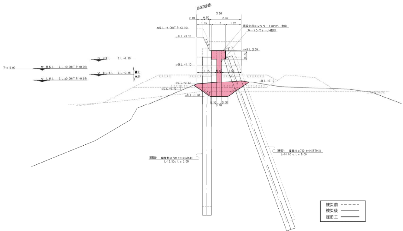
図-A.12.127 No. 17 仙台港区_高砂防波堤の断面図① (被災後)
