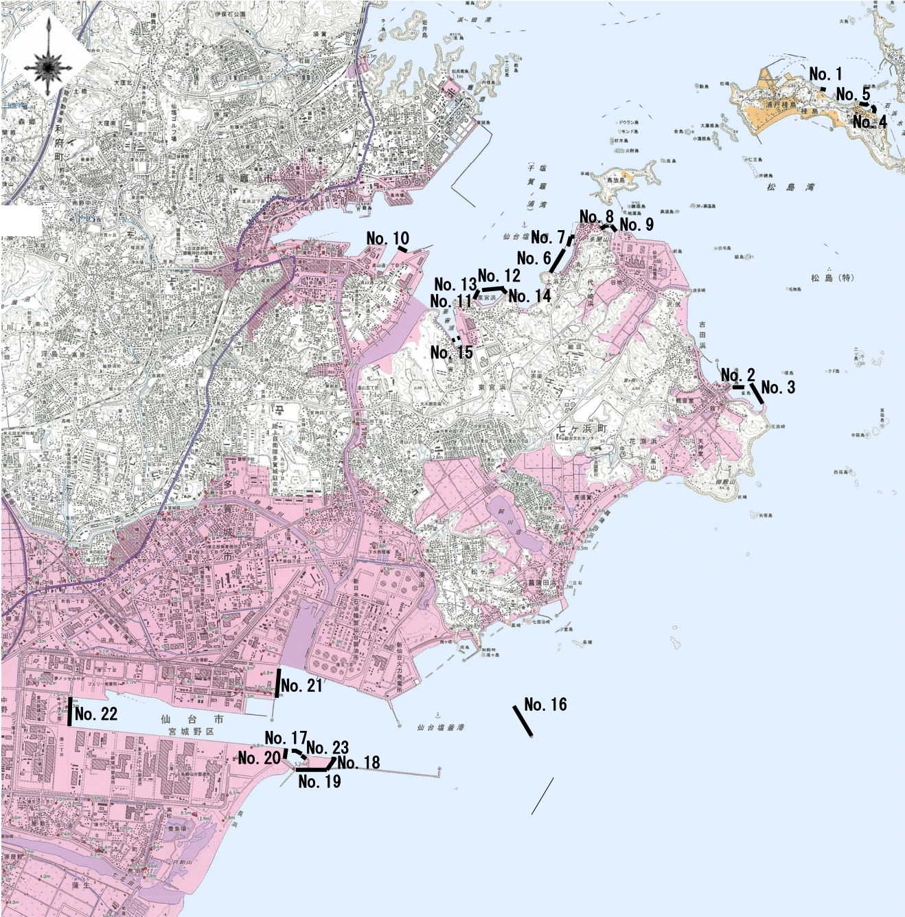
図-A. 12. 65 仙台塩釜港の被災港湾施設（外郭施設，補助分）
