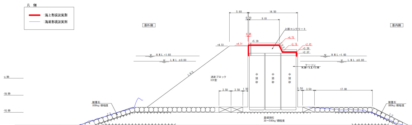
図-A.12.36 No.3 仙台港区_外港地区_沖防波堤の断面図 G-G' (被災後)
