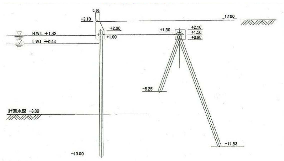
図一A. 12. 57 No. 5 仙台港区_中野地区_護岸Ⅱの断面図（被災前）
