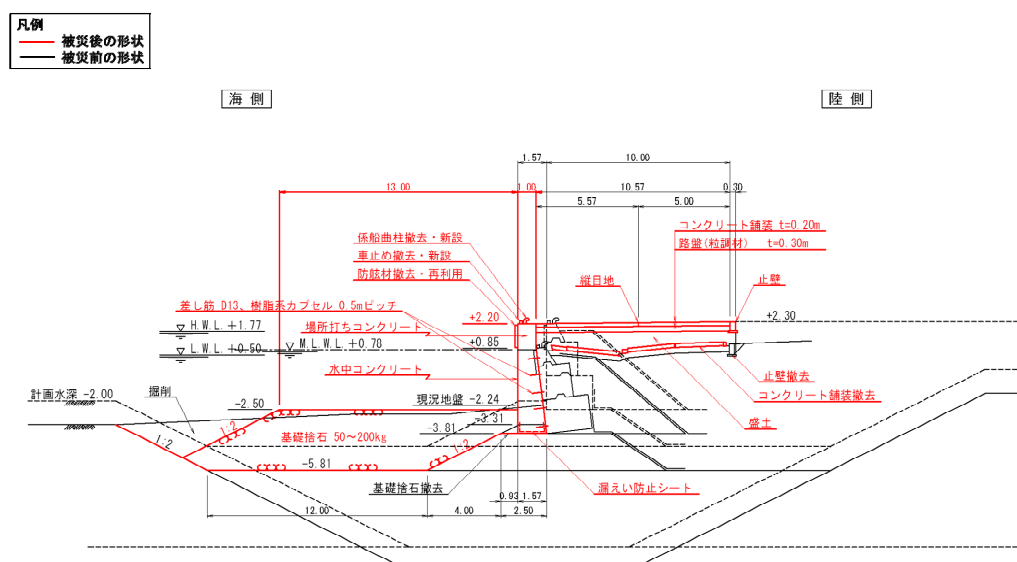
図-A.12.319 No.27 塩釜港区_東宮浜物揚場の断面図 No.5 地点 (復旧後)
