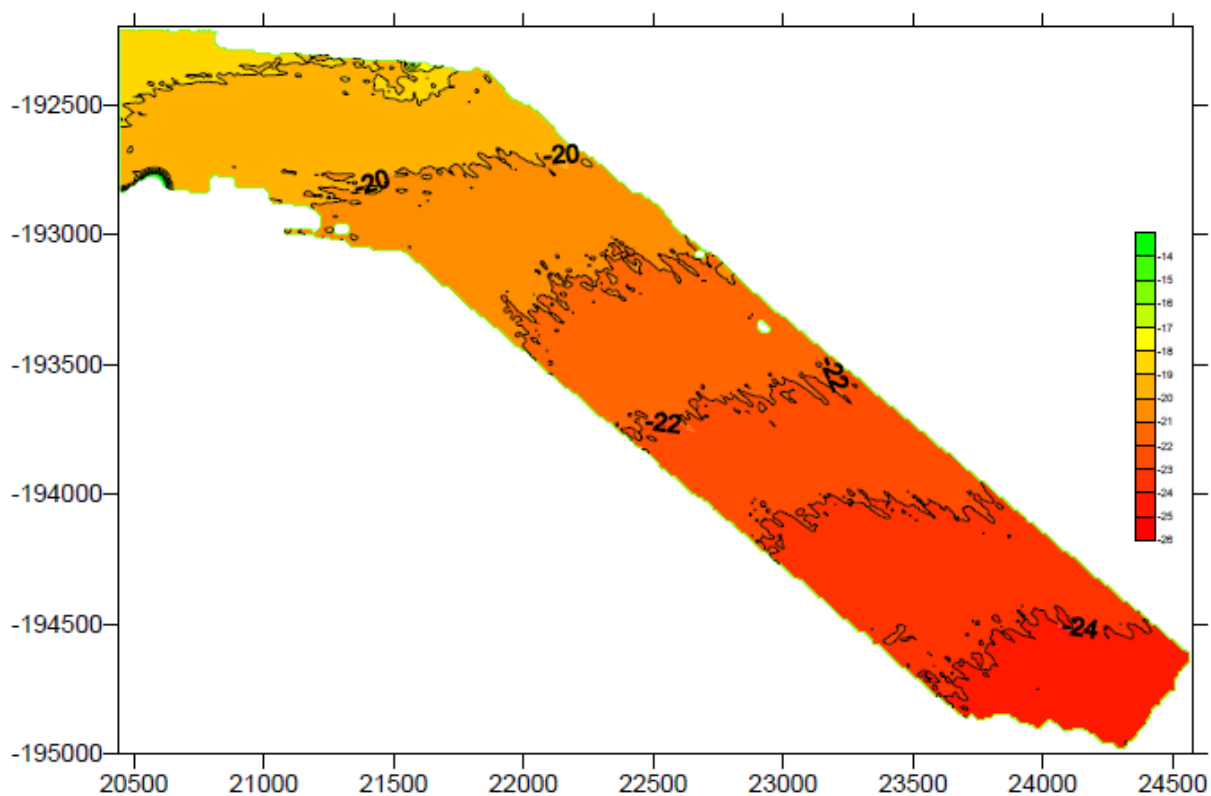
図-A.12.330 No.1 仙台港区_港外の深浅図
