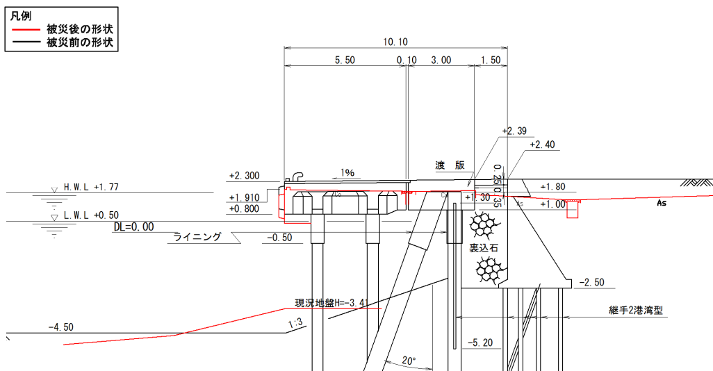
図-A. 12. 284 No. 16 塩釜港区_中ふ頭西側さん橋の断面図（被災後）
