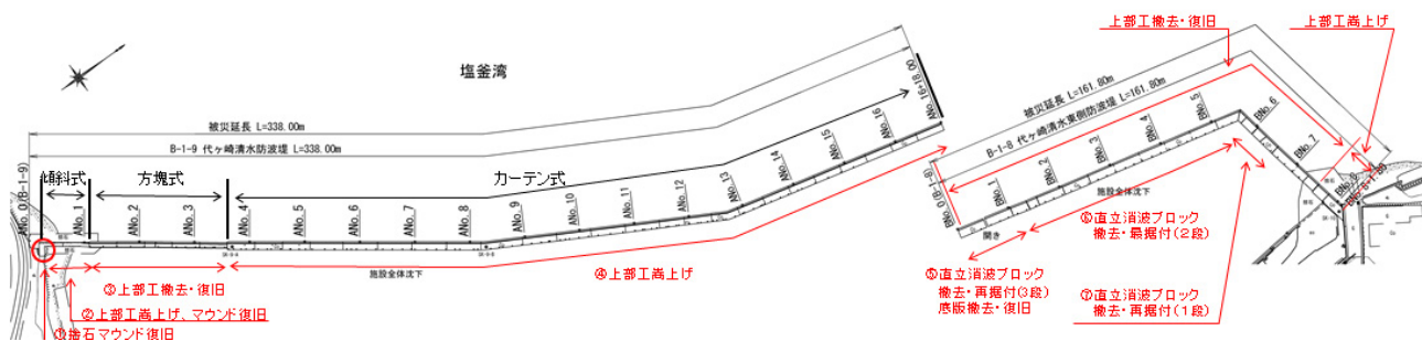
図-A.12.80 No.6 塩釜港区_代々崎清水防波堤の平面図（復旧後）
