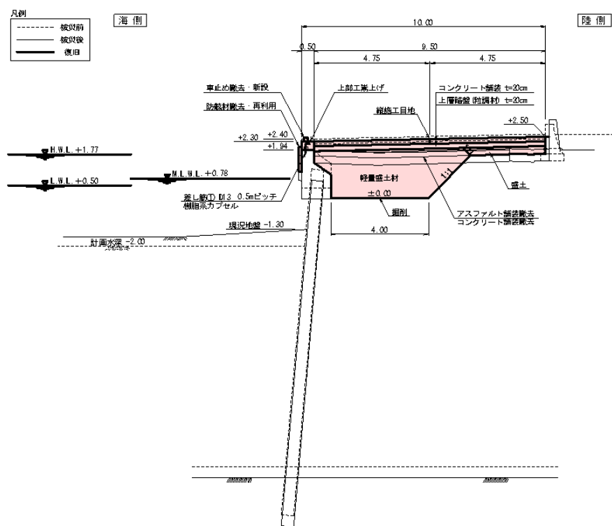
図-A. 12. 322 No. 28 塩釜港区_要害浦物揚場の断面図 No. 3 地点 (復旧後)
