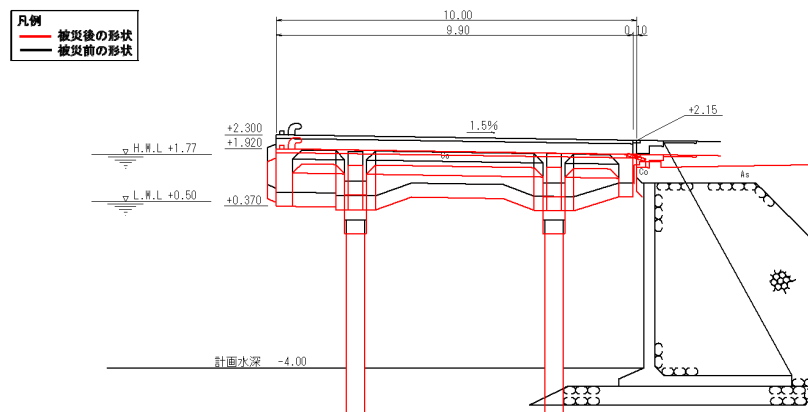
図-A.12.280 No. 15 塩釜港区_中ふ頭港橋前物揚場の断面図（被災後）
