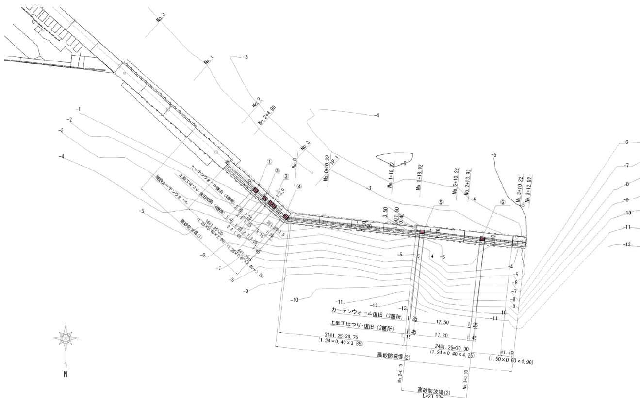
図-A.12.125 No.17 仙台港区_高砂防波堤の平面図 (被災後)
