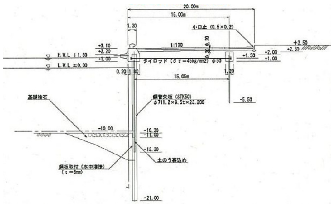
図-A. 12. 218 No.6 仙台港区_中野地区_3号岸壁 (-10m) の断面図 (被災前)
