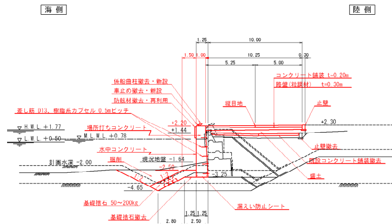
図一A. 12. 320 No. 27 塩釜港区_東宮浜物揚場の断面図 No11 地点 (復旧後)
