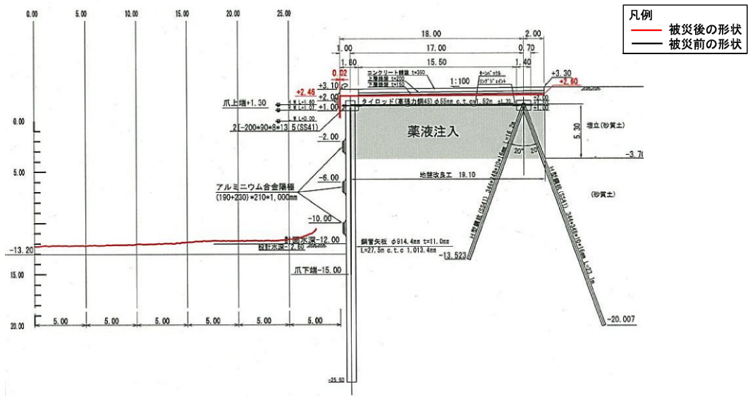
図-A. 12. 184 No.3 仙台港区_中野地区_高松木材埠頭岸壁 (-12m) の断面図 D-D' (被災後)
