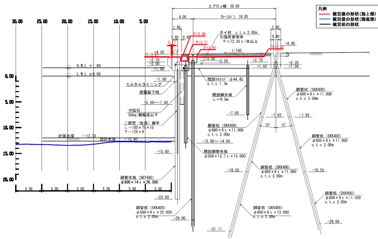
図-A.12.167 No.1 仙台港区_向洋地区_岸壁 (-12m) の断面図 E-E' (被災後)
