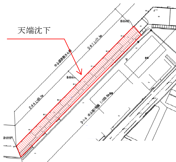
図一A. 12. 283 No. 16 塩釜港区_中ふ頭西側さん橋の平面図（被災後）
