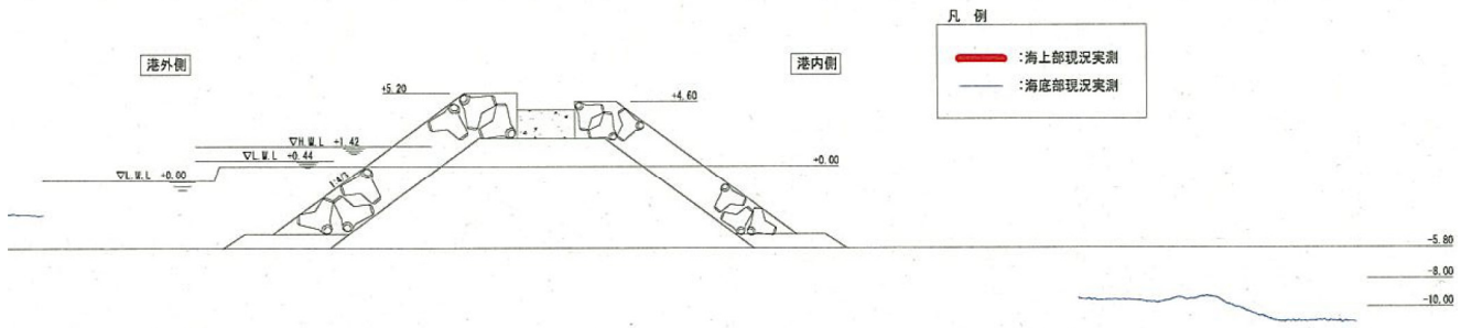
図-A.12.12 No.1 仙台港区_外港地区_北防波堤の断面図 A-A'（被災後）
