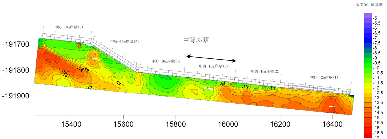
図-A.12.226 No.6 仙台港区_中野地区_3号岸壁 (-10m) のカラー段彩図 (被災後)
