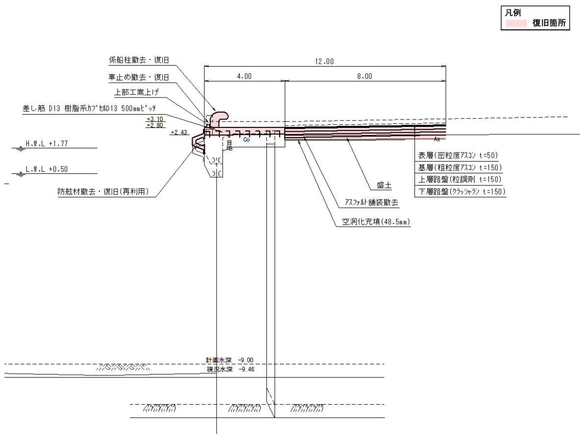
図一A.12.297 No. 20 塩釜港区_貞山ふ頭 1号岸壁の断面図 (標準部) (復旧後)
