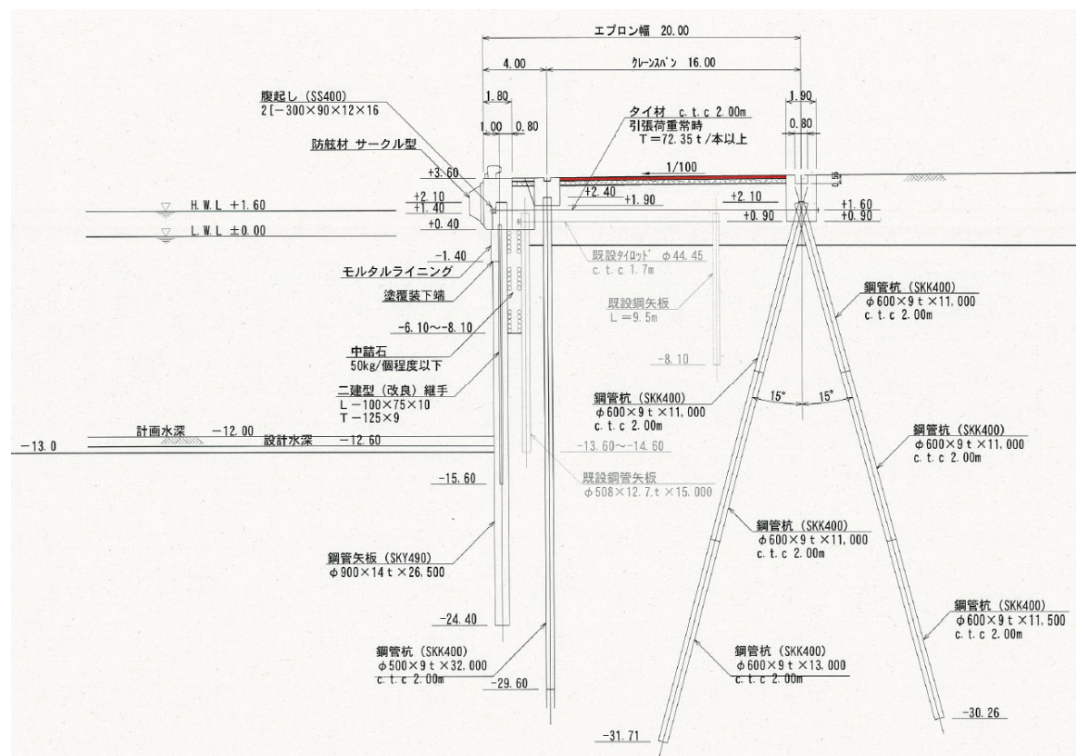
図-A.12.168 No.1 仙台港区_向洋地区_岸壁 (-12m) の断面図 (復旧後)
