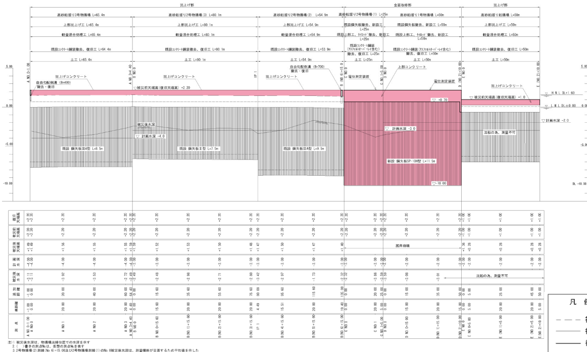
図一A.12.327 No. 30 仙台港区_高砂船溜物揚場の縦断面図（被災後）
