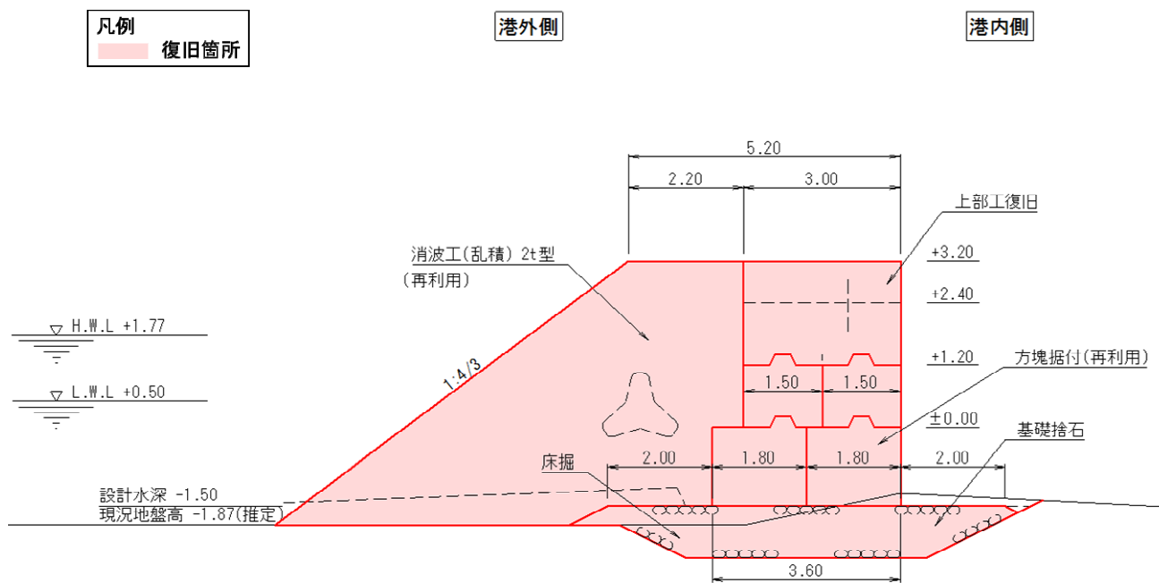
図-A. 12. 91 No. 8 塩釜港区_代ヶ崎東防波堤の断面図 A-2 区間 (復旧後)
