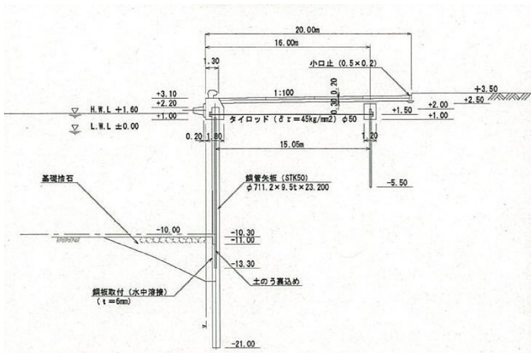
図-A. 12. 217 No.6 仙台港区_中野地区_2号岸壁 (-10m) の断面図 (被災前)
