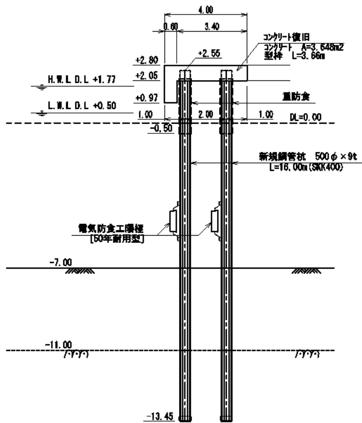
図-A. 12. 298 No. 20 塩釜港区_貞山ふ頭 1 号岸壁の断面図 (基部) (復旧後)
