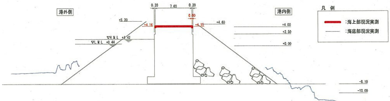
図-A.12.13 No.1 仙台港区_外港地区_北防波堤の断面図 B-B'（被災後）
