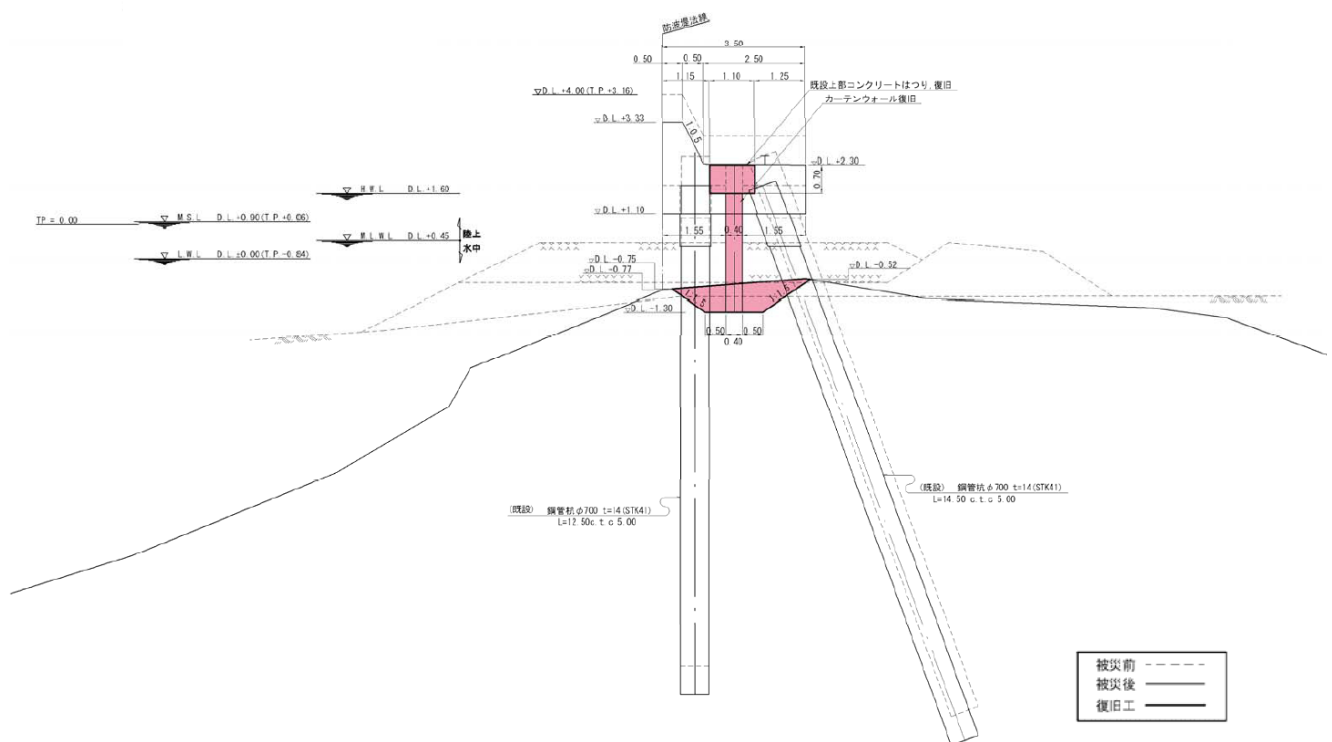
図-A.12.128 No. 17 仙台港区_高砂防波堤の断面図② (被災後)
