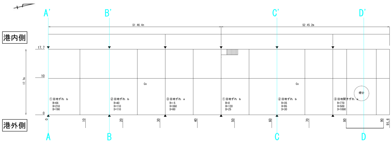
図-A.12.47 No.4 仙台港区_外港地区_C防波堤の平面図(被災後)
