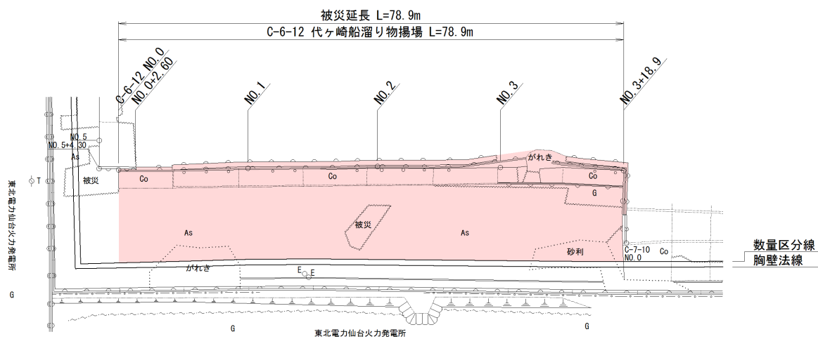
図-A.12.274 No.13 塩釜港区_代ヶ崎船たまり物揚場の閉平面図（被災後）
