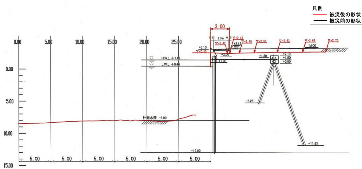
図-A. 12. 62 No. 5 仙台港区_中野地区_護岸Ⅱの断面図 D-D' (被災後)
