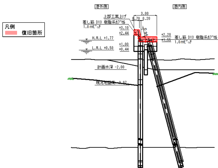
図-A.12.105 No.12 塩釜港区_東宮浜東防波堤の断面図（復旧後）
