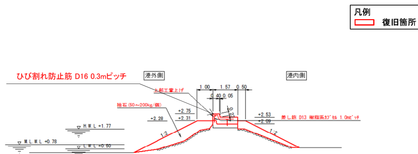
図-A.12.81 No.6 塩釜港区_代々崎清水防波堤の断面図 ANo.1（復旧後）
