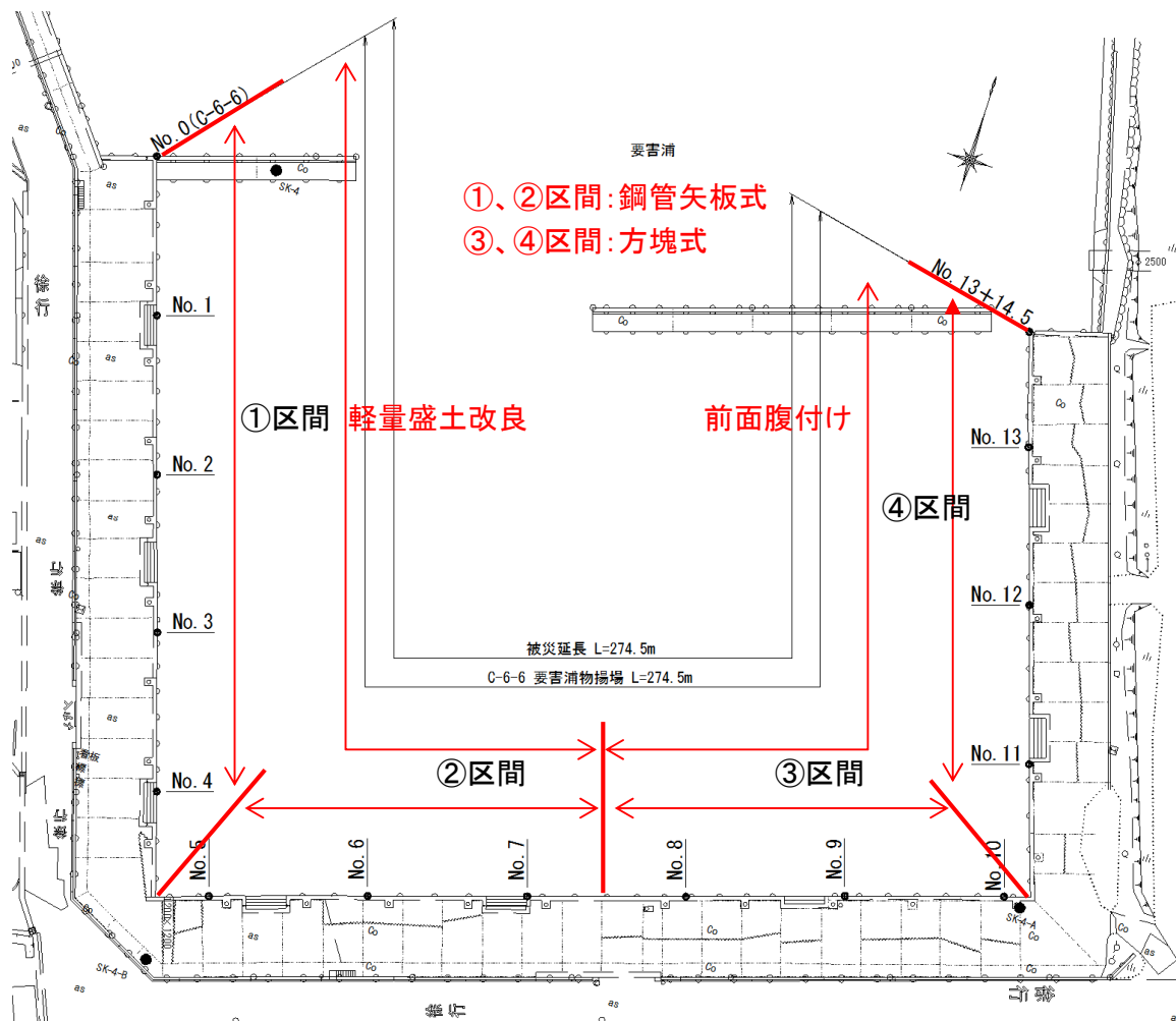
図-A.12.321 No.28 塩釜港区_要害浦物揚場の平面図（被災後）
