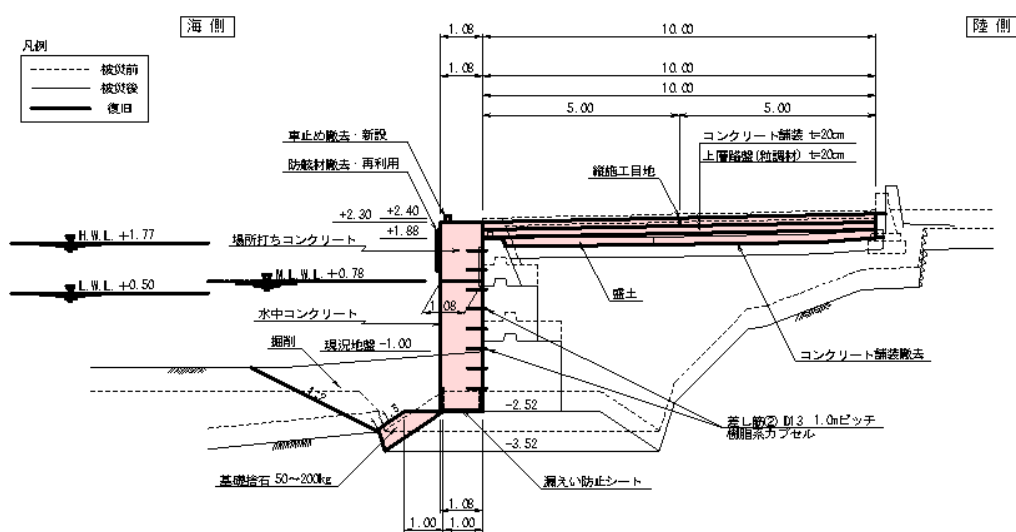
図-A. 12. 323 No. 28 塩釜港区_要害浦物揚場の断面図 No. 9 地点 (復旧後)
