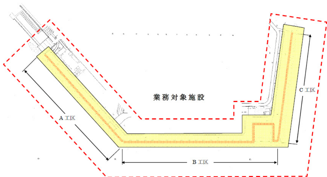
図-A.12.340 No.3 仙台港区_栄地区埋立護岸 ABC 工区の平面図（被災前）
