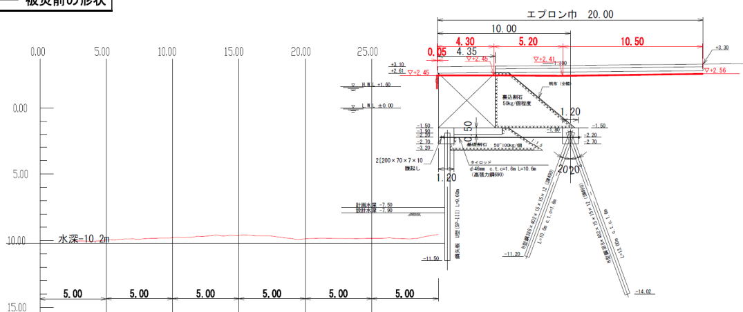
図-A. 12. 195 No.4 仙台港区_中野地区_岸壁 (-7.5m) の断面図 B-B' (被災後)
