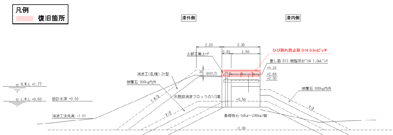
図-A.12.93 No. 9 塩釜港区_代ヶ崎防波堤の断面図 B-1 区間（復旧後）
