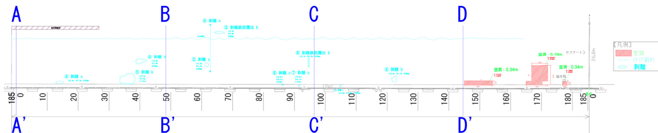
図-A.12.222 No.6 仙台港区_中野地区_2号岸壁 (-10m) の平面図 (被災後)
