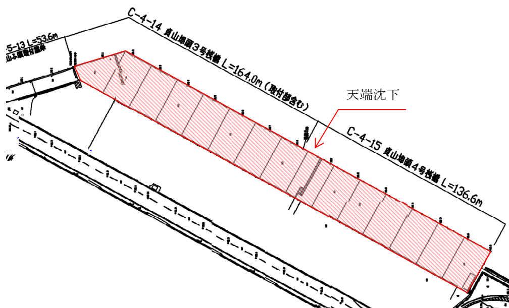
図-A. 12. 304 No. 22 塩釜港区_貞山ふ頭 3 号・4 号さん橋の平面図 (被災後)
