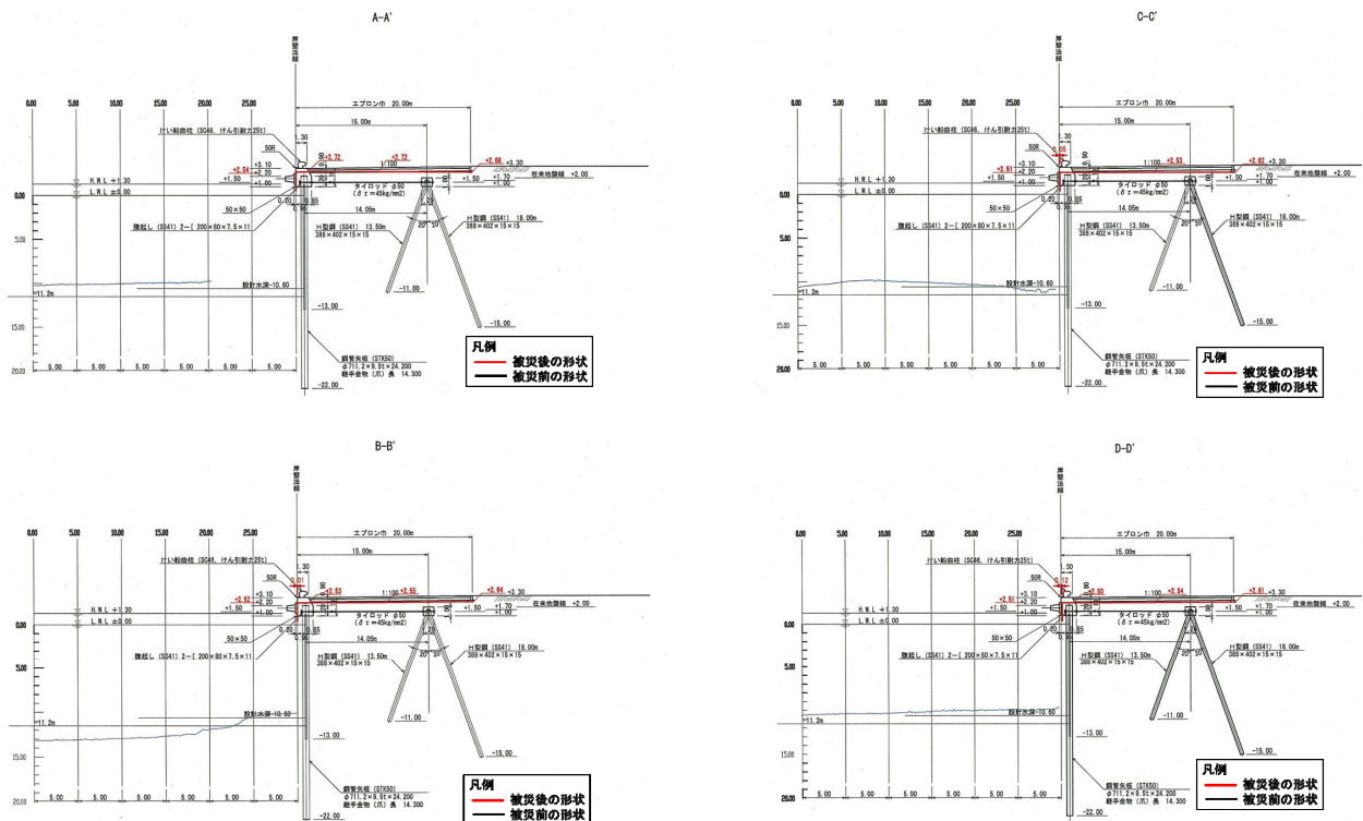
図-A.12.233 No.6 仙台港区_中野地区_5号岸壁 (-10m) の断面図 (被災後)
