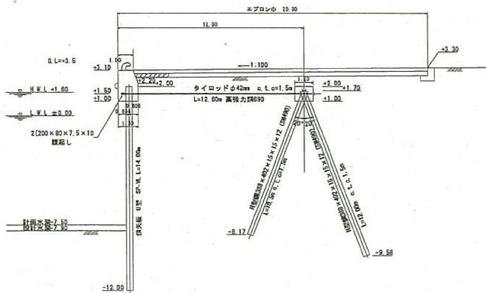
図-A. 12. 191 No.4 仙台港区_中野地区_岸壁 (-7.5m) の断面図 B-B (被災前)
