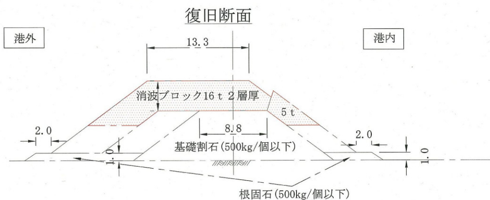
図-A.12.17 No.1 仙台港区_外港地区_北防波堤の断面図 A-A' (復旧後)
