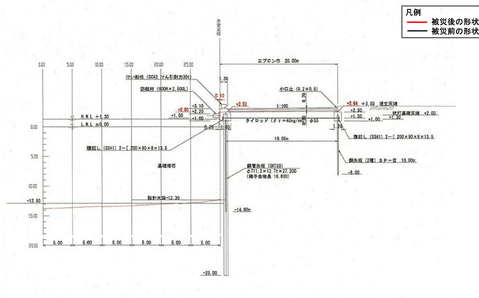
図-A.12.214 No.5 仙台港区_中野地区_岸壁 (-12m) の断面図 F・F' (被災後)
