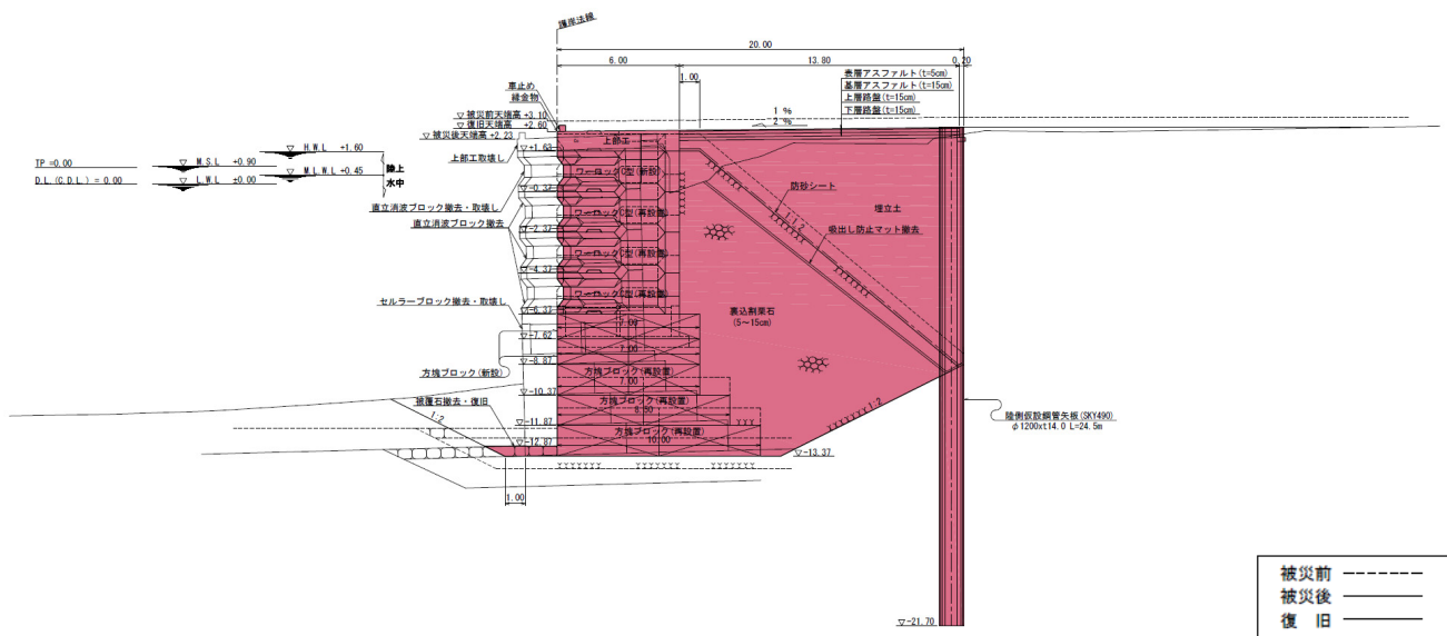
図-A.12.151 No. 21 仙台港区_北航路西C護岸の断面図（被災後）
