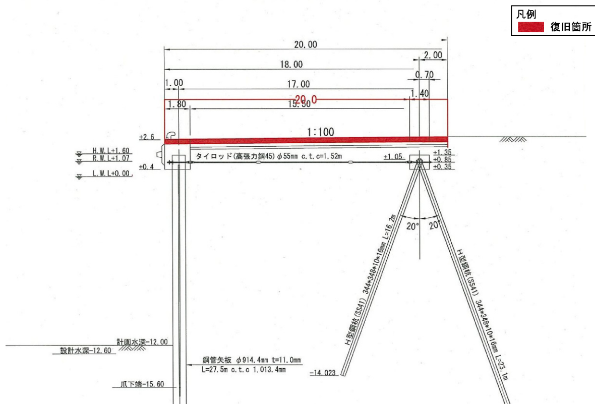
図-A. 12. 189 No.3 仙台港区_中野地区_高松木材埠頭岸壁 (-12m) の断面図 B-B' (復旧後)
