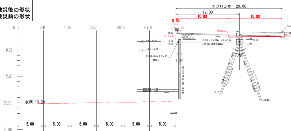
図-A.12.199 No.4 仙台港区_中野地区_岸壁 (-7.5m) の断面図 F-F' (被災後)
