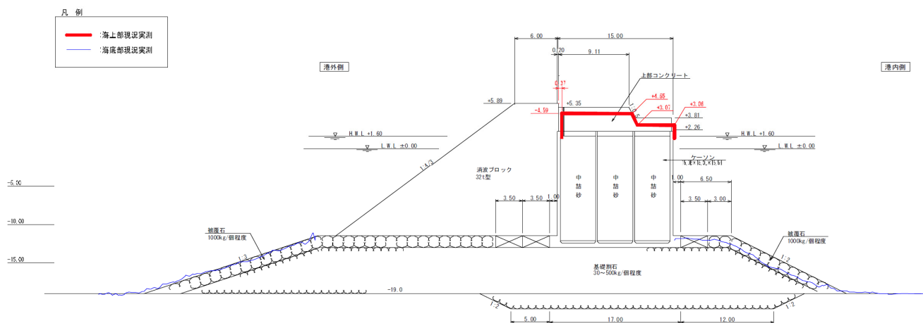
図-A.12.32 No.3 仙台港区_外港地区_沖防波堤の断面図 D-D' (被災後)
