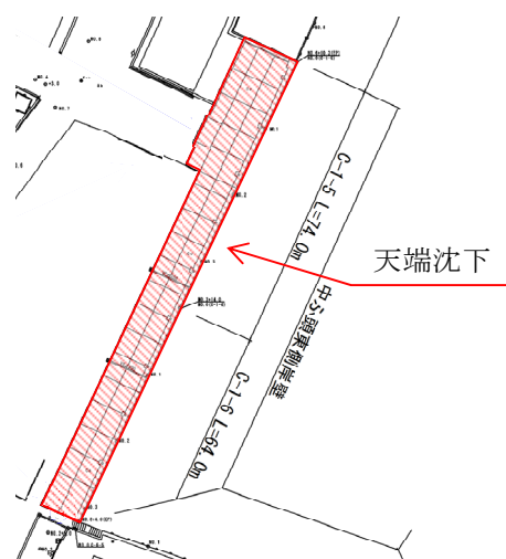
図-A.12.291 No. 18 塩釜港区_中ふ頭東側岸壁の平面図（被災後）
