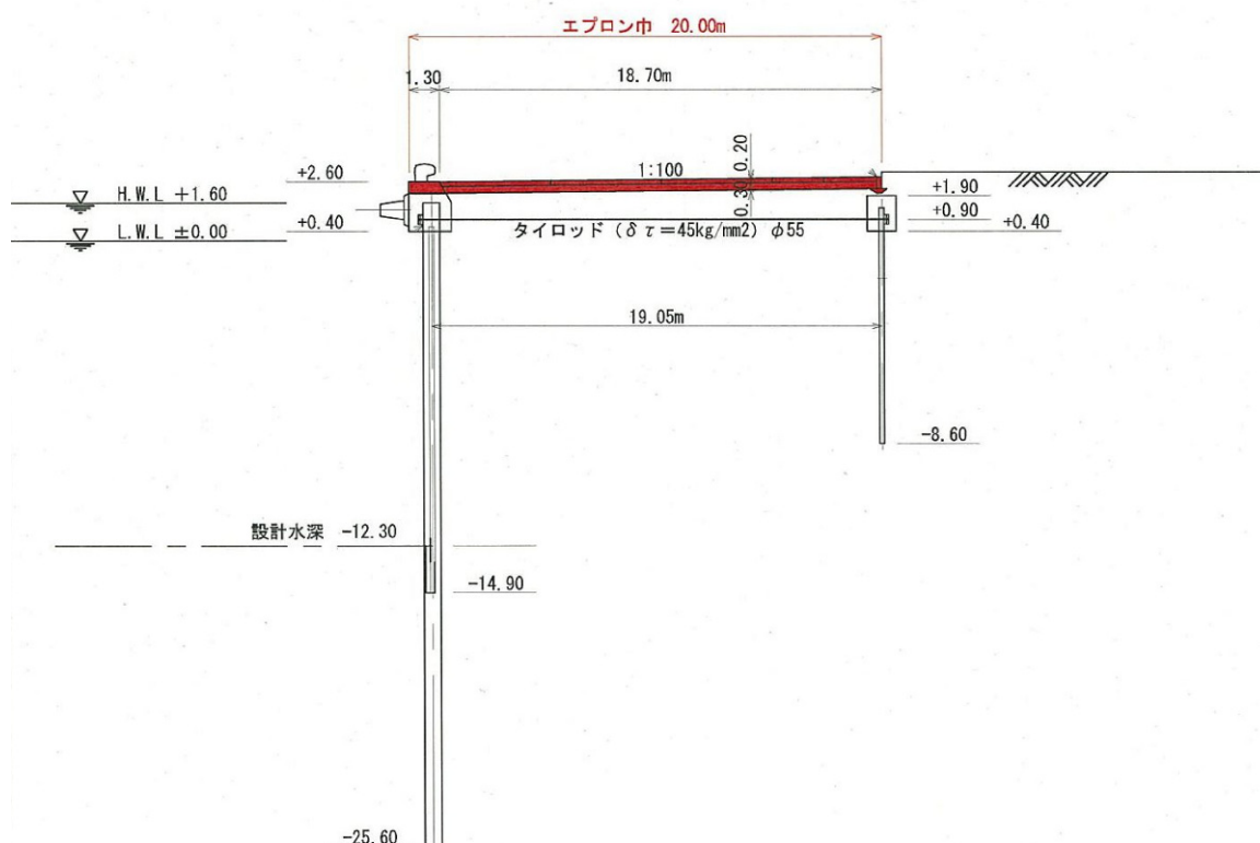
図-A. 12. 216 No.5 仙台港区_中野地区_岸壁 (-12m) の断面図 (復旧後)
