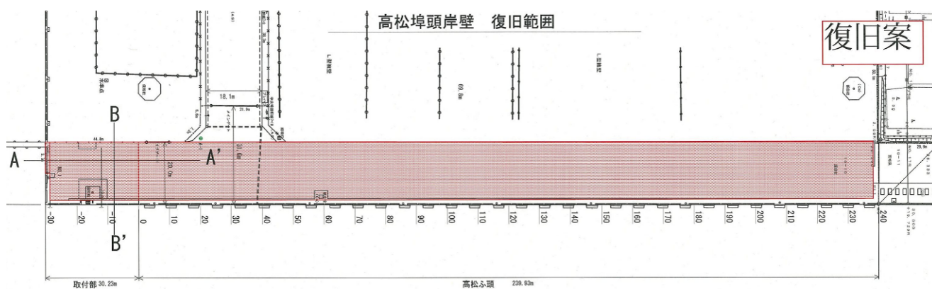
図-A.12.187 No.3 仙台港区_中野地区_高松木材埠頭岸壁 (-12m) の平面図 (復旧後)
