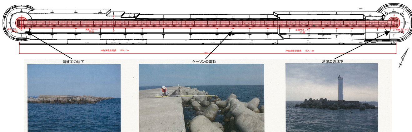
図-A.12.27 No.3 仙台港区_外港地区_沖防波堤の平面図（被災後）
