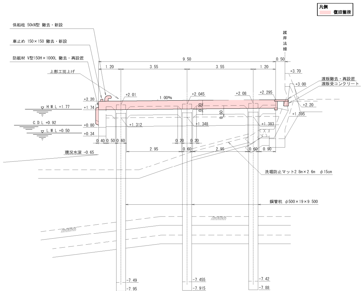
図-A.12.265 No. 8 塩釜港区_代ヶ崎清水 (A) さん橋の断面図 (復旧後)
