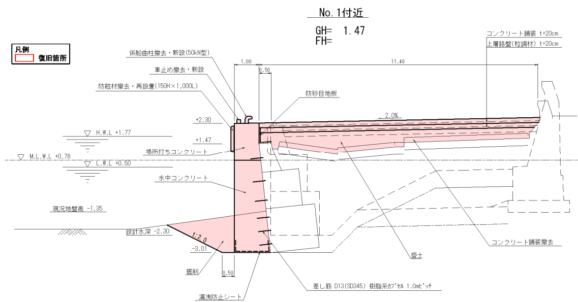
図-A.12.251 No.2 塩釜港区_小浜物揚場の断面図（復旧後）
