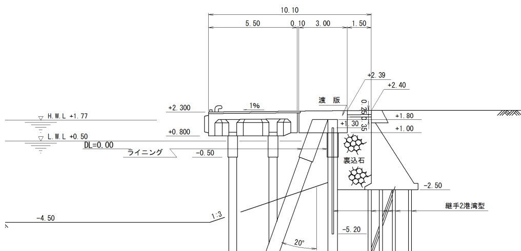
図一A. 12. 282 No. 16 塩釜港区_中ふ頭西側さん橋の断面図（被災前）
