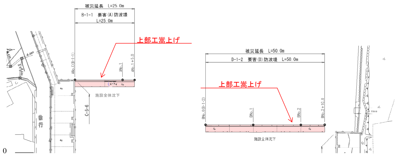
図-A.12.113 No.15 塩釜港区_要害(A) (B) 防波堤の平面図(被災後)
