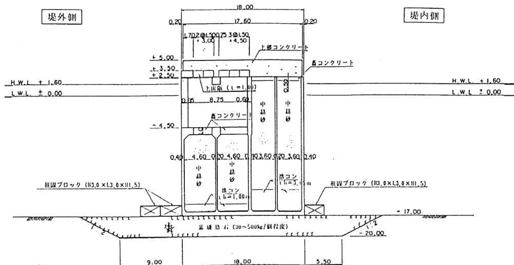
図-A.12.43 No.4 仙台港区_外港地区_C防波堤の断面図 (被災前)
