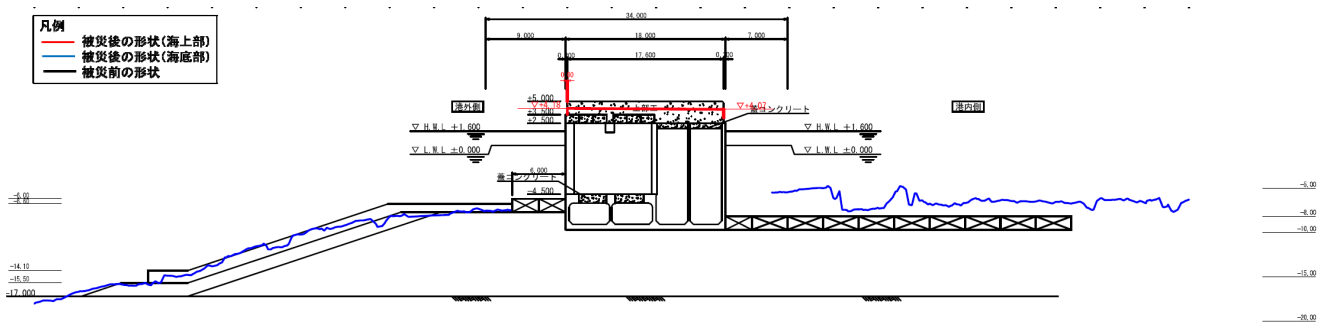
図-A.12.48 No.4 仙台港区_外港地区_C防波堤の断面図 A-A' (被災後)
