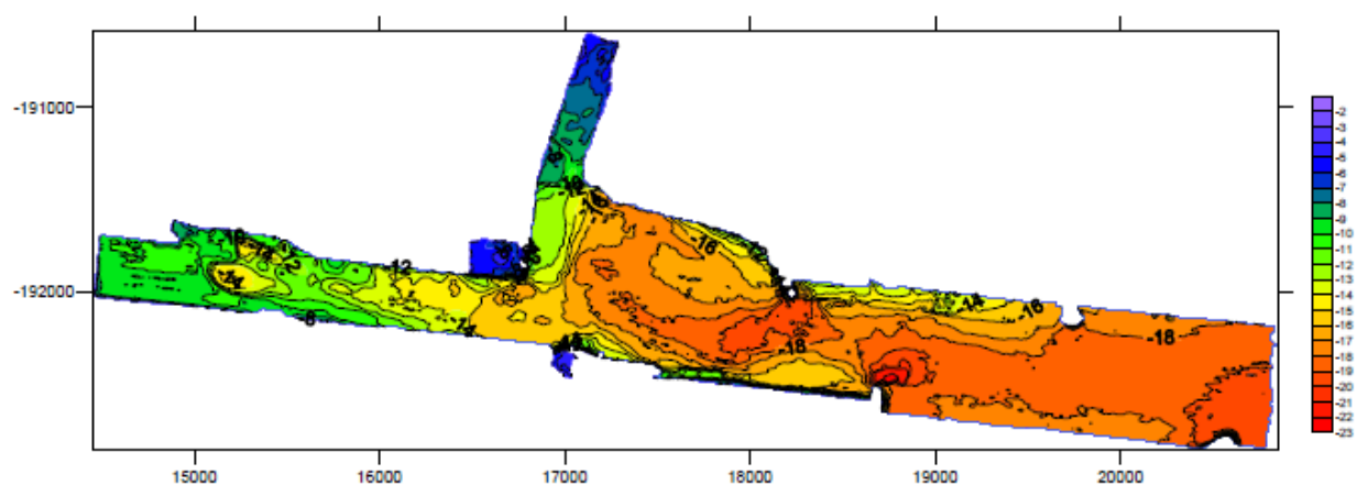
図-A.12.331 No.2 仙台港区_港外の深浅図
