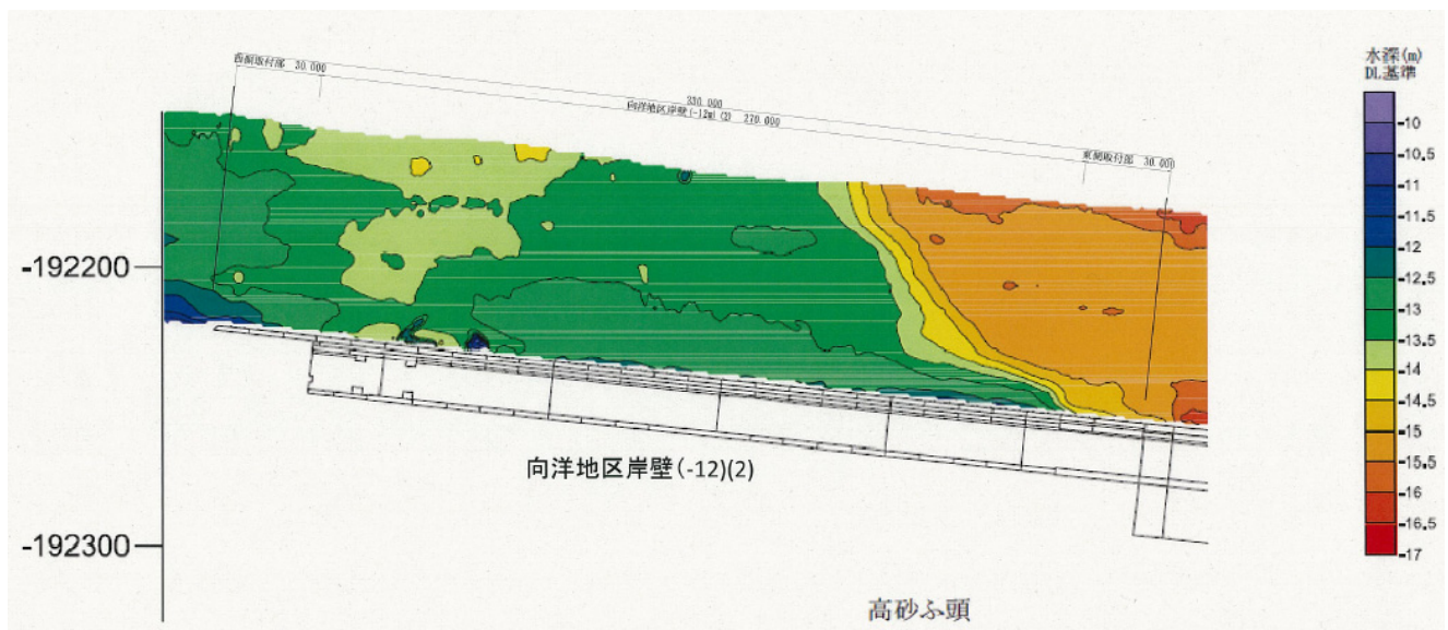
図-A.12.162 No.1 仙台港区_向洋地区_岸壁 (-12m) のカラー段彩図 (被災後)
