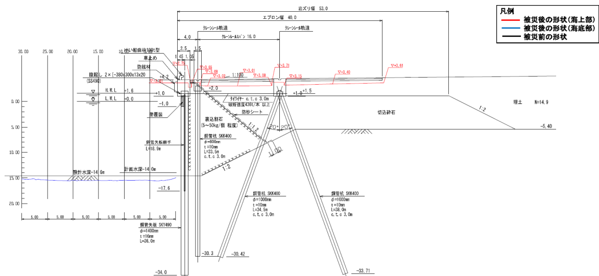
図-A. 12. 173 No.2 仙台港区_向洋地区_岸壁 (-14m) の断面図 B-B' (被災後)
