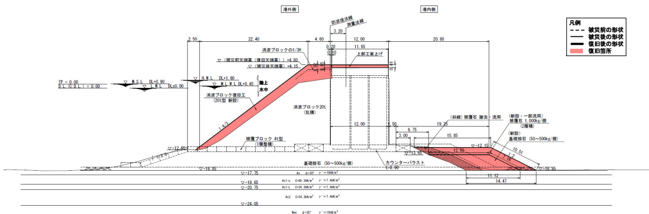
図-A.12.123 No.16 仙台区_新北防波堤の断面図 No.17 地点 (被災前・後_復旧後)
