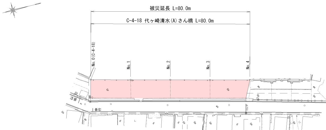
図-A.12.264 No. 8 塩釜港区_代ヶ崎清水 (A) さん橋の平面図 (被災後)
