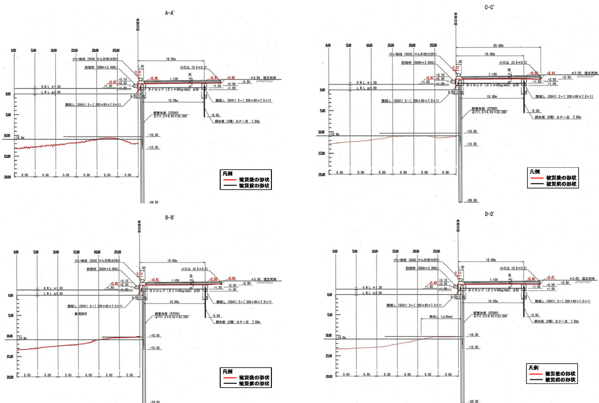
図-A.12.224 No.6 仙台港区_中野地区_2号岸壁 (-10m) の断面図 (被災後)
