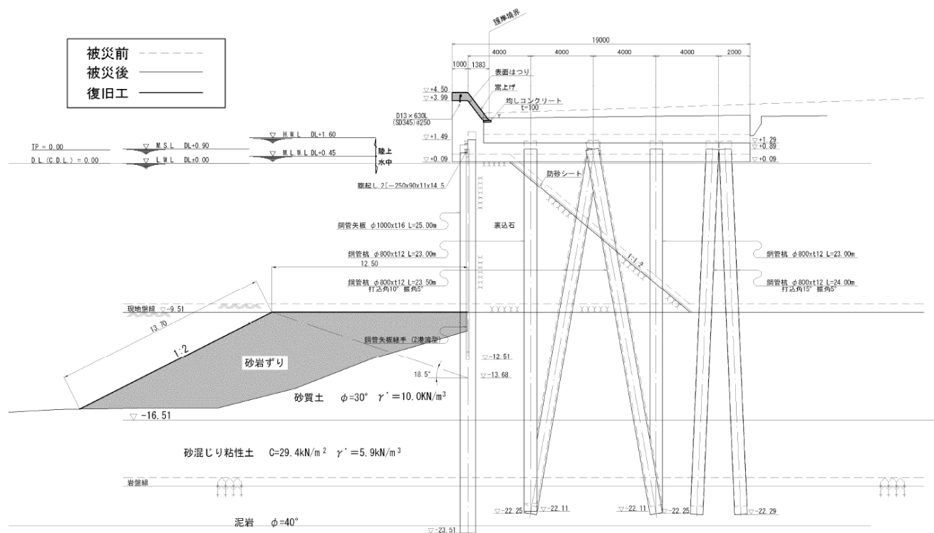
図-A. 12. 136 No. 18 仙台港区_向洋ふ頭防波護岸の断面図 (復旧後)
