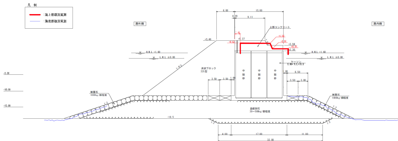
図-A.12.34 No.3 仙台区_外港地区_沖防波堤の断面図 E-E' (被災後)
