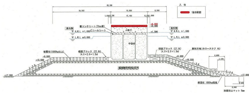
図-A.12.26 No.2 仙台港区_外港地区_南防波堤の断面図 D-D' (復旧後)
