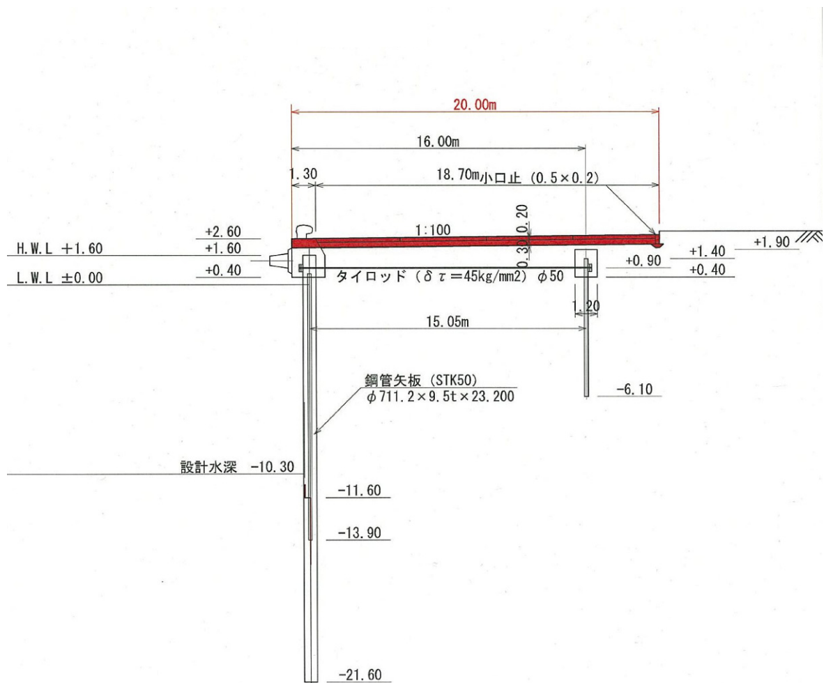
図-A. 12. 242 No.6 仙台港区_中野地区_4号岸壁 (-10m) の断面図 (復旧後)
