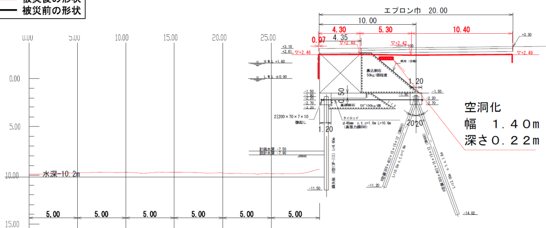
図-A. 12. 194 No.4 仙台港区_中野地区_岸壁 (-7.5m) の断面図 A-A' (被災後)
