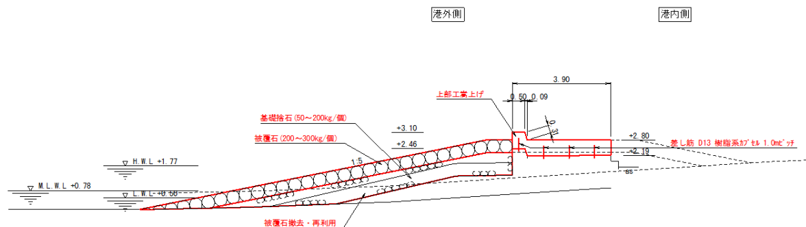
図-A. 12. 87 No. 7 塩釜港区_代ヶ崎清水東側防波堤の断面図 B No.8 (復旧後)
