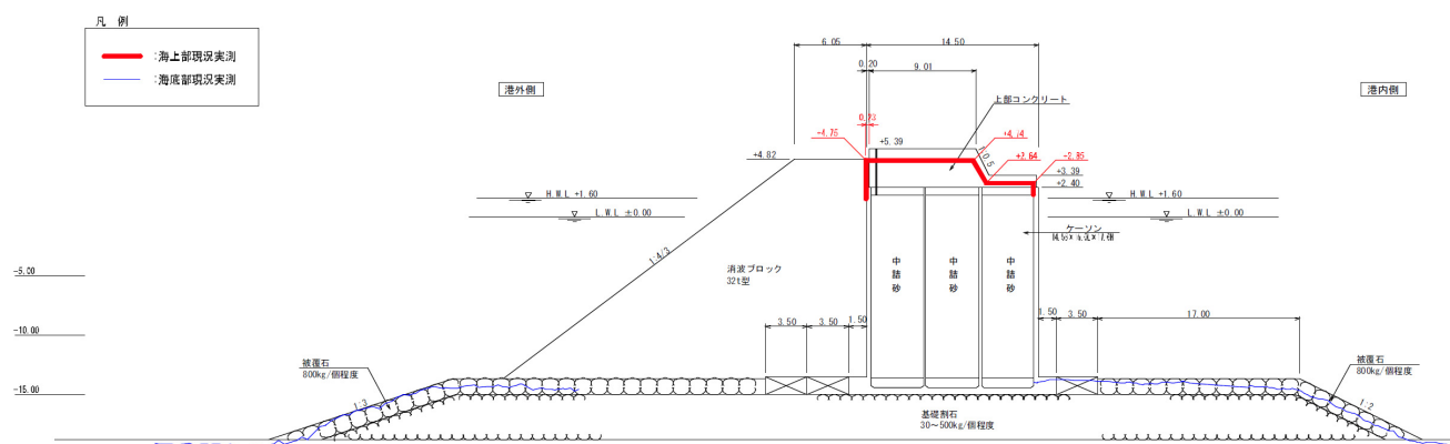
図-A.12.37 No.3 仙台港区_外港地区_沖防波堤の断面図 H-H' (被災後)
