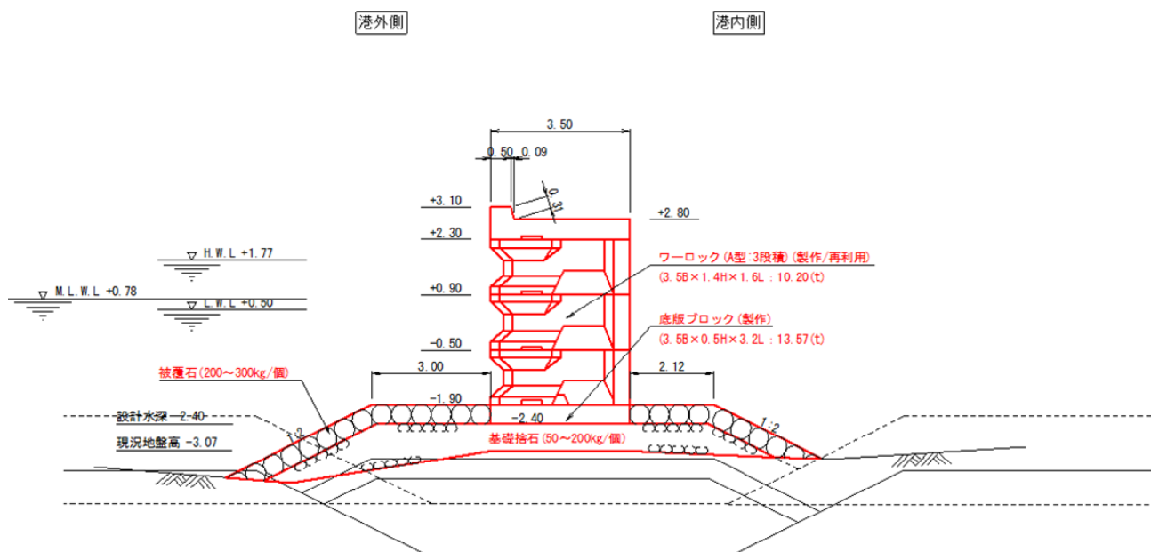
図-A.12.86 No.7 塩釜港区_代ヶ崎清水東側防波堤の断面図B No.0（復旧後）
