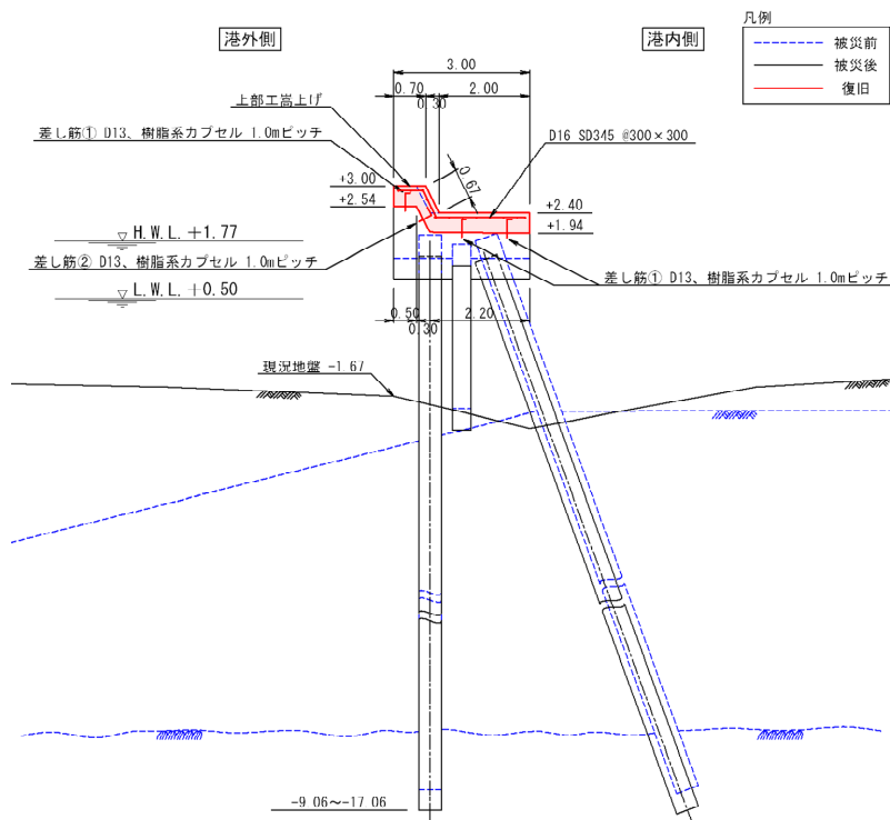
図-A.12.115 No. 15 塩釜港区_要害 (A) (B) 防波堤の断面図 (復旧後)
