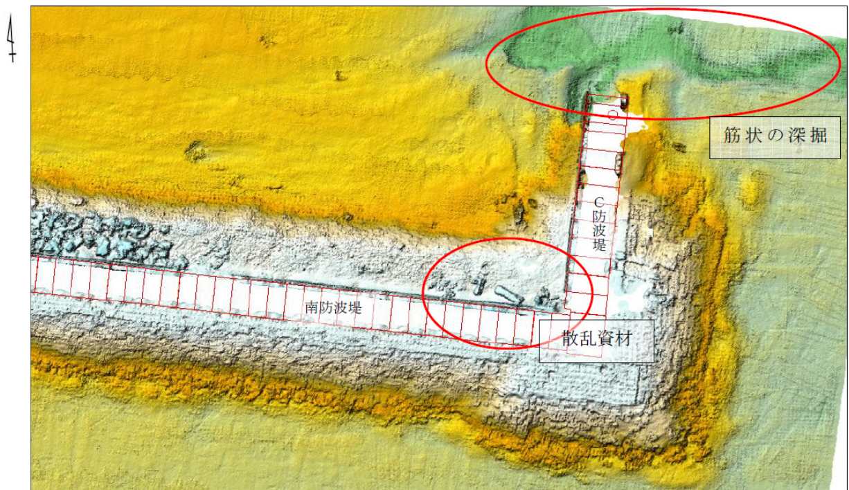
図-A.12.45 No.4 仙台港区_外港地区_C防波堤の平面図（被災後）
