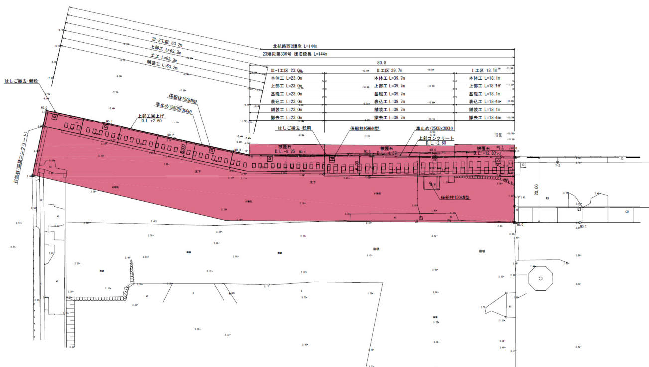
図－A.12.149 No. 21 仙台港区_北航路西 C 護岸の平面図（被災後）
