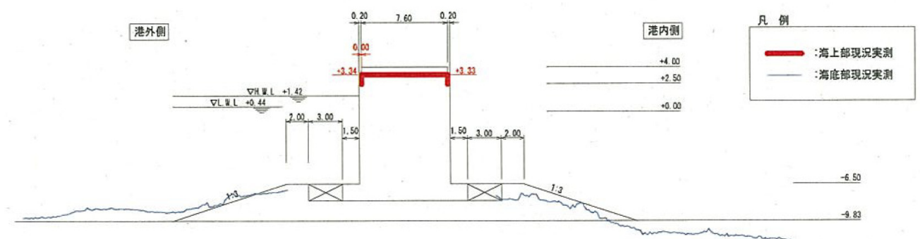
図-A.12.14 No.1 仙台港区_外港地区_北防波堤の断面図 C-C'（被災後）
