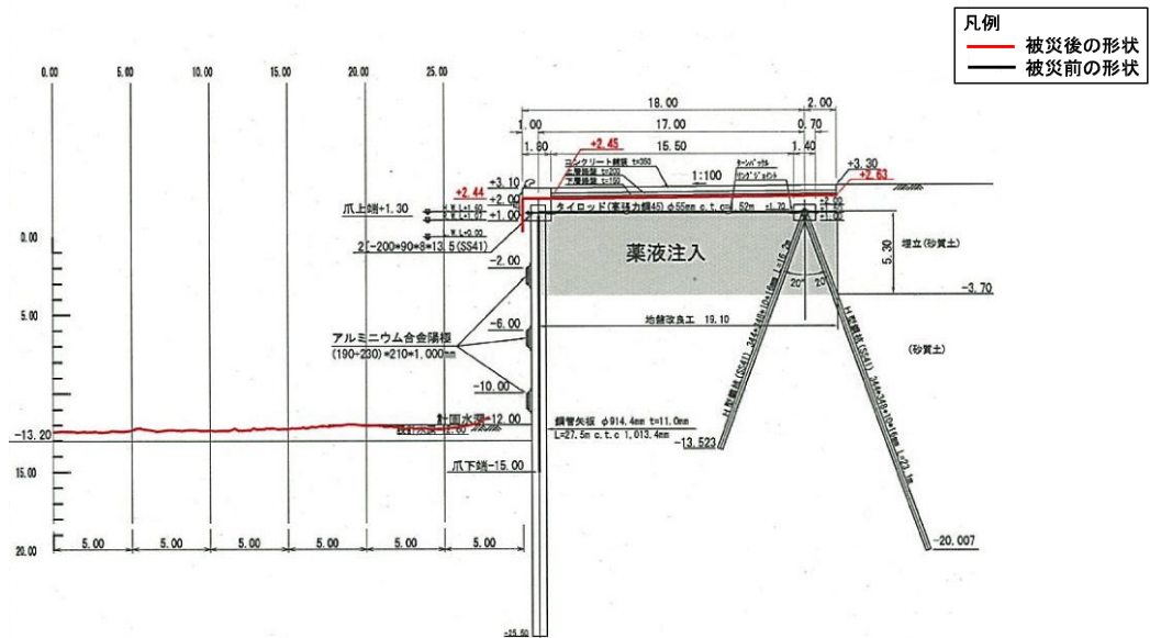
図-A. 12. 183 No.3 仙台港区_中野地区_高松木材埠頭岸壁 (-12m) の断面図 C-C' (被災後)
