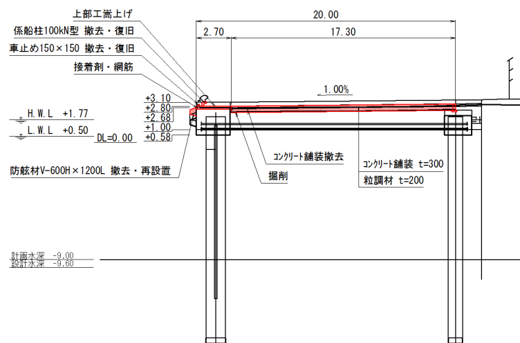
図-A. 12. 302 No. 21 塩釜港区_貞山ふ頭 2 号岸壁の断面図 (復旧後)
