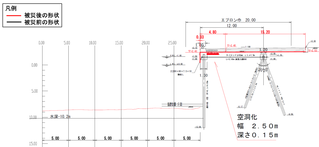
図-A.12.201 No.4 仙台港区_中野地区_岸壁 (-7.5m) の断面図 H-H' (被災後)
