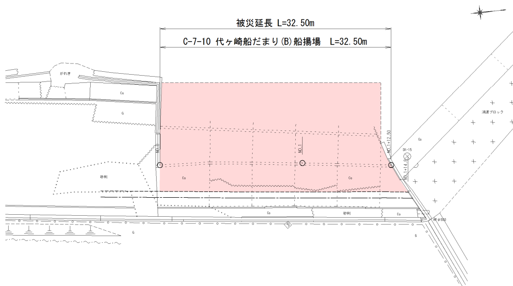
図-A.12.272 No.12 塩釜港区_代ヶ崎船たまり (B) 船揚場の平面図 (被災後)
