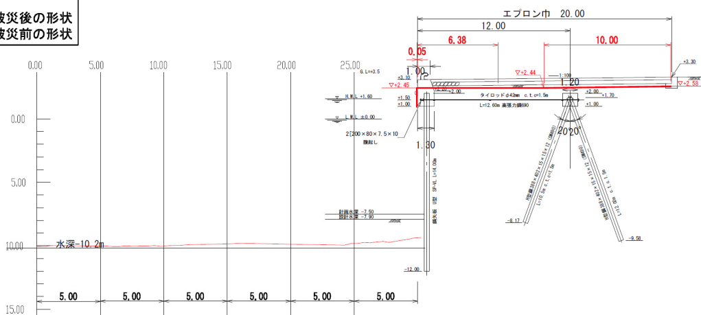
図-A.12.198 No.4 仙台港区_中野地区_岸壁 (-7.5m) の断面図 E-E' (被災後)
