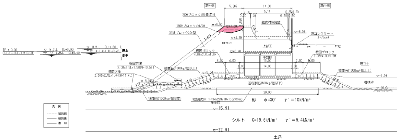
図-A. 12. 144 No. 19 仙台港区_南防波護岸の断面図 (被災後)
