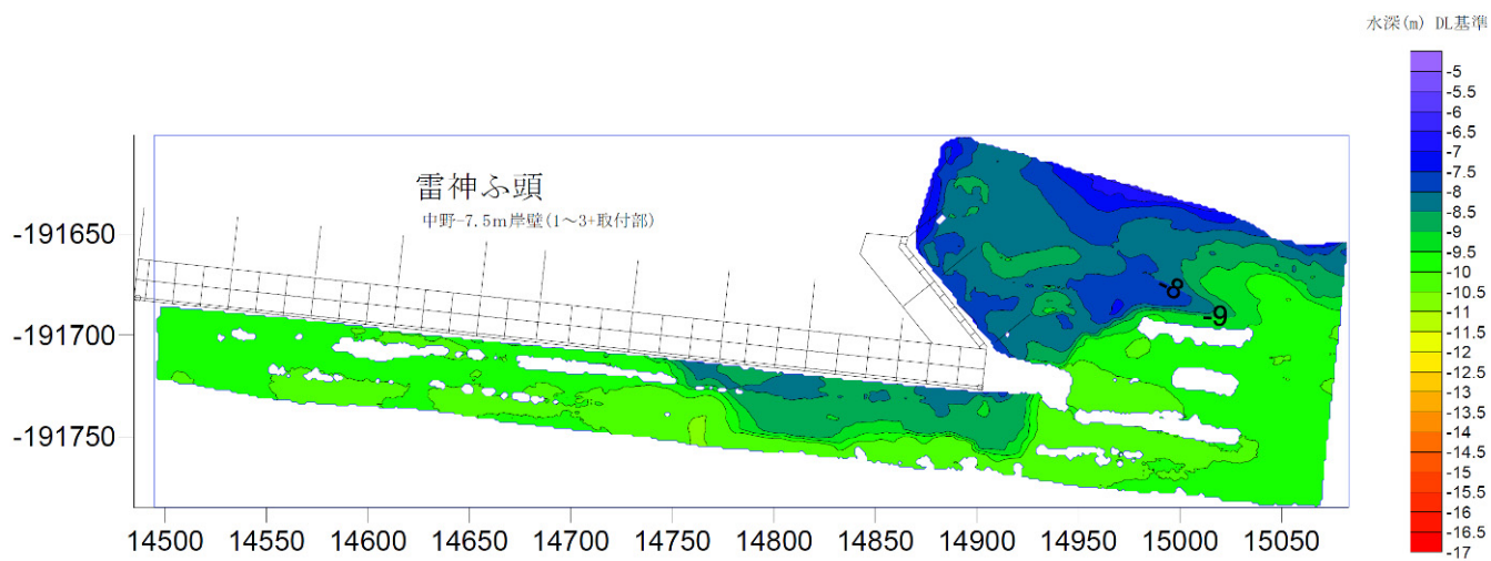
図-A. 12. 193 No.4 仙台港区_中野地区_岸壁 (-7.5m) のカラー段彩図 (被災後)
