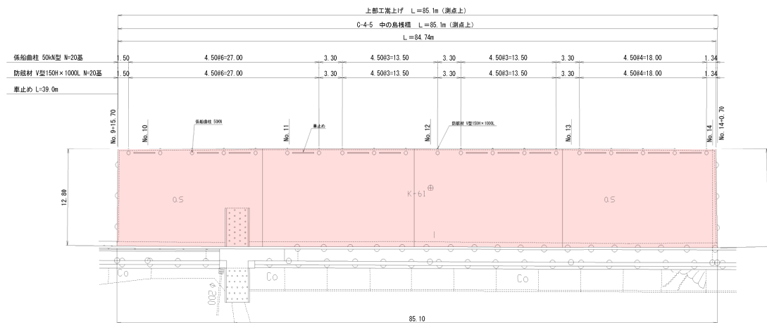
図-A.12.276 No.14 塩釜港区_中の島さん橋の平面図（被災後）
