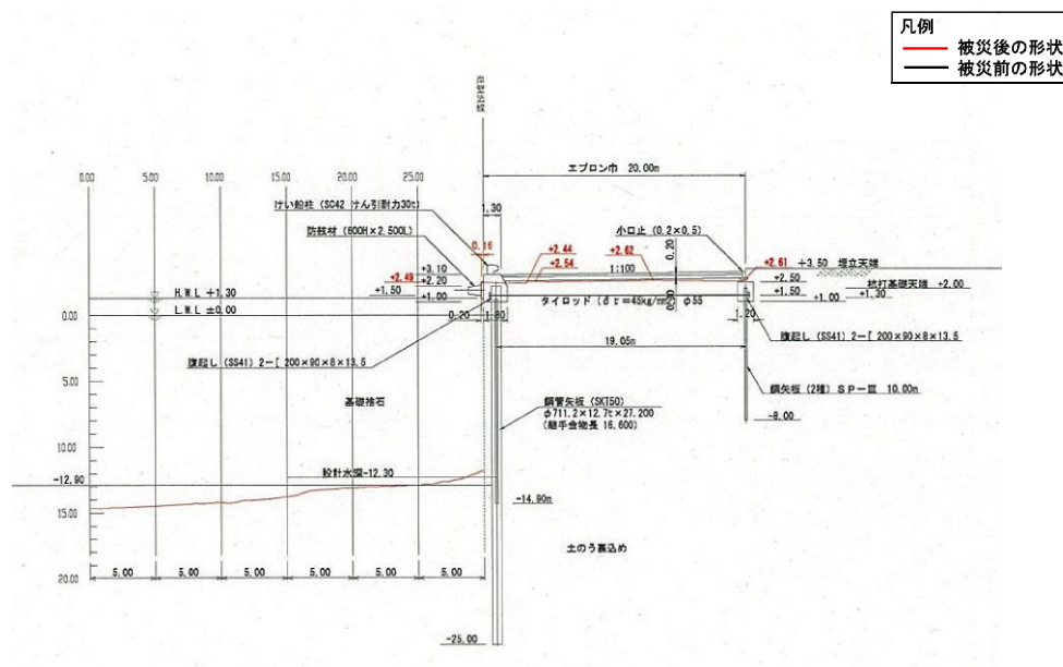
図-A.12.213 No.5 仙台港区_中野地区_岸壁 (-12m) の断面図 E-E' (被災後)
