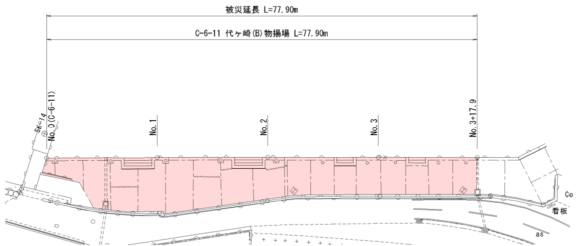
図-A. 12. 260 No. 6 塩釜港区_代ヶ崎 (B) 物揚場の平面図 (被災後)
