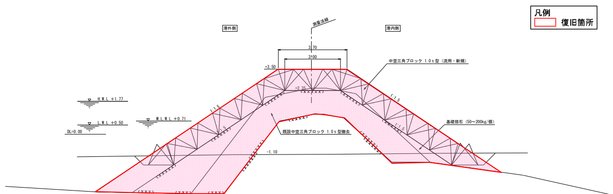
図-A. 12. 76 No. 4 塩釜港区_石浜南防波堤の A 断面図 (復旧後)
