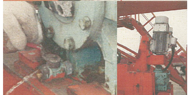
図一A. 12. 351 走行装置浸水被害（陸側：車輪軸受水没，減速機内海水混入，走行モータ，1号機）
