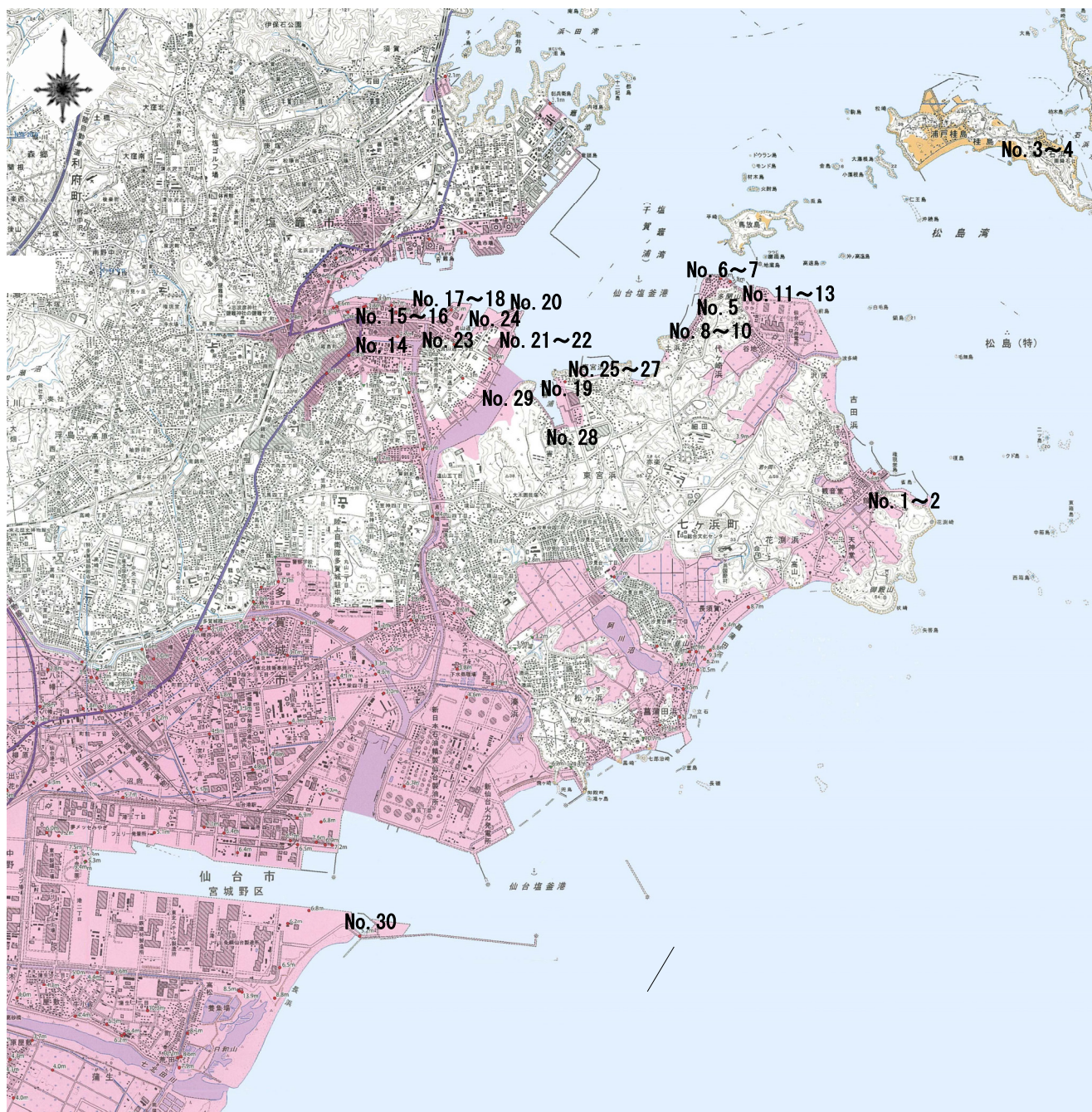
図一A. 12. 247 仙台塩釜港の被災港湾施設（係留施設，補助分）
