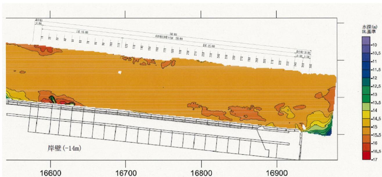
図-A.12.171 No.2 仙台港区_向洋地区_岸壁 (-14m) のカラー段彩図 (被災後)
