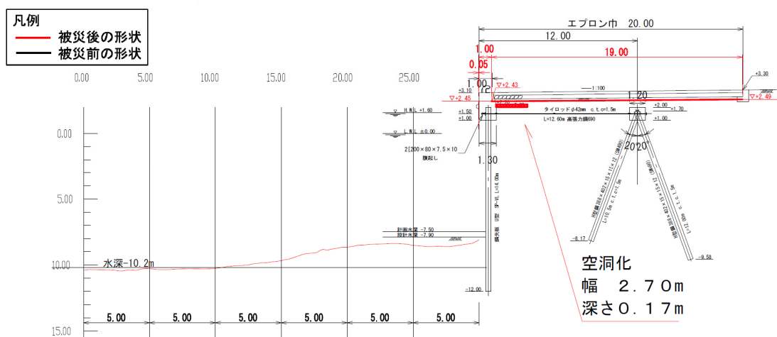
図-A.12.200 No.4 仙台港区_中野地区_岸壁 (-7.5m) の断面図 G-G' (被災後)
