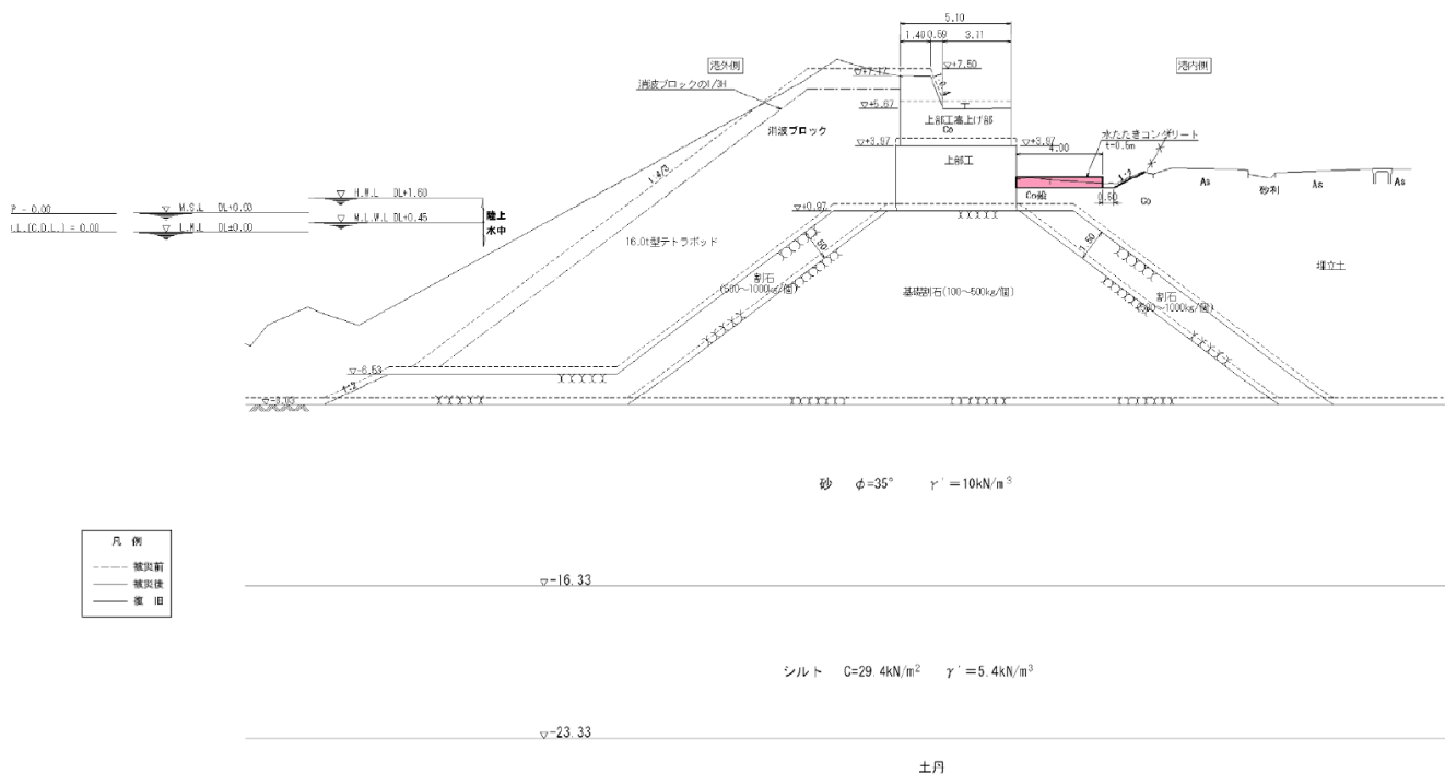
図-A. 12. 143 No. 19 仙台港区_南防波護岸の断面図 (被災後)
