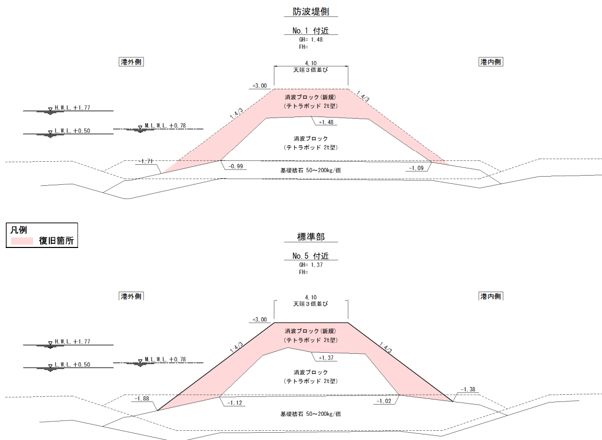
図-A. 12. 334 No. 1 塩釜港区_代ヶ崎離岸堤の断面図（復旧後）
