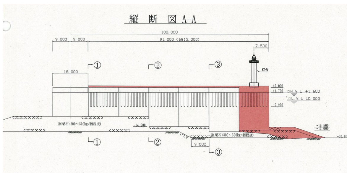
図-A. 12. 53 No. 4 仙台港区_外港地区_C 防波堤の縦断図 A-A'（復旧後）
