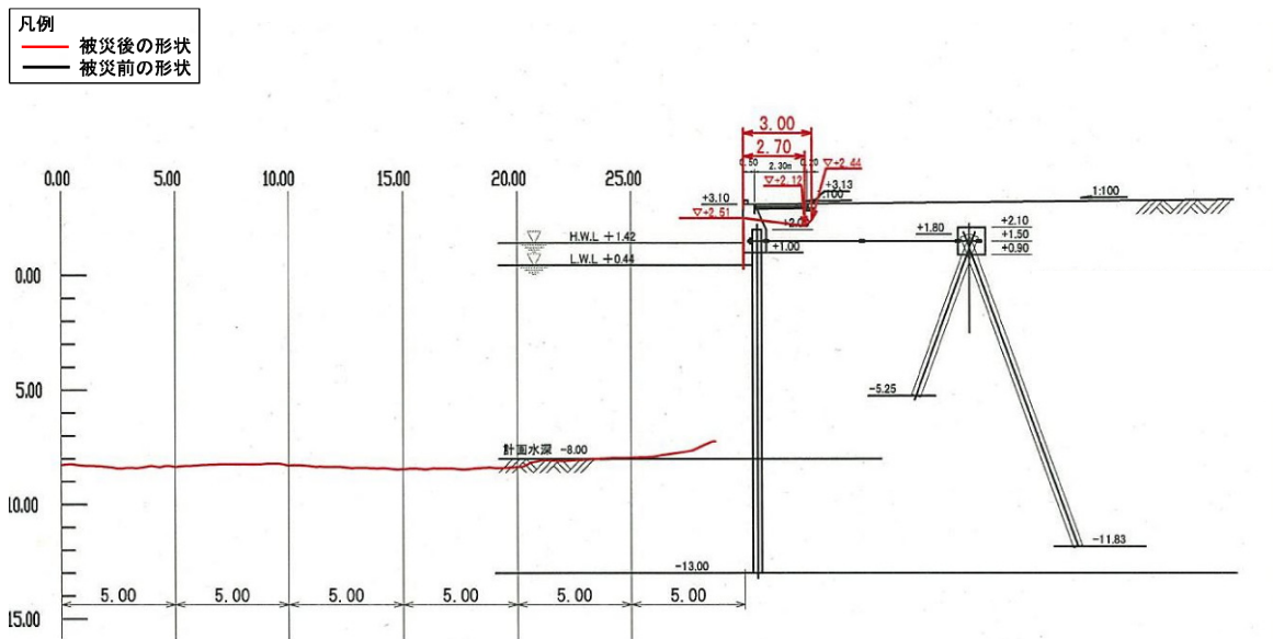
図-A. 12. 59 No. 5 仙台港区_中野地区_護岸Ⅱの断面図 A-A' (被災後)
