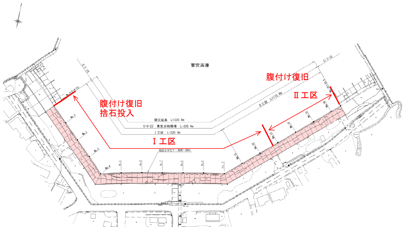
図-A.12.318 No.27 塩釜港区_東宮浜物揚場の平面図 (被災後)
