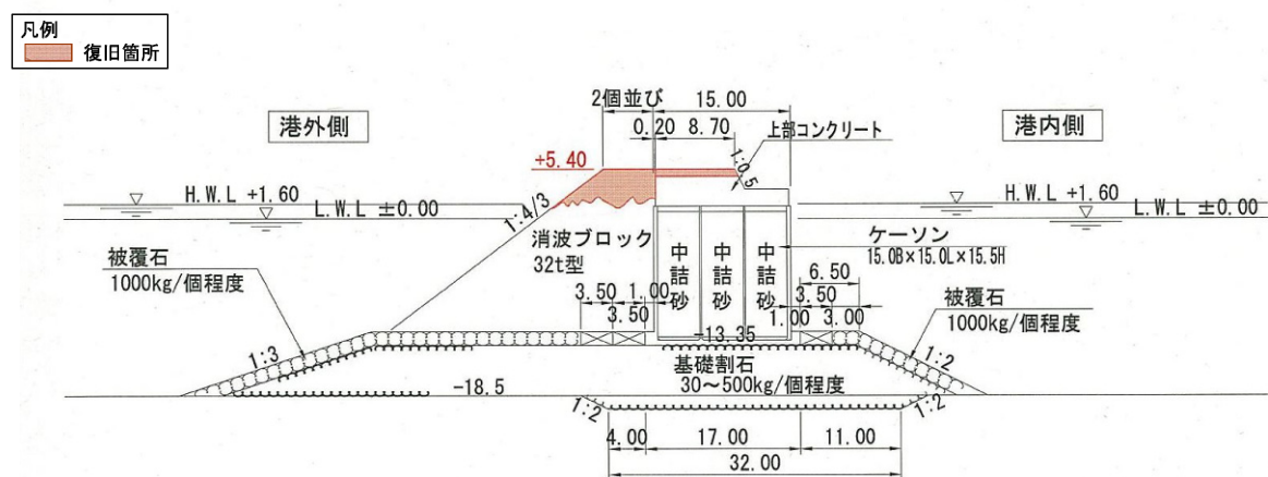
図-A.12.40 No.3 仙台港区_外港地区_沖防波堤の断面図（標準部）（復旧後）
