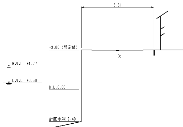
図-A. 12. 307 No. 23 塩釜港区_東ふ頭・中ふ頭間物揚場の断面図（被災前）
