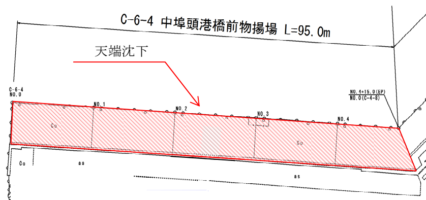
図-A.12.279 No. 15 塩釜港区_中ふ頭港橋前物揚場の平面図（被災後）
