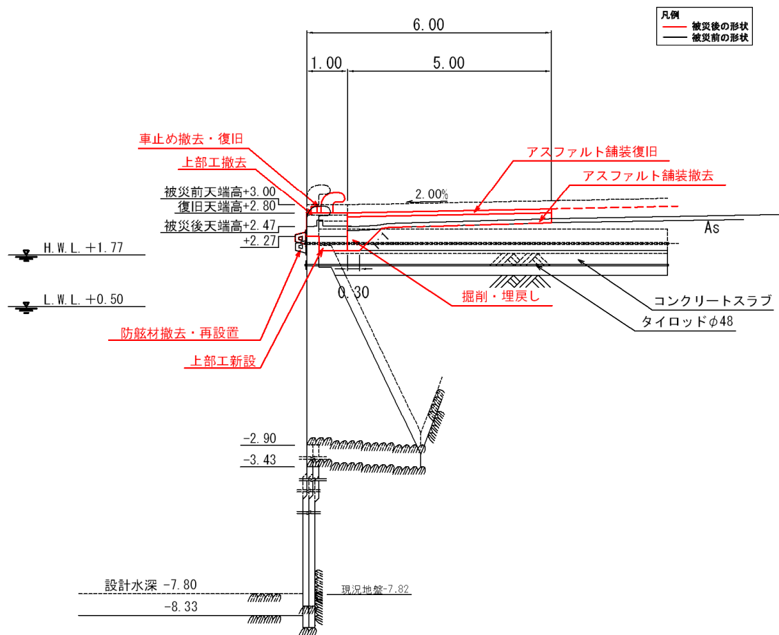
図-A. 12. 313 No. 24 塩釜港区_東ふ頭岸壁の断面図（復旧後）
