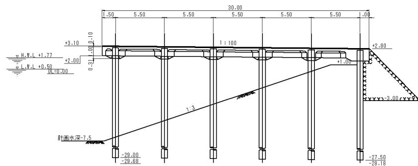
図-A. 12. 303 No. 22 塩釜港区_貞山ふ頭 3 号・4 号さん橋の断面図 (被災前)
