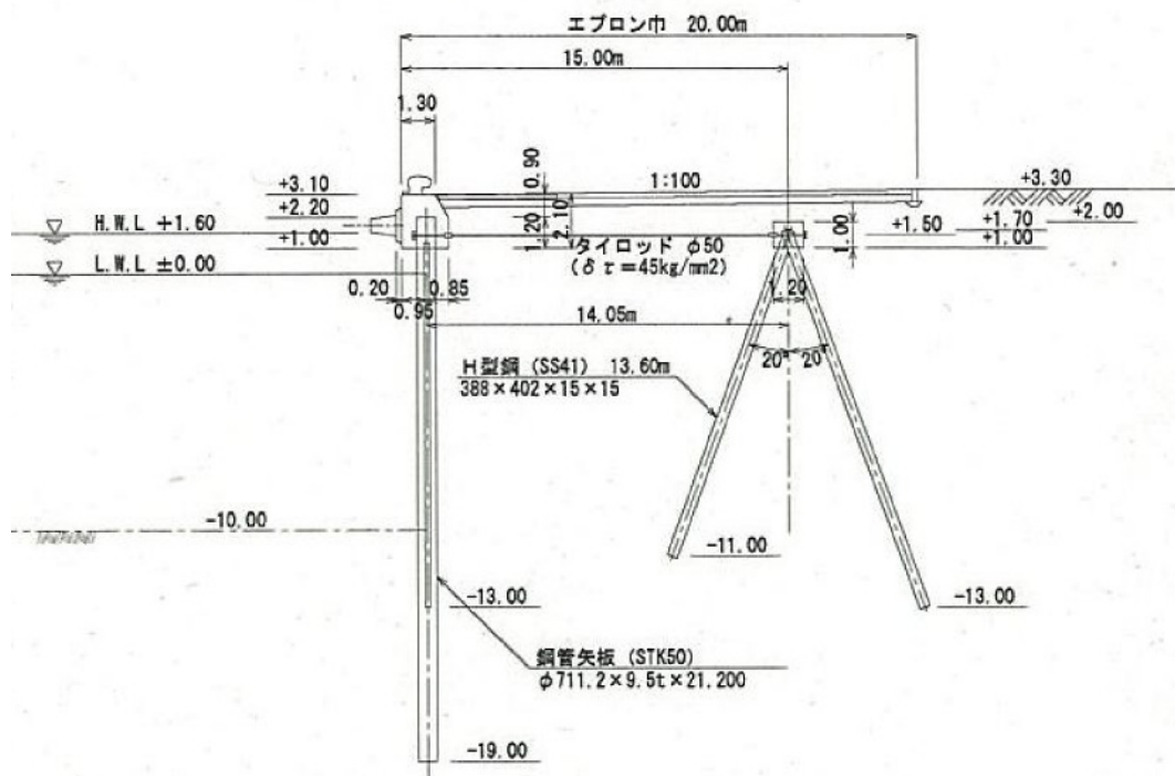
図-A. 12. 221 No.6 仙台港区_中野地区_6号岸壁 (-10m) の断面図 (被災前)
