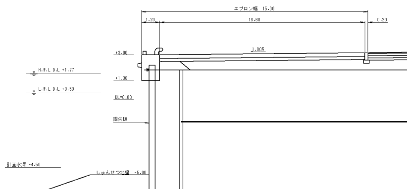
図-A.12.290 No. 18 塩釜港区_中ふ頭東側岸壁の断面図（被災前）
