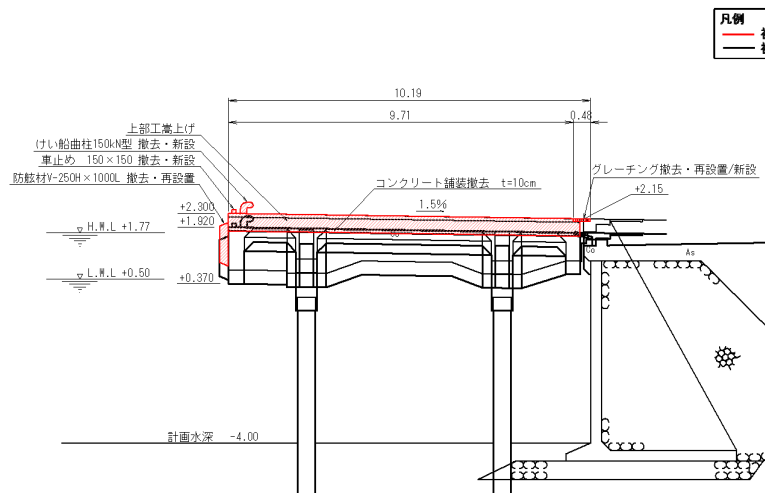
図一A. 12. 281 No. 15 塩釜港区_中ふ頭港橋前物揚場の断面図（復旧後）
