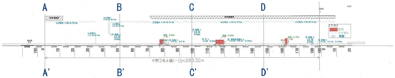
図-A.12.225 No.6 仙台港区_中野地区_3号岸壁 (-10m) の平面図 (被災後)
