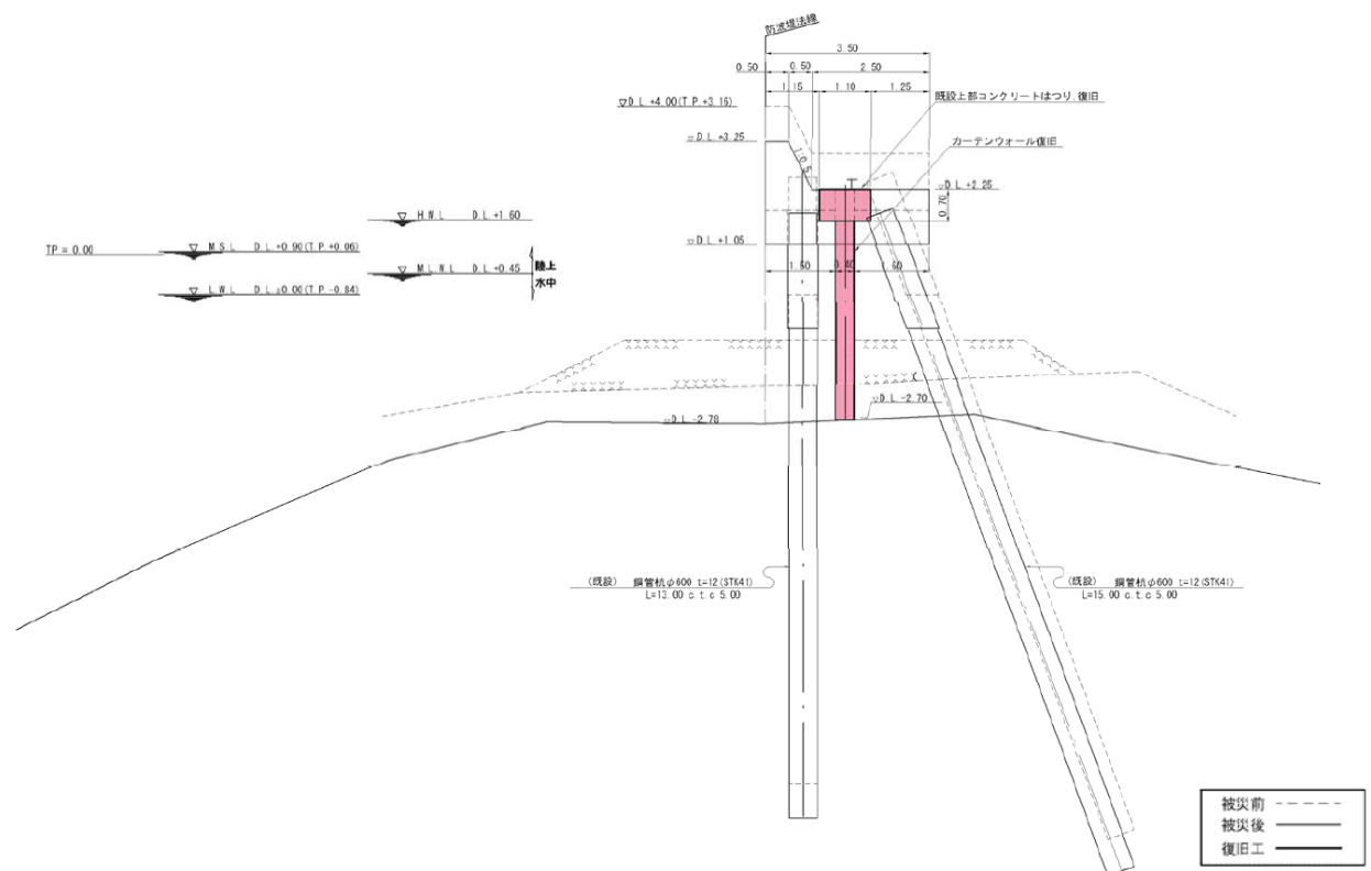
図-A. 12. 132 No. 17 仙台港区_高砂防波堤の断面図⑥ (被災後)
