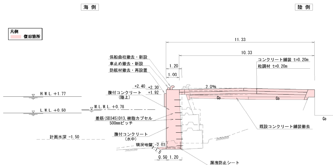
図-A.12.263 No.7 塩釜港区_代ヶ崎 (C) 物揚場の断面図 (復旧後)
