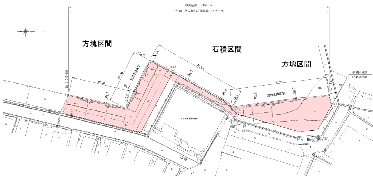
図-A.12.257 No.5 塩釜港区_代ヶ崎 (A) 物揚場の平面図 (被災後)
