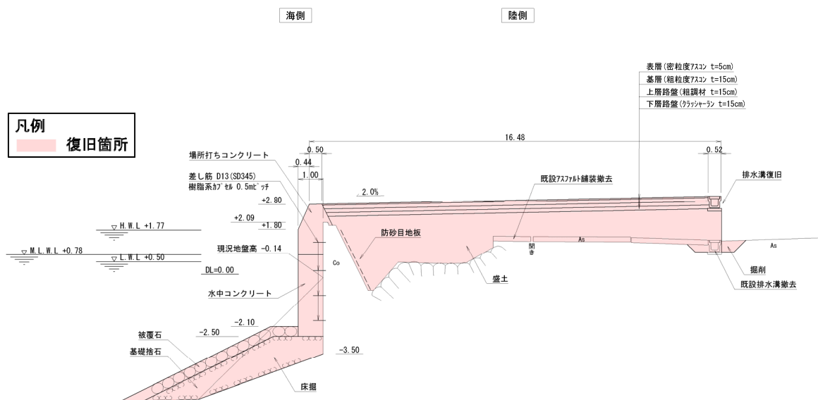
図一A.12.98 No.10 塩釜港区_東ふ頭護岸・貞山ふ頭西護岸の断面図 CN0.0 (復旧後)
