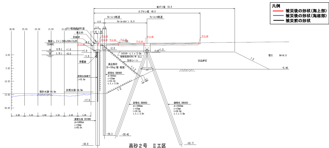
図-A. 12. 172 No.2 仙台港区_向洋地区_岸壁 (-14m) の断面図 A-A' (被災後)
