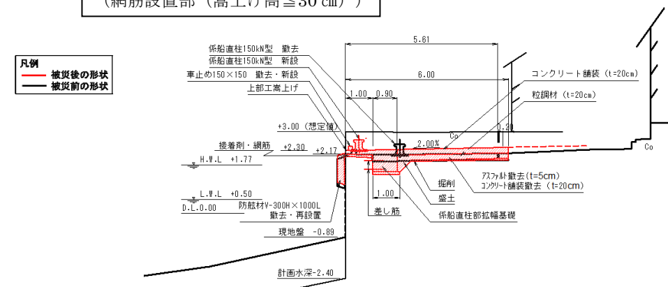
図-A. 12. 311 No. 23 塩釜港区_東ふ頭・中ふ頭間物揚場の断面図 (復旧後)
