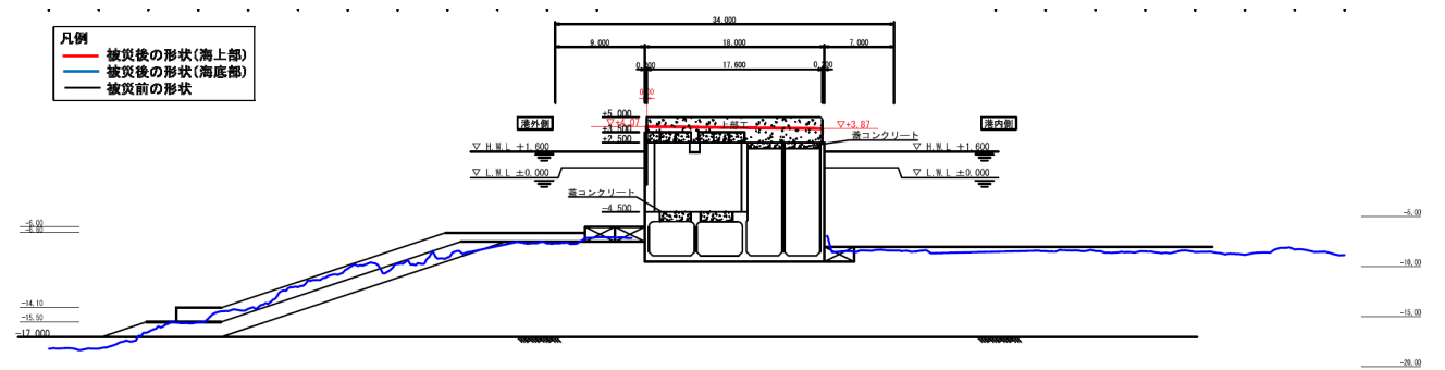
図-A.12.49 No.4 仙台港区_外港地区_C防波堤の断面図 B-B' (被災後)
