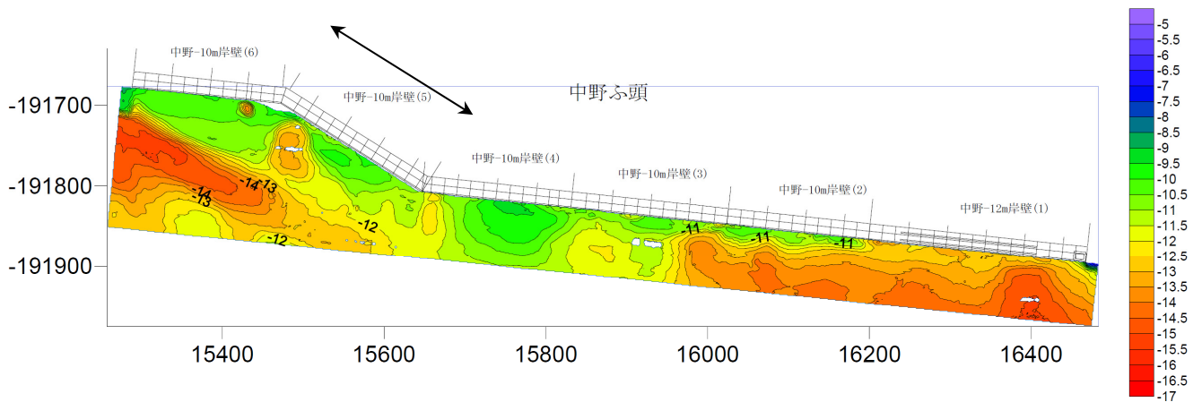
図-A.12.232 No.6 仙台港区_中野地区_5号岸壁 (-10m) のカラー段彩図 (被災後)
