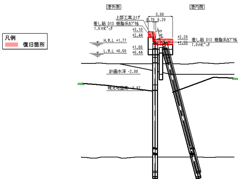
図-A.12.109 No.13 塩釜港区_東宮浜西防波堤の断面図（復旧後）
