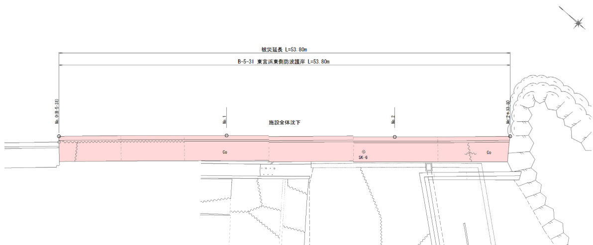
図-A.12.110 No. 14 塩釜港区_東宮浜東側防波護岸の平面図（被災後）
