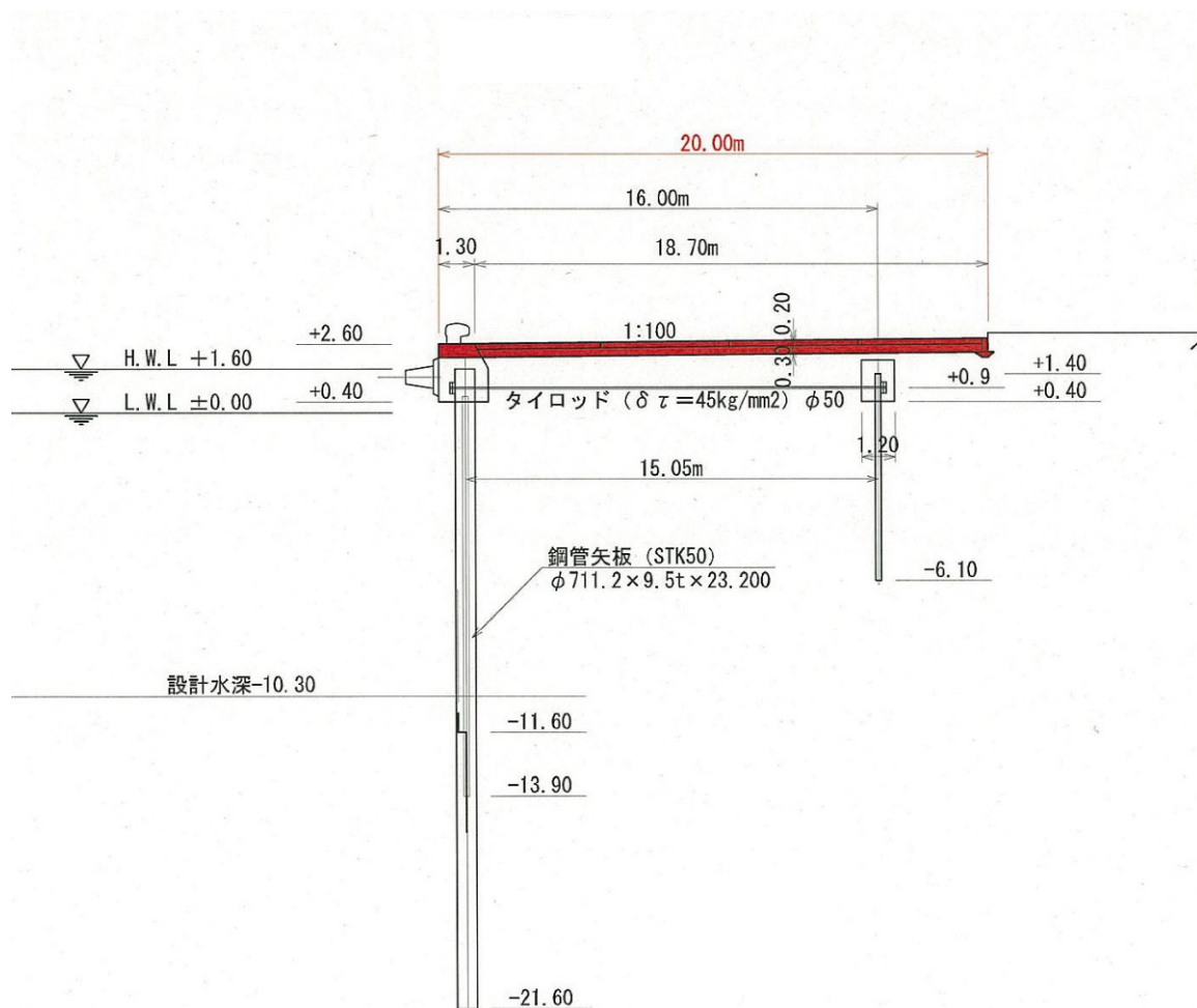
図-A. 12. 238 No.6 仙台港区_中野地区_2号岸壁 (-10m) の断面図 (復旧後)
