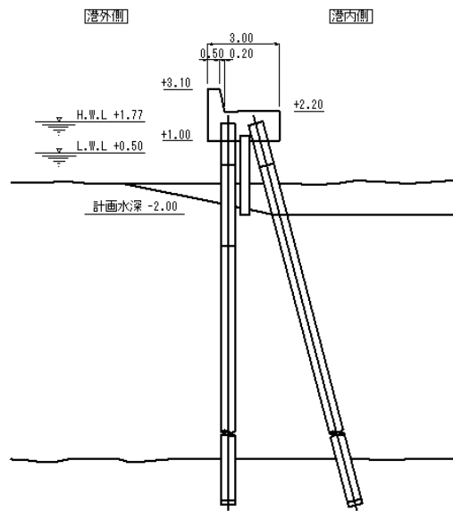
図-A. 12. 102 No. 12 塩釜港区_東宮浜東防波堤の断面図（被災前）
