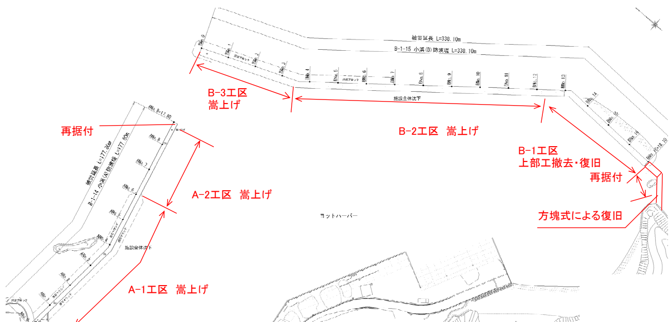
図-A.12.69 No.2 塩釜港区_小浜防波堤 (A)の平面図（復旧後）
