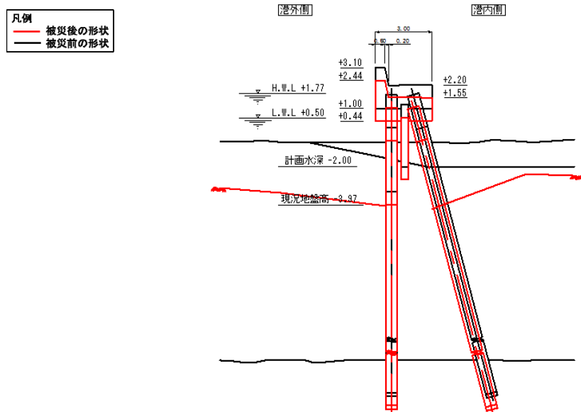
図-A.12.108 No.13 塩釜港区_東宮浜西防波堤の断面図（被災後）
