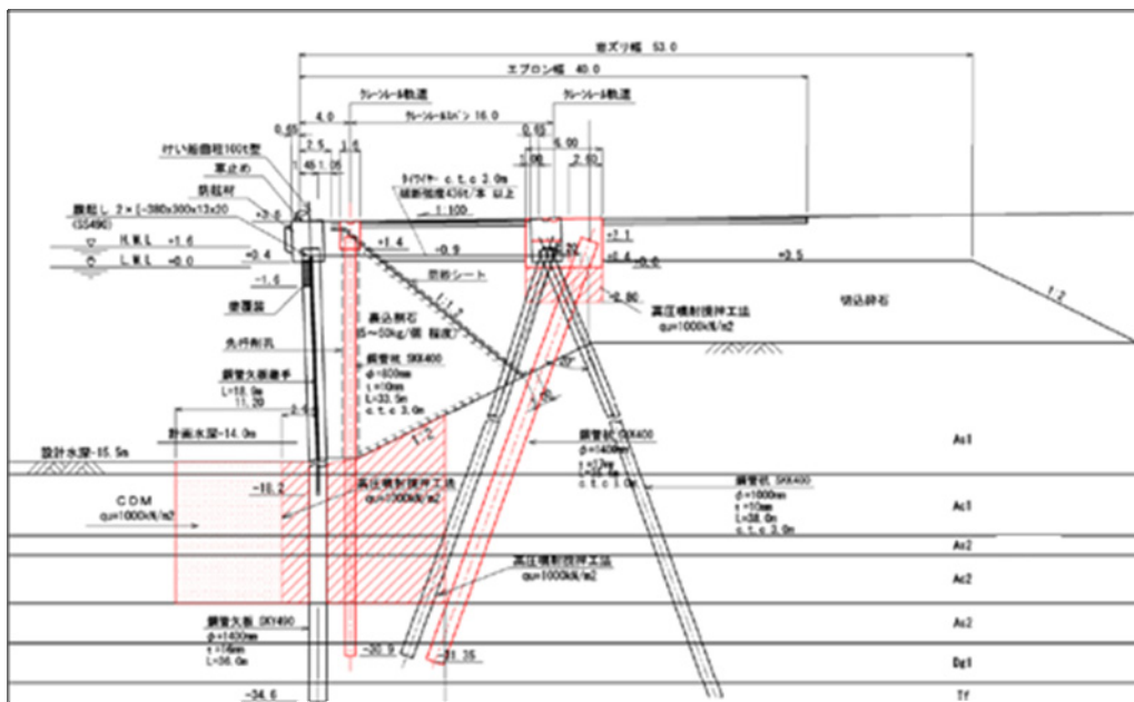
図-A.12.177 No.2 仙台港区_向洋地区_岸壁 (-14m) の断面図 (Ⅱ区) (復旧後)
