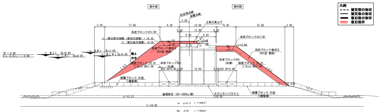
図一A.12.118 No.16 仙台港区_新北防波堤の断面図 No.0 地点 (被災前・後_復旧後)
