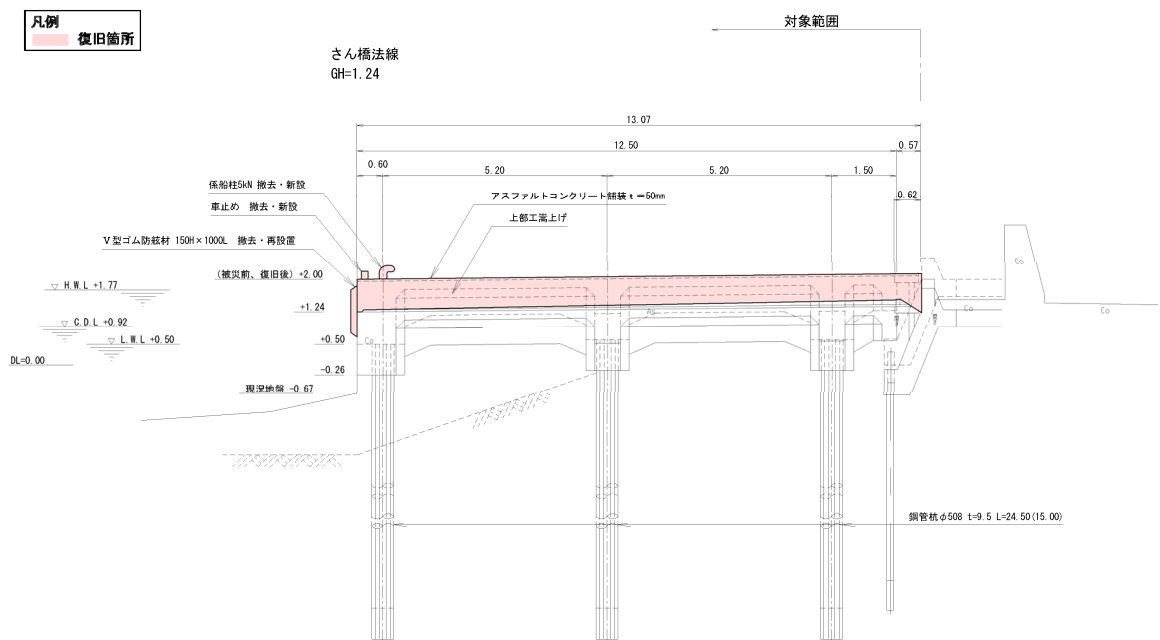
図-A.12.277 No.14 塩釜港区_中の島さん橋の断面図（復旧後）
