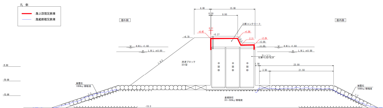
図-A.12.30 No.3 仙台港区_外港地区_沖防波堤の断面図 B-B' (被災後)
