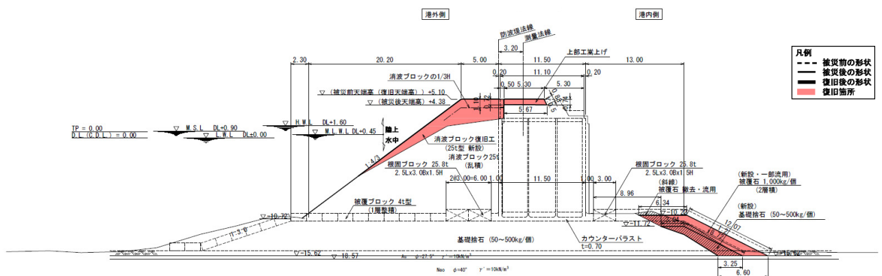
図一A.12.120 No.16 仙台港区_新北防波堤の断面図 No.7 地点 (被災前・後_復旧後)
