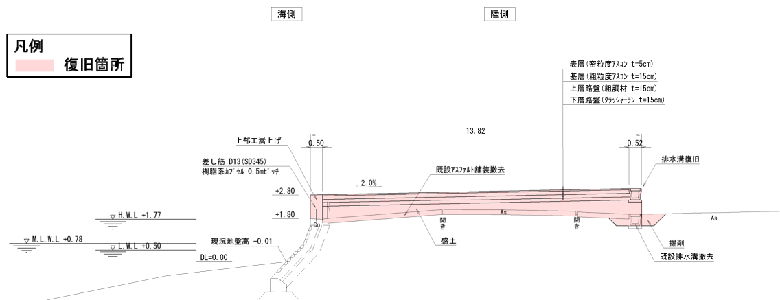
図一A.12.96 No.10 塩釜港区_東ふ頭護岸・貞山ふ頭西護岸の断面図 BN0.3 (復旧後)
