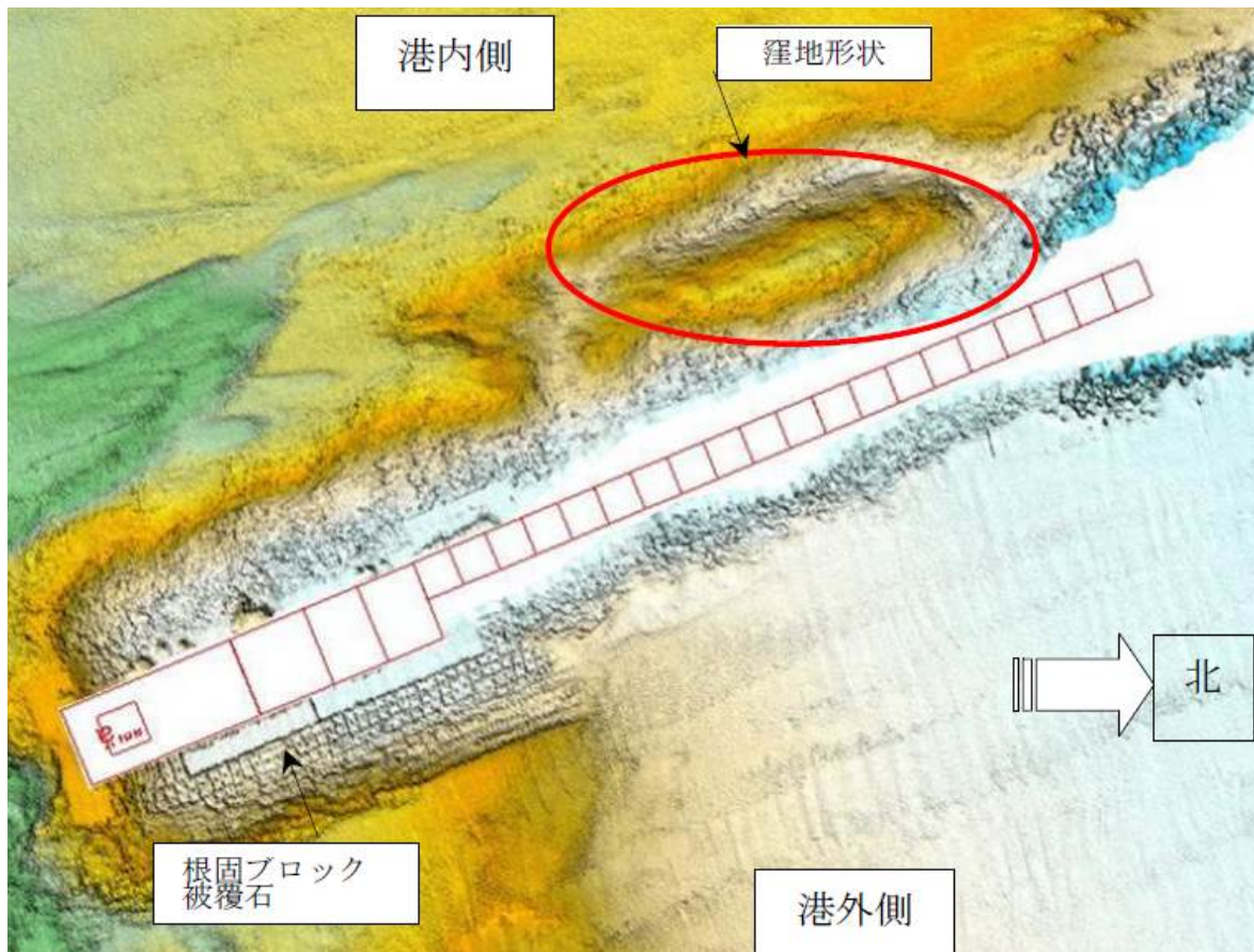
図-A. 12. 10 No. 1 仙台港区_外港地区_北防波堤の平面図（被災後）
