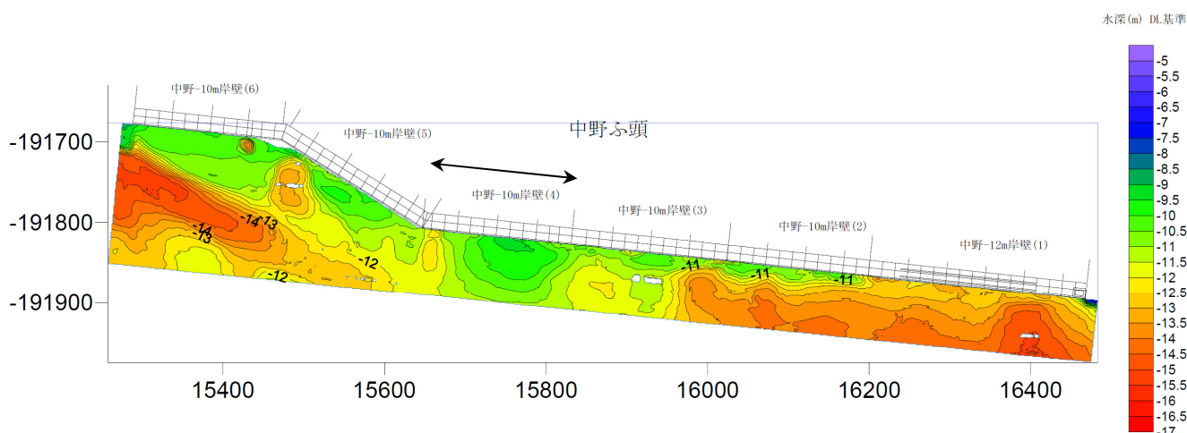
図-A.12.229 No.6 仙台港区_中野地区_4号岸壁 (-10m) のカラー段彩図 (被災後)
