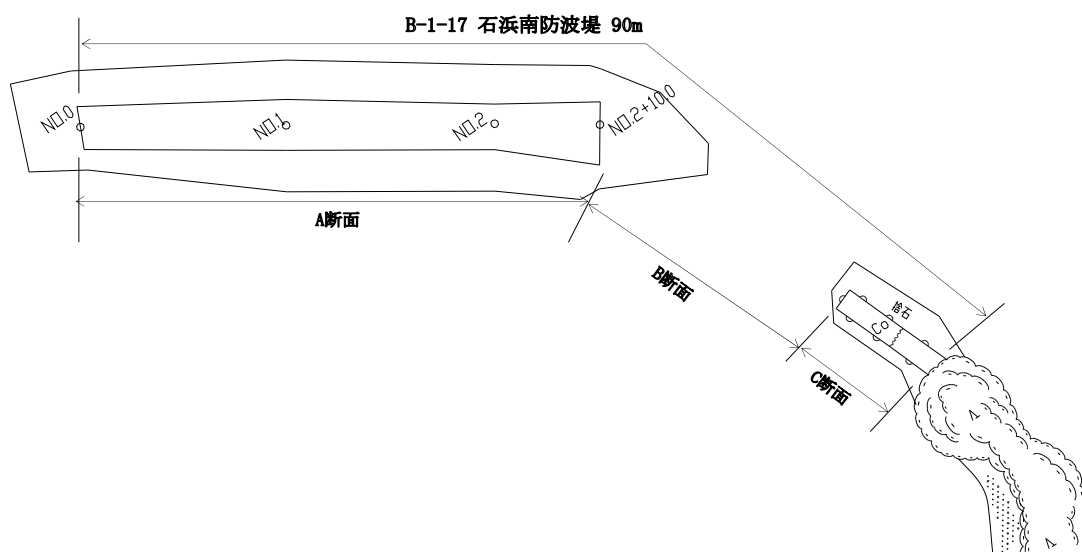
図-A. 12. 75 No. 4 塩釜港区_石浜南防波堤の平面図 (被災後)
