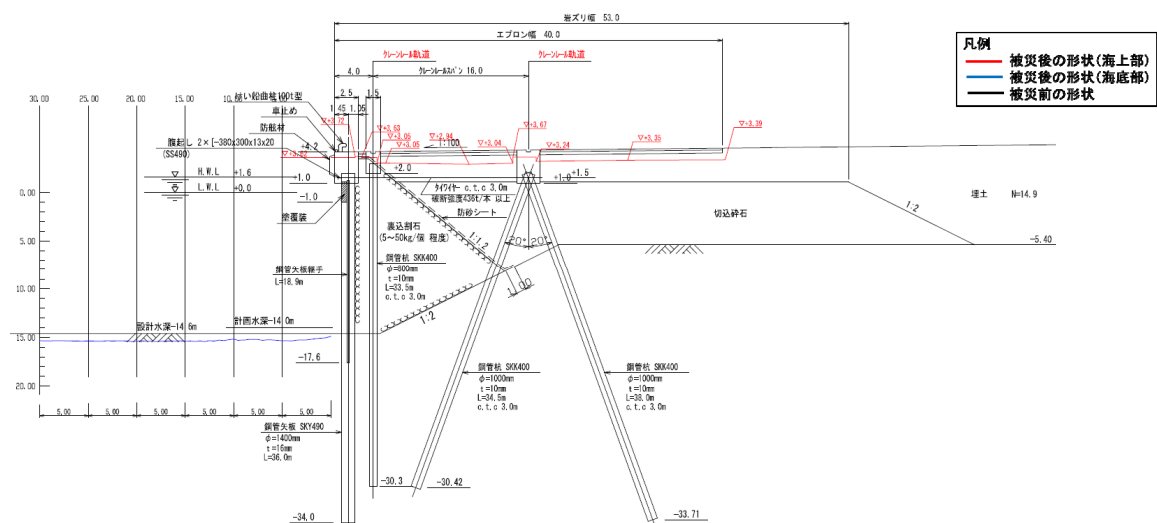
図-A. 12. 174 No.2 仙台港区_向洋地区_岸壁 (-14m) の断面図 C-C' (被災後)
