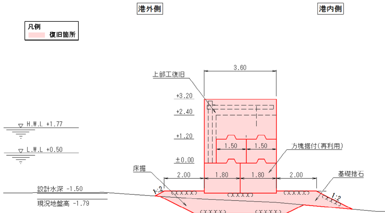
図-A. 12. 90 No. 8 塩釜港区_代ヶ崎東防波堤の断面図 A-2 区間 (復旧後)
