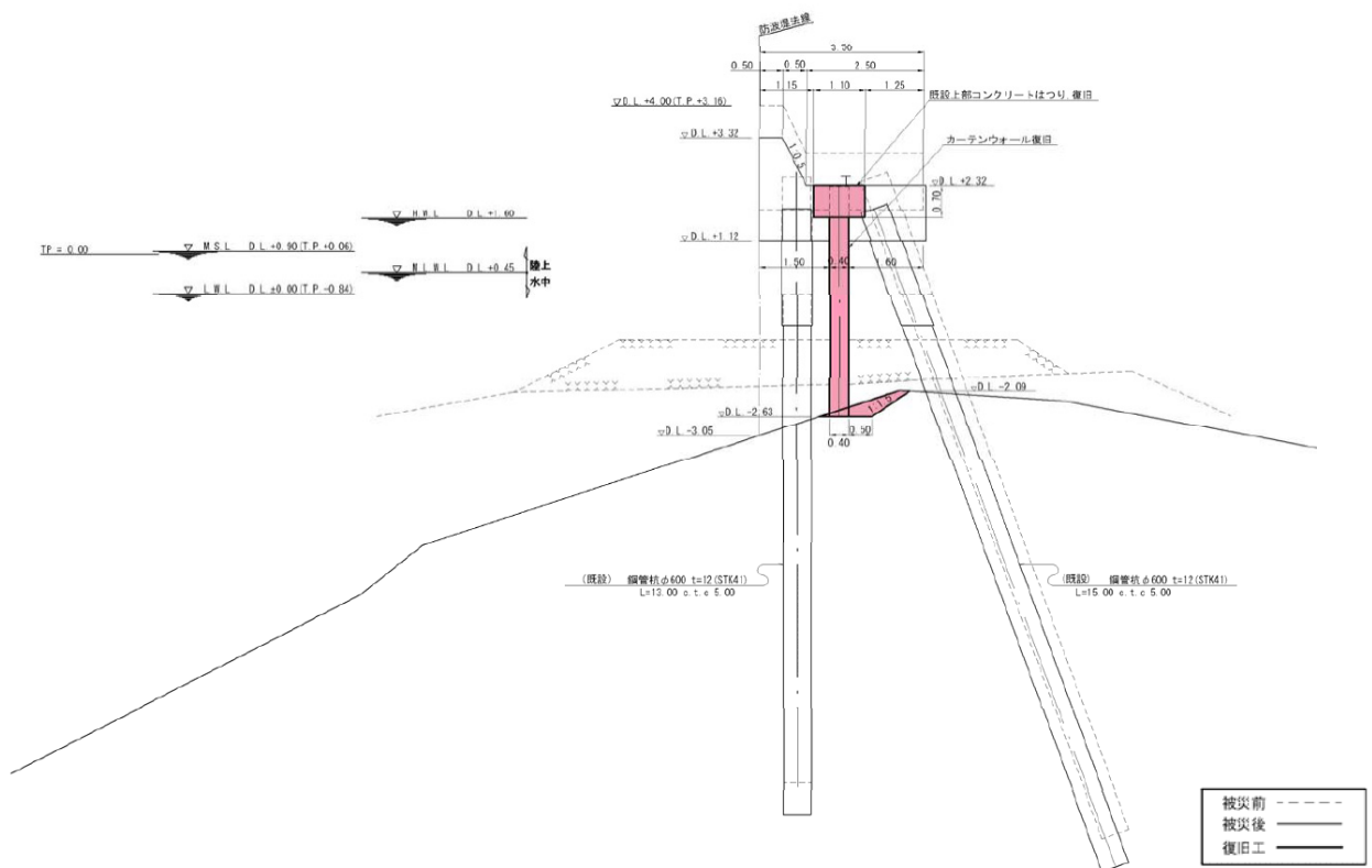
図-A. 12. 131 No. 17 仙台港区_高砂防波堤の断面図⑤ (被災後)
