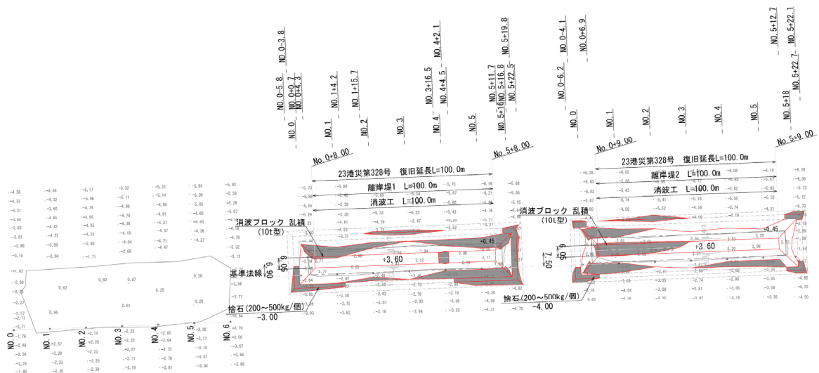
図-A.12.336 No.2 仙台港区_湊浜離岸堤の平面図 (被災後)
