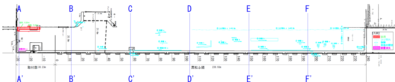
図-A.12.179 No.3 仙台港区_中野地区_高松木材埠頭岸壁（-12m）の平面図（被災後）
