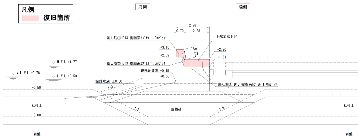
図－A.12.100 No.11 塩釜港区_東宮浜西側防波護岸の断面図No.1（復旧後）
