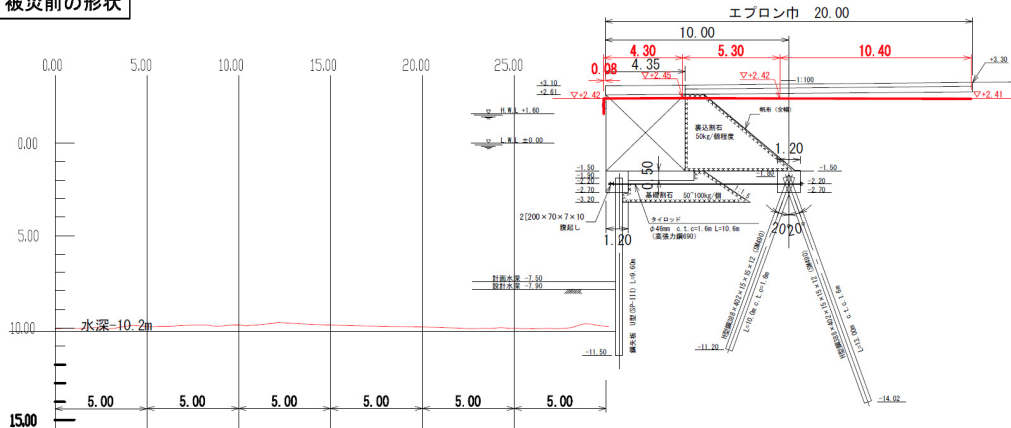
図-A. 12. 196 No.4 仙台港区_中野地区_岸壁 (-7.5m) の断面図 C-C' (被災後)
