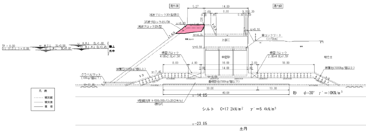
図-A. 12. 145 No. 19 仙台港区_南防波護岸の断面図 (被災後)
