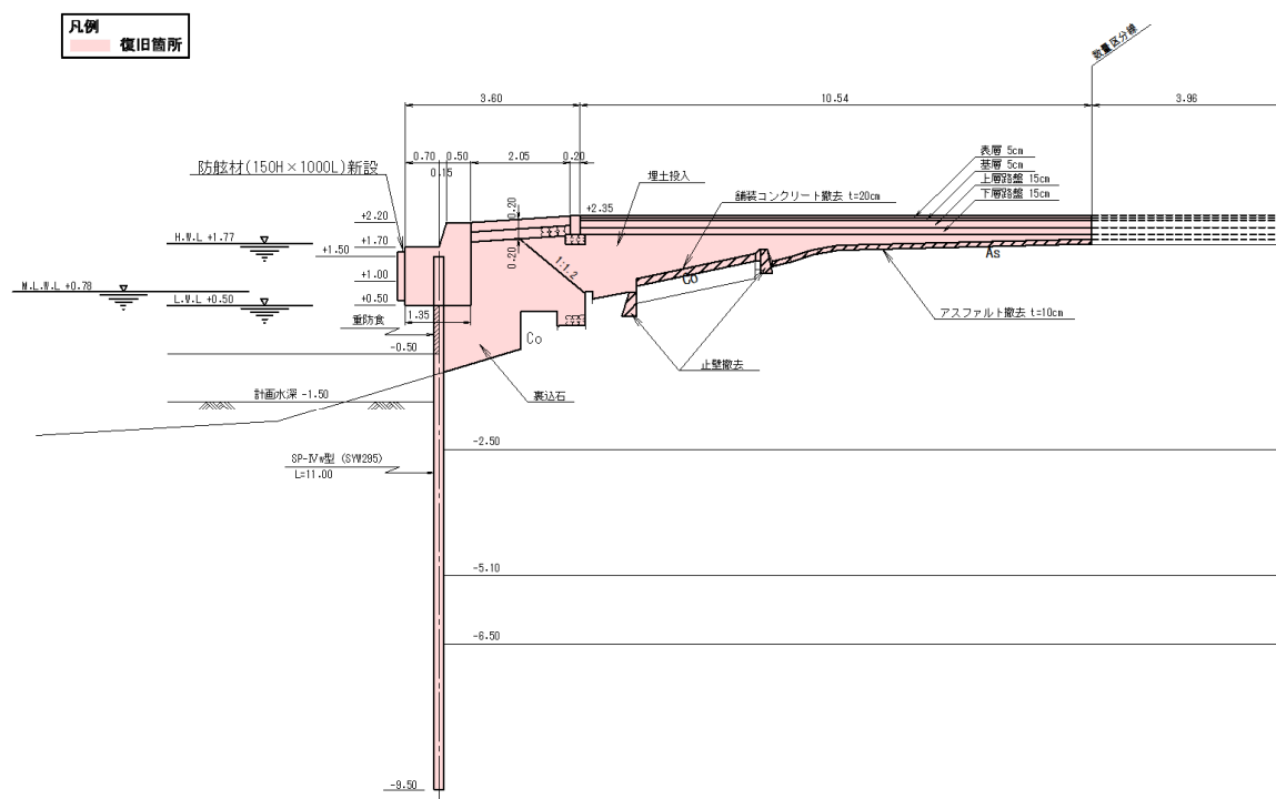
図-A.12.275 No.13 塩釜港区_代ヶ崎船たまり物揚場の断面図（復旧後）
