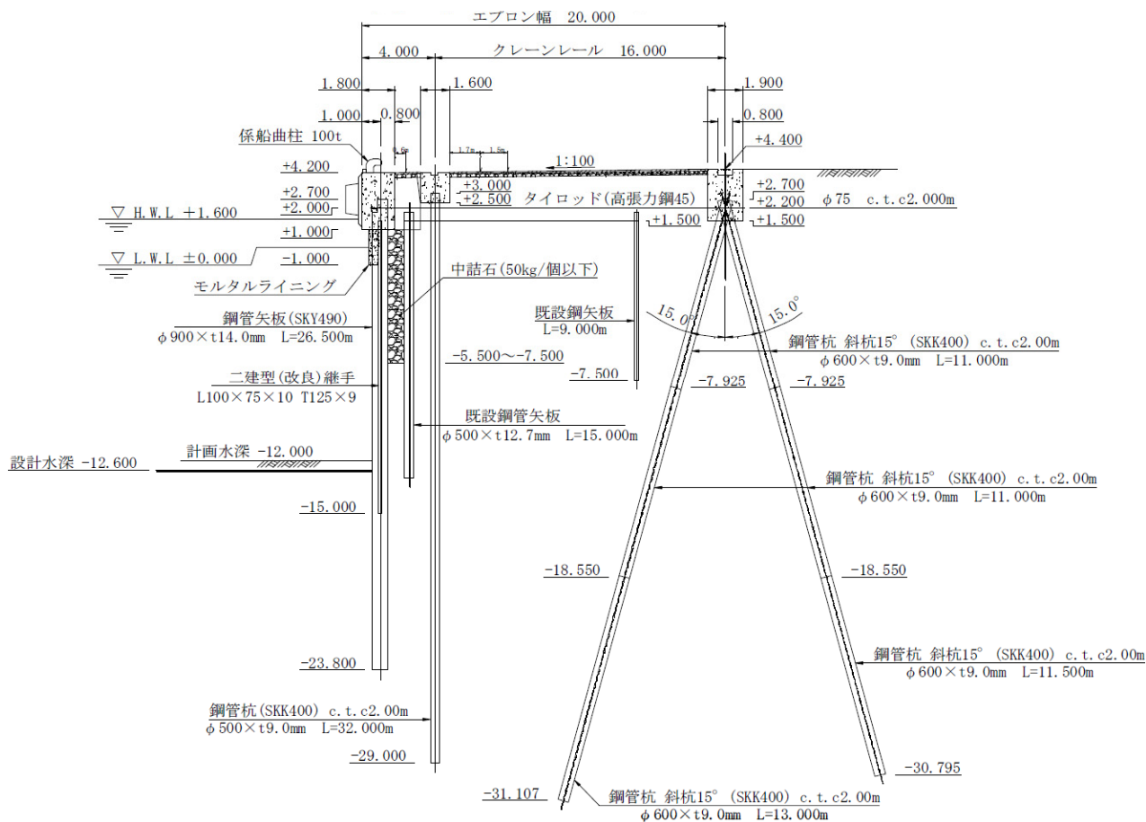
図-A.12.160 No.1 仙台港区_向洋地区_岸壁 (-12m) の断面図 (標準) (被災前)
