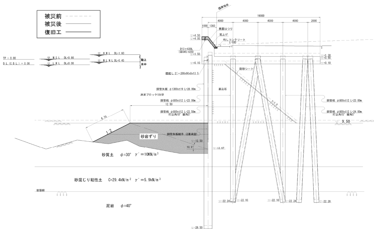
図-A. 12. 135 No. 18 仙台港区_向洋ふ頭防波護岸の断面図 (復旧後)
