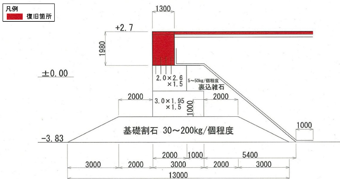
図-A.12.188 No.3 仙台港区_中野地区_高松木材埠頭岸壁 (-12m) の断面図 A-A' (復旧後)
