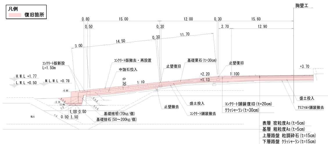
図-A.12.317 No. 26 塩釜港区_東宮浜東側船揚場の断面図（復旧後）
