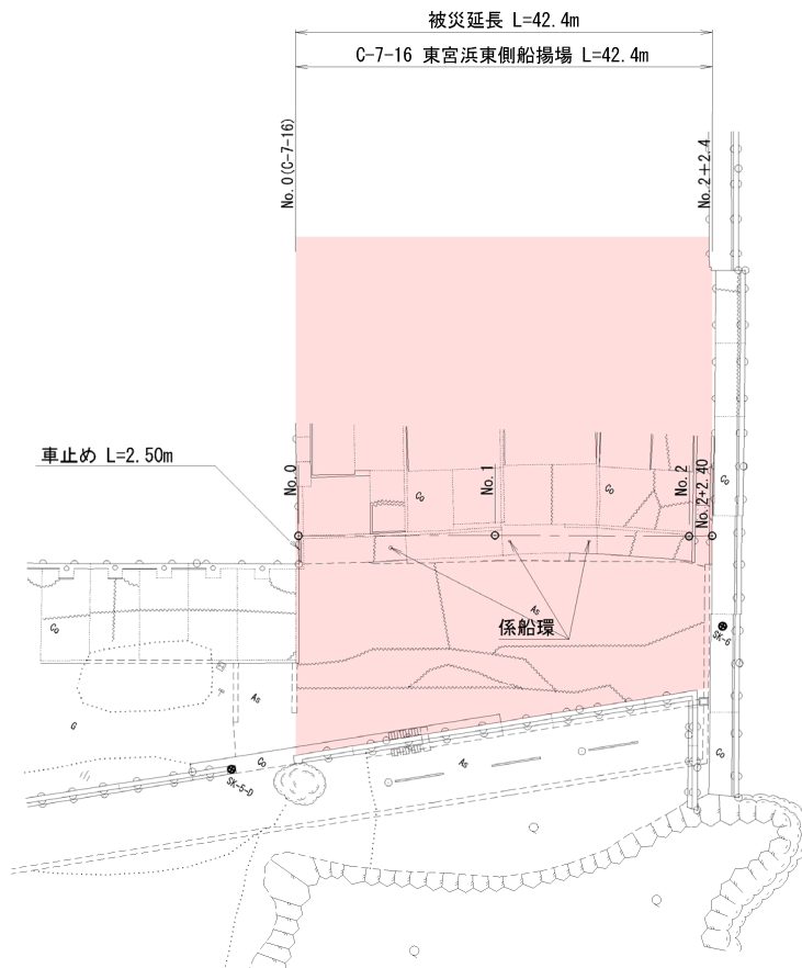
図-A.12.316 No. 26 塩釜港区_東宮浜東側船揚場の平面図（被災後）
