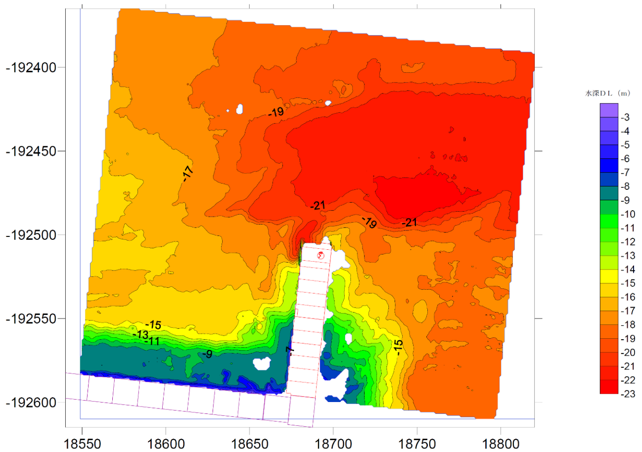
図-A.12.46 No.4 仙台港区_外港地区_C防波堤のカラー段彩図（被災後）
