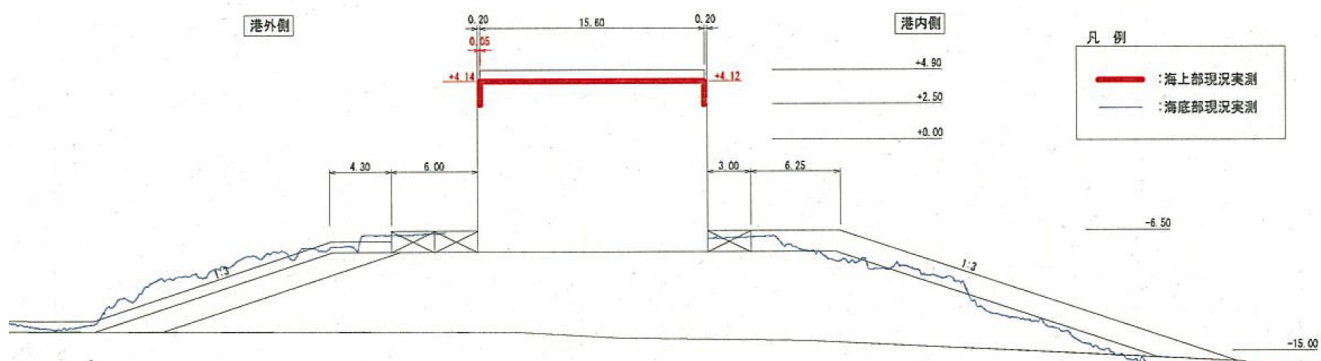
図-A.12.15 No.1 仙台港区_外港地区_北防波堤の断面図 D-D' (被災後)
