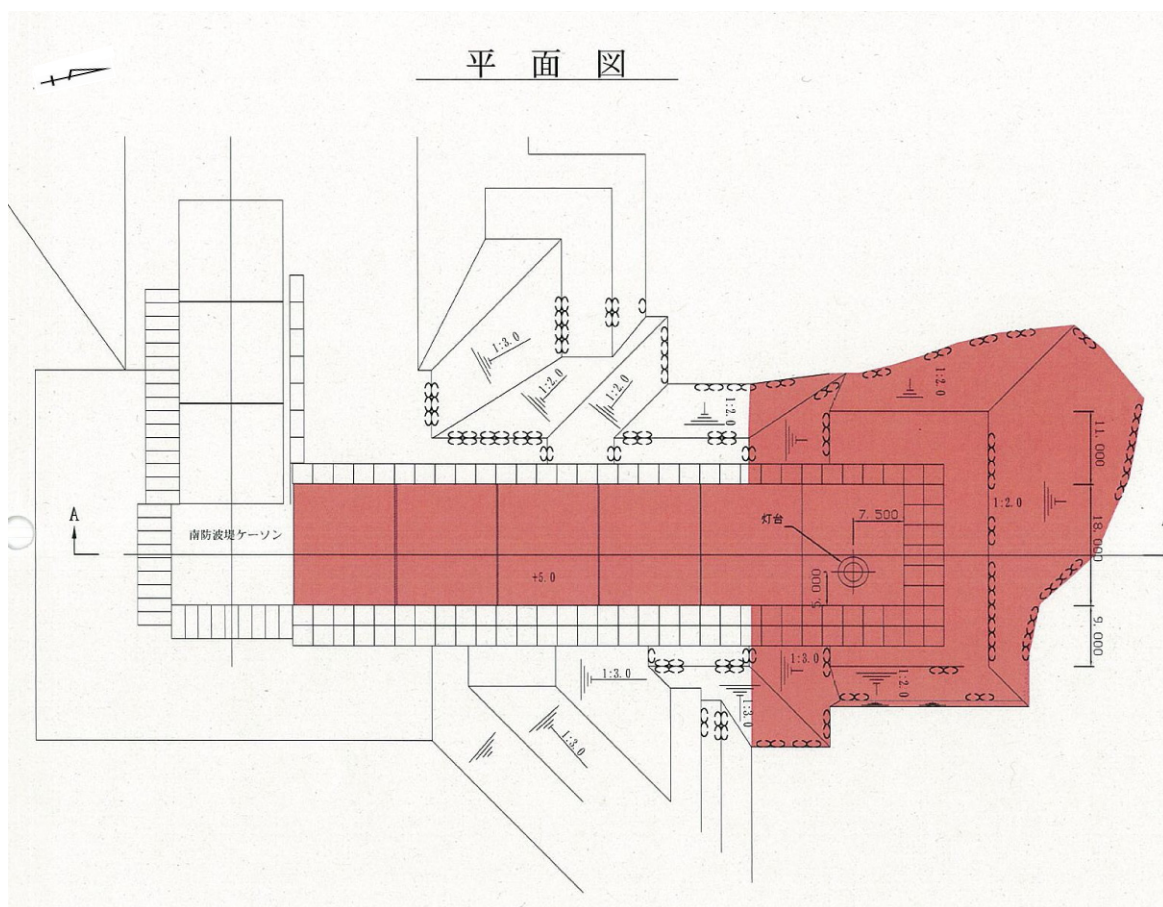
図-A. 12. 52 No. 4 仙台港区_外港地区_C 防波堤の平面図（復旧後）
