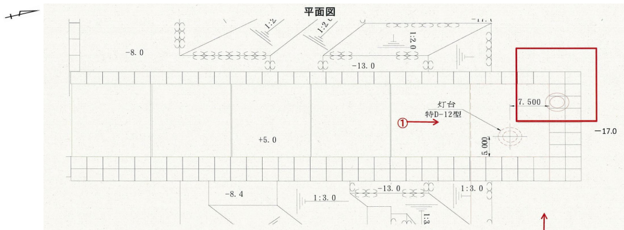
図-A.12.42 No.4 仙台港区_外港地区_C防波堤の平面図 (被災前)
