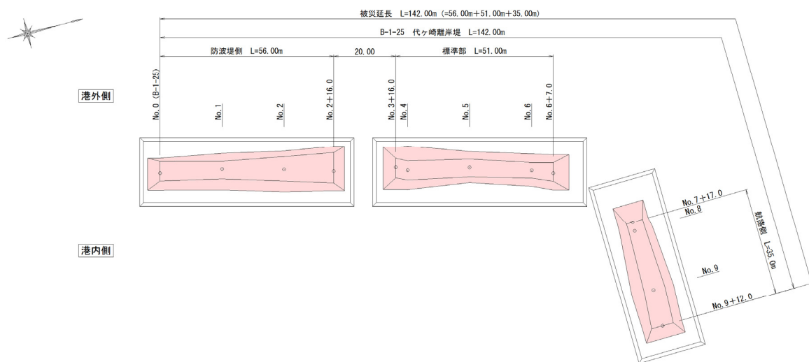
図-A. 12. 333 No. 1 塩釜港区_代ヶ崎離岸堤の平面図（被災後）
