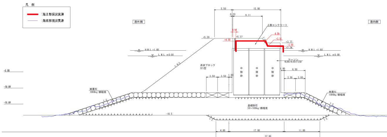
図-A.12.35 No.3 仙台区_外港地区_沖防波堤の断面図 F-F' (被災後)
