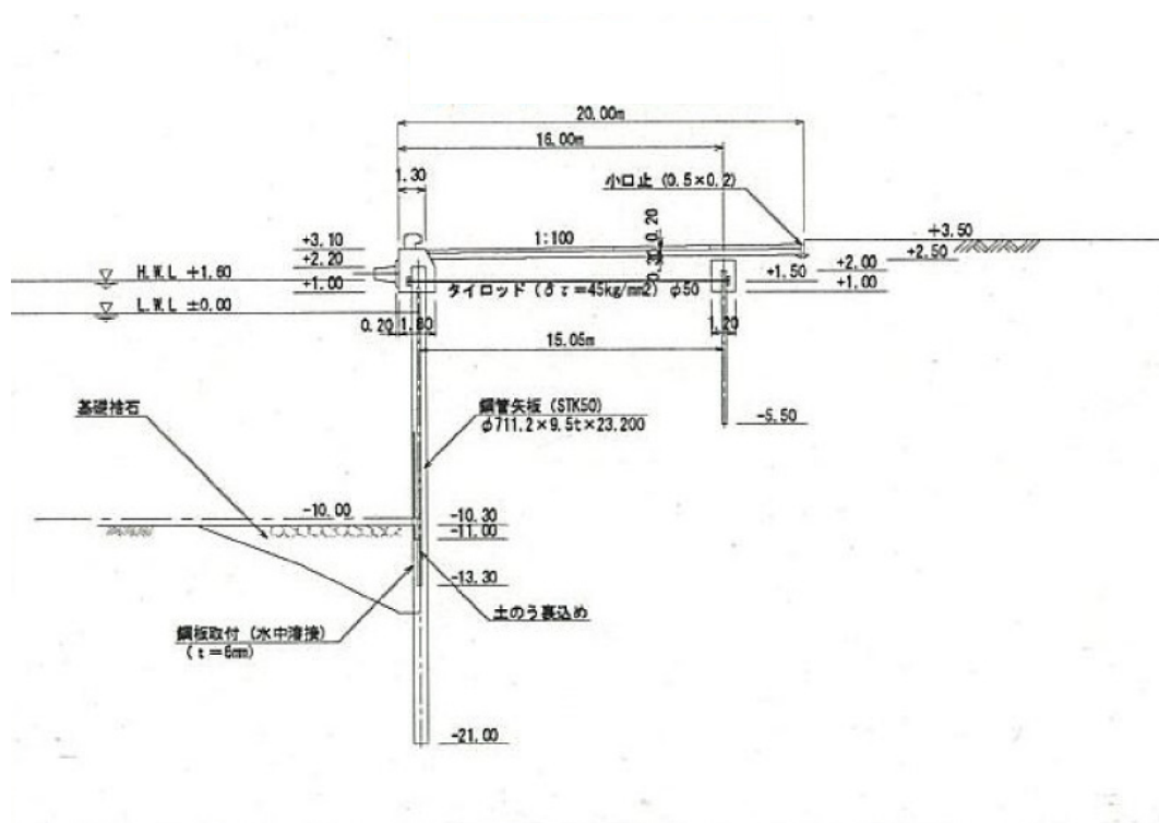
図-A. 12. 219 No.6 仙台港区_中野地区_4号岸壁 (-10m) の断面図 (被災前)
