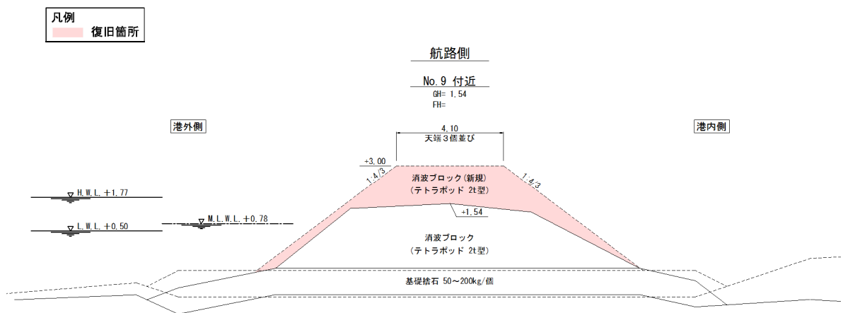
図-A. 12. 335 No. 1 塩釜港区_代ヶ崎離岸堤の断面図 (復旧後)
