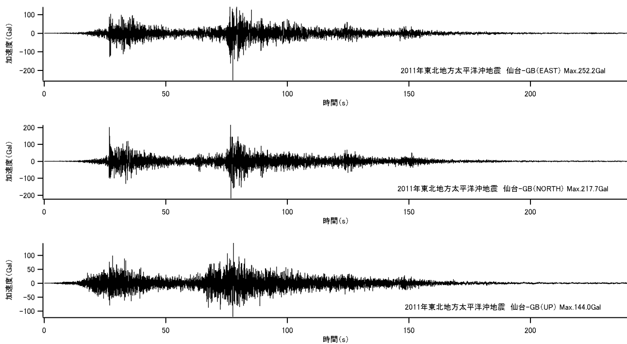
図－A. 12. 3 仙台塩釜港（仙台港区）の地中（仙台-GB）において観測された本震の加速度波形 28)
