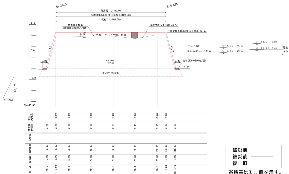
図-A.12.337 No.2 仙台港区_湊浜離岸堤の縦断面図 (被災後)
