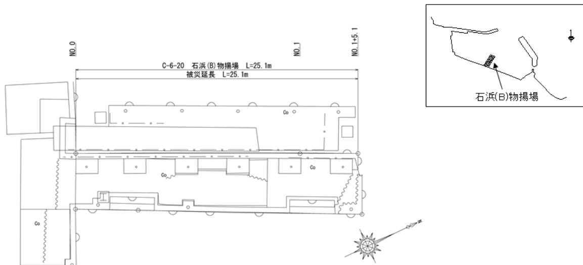
図-A.12.255 No.4 塩釜港区_石浜 (B) 物揚場の平面図 (被災後)
