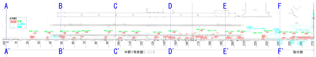
図-A.12.207 No.5 仙台港区_中野地区_岸壁 (-12m) の平面図 (被災後)
