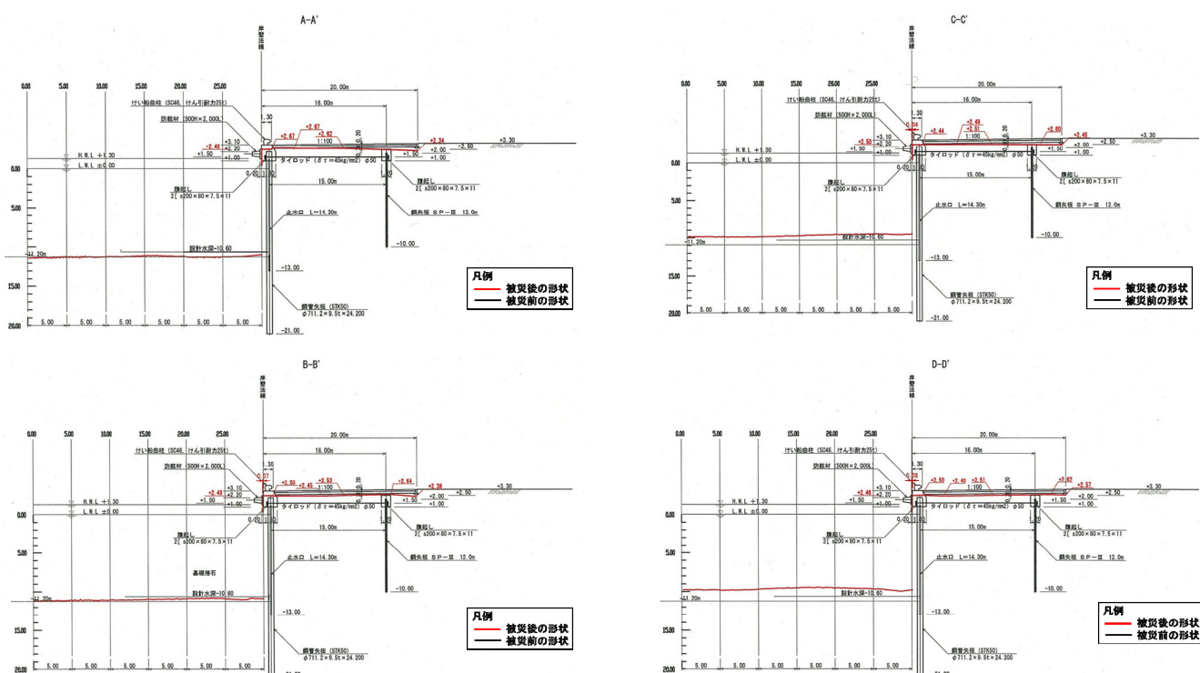
図-A.12.230 No.6 仙台港区_中野地区_4号岸壁 (-10m) の断面図 (被災後)
