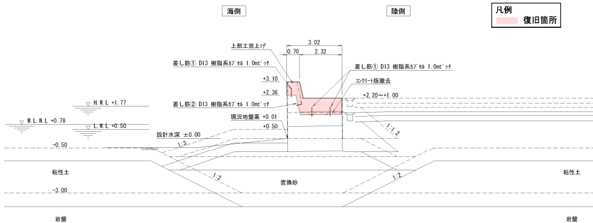
図-A.12.112 No. 14 塩釜港区_東宮浜東側防波護岸の断面図 No. 2 地点（復旧後）
