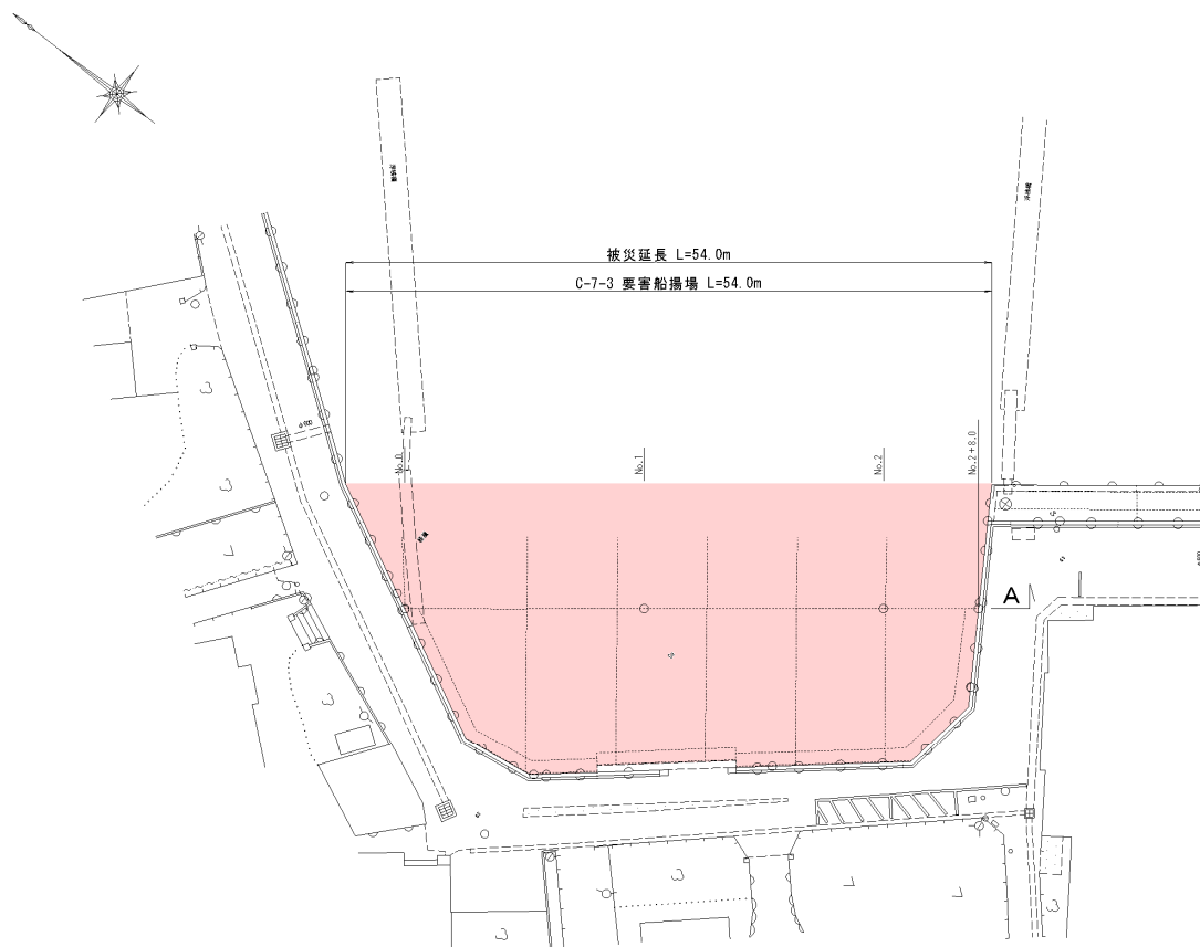
図-A. 12. 324 No. 29 塩釜港区_要害船揚場の平面図（被災後）
