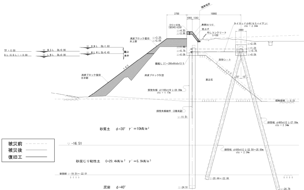
図-A.12.134 No. 18 仙台港区_向洋ふ頭防波護岸の断面図（復旧後）
