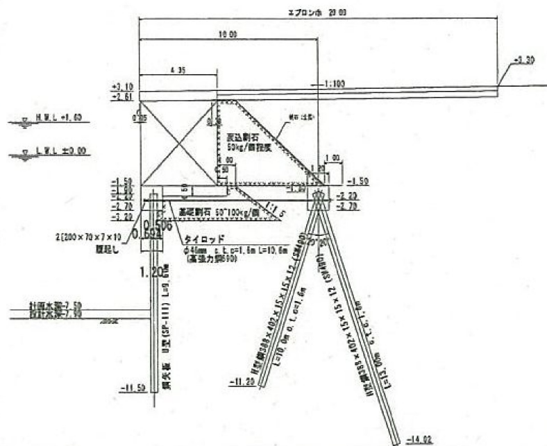
図-A. 12. 190 No.4 仙台港区_中野地区_岸壁 (-7.5m) の断面図 A-A (被災前)
