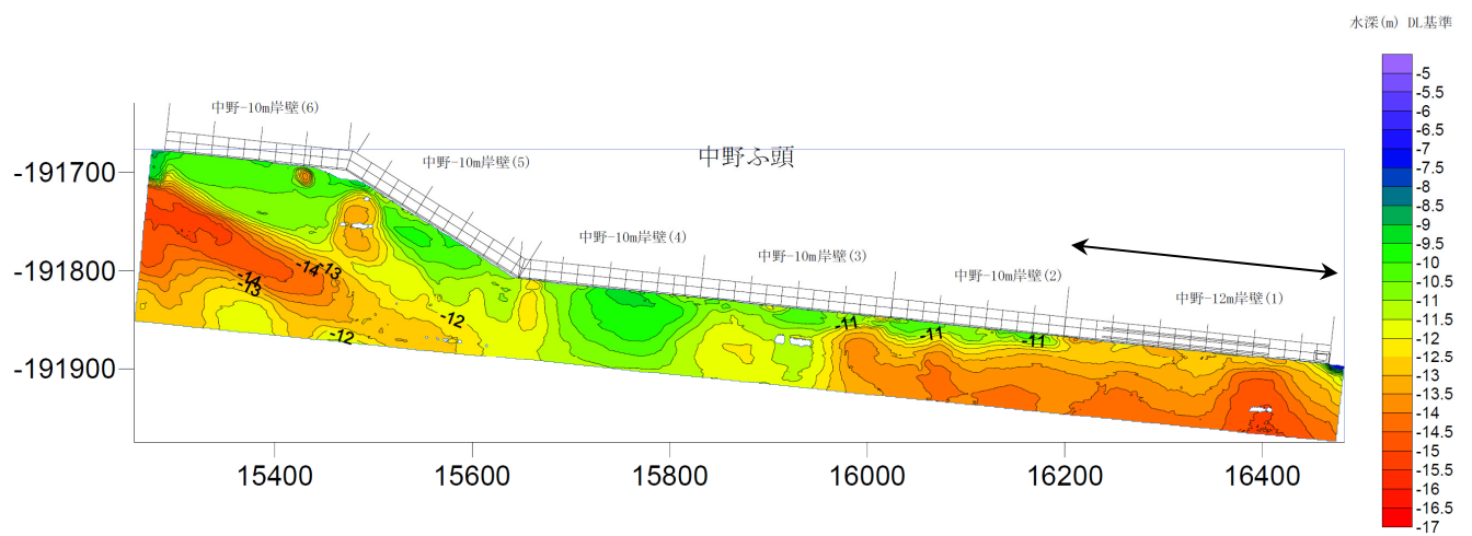
図-A.12.208 No.5 仙台港区_中野地区_岸壁 (-12m) のカラー段彩図 (被災後)
