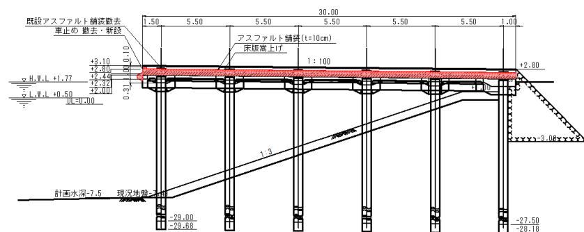
図-A. 12. 306 No. 22 塩釜港区_貞山ふ頭 3 号・4 号さん橋の断面図 (復旧後)
