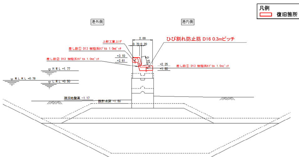
図-A.12.82 No.6 塩釜港区_代々崎清水防波堤の断面図 ANo.1+1.74（復旧後）
