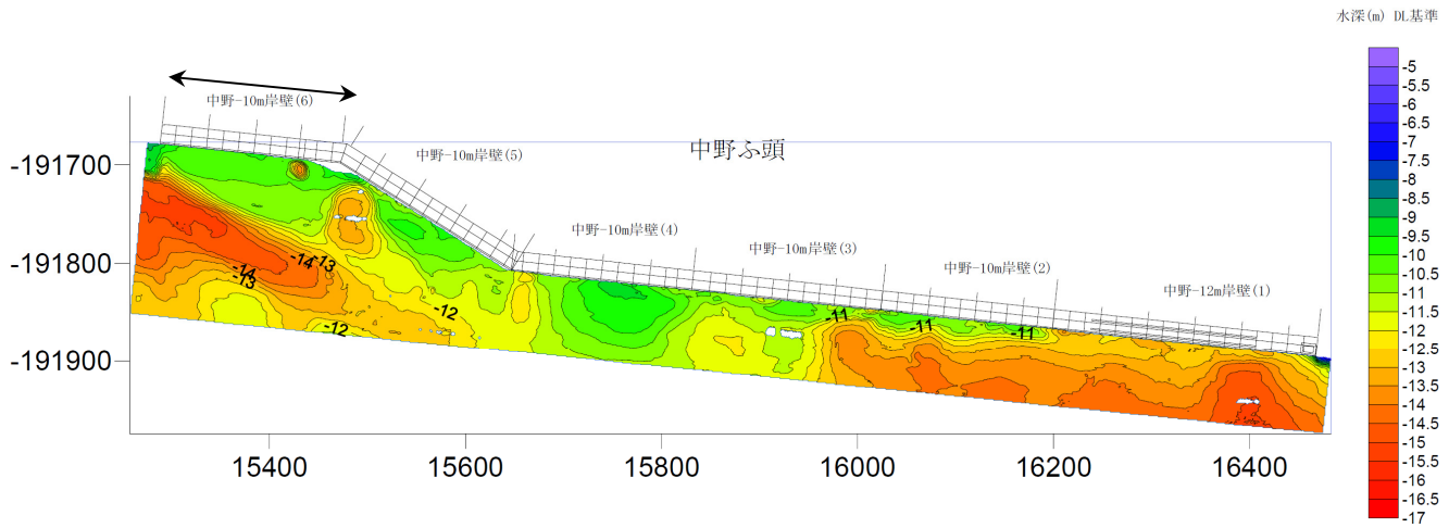
図-A.12.235 No.6 仙台港区_中野地区_6号岸壁 (-10m) のカラー段彩図 (被災後)
