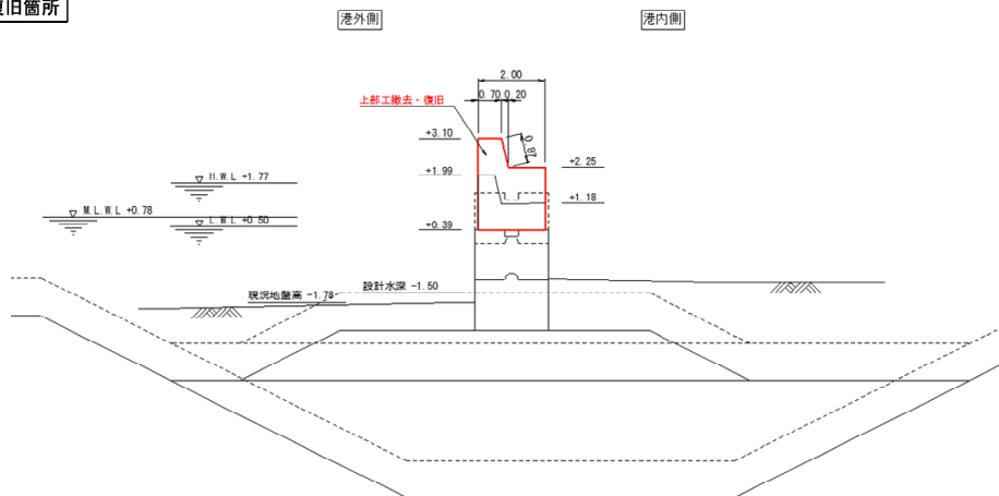
図一A.12.83 No.6 塩釜港区_代ヶ崎清水防波堤の断面図 ANo.3 (復旧後)
