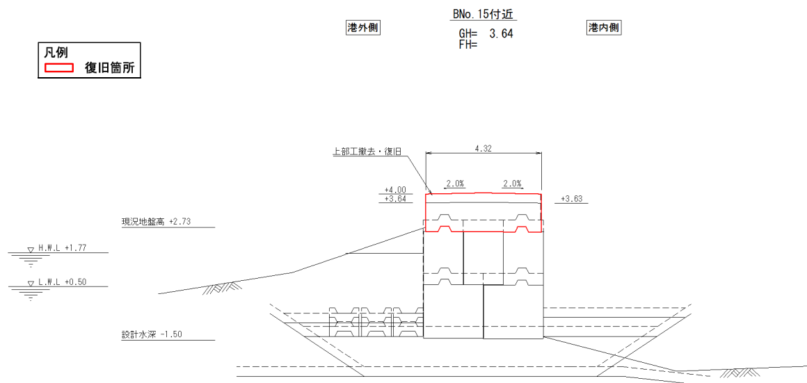
図-A.12.73 No.3 塩釜港区_小浜防波堤 (B)断面図 B-1 工区 (復旧後)
