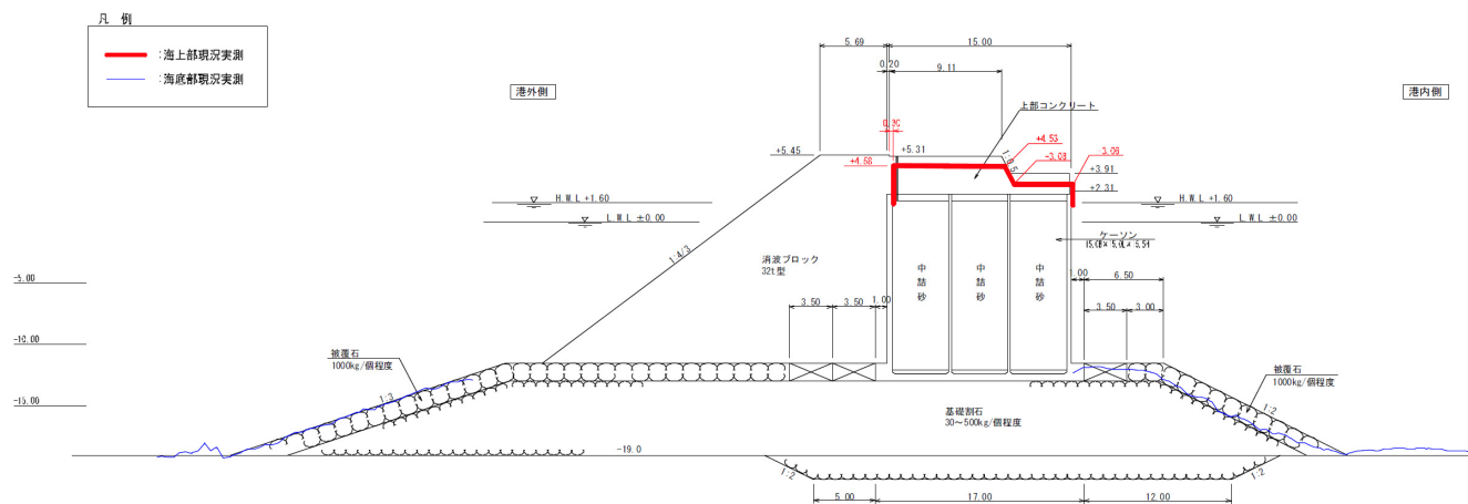
図-A.12.31 No.3 仙台港区_外港地区_沖防波堤の断面図 C-C' (被災後)
