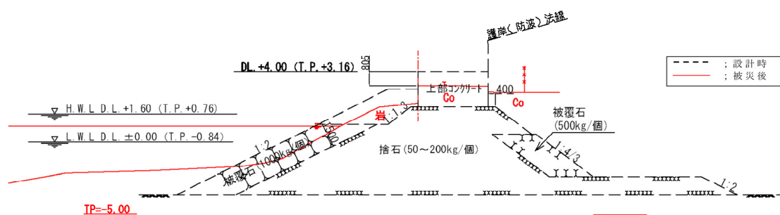
図-A.12.157 No.23 仙台港区_向洋埠頭西護岸の断面図(被災後)
