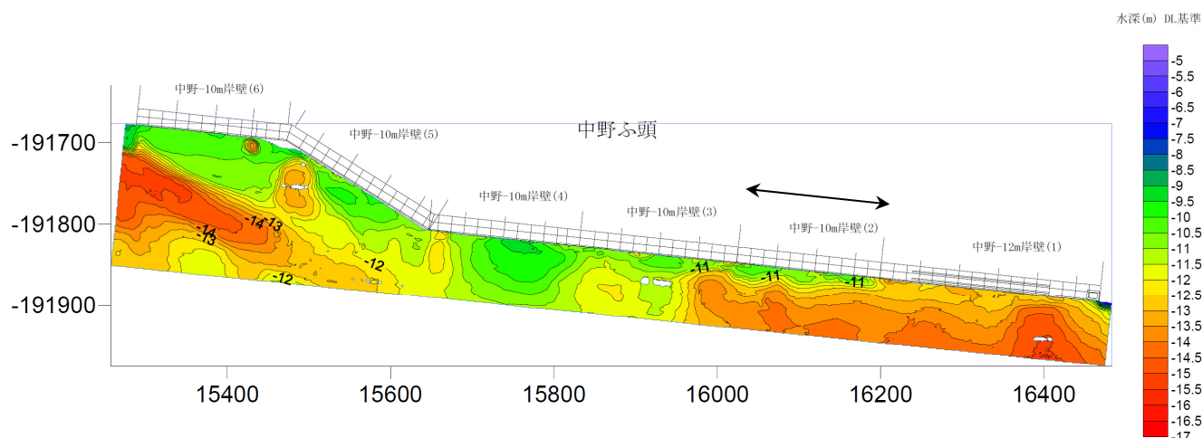
図-A.12.223 No.6 仙台港区_中野地区_2号岸壁 (-10m) のカラー段彩図 (被災後)
