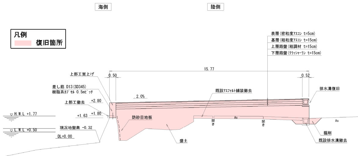
図一A.12.97 No.10 塩釜港区_東ふ頭護岸・貞山ふ頭西護岸の断面図 BN0.3+19.10 (復旧後)
