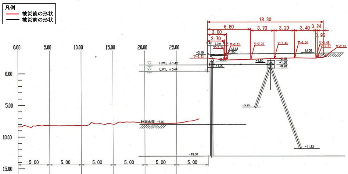
図-A. 12. 60 No. 5 仙台港区_中野地区_護岸Ⅱの断面図 B-B' (被災後)
