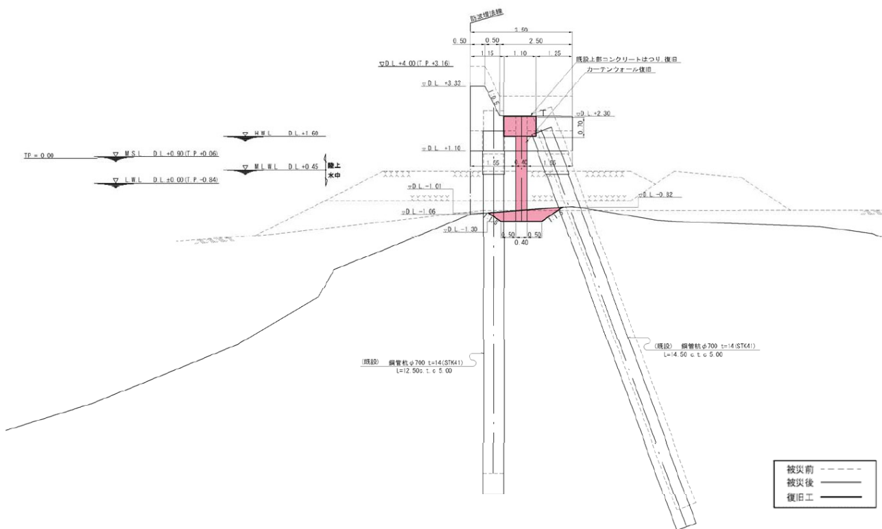
図-A. 12. 129 No. 17 仙台港区_高砂防波堤の断面図③ (被災後)
