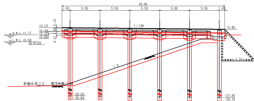
図-A. 12. 305 No. 22 塩釜港区_貞山ふ頭 3 号・4 号さん橋の断面図 (被災後)
