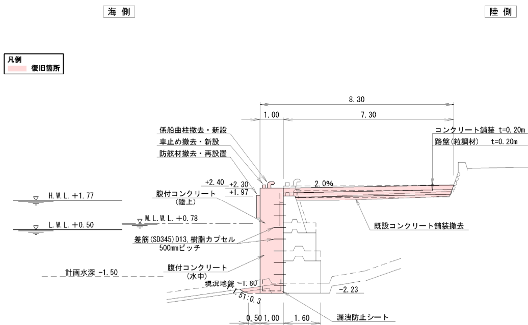
図-A. 12. 261 No. 6 塩釜港区_代ヶ崎 (B) 物揚場の断面図 (復旧後)
