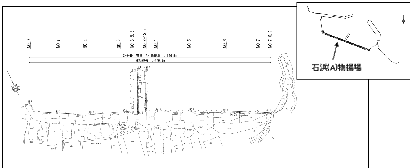
図－A.12.253 No.3 塩釜港区_石浜 (A) 物揚場の平面図（被災後）
