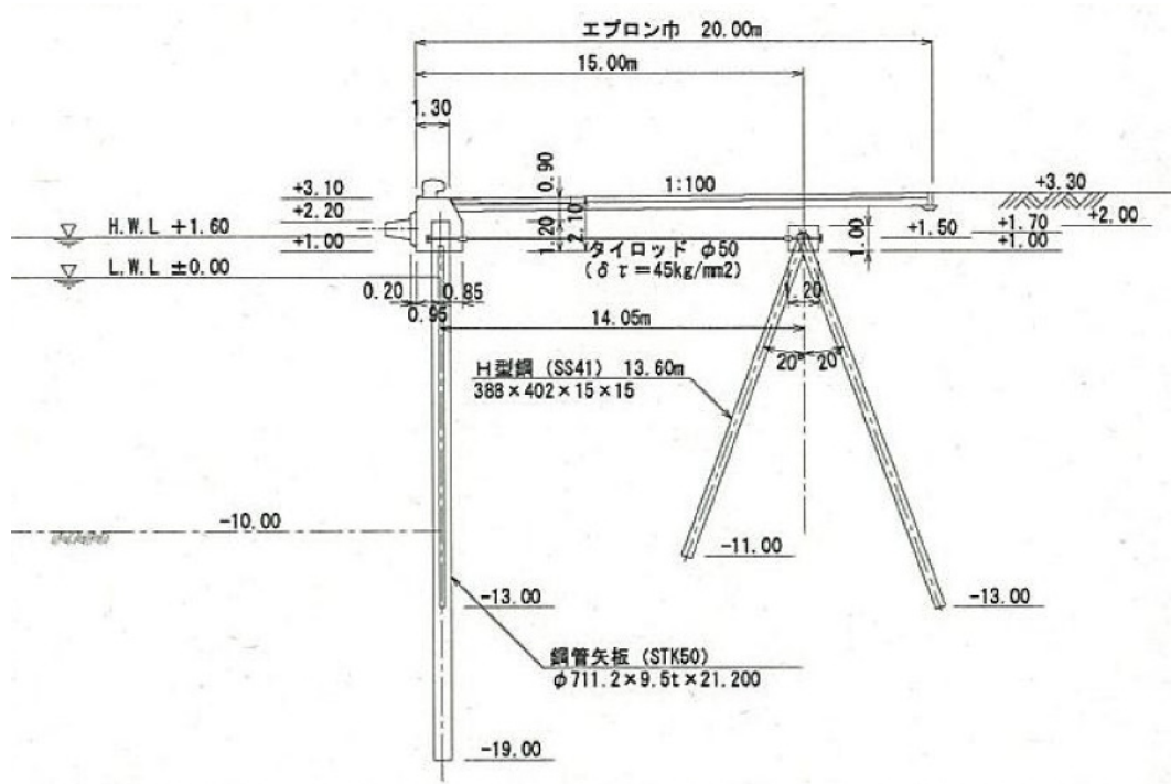
図-A. 12. 220 No.6 仙台港区_中野地区_5号岸壁 (-10m) の断面図 (被災前)
