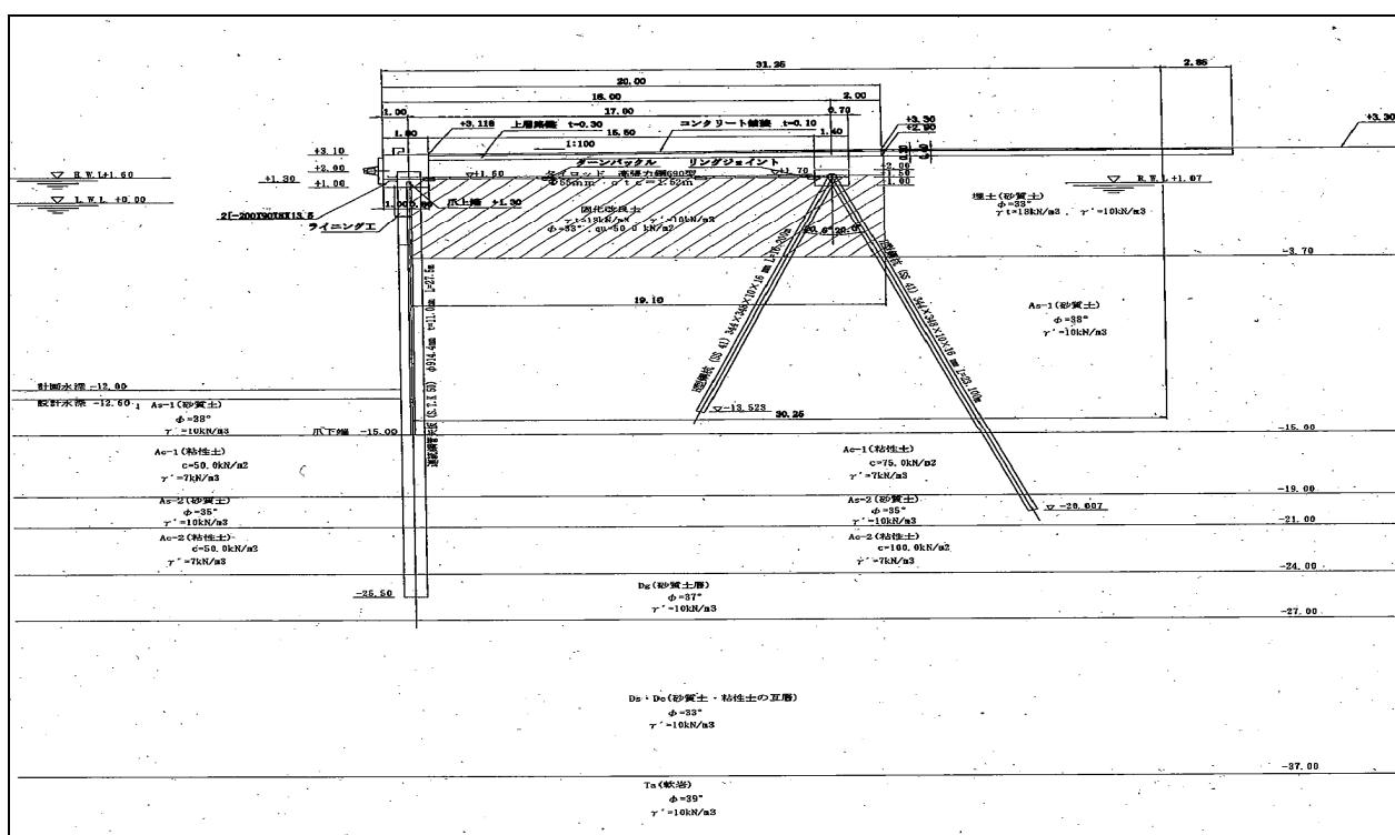
図-A.12.178 No.3 仙台港区_中野地区_高松木材埠頭岸壁 (-12m) の断面図 (標準) (被災前)
