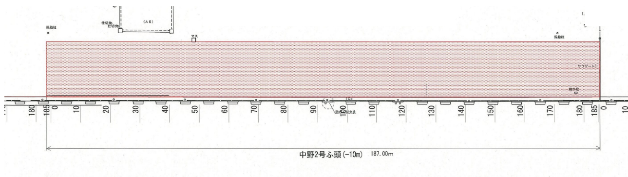
図-A. 12. 237 No.6 仙台港区_中野地区_2号岸壁 (-10m) の平面図 (復旧後)
