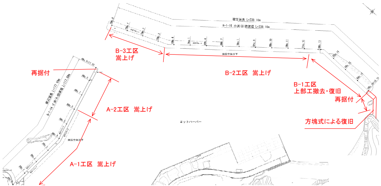
図-A.12.72 No.3 塩釜港区_小浜防波堤 (B)の平面図 (復旧後)
