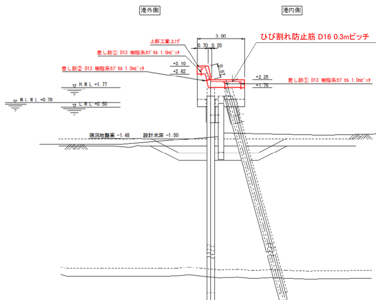
図一A.12.84 No.6 塩釜港区_代ヶ崎清水防波堤の断面図 ANo.6 (復旧後)
