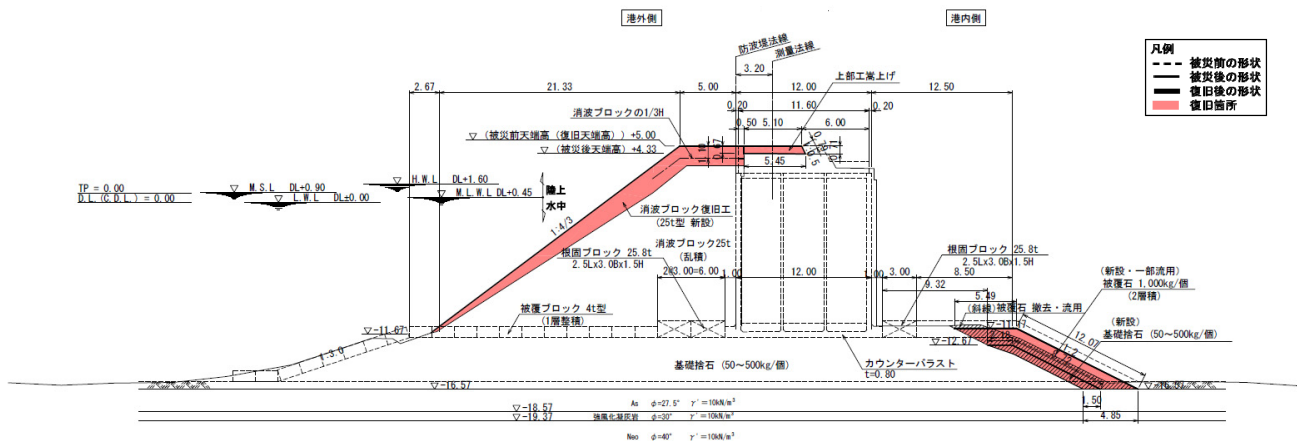
図-A.12.121 No.16 仙台区_新北防波堤の断面図 No.12 地点 (被災前・後_復旧後)
