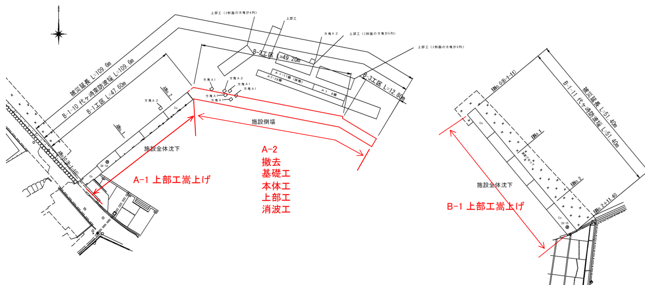
図-A.12.92 No. 9 塩釜港区_代ヶ崎防波堤の平面図（復旧後）
