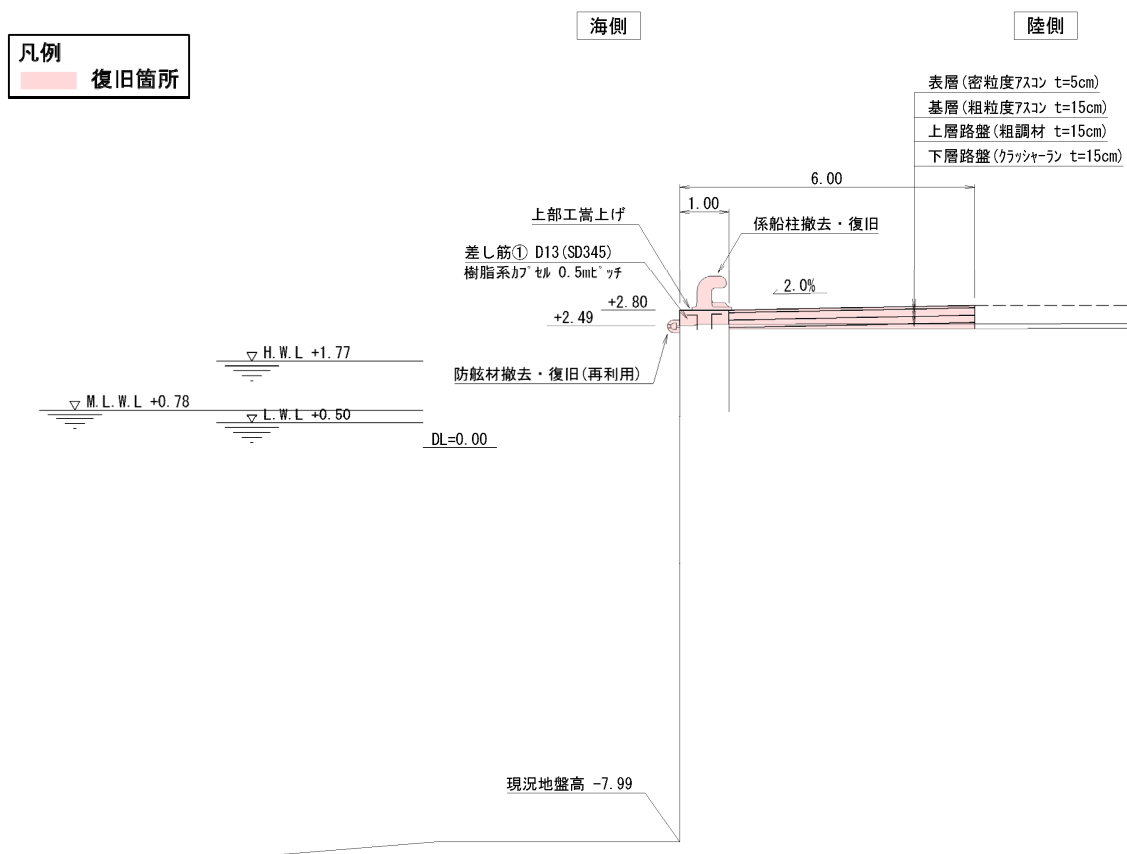
図-A.12.95 No.10 塩釜港区_東ふ頭護岸・貞山ふ頭西護岸の断面図 BN0.0（復旧後）
