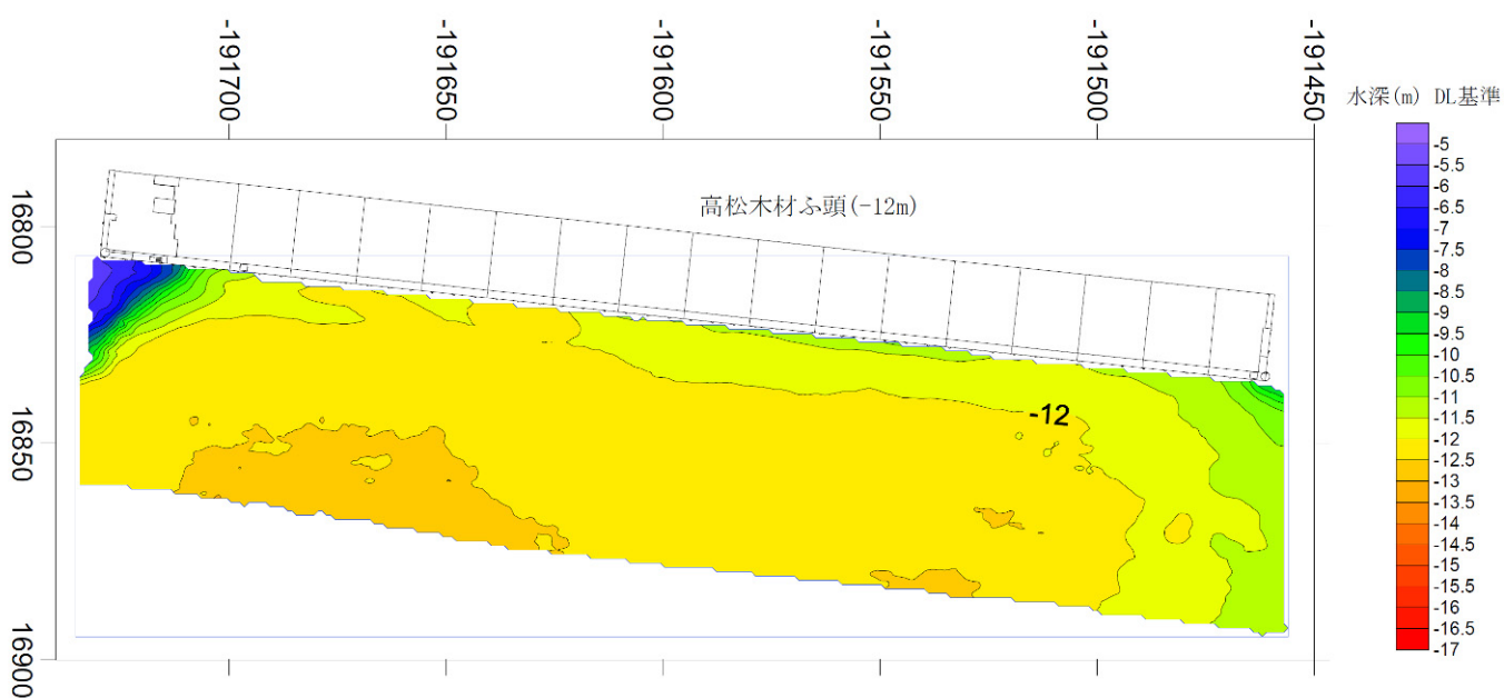
図-A.12.180 No.3 仙台港区_中野地区_高松木材埠頭岸壁（-12m）のカラー段彩図（被災後）
