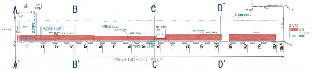
図-A.12.234 No.6 仙台港区_中野地区_6号岸壁 (-10m) の平面図 (被災後)
