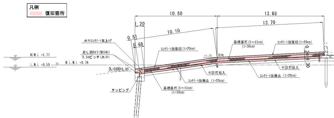
図-A. 12. 325 No. 29 塩釜港区_要害船揚場の断面図（復旧後）
