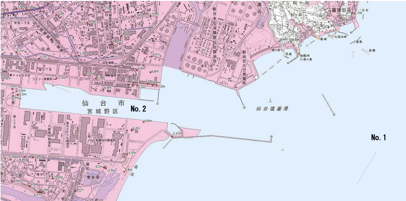
図－A. 12. 329 仙台塩釜港の被災港湾施設（水域施設，直轄分）
