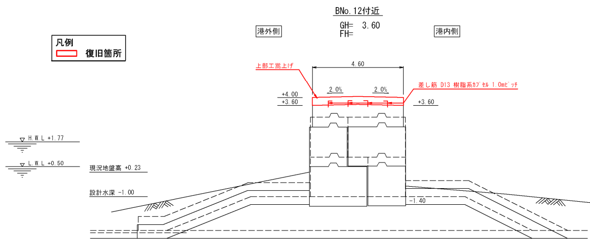
図-A. 12. 74 No. 3 塩釜港区_小浜防波堤 (B)断面図 B-2 工区 (復旧後)
