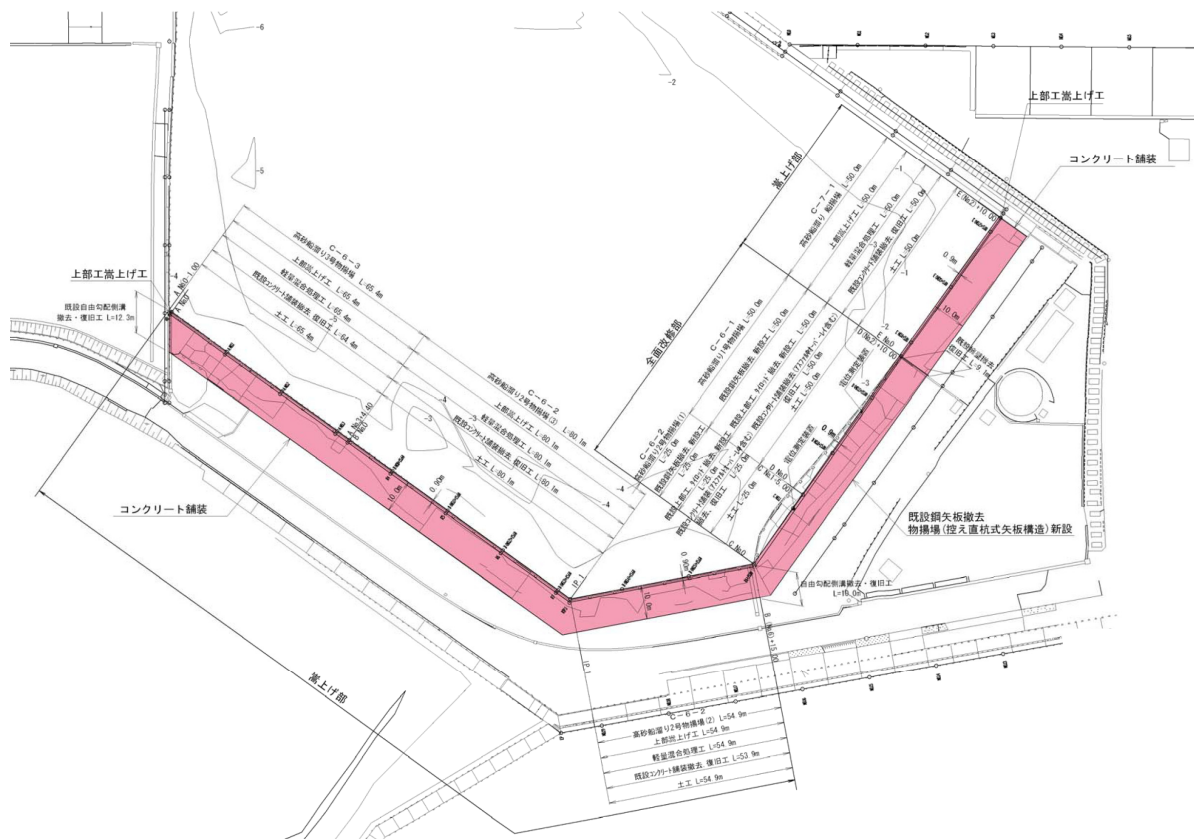
図一A.12.326 No. 30 仙台港区_高砂船溜物揚場の平面図（被災後）
