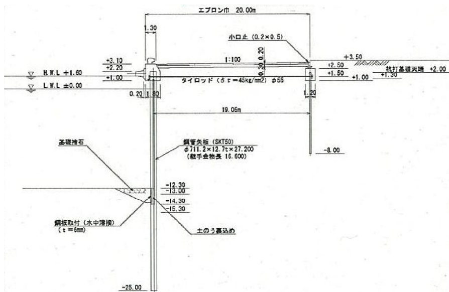
図-A. 12. 206 No.5 仙台港区_中野地区_岸壁 (-12m) の平面図 (被災前)
