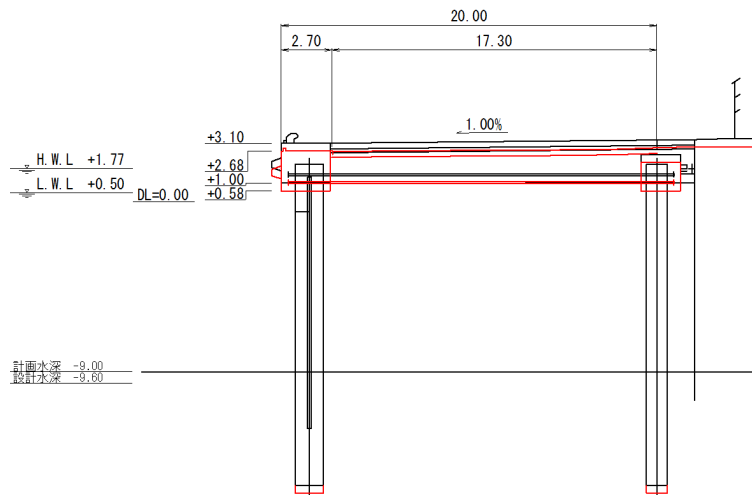
図-A. 12. 301 No. 21 塩釜港区_貞山ふ頭 2 号岸壁の断面図 (被災後)
