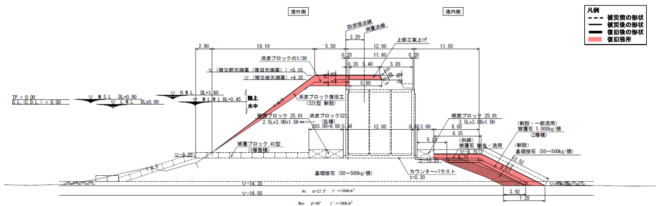
図一A.12.119 No.16 仙台港区_新北防波堤の断面図 No.3 地点 (被災前・後_復旧後)
