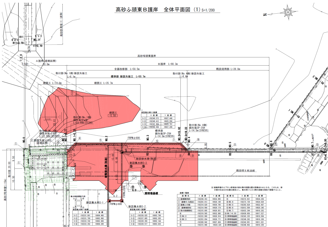
図-A.12.146 No.20 仙台港区_高砂ふ頭東B護岸の平面図(被災後)
