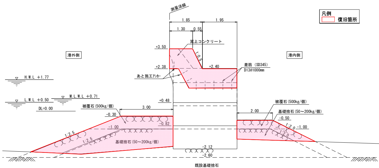
図-A.12.79 No. 5 塩釜港区_石浜北防波堤の断面図（復旧後）
