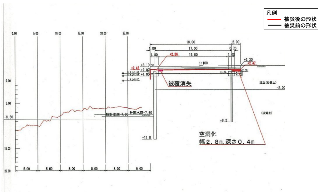
図-A. 12. 181 No.3 仙台区_中野地区_高松木材埠頭岸壁（-12m）の断面図 A-A'（被災後）
