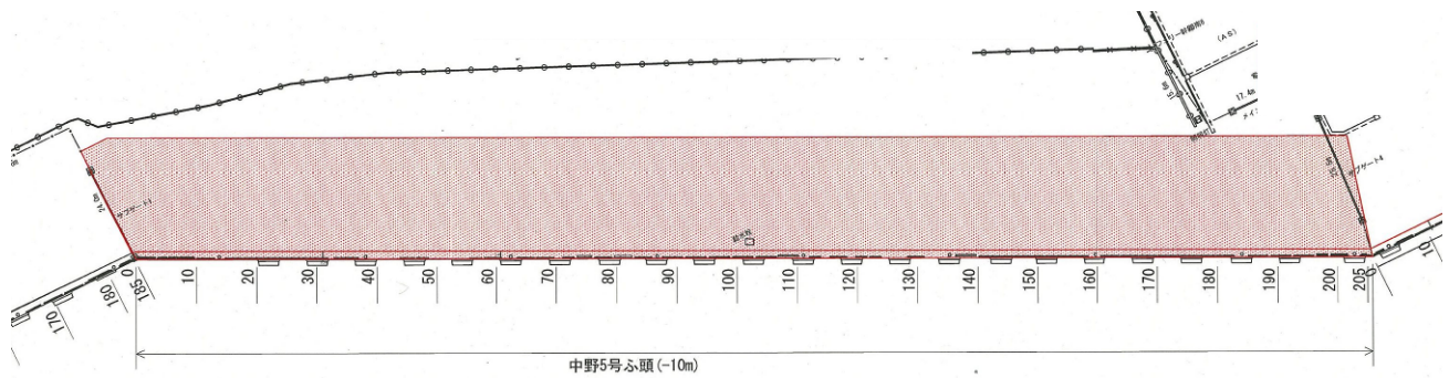
図-A.12.243 No.6 仙台港区_中野地区_5号岸壁 (-10m) の平面図 (復旧後)
