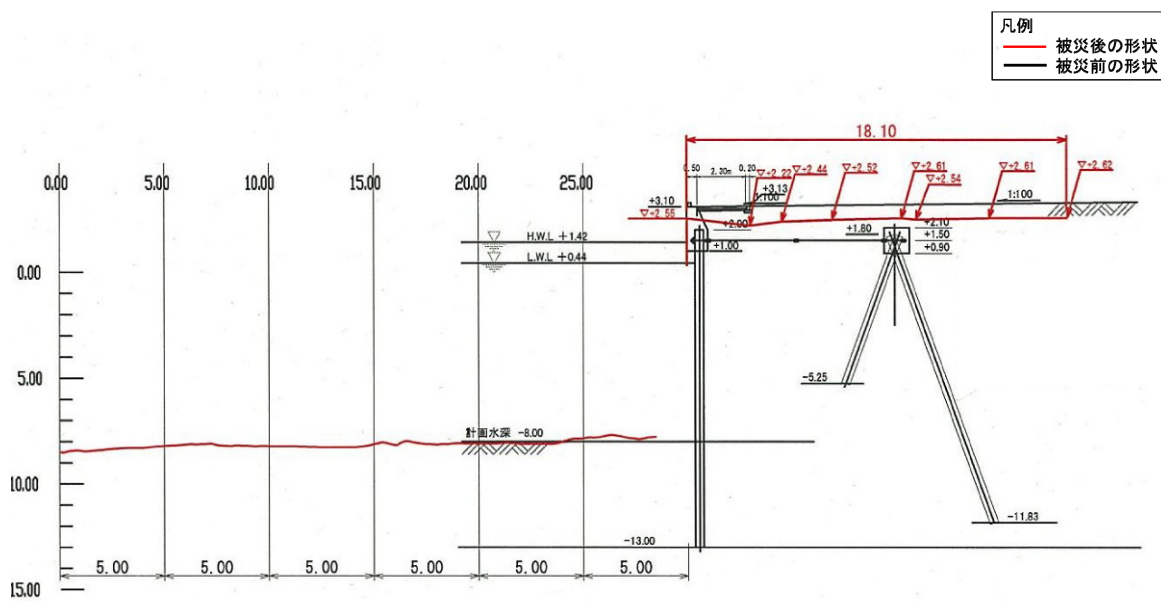
図-A. 12. 61 No. 5 仙台港区_中野地区_護岸Ⅱの断面図 C-C' (被災後)
