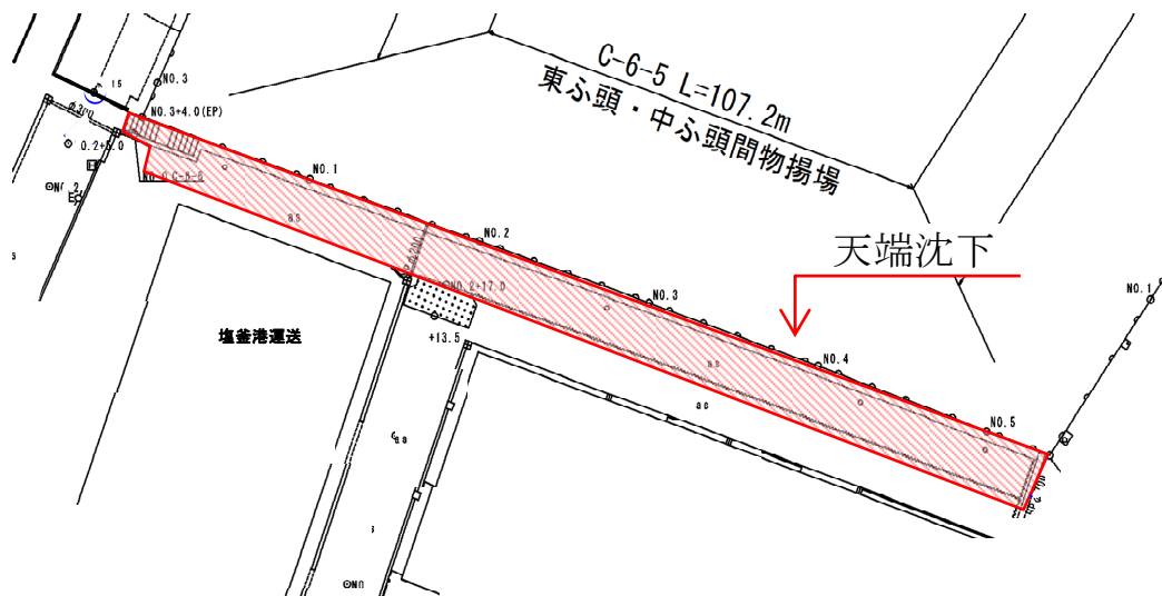
図-A. 12. 308 No. 23 塩釜港区_東ふ頭・中ふ頭間物揚場の平面図（被災後）
