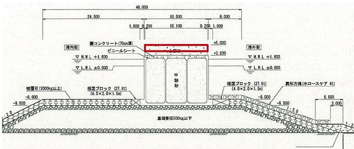
図-A. 12. 20 No. 2 仙台港区_外港地区_南防波堤の断面図 A-A' (被災後)
