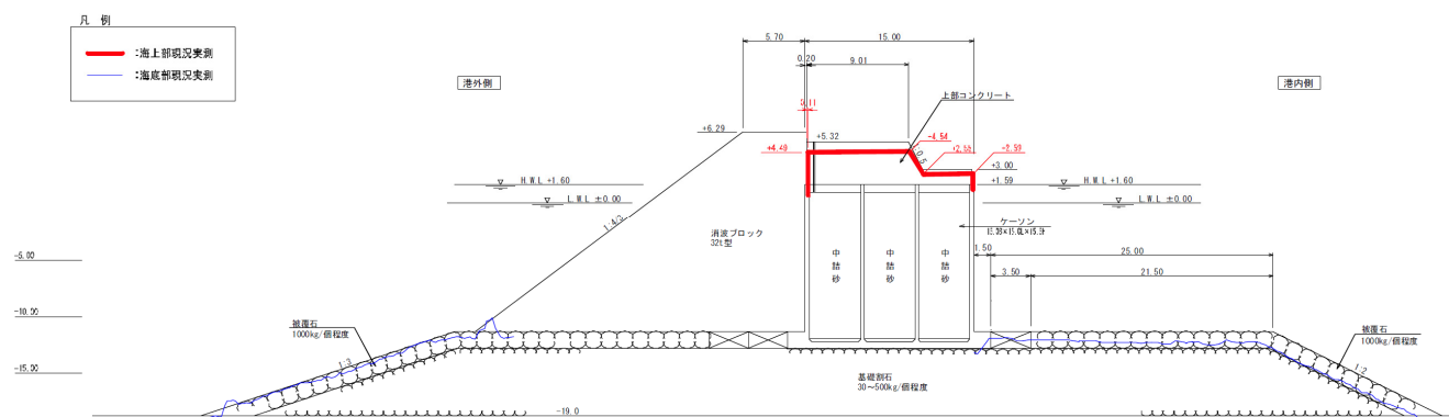
図-A.12.29 No.3 仙台港区_外港地区_沖防波堤の断面図 A-A'（被災後）
