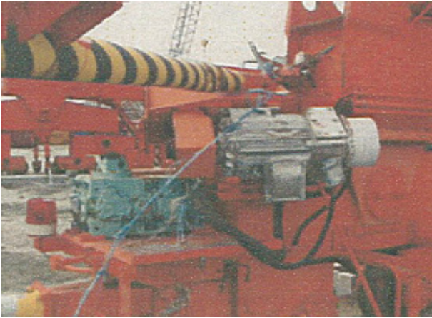
図-A. 12. 353 走行モータ軸の折損(海脚, 1号機)
