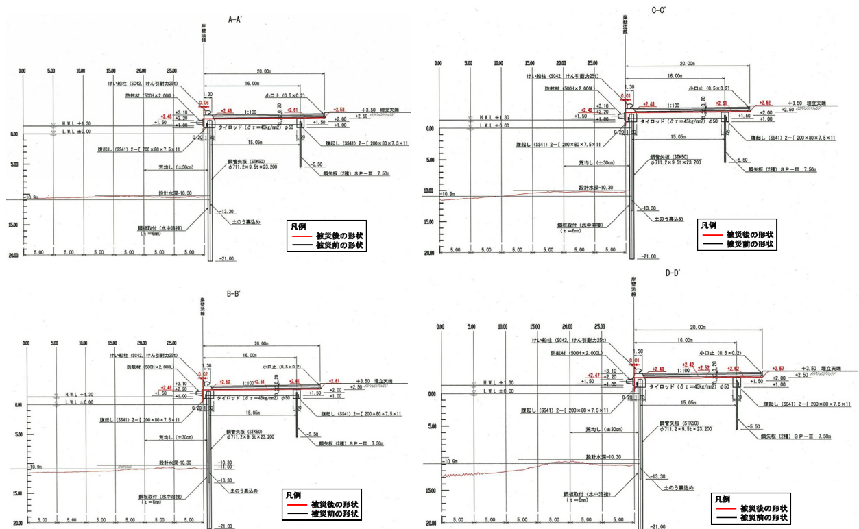
図-A.12.227 No.6 仙台港区_中野地区_3号岸壁 (-10m) の断面図 (被災後)
