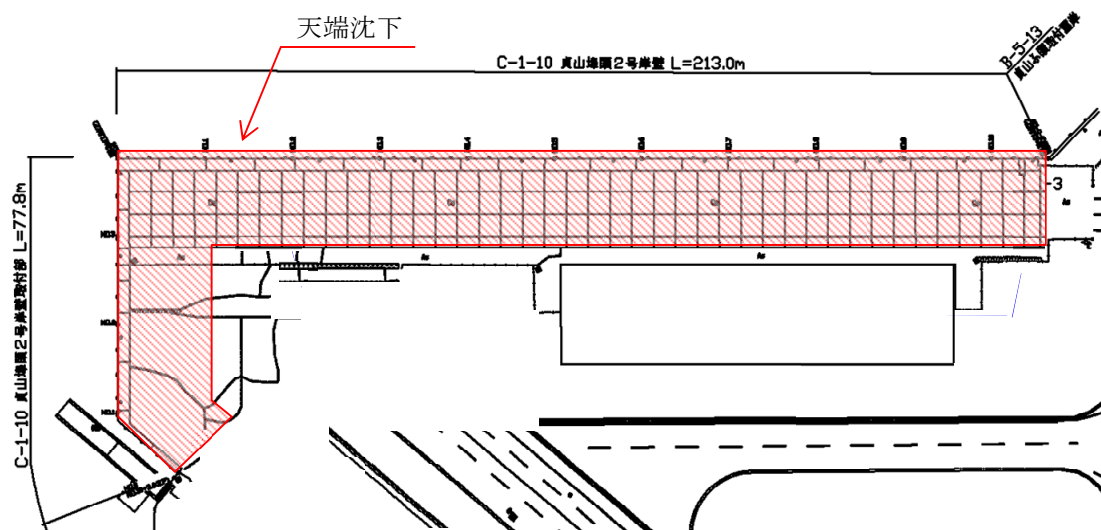
図-A. 12. 300 No. 21 塩釜港区_貞山ふ頭 2 号岸壁の平面図 (被災後)
