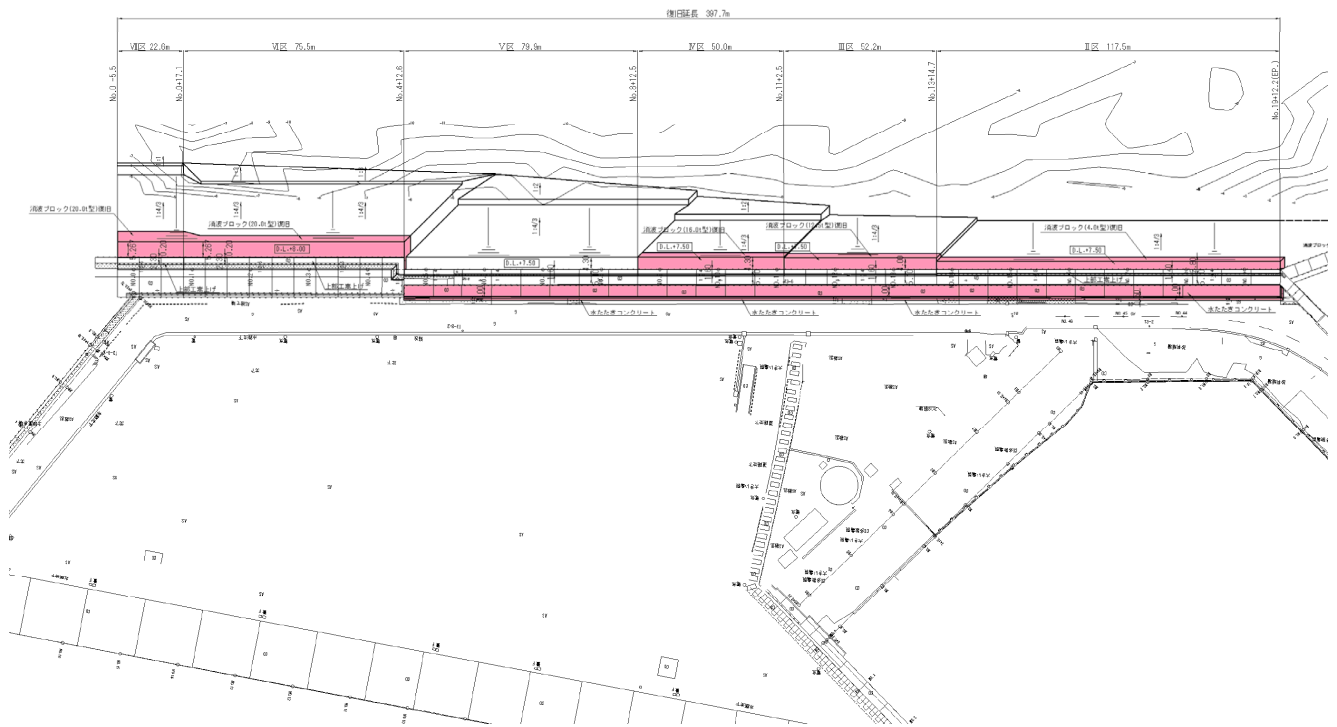
図-A.12.138 No.19 仙台港区_南防波護岸の平面図（被災後）
