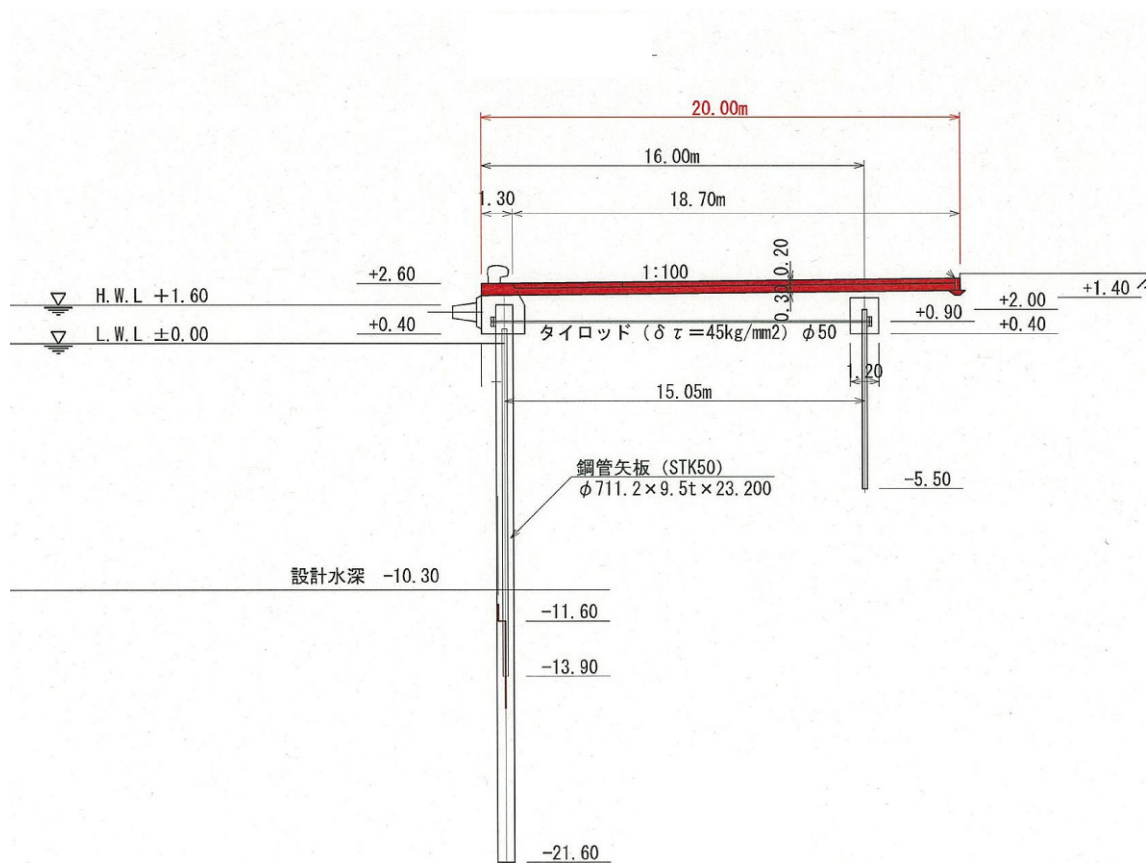
図-A.12.240 No.6 仙台港区_中野地区_3号岸壁 (-10m) の断面図 (復旧後)
