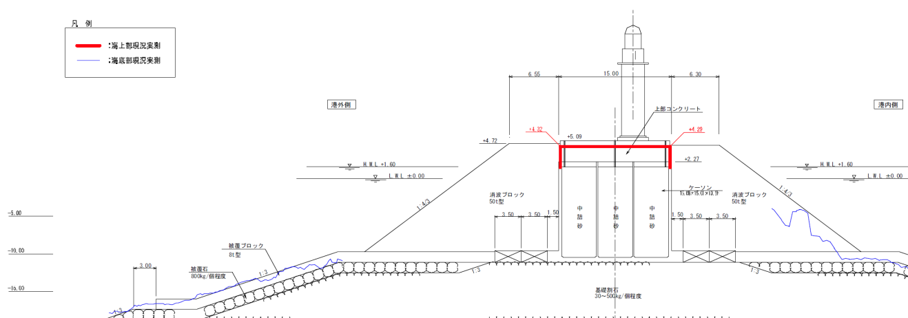
図-A.12.38 No.3 仙台港区_外港地区_沖防波堤の断面図 I-I' (被災後)
