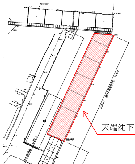
図-A.12.287 No. 17 塩釜港区_中ふ頭東側さん橋の平面図（被災後）
