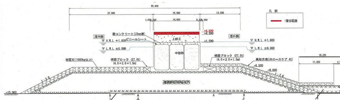
図-A.12.25 No.2 仙台港区_外港地区_南防波堤の断面図 C-C' (復旧後)
