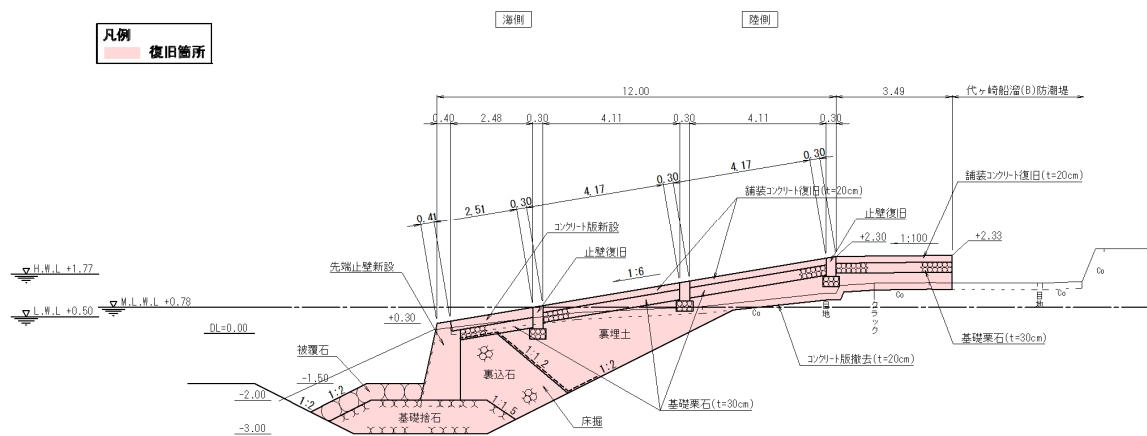
図-A.12.273 No.12 塩釜港区_代ヶ崎船たまり (B) 船揚場の断面図 (復旧後)
