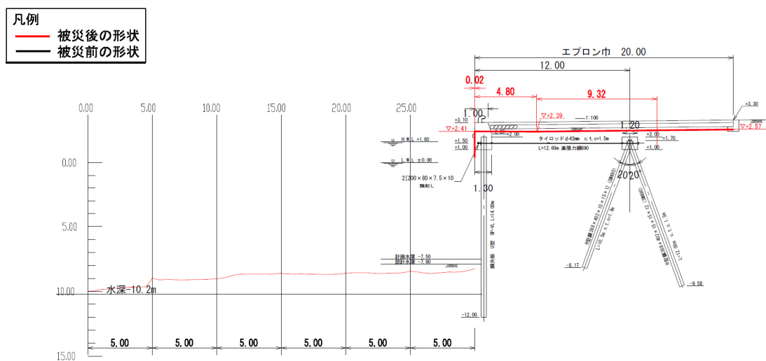
図-A.12.202 No.4 仙台港区_中野地区_岸壁 (-7.5m) の断面図 I-I' (被災後)
