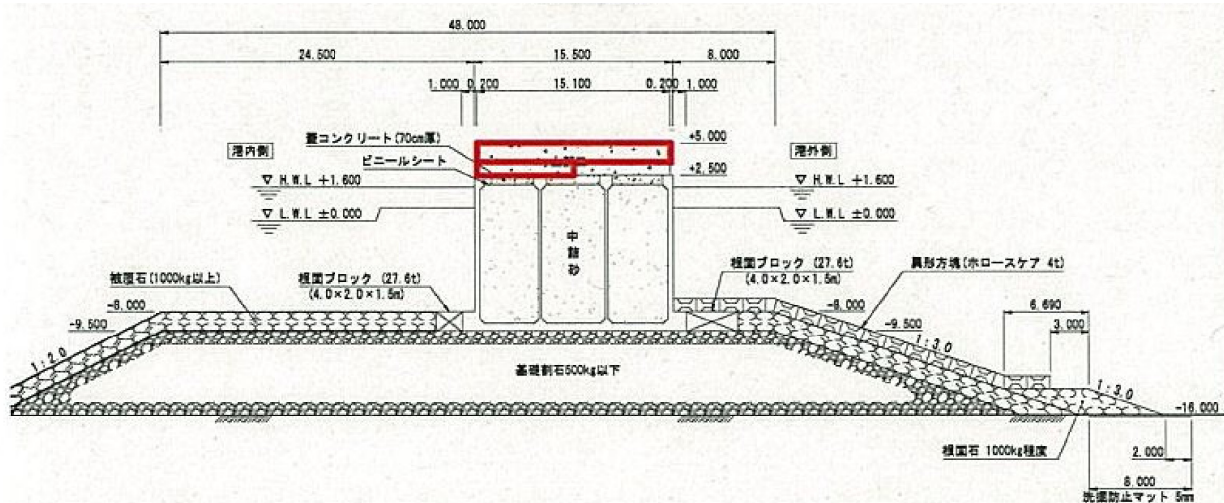
図-A. 12. 21 No. 2 仙台港区_外港地区_南防波堤の断面図 B-B' (被災後)
