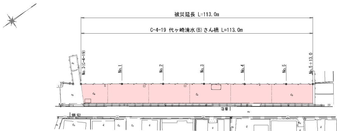
図-A.12.266 No.9 塩釜港区_代ヶ崎清水 (B) さん橋の平面図 (被災後)
