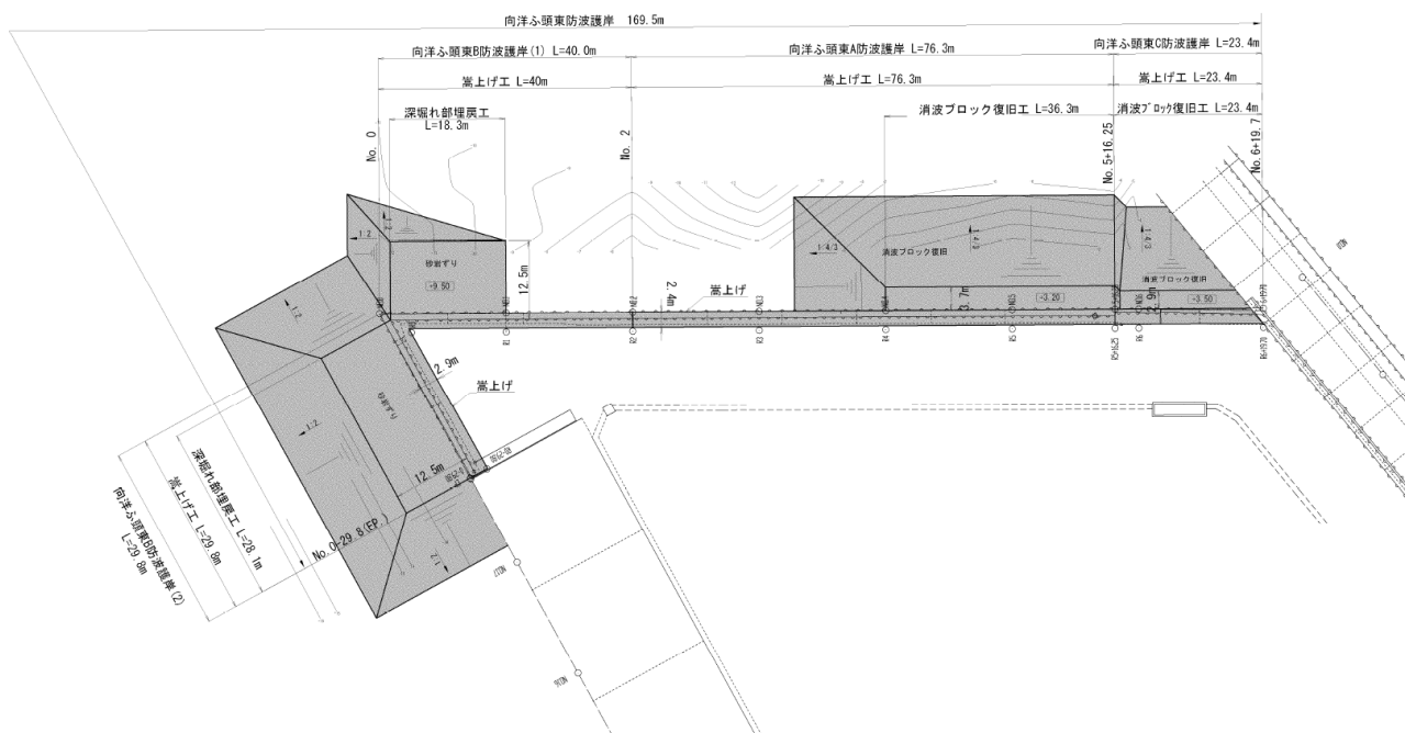
図-A.12.133 No. 18 仙台港区_向洋ふ頭防波護岸の平面図（復旧後）
