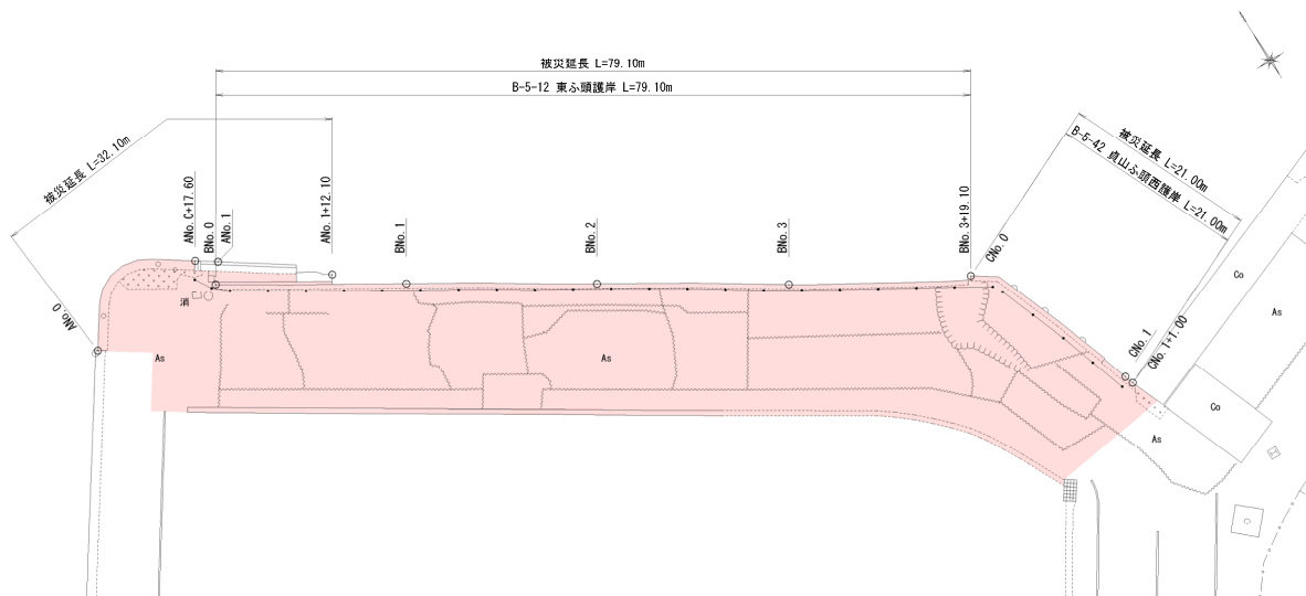
図-A.12.94 No.10 塩釜港区_東ふ頭護岸・貞山ふ頭西護岸の平面図（復旧後）
