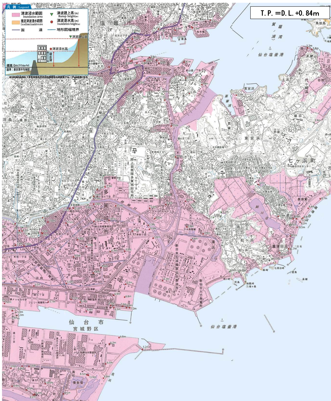
図-A.12.5 仙台塩釜港の津波痕跡図 1)
