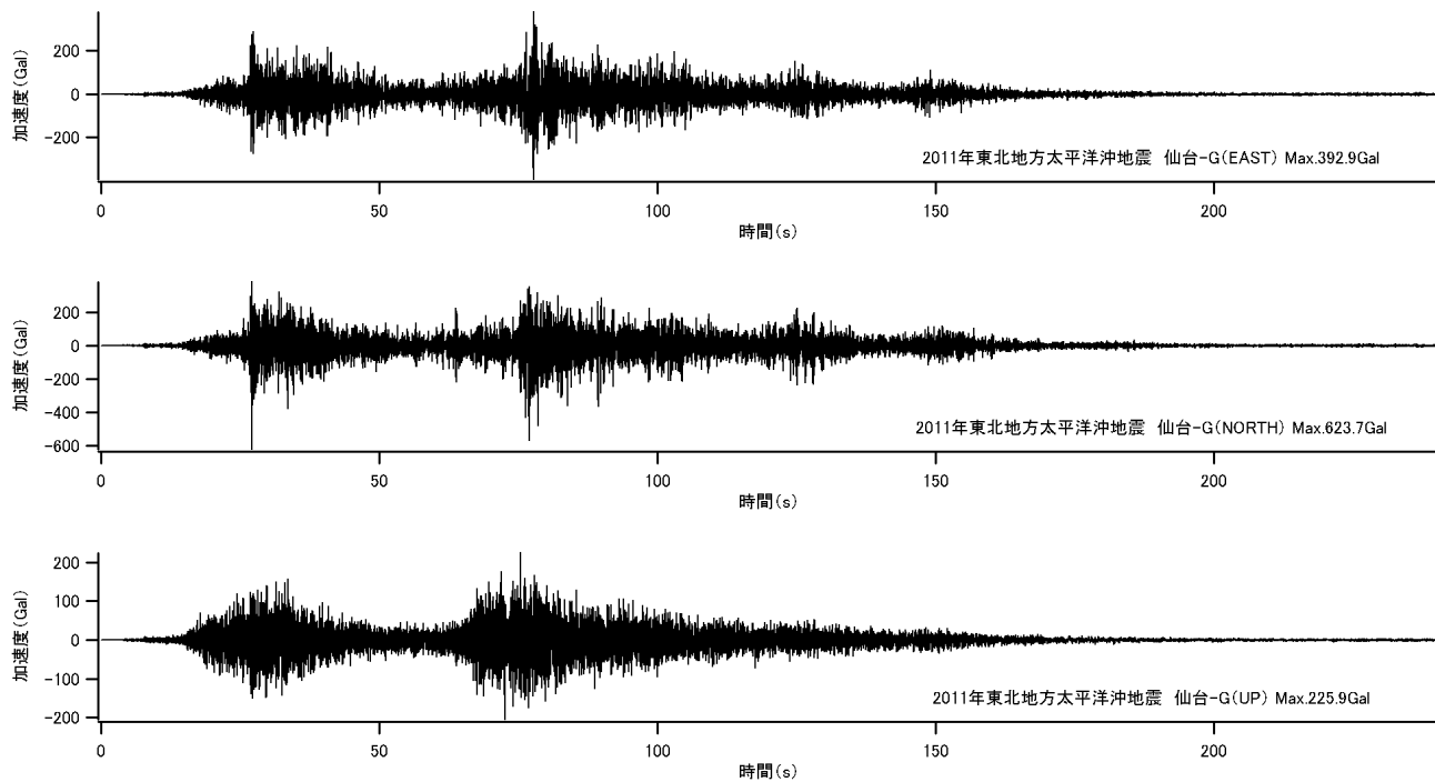
図－A. 12. 4 仙台塩釜港（仙台港区）の地表（仙台-G）において観測された本震の加速度波形 28)
