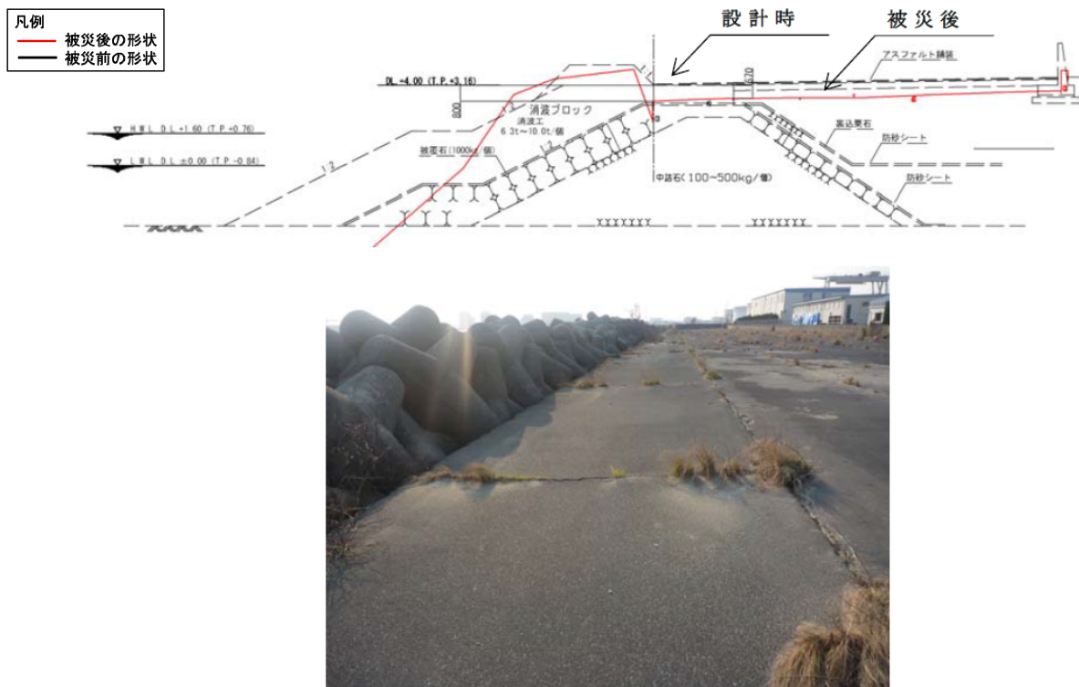
図-A. 12. 344 No. 3 仙台港区_栄地区埋立護岸 A 工区の断面図 (被災後)
