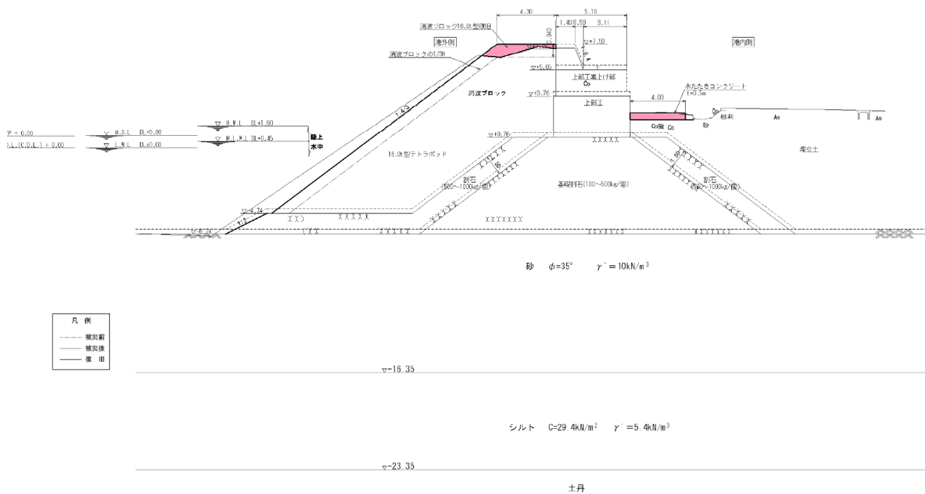
図-A. 12. 142 No. 19 仙台港区_南防波護岸の断面図 (被災後)
