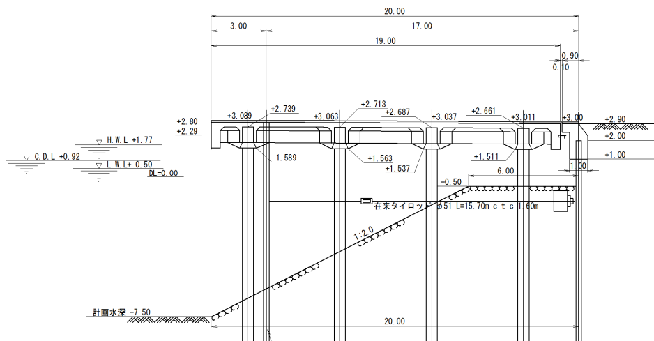
図-A.12.286 No. 17 塩釜港区_中ふ頭東側さん橋の断面図（被災前）
