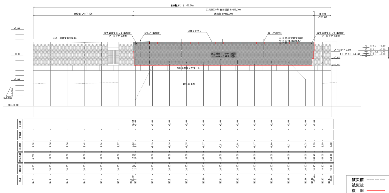
図-A.12.153 No.22 仙台港区_雷神護岸 I の縦断面図 (被災後)
