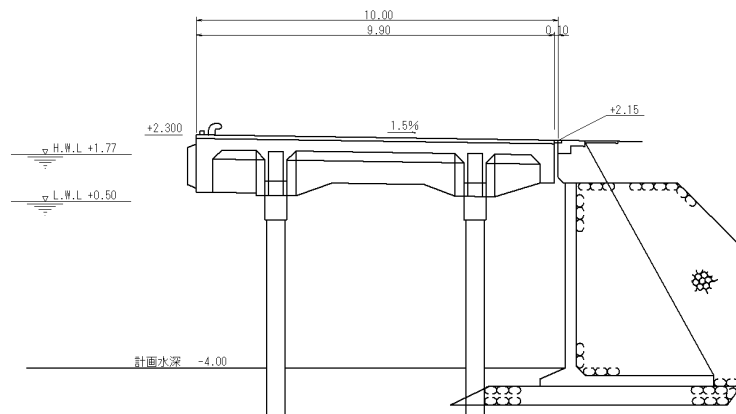
図-A.12.278 No. 15 塩釜港区_中ふ頭港橋前物揚場の断面図（被災前）
