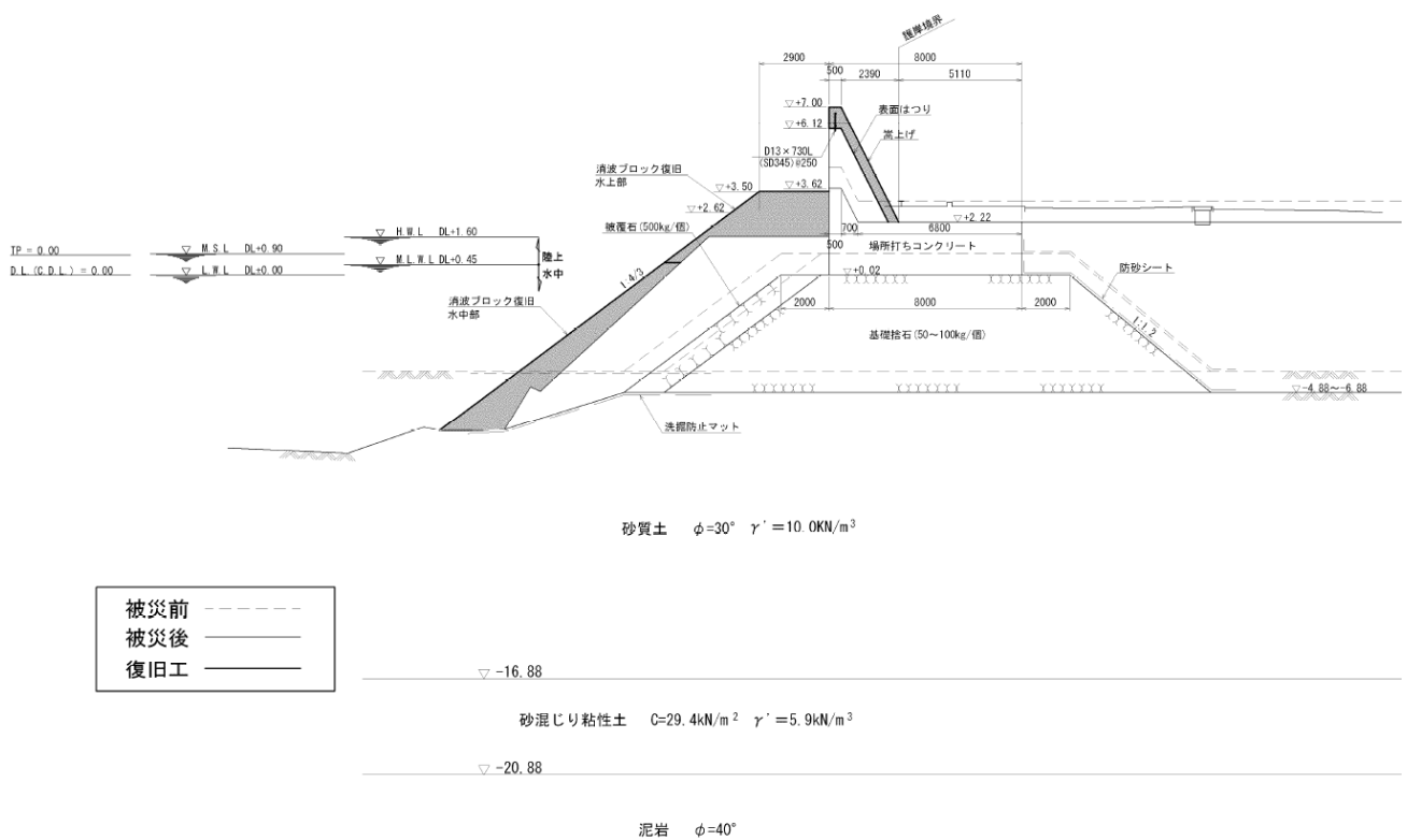
図-A. 12. 137 No. 18 仙台港区_向洋ふ頭防波護岸の断面図（復旧後）
