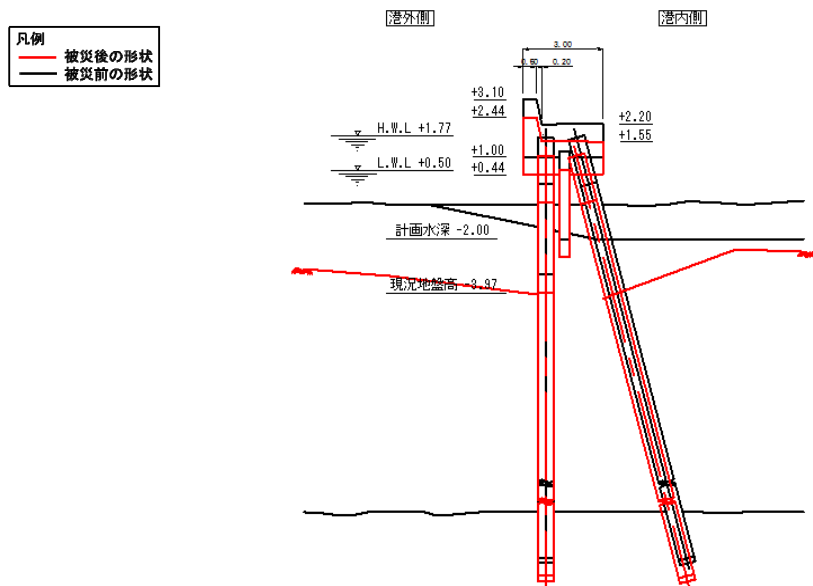
図-A.12.104 No.12 塩釜港区_東宮浜東防波堤の断面図（被災後）
