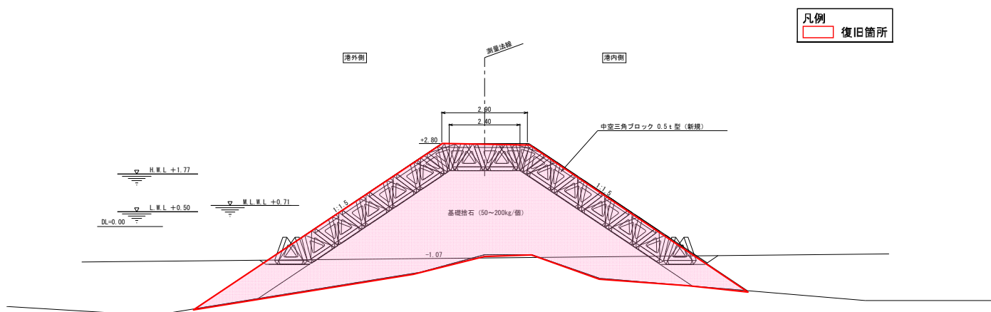
図-A. 12. 77 No. 4 塩釜港区_石浜南防波堤の B 断面図 (復旧後)
