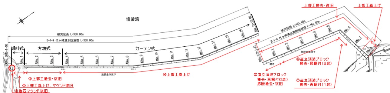
図-A.12.85 No.7 塩釜港区_代ヶ崎清水東側防波堤の平面図（復旧後）
