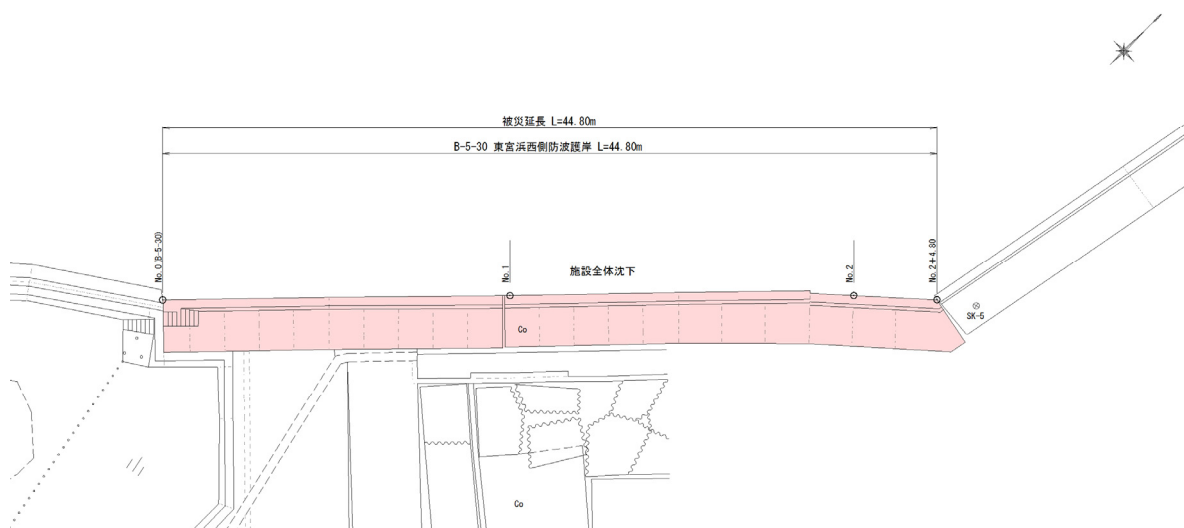
図－A.12.99 No.11 塩釜港区_東宮浜西側防波護岸の平面図（被災後）
