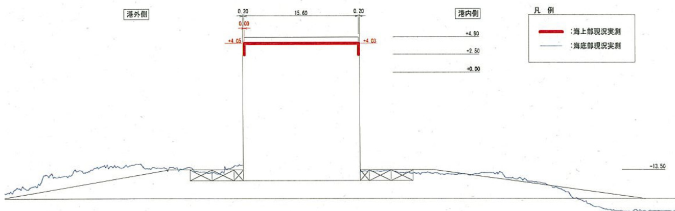
図-A.12.16 No.1 仙台港区_外港地区_北防波堤の断面図 E-E' (被災後)
