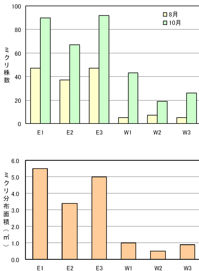
図－植物 45－2 ミクリ株数及び分布面積（平成 14 年）
