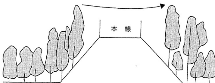
図－事例 17－3 鳥類の横断経路対策
