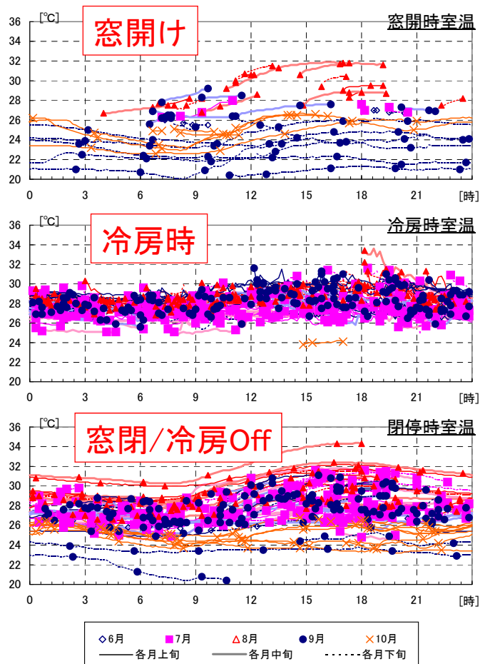
図 3.1.59 【住戸⑫LD 隣接室】各モードでの室温の推移 (2010/6/30～10/10)
