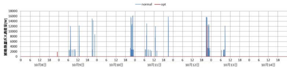
図 3.4.31 給湯負荷・排熱回収量・貯湯タンク熱量の比較(中間期)
