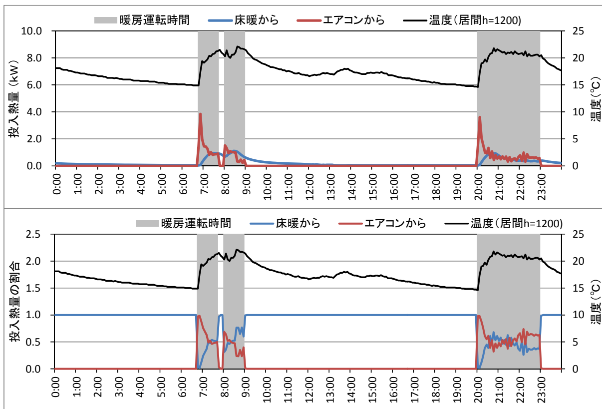
図 3.5.9 外出 床暖 (4_ON) _ AC (20) の場合の時系列変動 (2011/1/24) (上: 投入熱量の絶対値、下: 投入熱量の割合)
