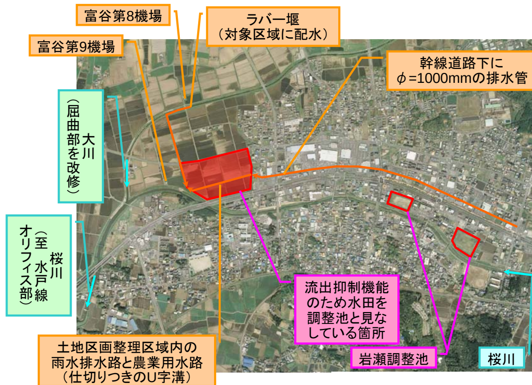
図8 岩瀬駅前土地区画整理事業における防災調整池位置図
