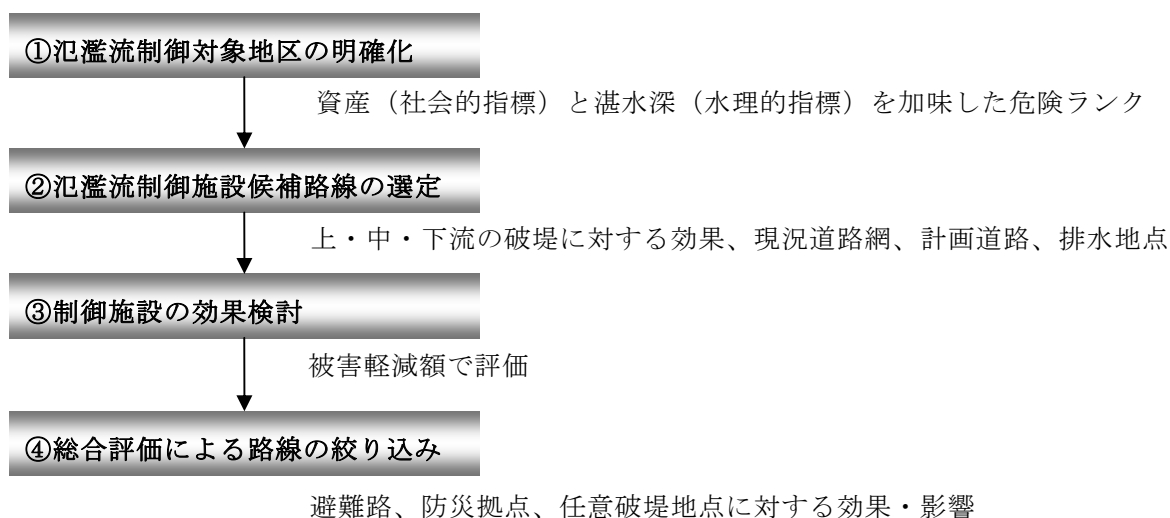
図 13 路線選定フロー
