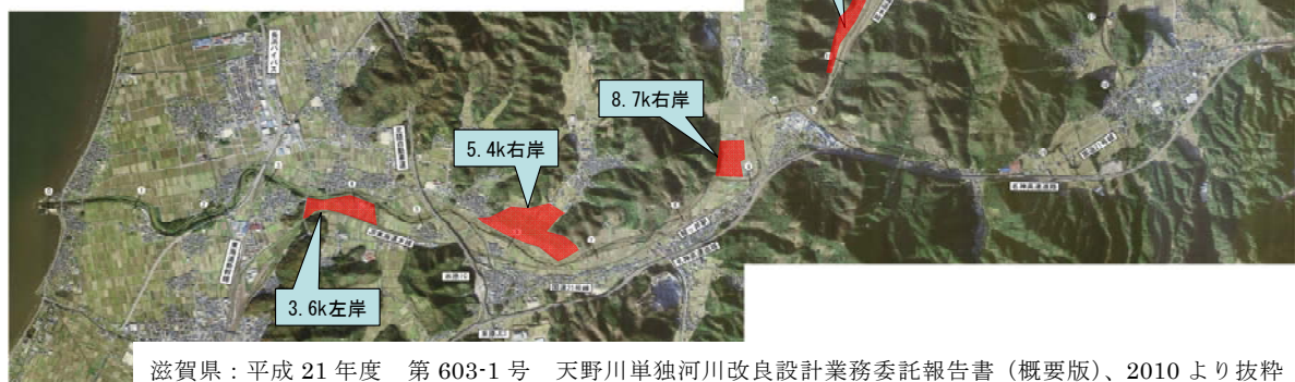
図 9 天野川流域の氾濫流制御施設の位置図
