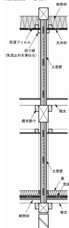
図 31 土塗壁の例
