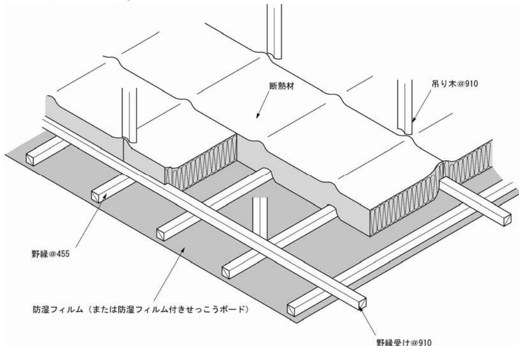
図 40 天井断熱-1
