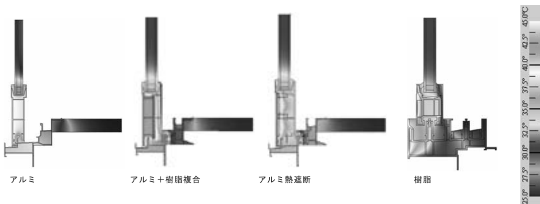
図5 各種フレーム断面における温度分布図
