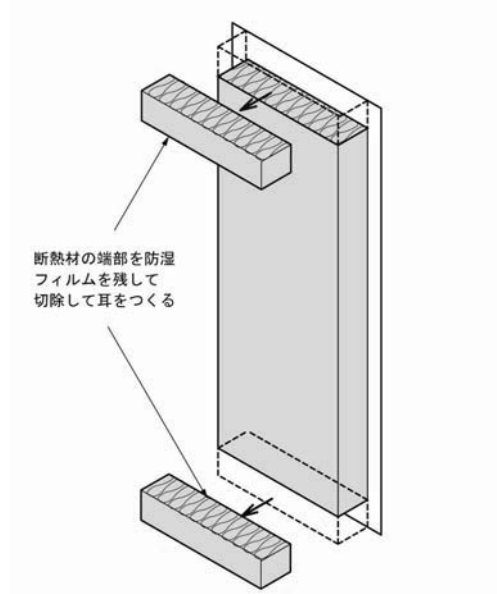
図 39 外壁断熱(耳のない断熱材の施工)
