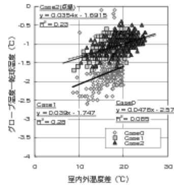
図8 グローブ温度と乾球温度の差
