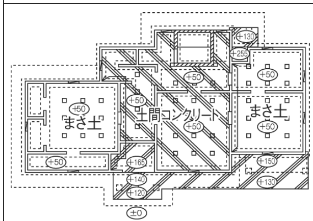
図3 基礎伏図
