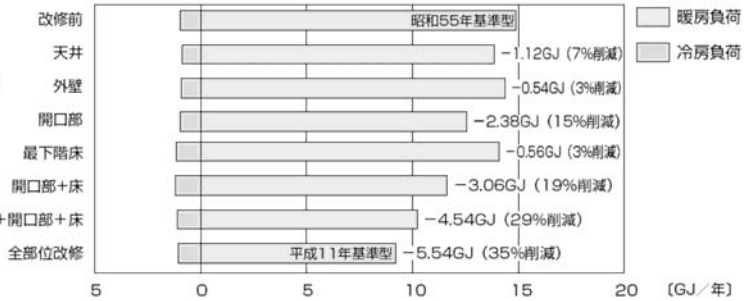
図4 断熱改修による年間の暖冷房エネルギー消費量の試算結果(1戸当たり) 改修前の1年間の暖冷房エネルギー消費量と、改修後の暖冷房エネルギー消費量及び消費量削減率を示した。全部位改修を行った場合には、35%の削減効果が見込まれる。 (図4はAE-CADを用いて、年間の暖冷房エネルギー消費量をシミュレーションした結果)
