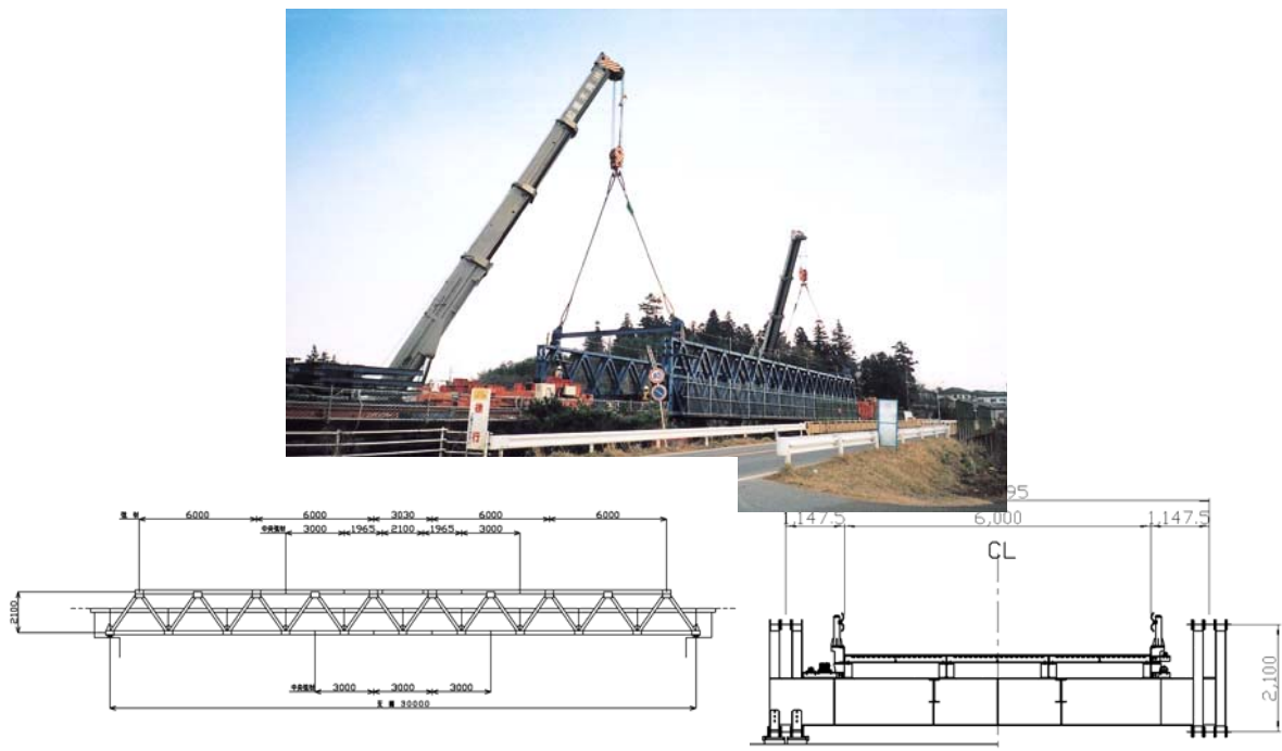
図 4-33 トラス橋の事例
