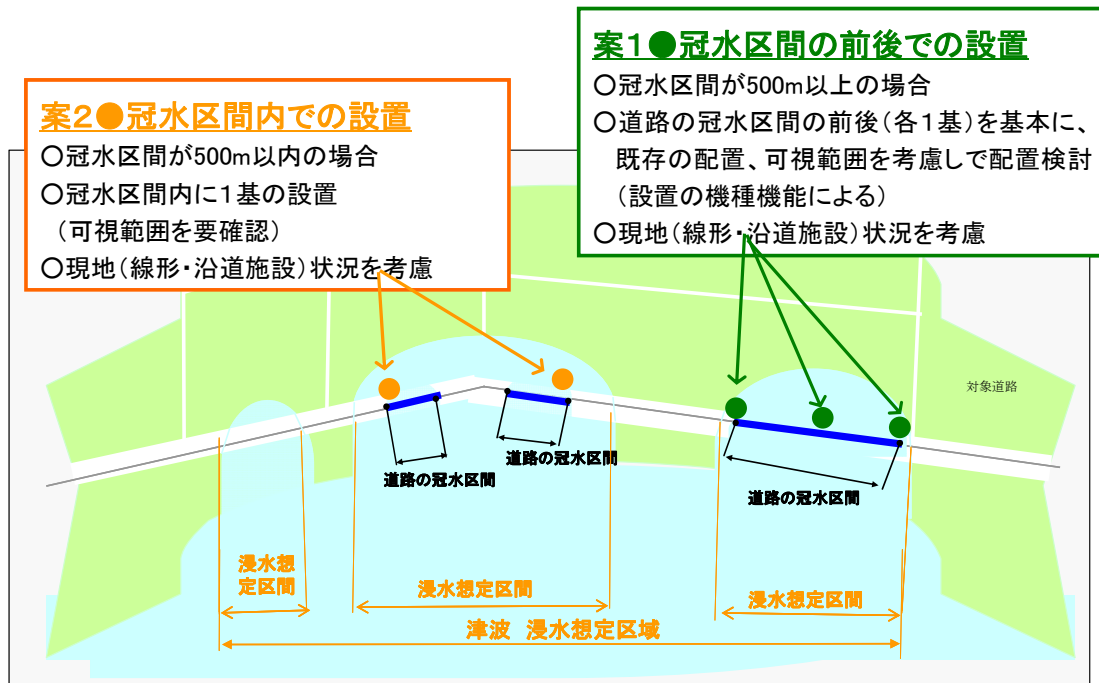
図 4-6 CCTV の配置計画例
