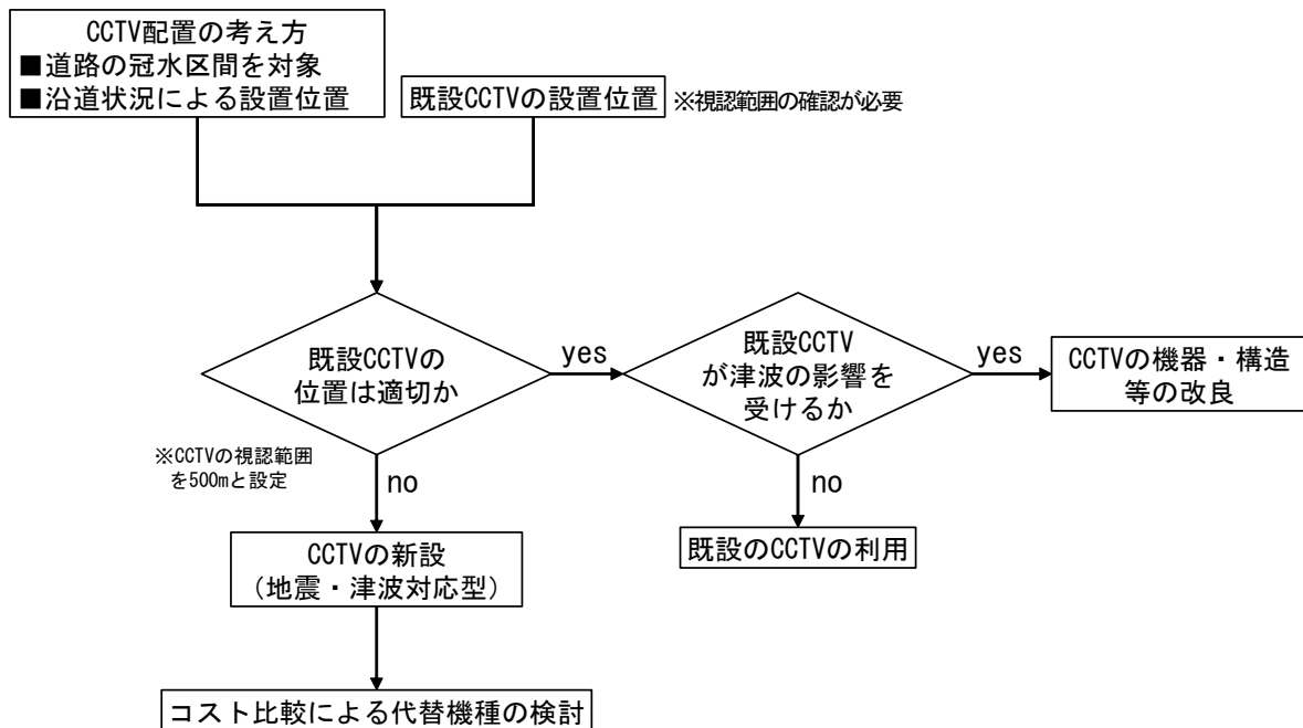
図 4-4 CCTV 設置計画検討フロー
