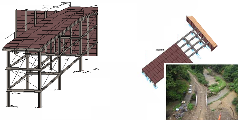
図 4-31 仮栈橋を採用する場合
