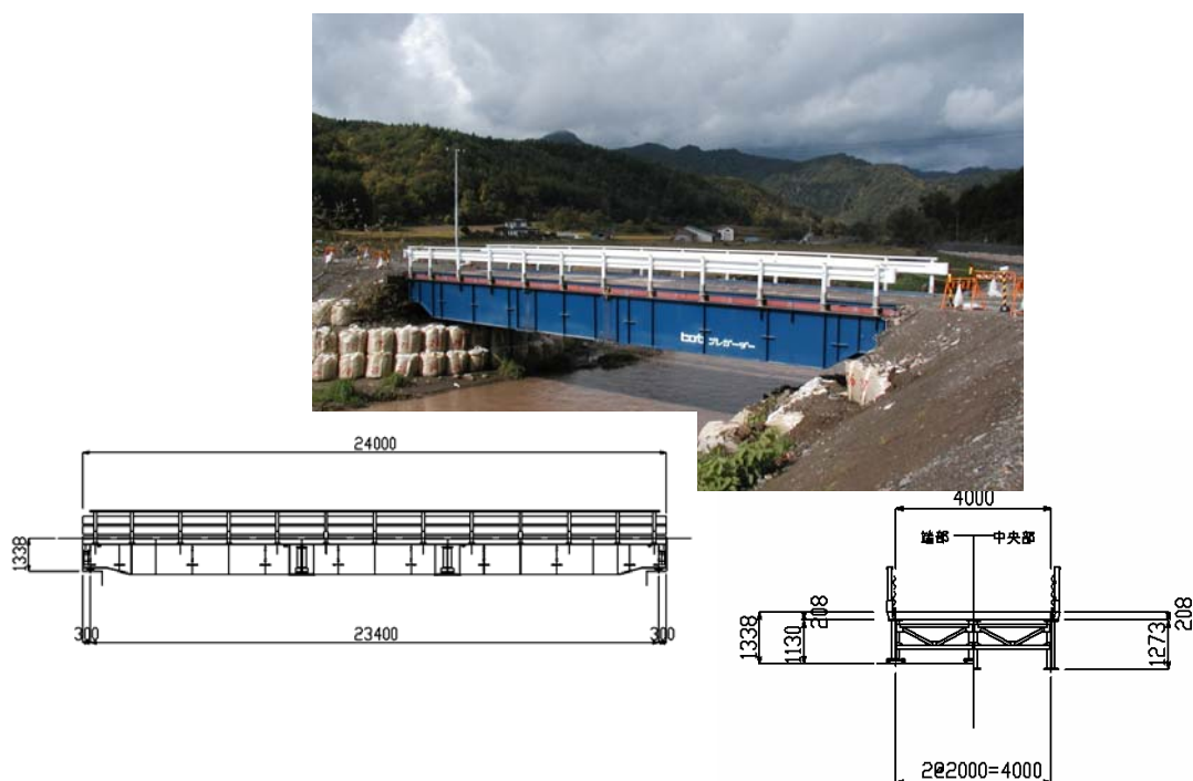
図 4-32 単純梁鉸桁橋の事例
