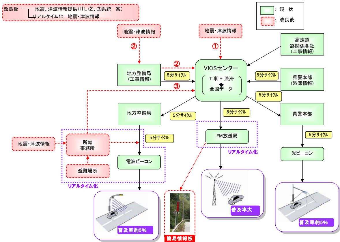
図4-13 VICSを活用した情報提供イメージ（地震・津波情報提供）
