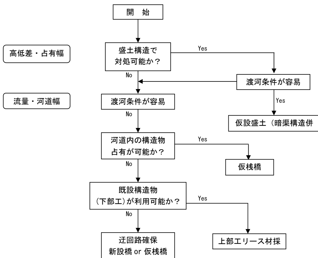
図 4-29 復旧方法選定フロー
