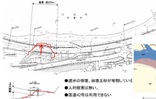
図 道路崩壊
