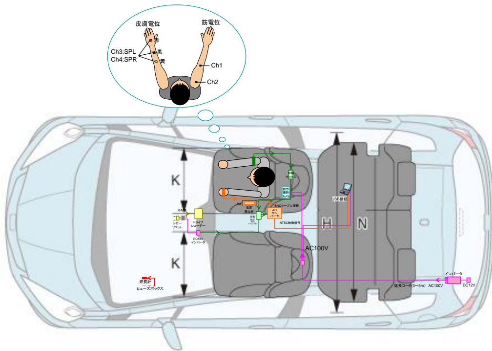
図 8.4-6 機器配置図
