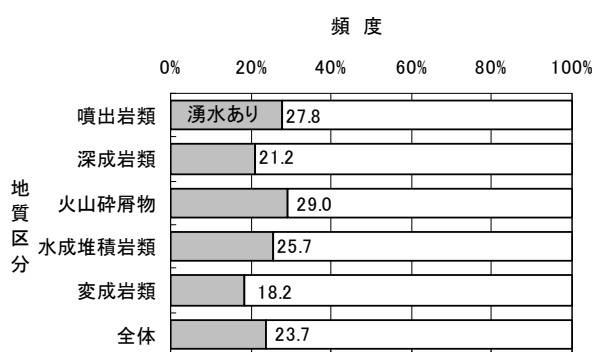
図-13.1.2 地質区分毎の湧水と崩壊の関係（昭和47年～平成11年）（降雨によるもの）
