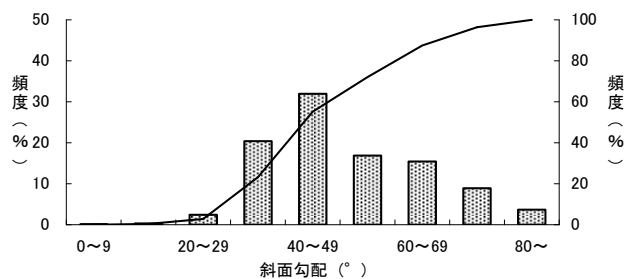
図-11.3.2 斜面の傾斜頻度分布（昭和47年～平成11年） （降雨によるもの）
