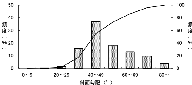
図-11.3.4 斜面の傾斜頻度分布（昭和47年～平成11年） （融雪によるもの）
