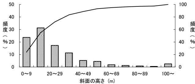
図-11.1.1 斜面の高さ（昭和47年～平成19年）
