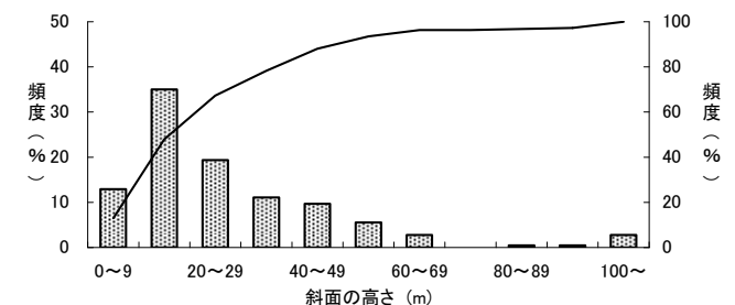
図-11.1.4 斜面の高さ（昭和47年～平成19年） （融雪によるもの）
