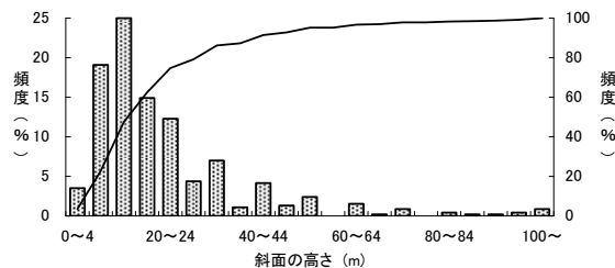
図-11.2.3 斜面の高さ（昭和47年～平成19年） （地震によるもの）
