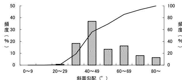
図-11.3.3 斜面の傾斜頻度分布（昭和47年～平成11年） （地震によるもの）
