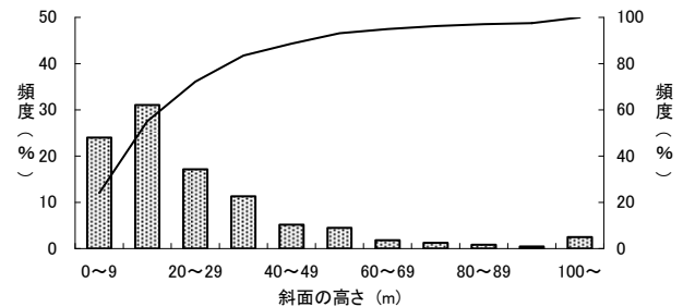
図-11.1.2 斜面の高さ（昭和47年～平成19年） （降雨によるもの）
