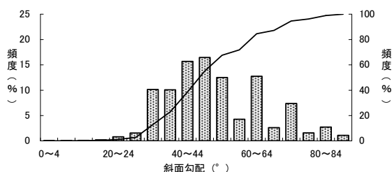
図-11.4.1 斜面の傾斜頻度分布（昭和47年～平成11年）
