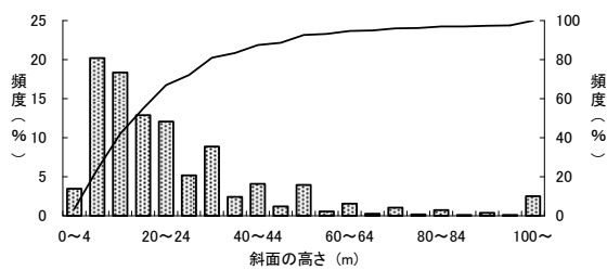
図-11.2.1 斜面の高さ（昭和47年～平成19年）
