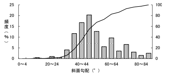
図-11.4.4 斜面の傾斜頻度分布（昭和47年～平成11年） （融雪によるもの）
