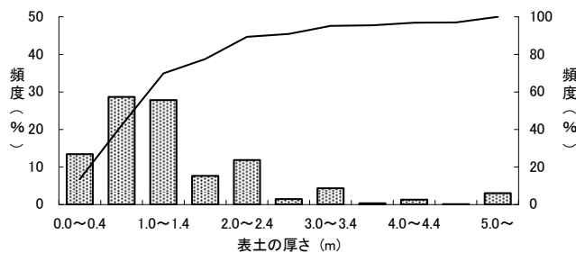
図-11.5.1 表土の厚さ頻度分布（昭和47年～平成11年）
