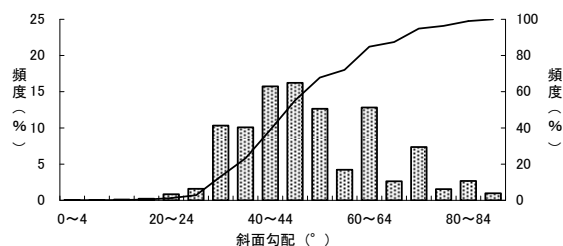
図-11.4.2 斜面の傾斜頻度分布（昭和47年～平成11年） （降雨によるもの）
