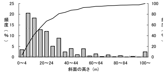
図-11.2.2 斜面の高さ（昭和47年～平成19年） （降雨によるもの）
