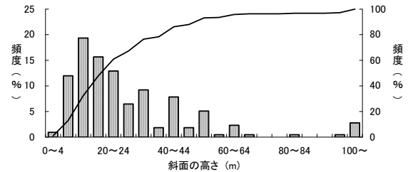
図-11.2.4 斜面の高さ（昭和47年～平成19年） （融雪によるもの）
