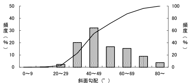
図-11.3.1 斜面の傾斜頻度分布（昭和47年～平成11年）
