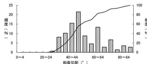
図-11.4.3 斜面の傾斜頻度分布（昭和47年～平成11年） （地震によるもの）
