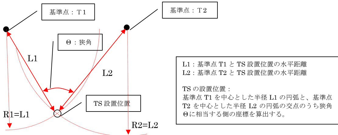
図-6 後方交会法での器械位置算出 (例)
