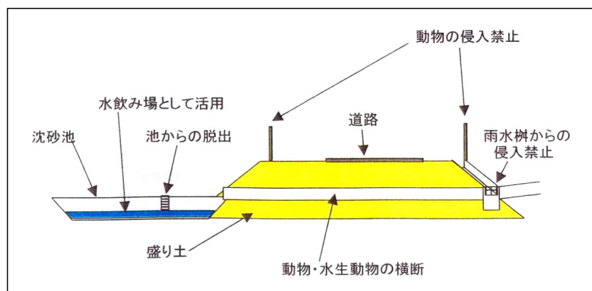
図一事例 6-2 横断路の整備の模式断面
