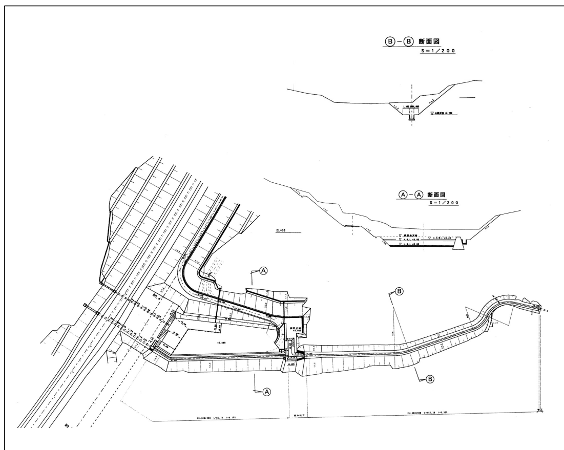
図一事例 6-5 横断路設置位置周辺の平面図
