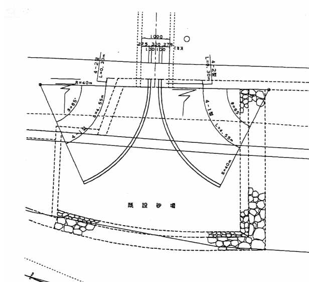
图一事例 4-3 横断路入口平面图
