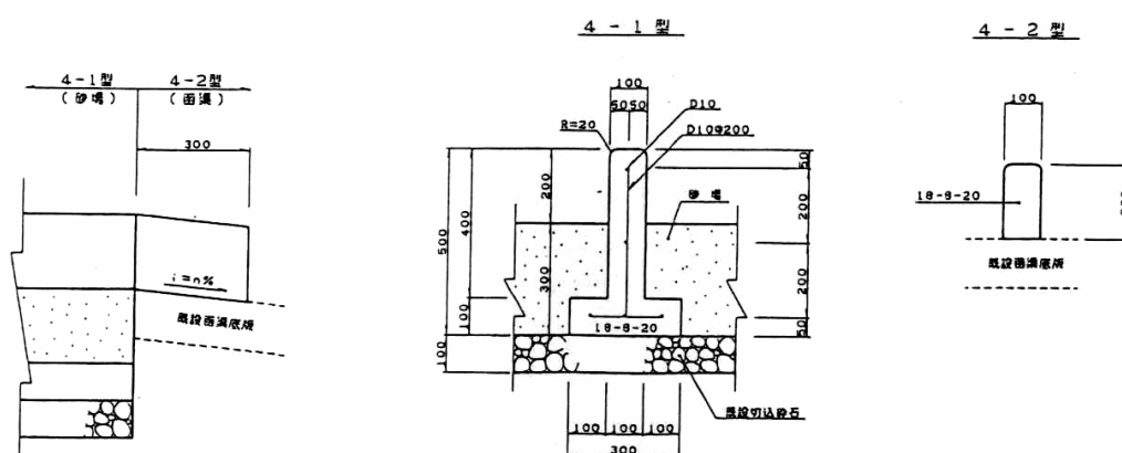
図一事例 4-4 誘導パネルの断面図
