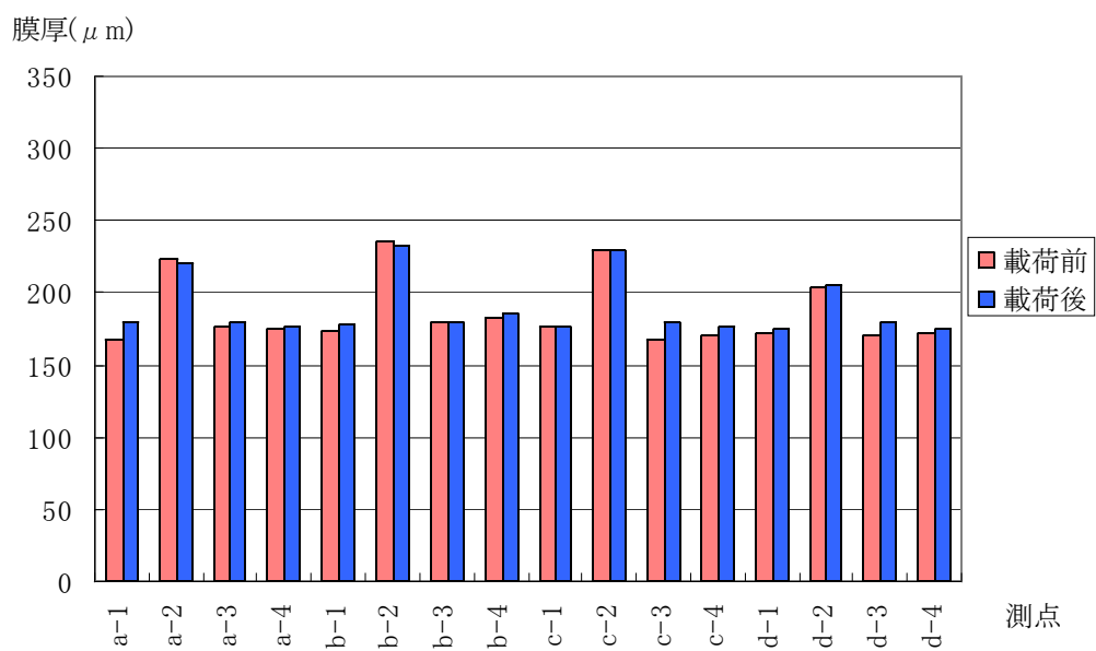
付図 4.4.90 N1 供試体の測点毎の最小値
