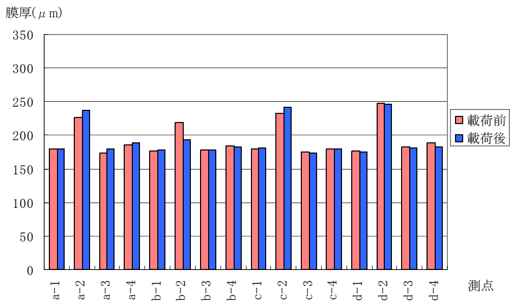
付図 4.4.88 B2 供試体の測点毎の最小値
