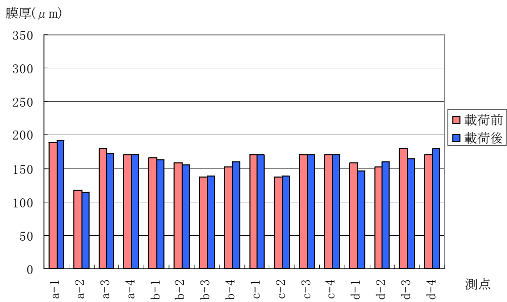
付図 4.4.87 B1 供試体の測点毎の最小値
