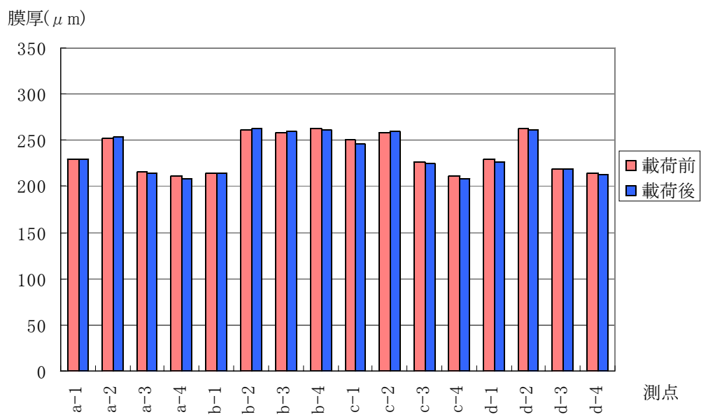
付図 4.4.82 B1 供試体の測点毎の平均値
