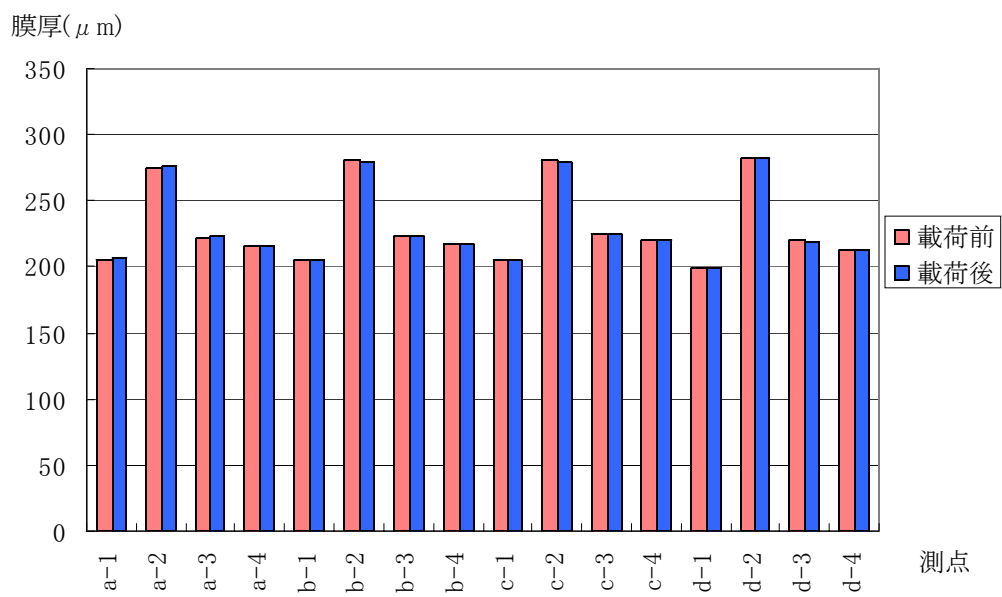
付図 4.4.84 AB1 供試体の測点毎の平均値
