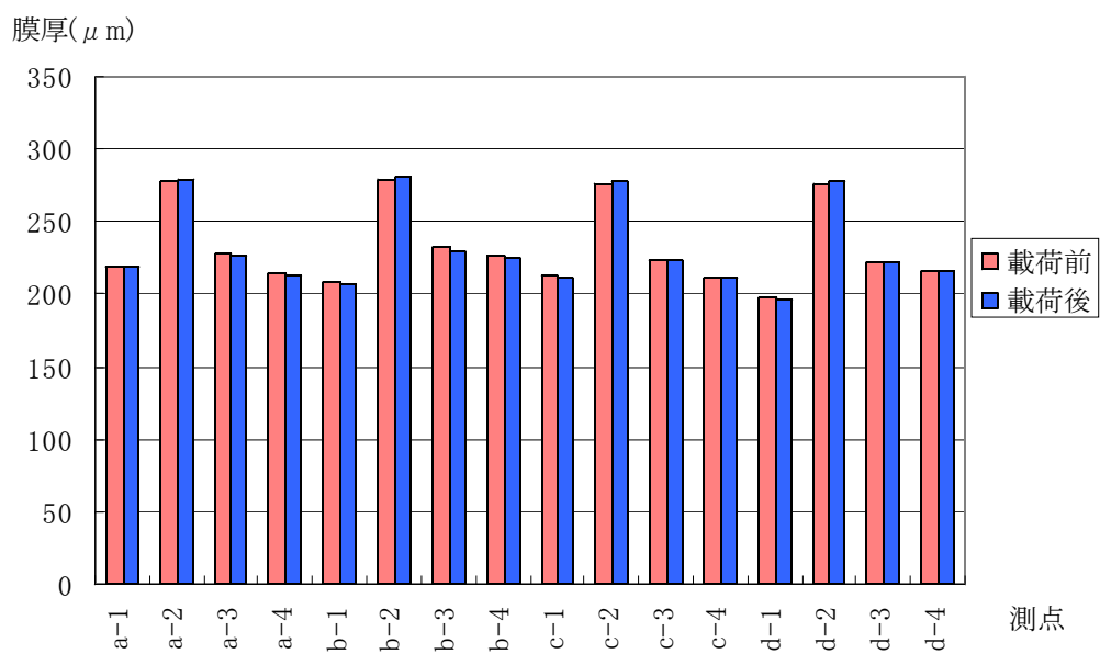
付図 4.4.85 N1 供試体の測点毎の平均値
