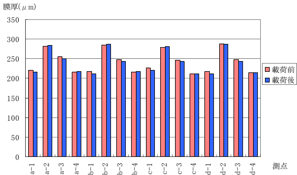
付図 4.4.81 A1 供試体の測点毎の平均値
