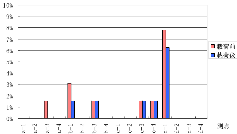
付図 4.4.93 B2 供試体の測点毎の下限值の超過確率
