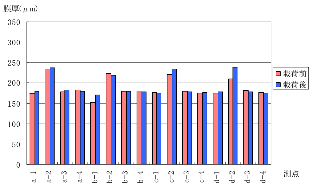
付図 4.4.89 AB1 供試体の測点毎の最小値
