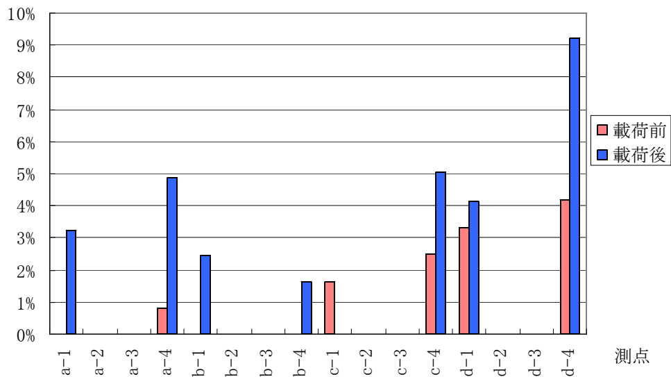
付図 4.4.91 A1 供試体の測点毎の下限値の超過確率
