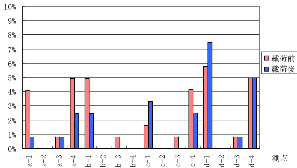
付図 4.4.95 N1 供試体の測点毎の下限值の超過確率
