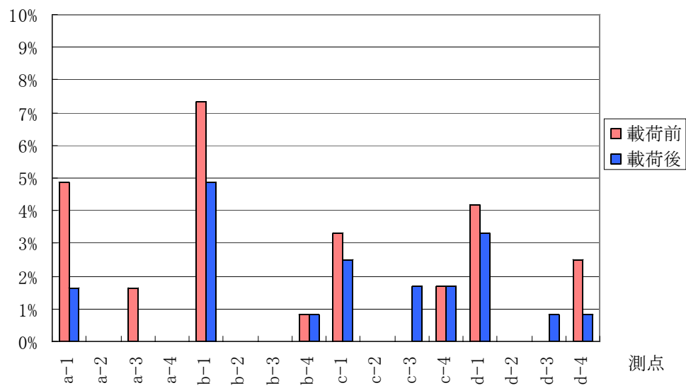
付図 4.4.94 AB1 供試体の測点毎の下限值の超過確率
