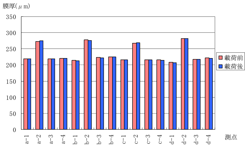
付図 4.4.83 B2 供試体の測点毎の平均値
