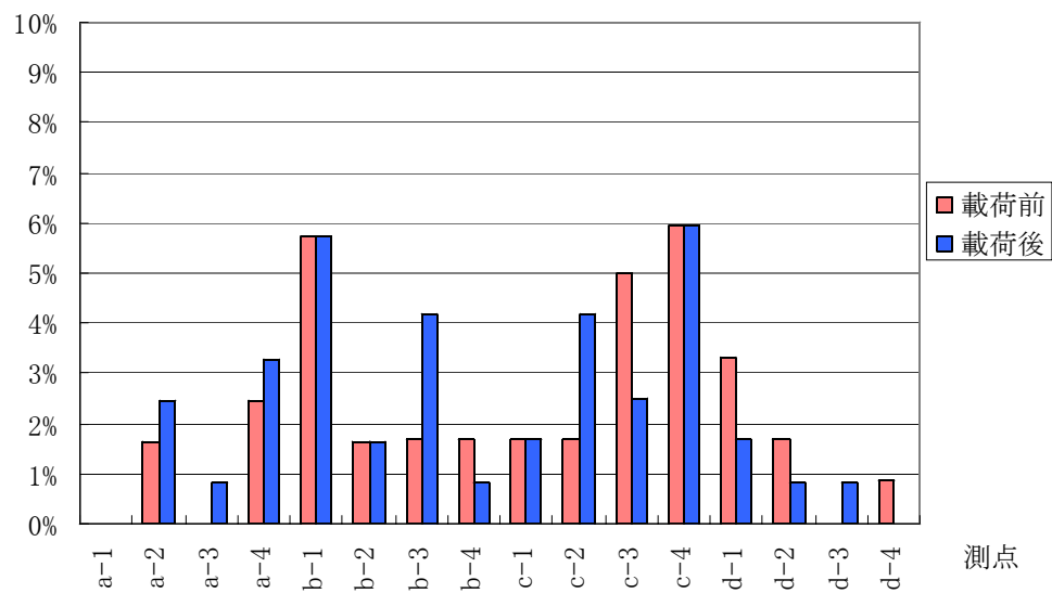
付図 4.4.92 B1 供試体の測点毎の下限值の超過確率
