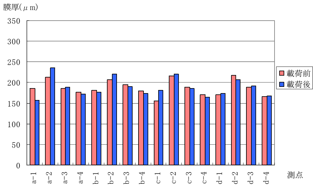
付図 4.4.86 A1 供試体の測点毎の最小値
