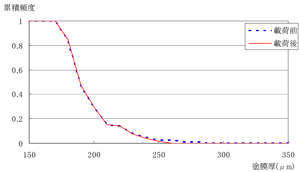
付図 4.4.77 N1 塗膜厚の累積頻度分布 (d-1)
