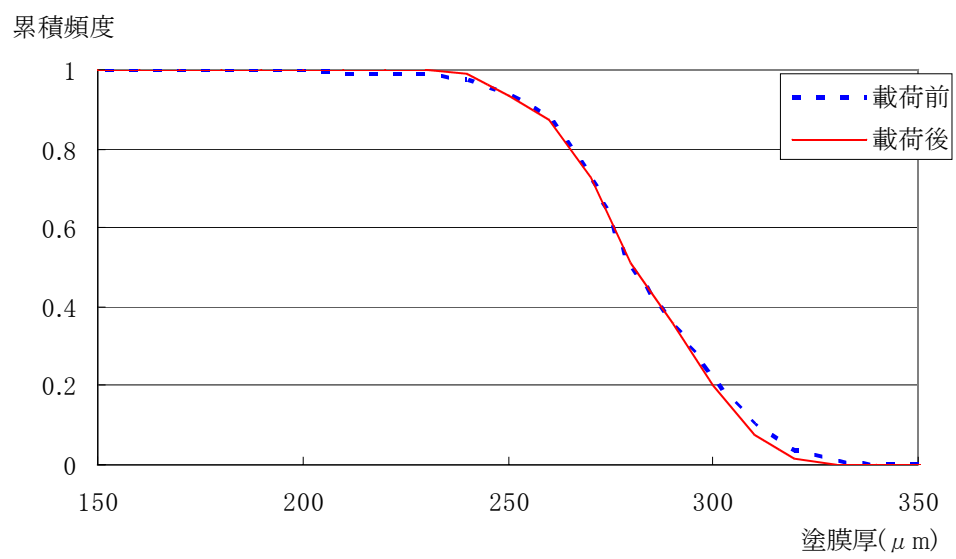
付図 4.4.62 AB1 塗膜厚の累積頻度分布 (d-2)
