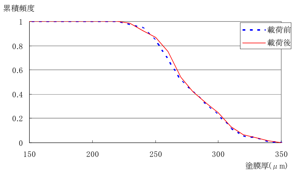
付図 4.4.66 N1 塗膜厚の累積頻度分布 (a-2)
