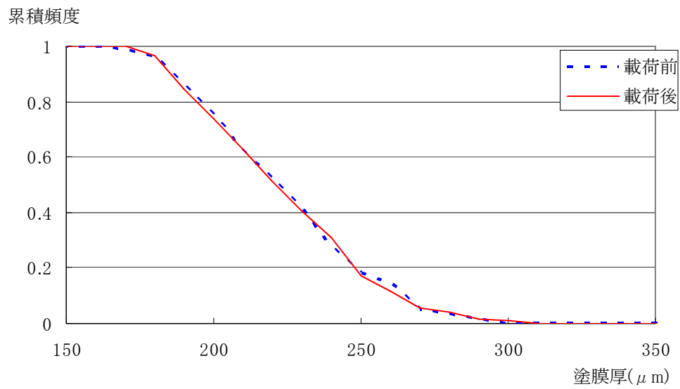
付図 4.4.75 N1 塗膜厚の累積頻度分布(c-3)
