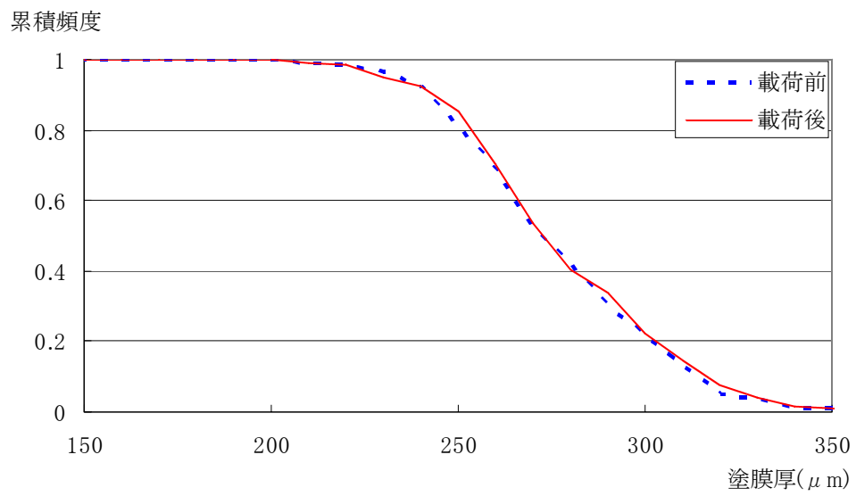
付図 4.4.78 N1 塗膜厚の累積頻度分布 (d-2)
