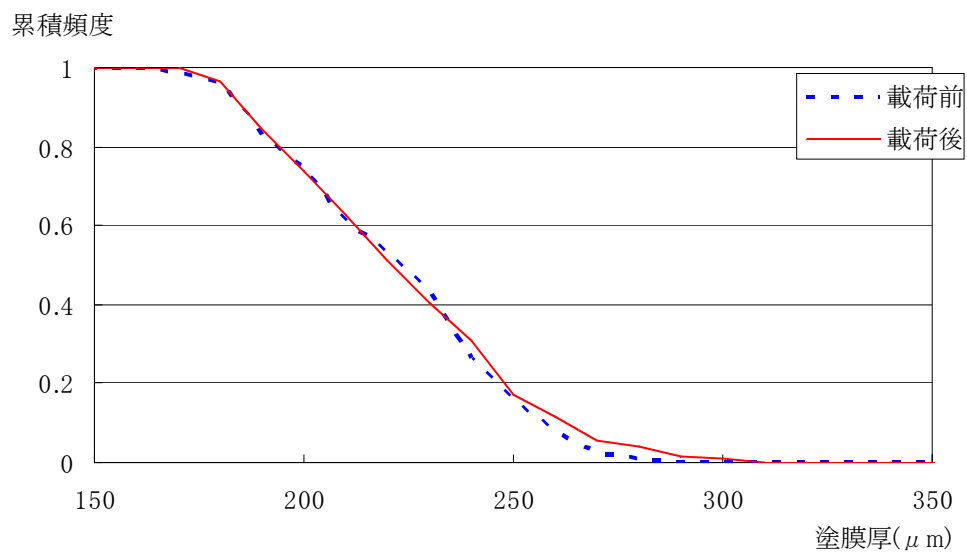
付図 4.4.79 N1 塗膜厚の累積頻度分布(d-3)
