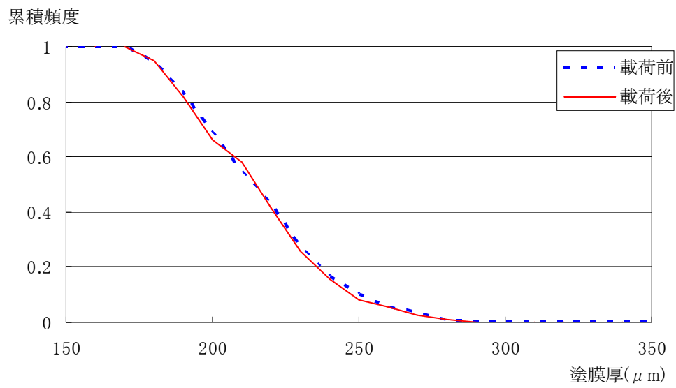
付図 4.4.80 N1 塗膜厚の累積頻度分布(d-4)
