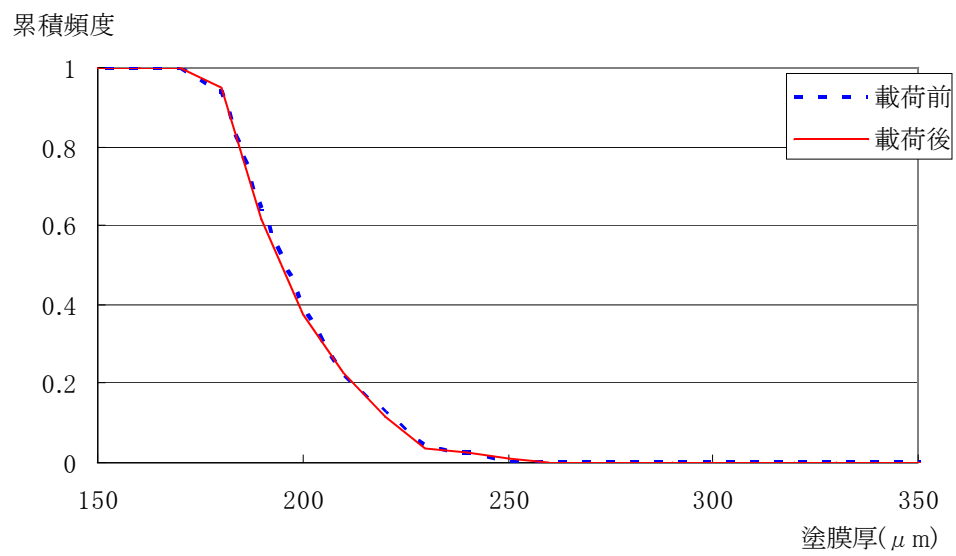
付図 4.4.61 AB1 塗膜厚の累積頻度分布 (d-1)
