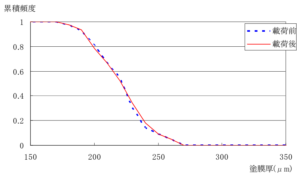
付図 4.4.60 AB1 塗膜厚の累積頻度分布 (c-4)
