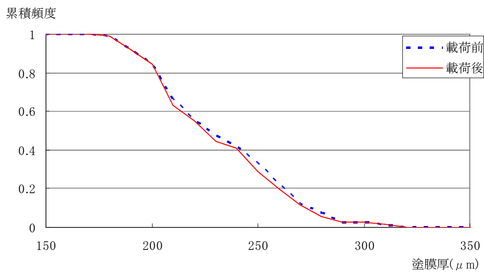
付図 4.4.71 N1 塗膜厚の累積頻度分布 (b-3)
