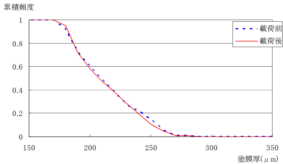
付図 4.4.68 N1 塗膜厚の累積頻度分布 (a-4)
