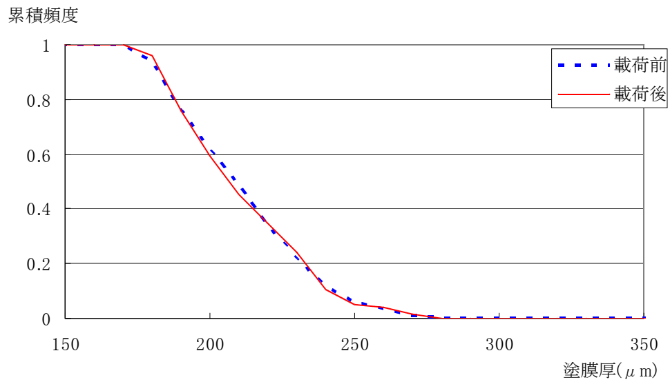
付図 4.4.76 N1 塗膜厚の累積頻度分布(c-4)
