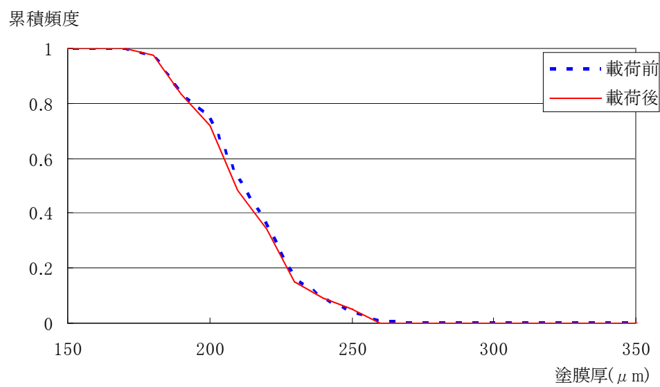
付図 4.4.64 AB1 塗膜厚の累積頻度分布 (d-4)
