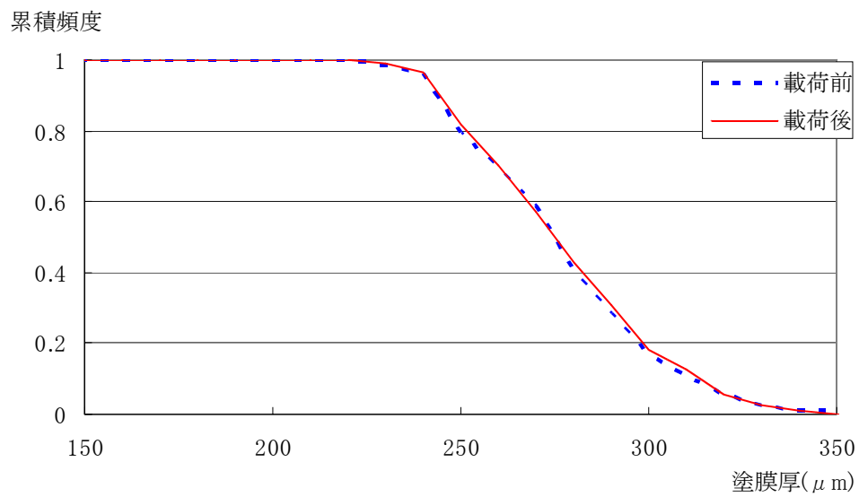
付図 4.4.74 N1 塗膜厚の累積頻度分布 (c-2)
