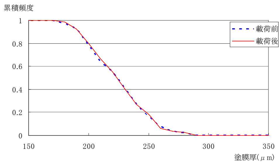
付図 4.4.59 AB1 塗膜厚の累積頻度分布 (c-3)
