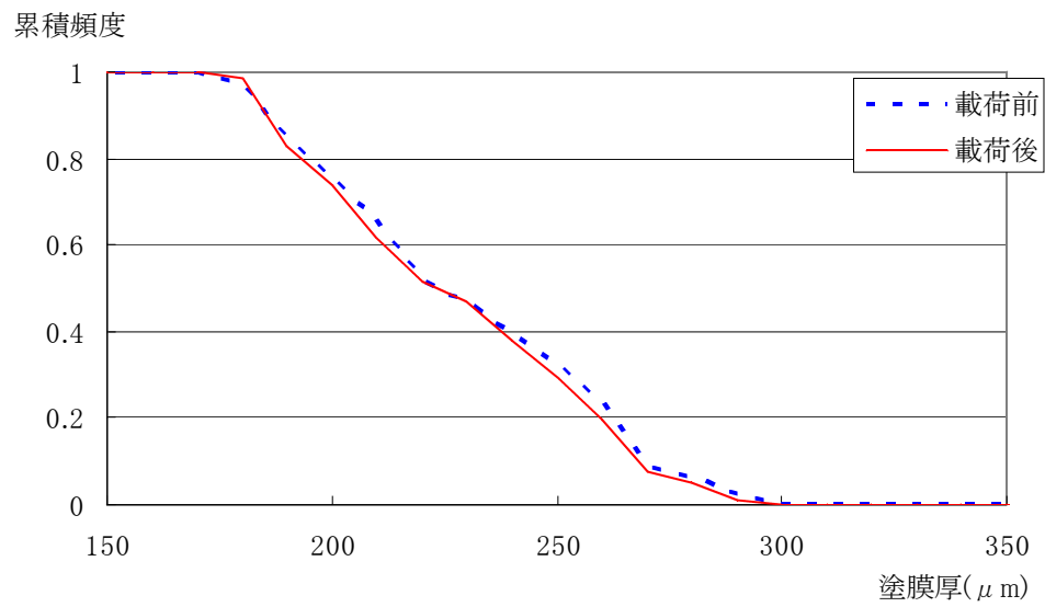
付図 4.4.67 N1 塗膜厚の累積頻度分布 (a-3)
