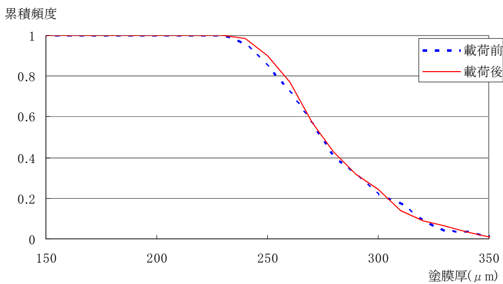
付図 4.4.70 N1 塗膜厚の累積頻度分布 (b-2)
