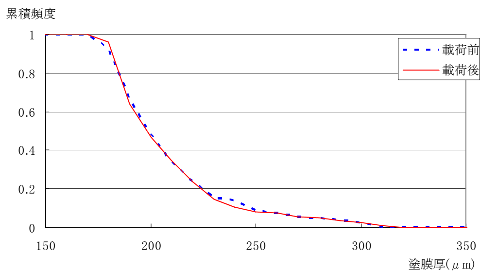
付図 4.4.69 N1 塗膜厚の累積頻度分布 (b-1)
