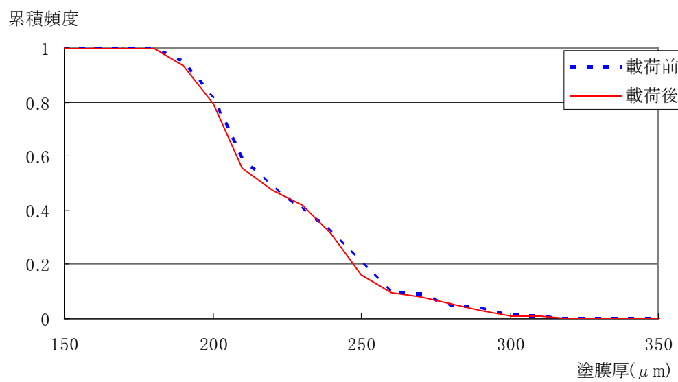
付図 4.4.72 N1 塗膜厚の累積頻度分布 (b-4)
