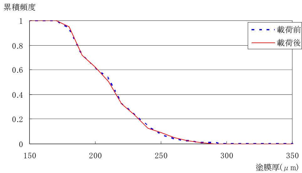
付図 4.4.73 N1 塗膜厚の累積頻度分布 (c-1)
