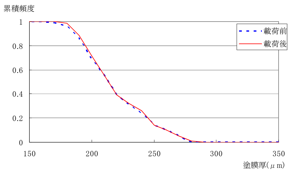
付図 4.4.65 N1 塗膜厚の累積頻度分布 (a-1)
