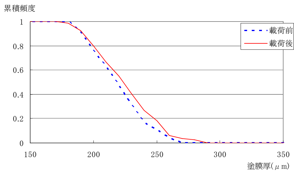
付図 4.4.63 AB1 塗膜厚の累積頻度分布 (d-3)
