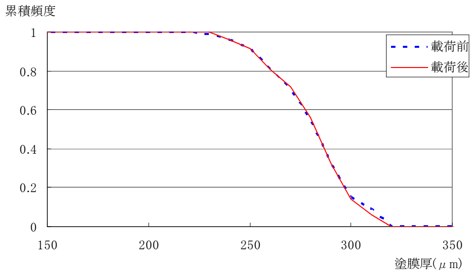
付図 4.4.58 AB1 塗膜厚の累積頻度分布 (c-2)
