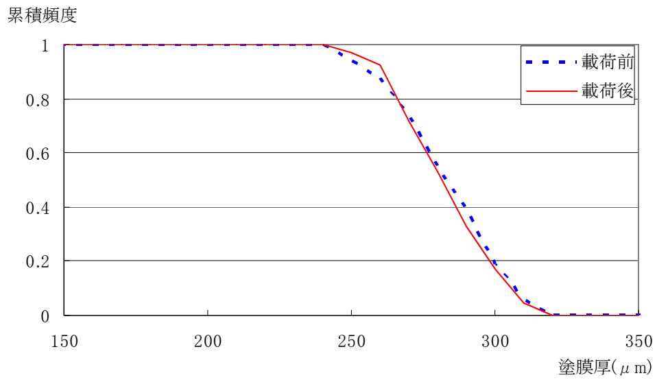
付図 4.4.46 B2 塗膜厚の累積頻度分布 (d-2)
