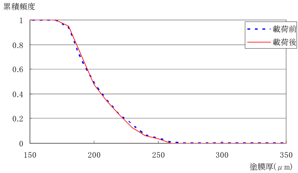
付図 4.4.57 AB1 塗膜厚の累積頻度分布 (c-1)
