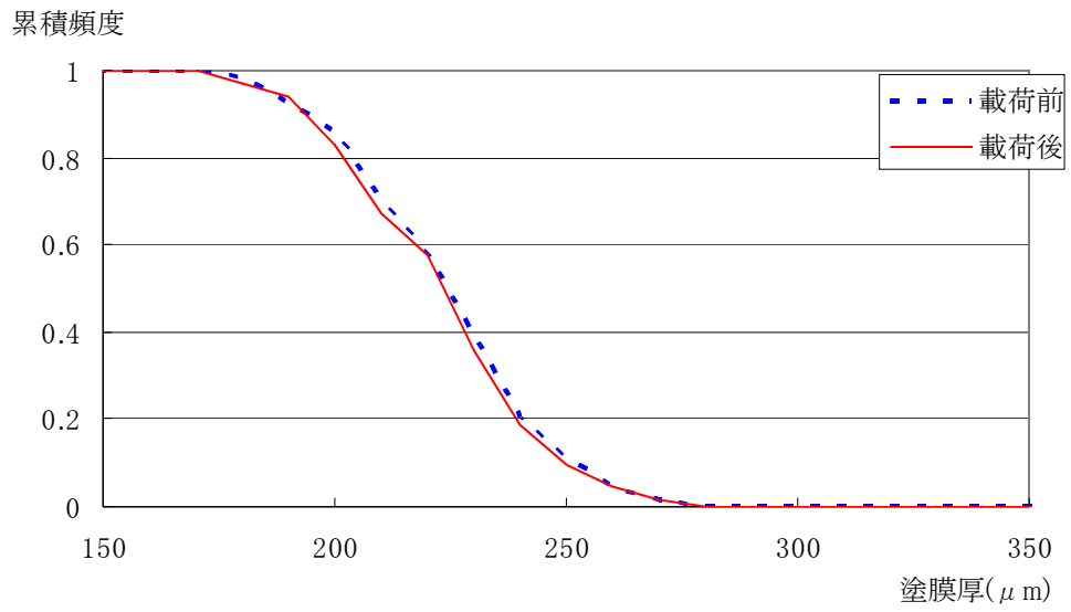
付図 4.4.39 B2 塗膜厚の累積頻度分布 (b-3)
