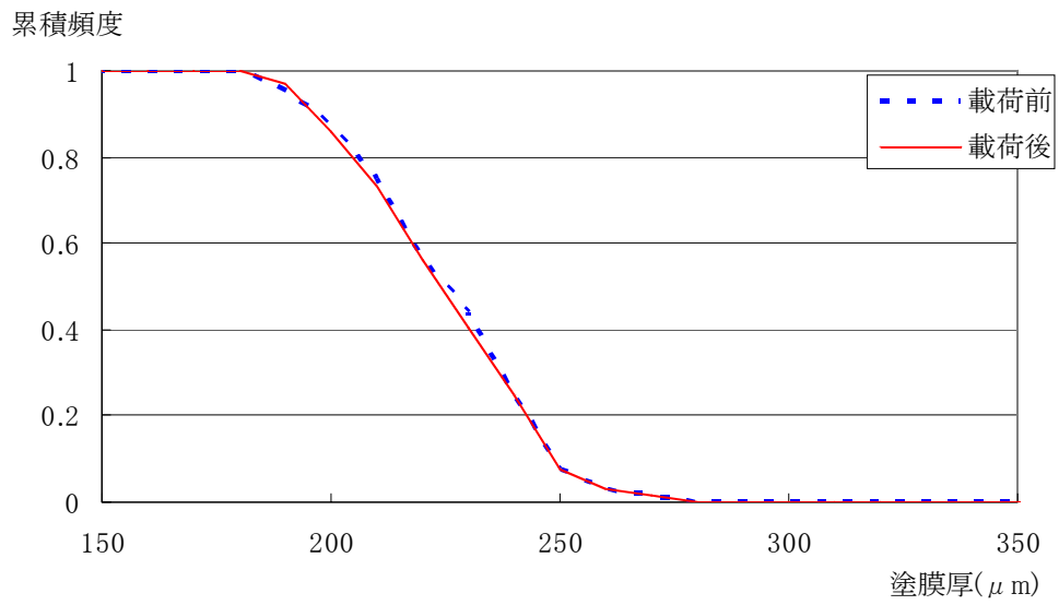
付図 4.4.40 B2 塗膜厚の累積頻度分布 (b-4)
