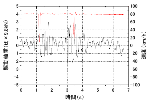
(a) 動的軸重波形 (ケース 1)
