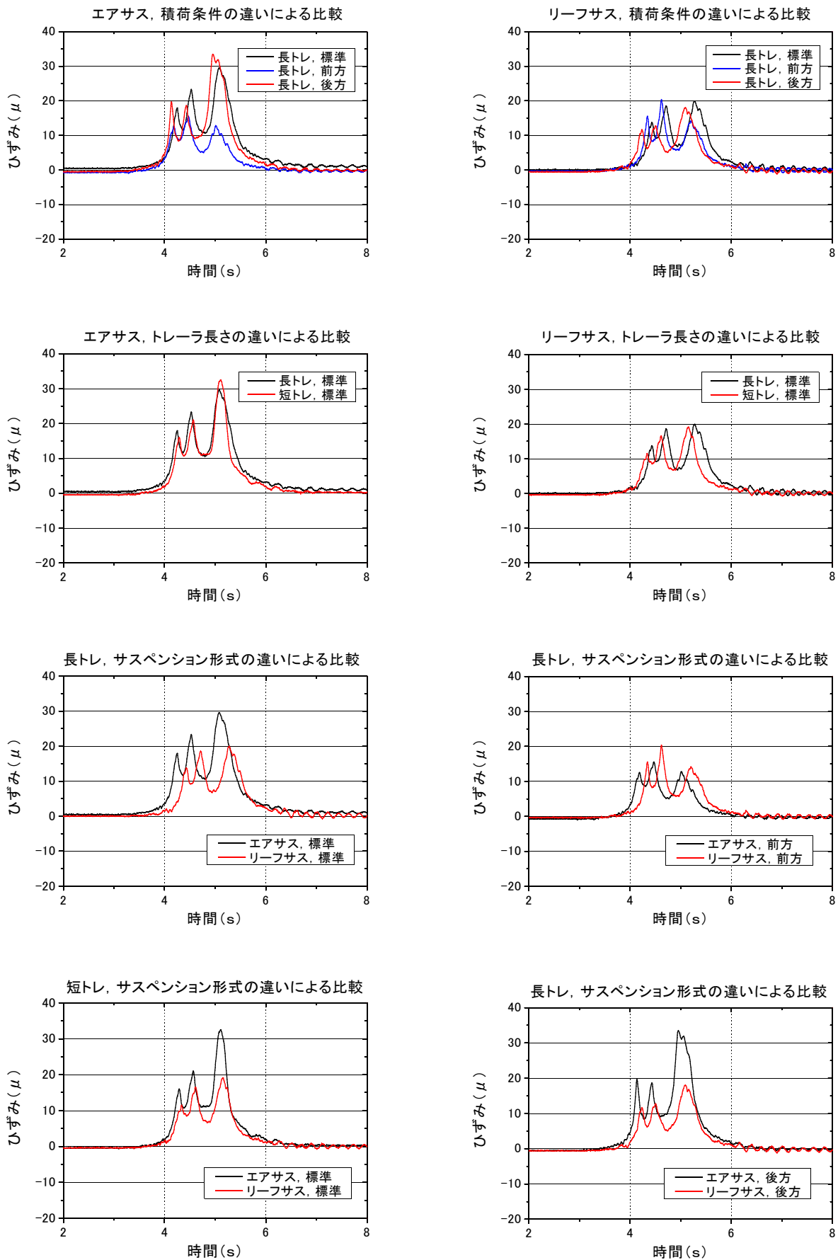
図-2.6.6 床版ひずみ (中央部・橋軸直角方向) での比較
