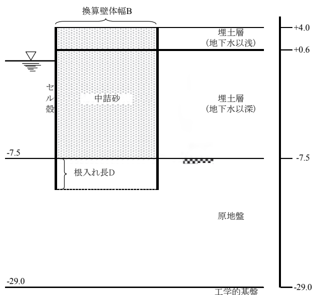
図-5 検討断面模式図
