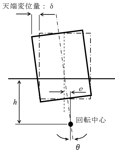
図-2 セルの回転中心
