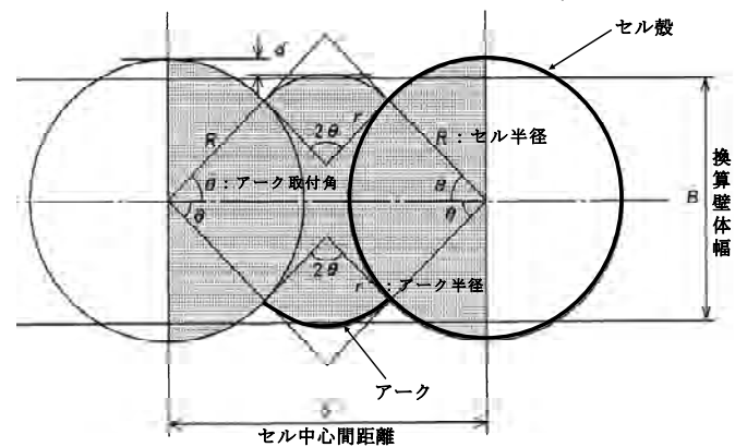
図-3 セルの面積と換算壁体幅
