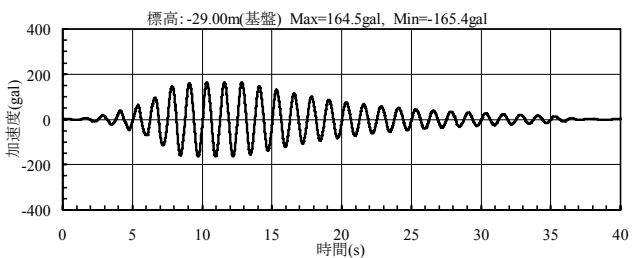
図- 14 応答加速度時刻歴 (D=4.0m)
