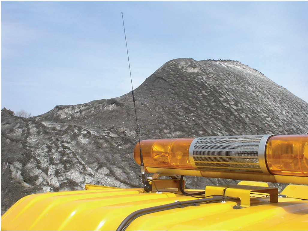
図 5-8 薬剤散布車への位置特定機器の設置状況（FM アンテナ）
