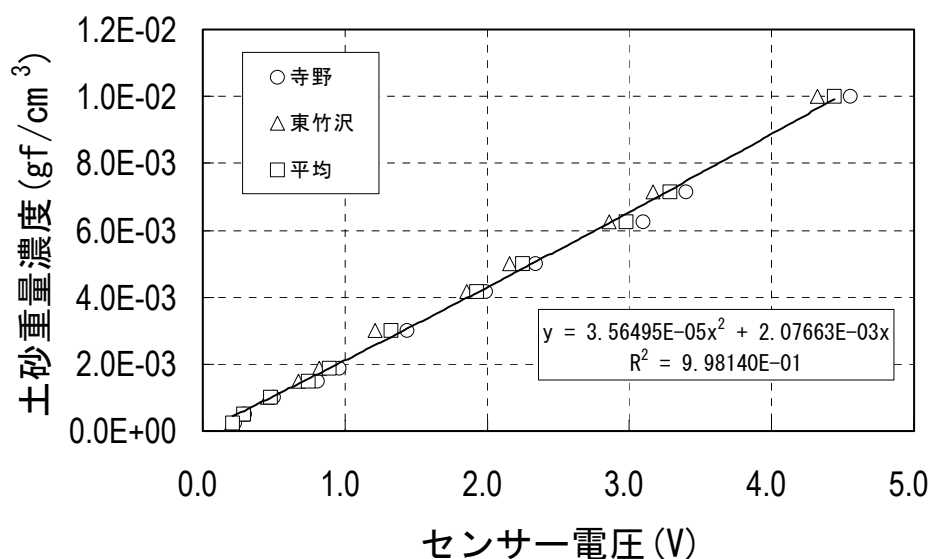
図-参3. 1 電圧 (V) - 土砂重量濃度 (gf/cm³) の関係図
