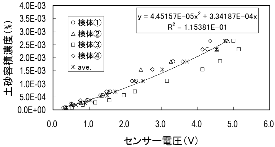
図一参 1. 2. 2 電圧 (V) - 土砂容積濃度 (%) の関係図
