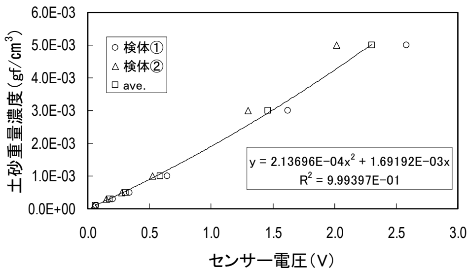
図一参 1. 1. 1 電圧 (V) - 土砂重量濃度 (gf/cm 3 ) の関係図
