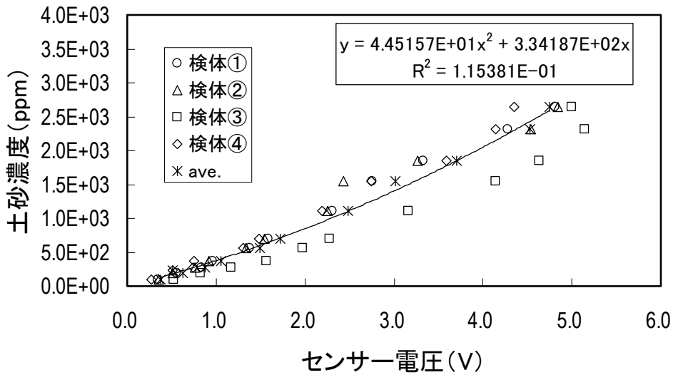
図一参 1. 2. 3 電圧 - 土砂濃度 (ppm) の関係図
