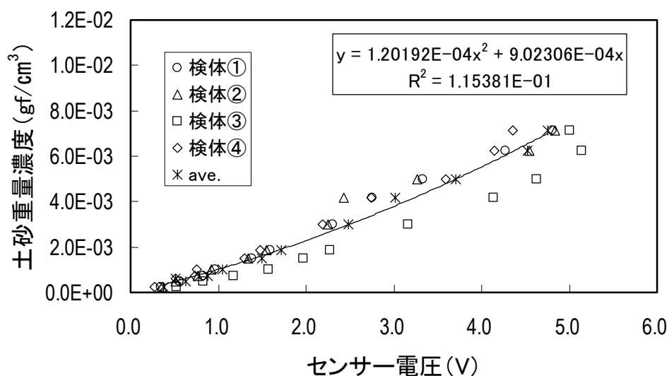
図一参 1. 2. 1 電圧 (V) - 土砂重量濃度 (gf/cm³) の関係図
