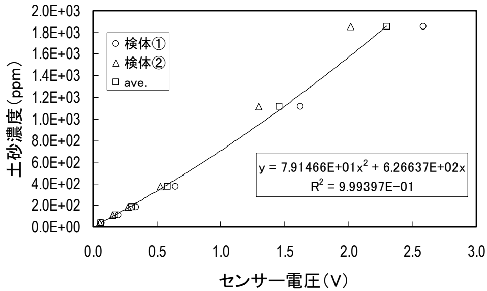
図一参 1. 1. 3 電圧－土砂濃度 (ppm) の関係図
