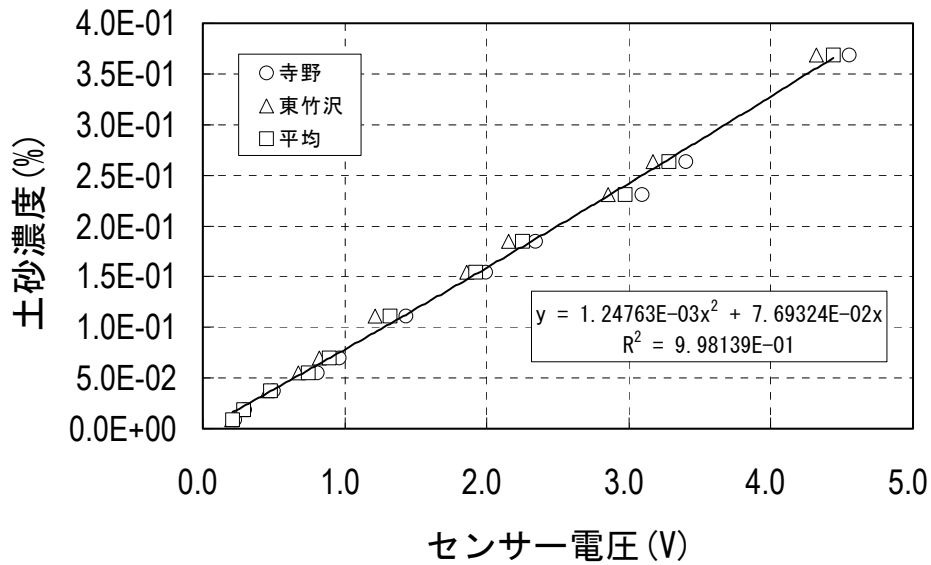
図-参3. 2 電圧 (V) - 土砂容積濃度 (%) の関係図
