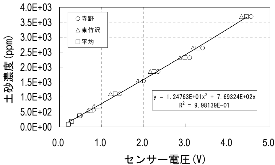
図-参3. 3 電圧-土砂濃度 (ppm) の関係図
