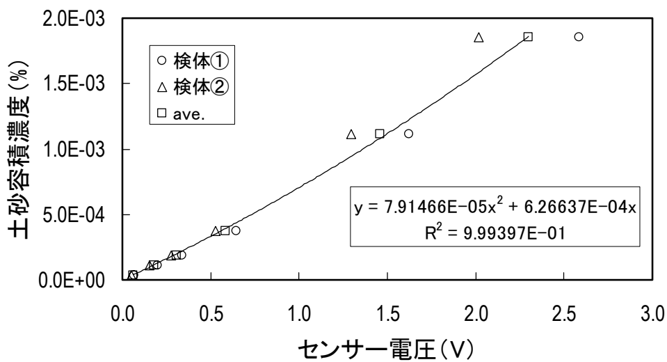
図一参 1. 1. 2 電圧 (V) - 土砂容積濃度 (%) の関係図
