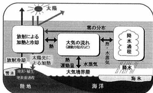
図-1 大気現象の物理素過程
