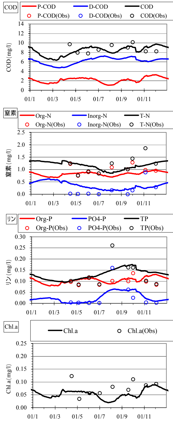
図- 4.3.1.10(3) 湖沼水質 計算結果と実測値の比較(BOX5、BOX6 : 2001 年)
