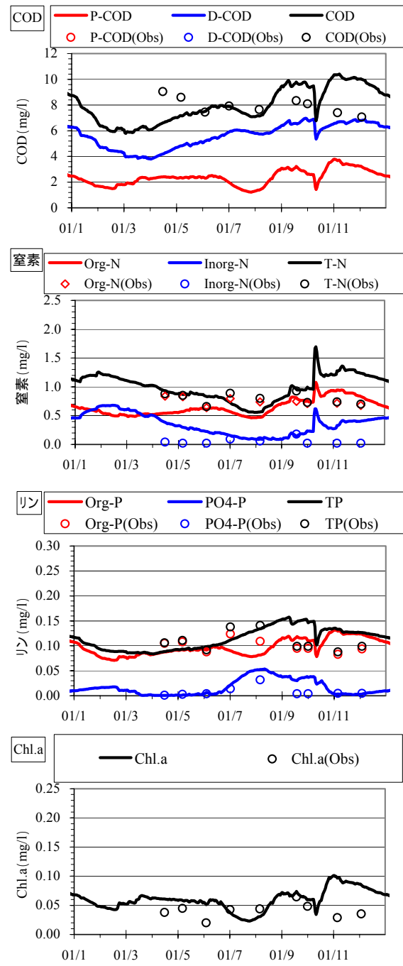
図- 4.3.1.10(2) 湖沼水質 計算結果と実測値の比較(BOX3、BOX4 : 2001 年)
