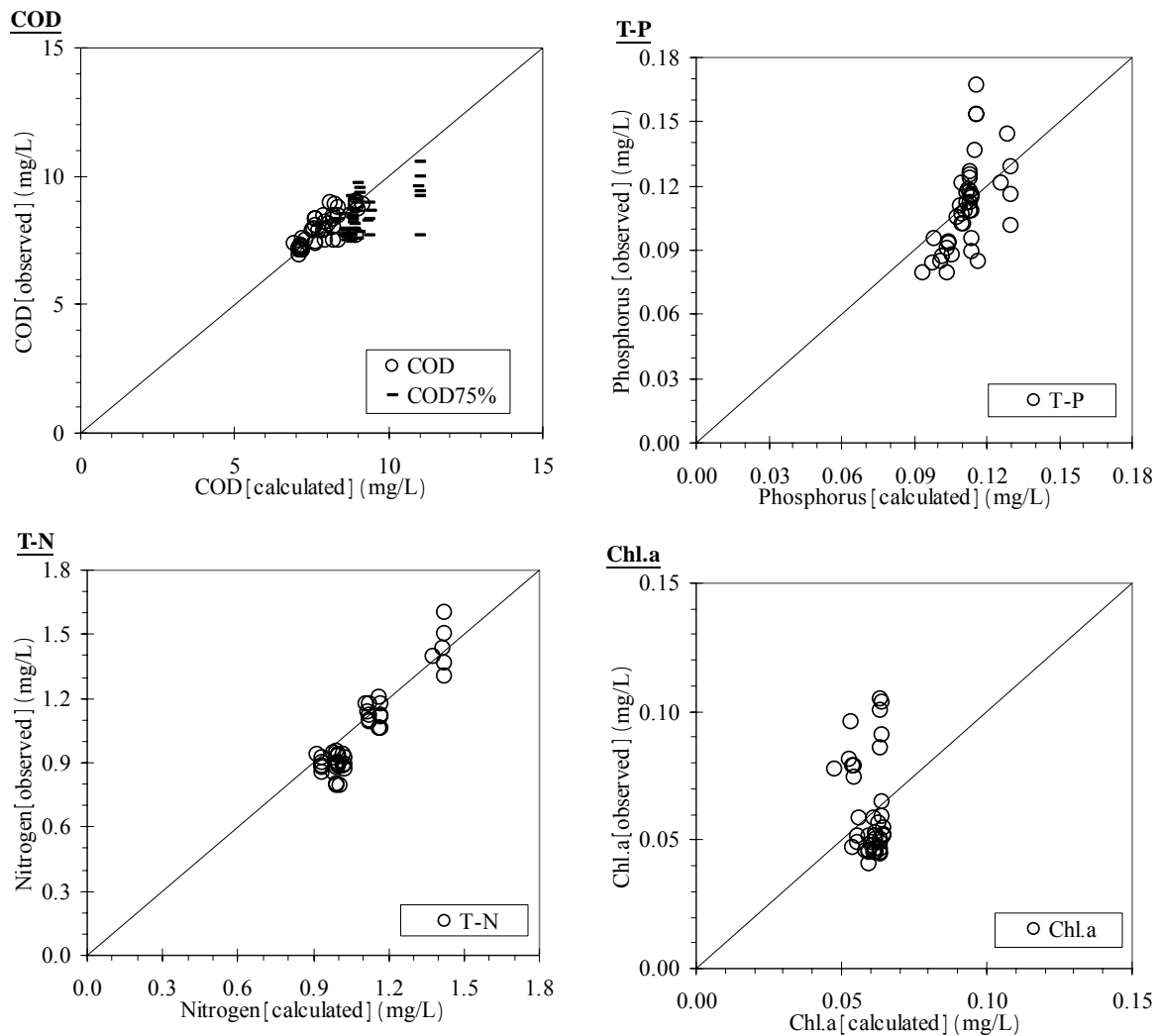
図- 4.3.1.9 湖沼水質年平均値の計算結果と実測値の比較(2001 年)(COD は 75%値も)
