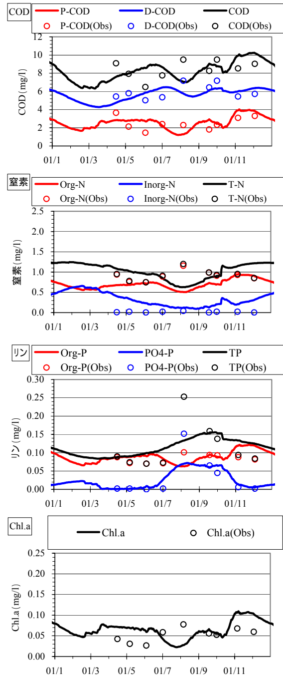
図- 4.3.1.10(3) 湖沼水質 計算結果と実測値の比較(BOX5、BOX6 : 2001 年)
