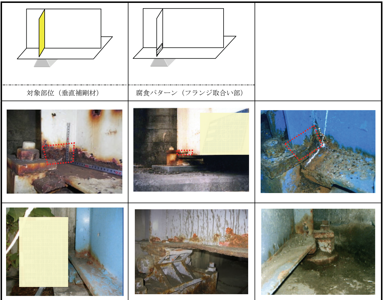
図-3.10(1) 腐食事例（支点上垂直補剛材）
