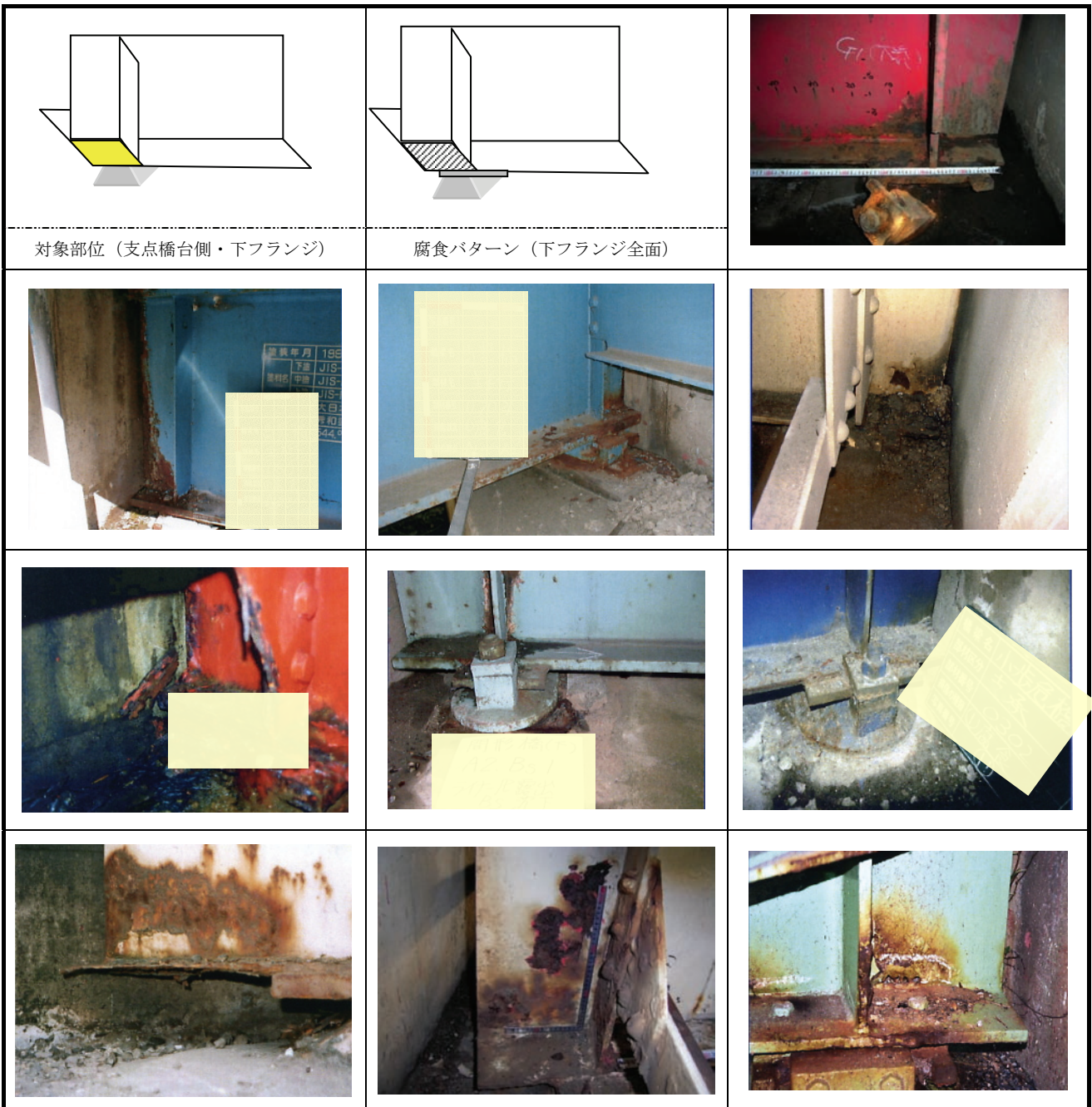
図-3.8 (1) 腐食事例 (支点橋台側・下フランジ)
