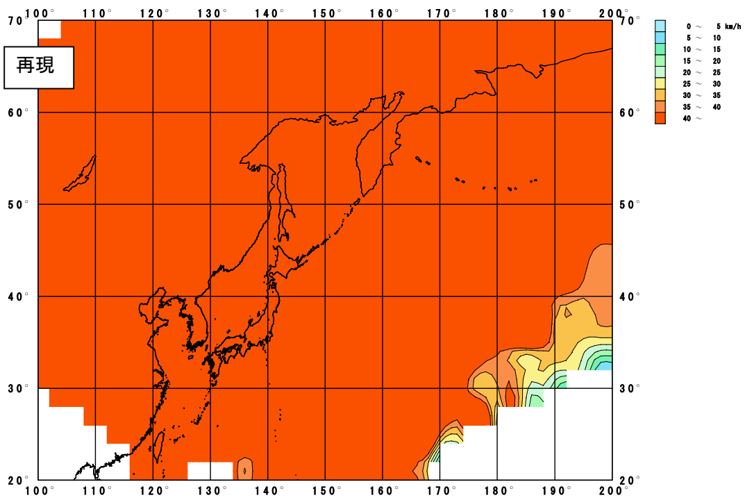
図-52 低気圧の移動速度の標準偏差(上:実測, 下:再現)
