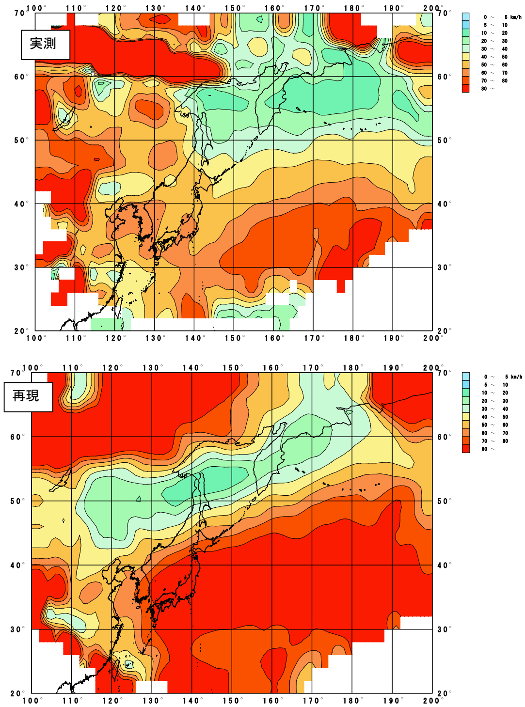
図-49 低気圧の移動速度の平均値(上:実測, 下:再現)
