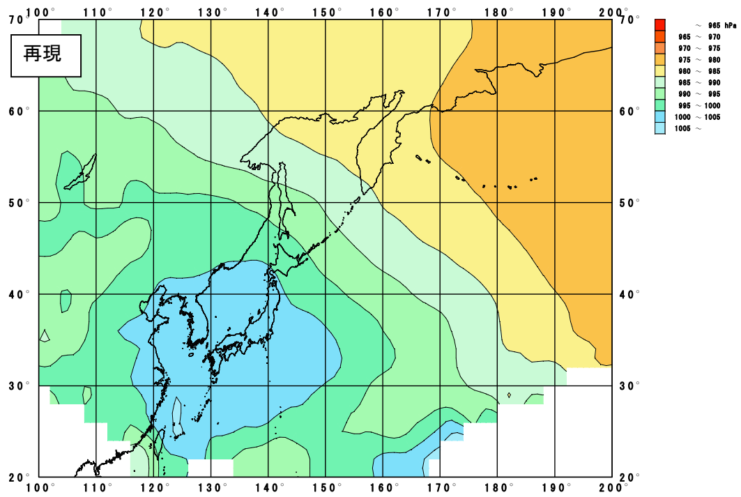
図-48 低気圧の中心気圧の平均値(上:実測, 下:再現)
