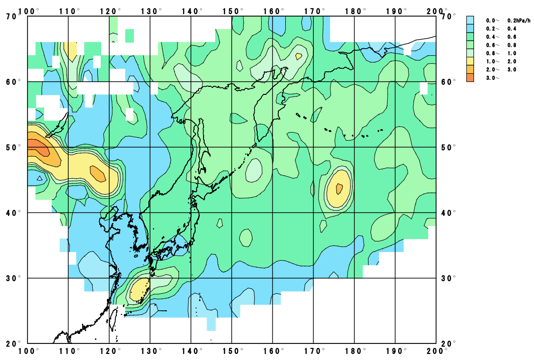
図-39(1) 中心気圧の時間変化量の平均値(上)および標準偏差(下)
