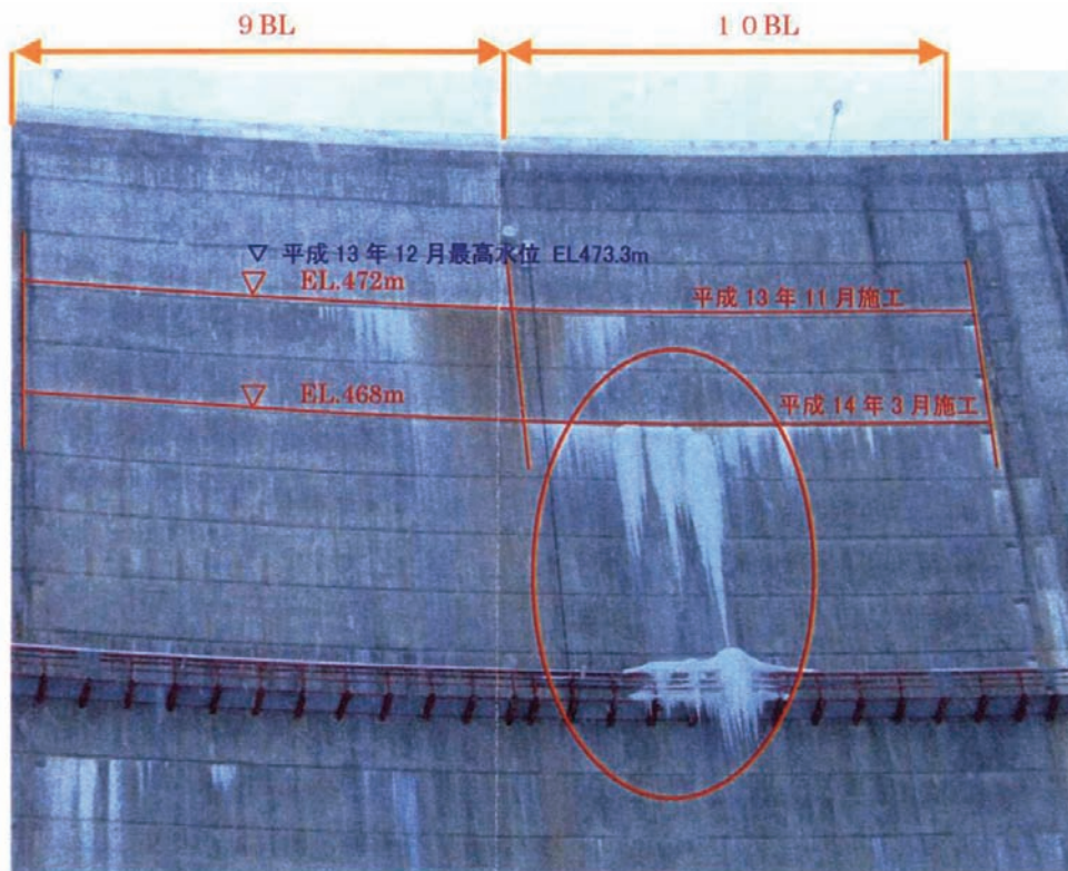
写真 3.10 試験施工前の氷塊発生状況(平成 7 年 1 月)
