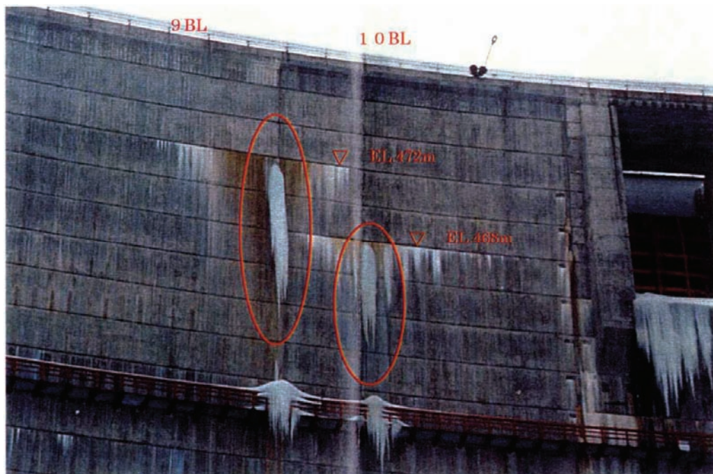
写真 3.10 試験施工前の氷塊発生状況(平成 7 年 1 月)
