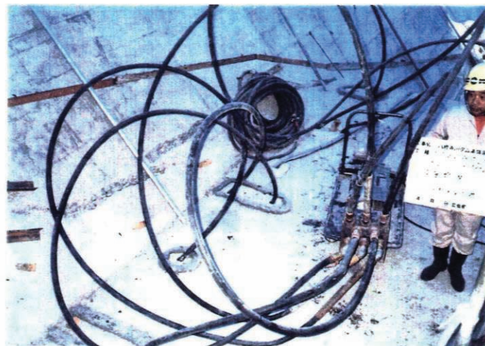
写真 3.7 C工法 温風乾燥工状況
