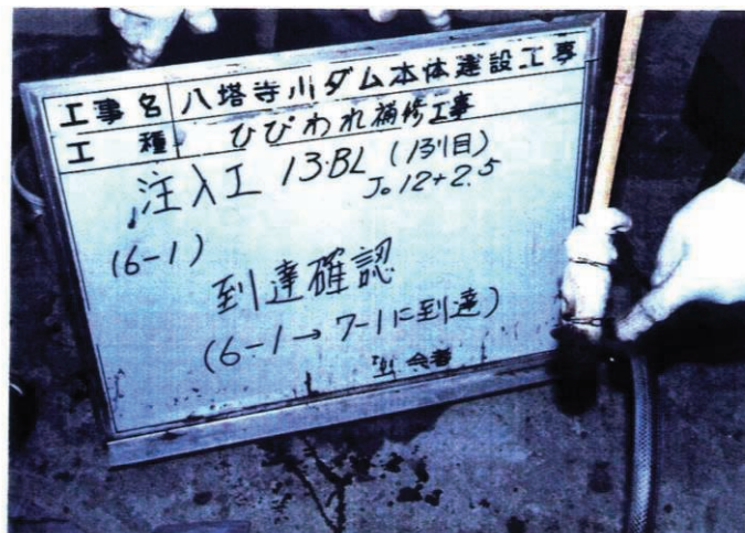
写真 3.8 C工法 樹脂到達確認状況
