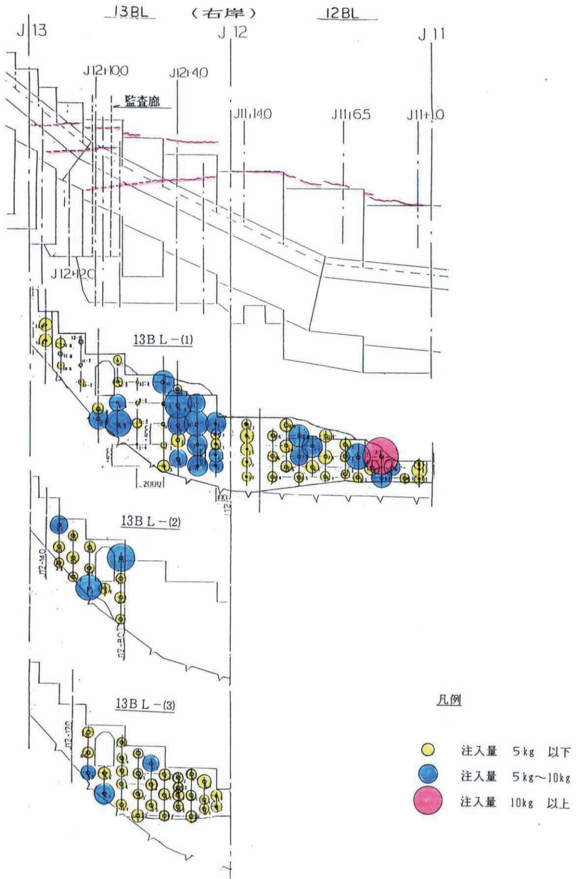
図 3.15 下流フーチング部注入工 注入量マップ(2)
