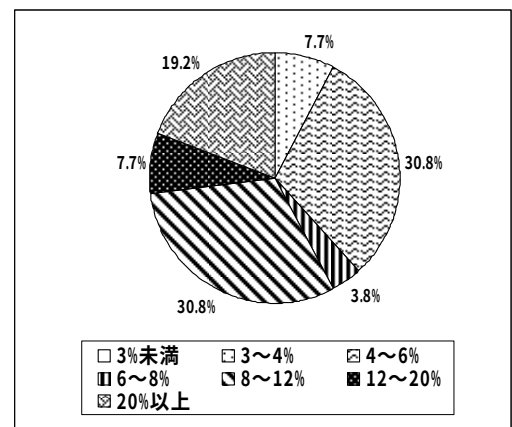
図-2 路床の設計 CBR の分布：全数 26
