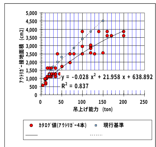
図-18 吊上げ能力と接地面積
