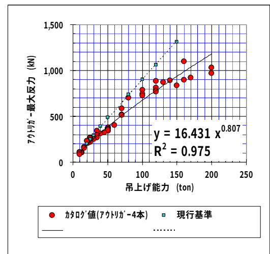
図-17 吊上げ能力と最大反力
