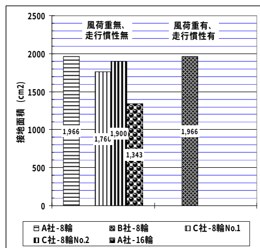
図-29 接地面積
