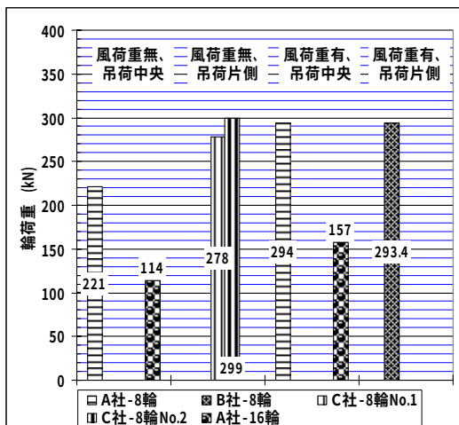
図-31 輪荷重
