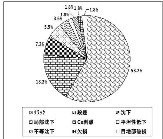
図-5 Co舗装の破損性状：全数 55
