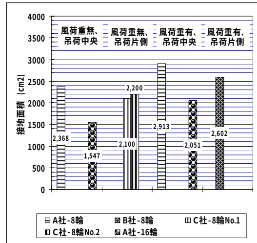
図-32 接地面積
