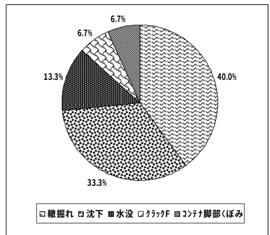
図-6 As舗装の破損性状：全数 15
