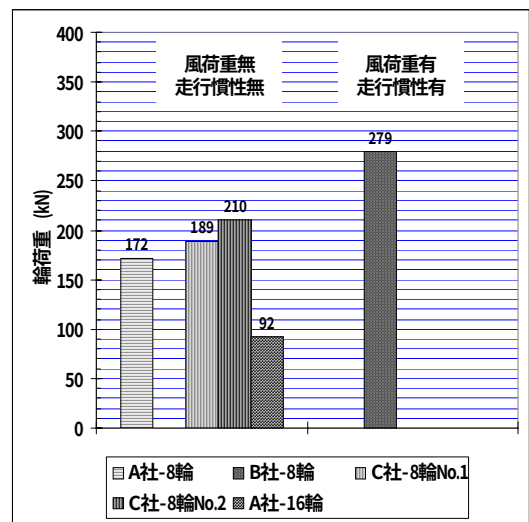
図-28 輪荷重
