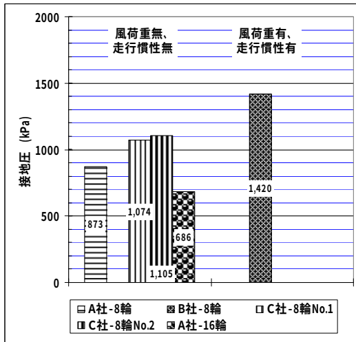
図-30 接地圧
