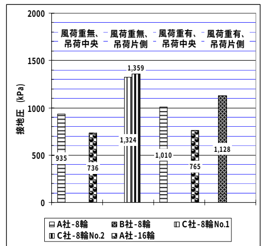
図-33 接地圧
