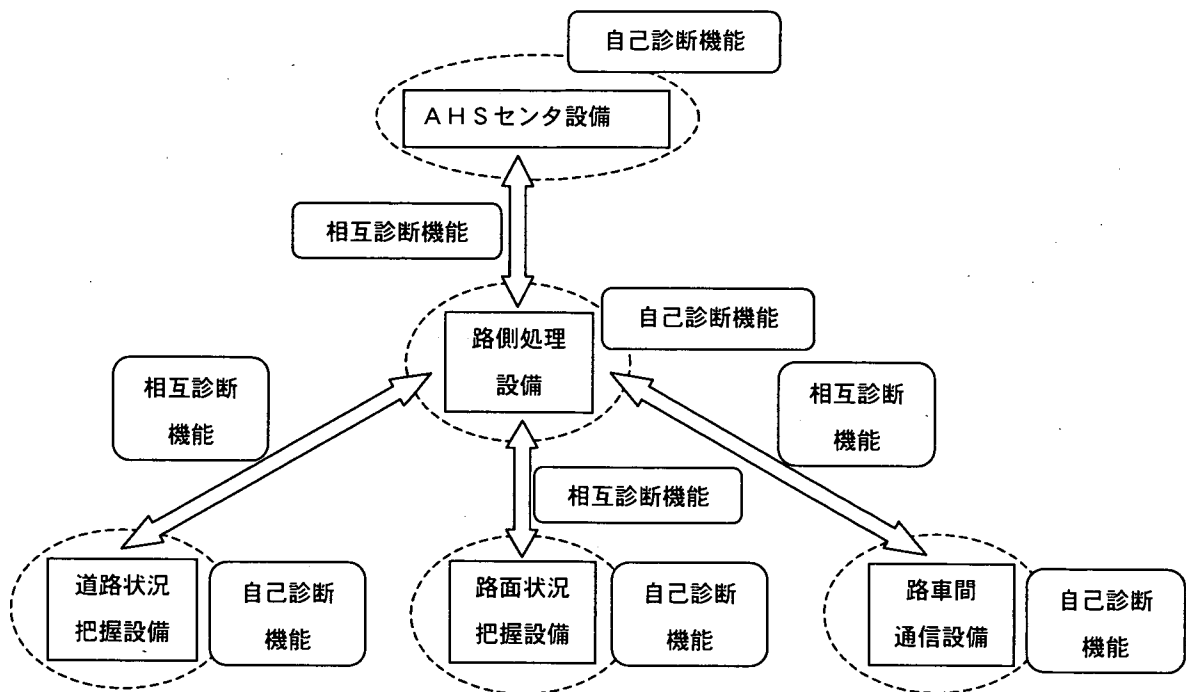
図 5.1-3 路側のAHS設備の設備管理機能の分担
