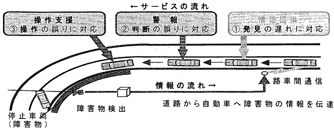
図 1.3.2-2 支援のイメージ（前方障害物衝突防止の例） AHSはカーブの先の障害物を検出して路車間通信により自動車に情報を伝達する。自動車はドライバにその情報を提供する。減速などのドライバによる回避行動が不十分なときは警告を発し、それでも十分な回避行動が行われないときには、自動ブレーキなどの操作支援を行う。
