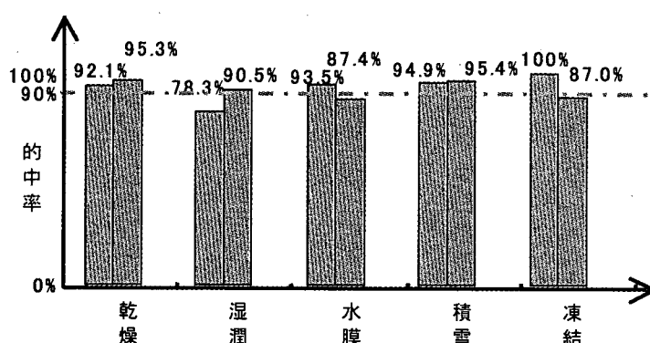
図 2.4.1-1 路面5状態判別精度/的中率 積雪を例にとると、的中率とは、センサが積雪と出力した場合に観測路面(真値)が積雪である確率、正解率とは、観測路面(真値)が積雪である場合にセンサが積雪と出力する確率である。
