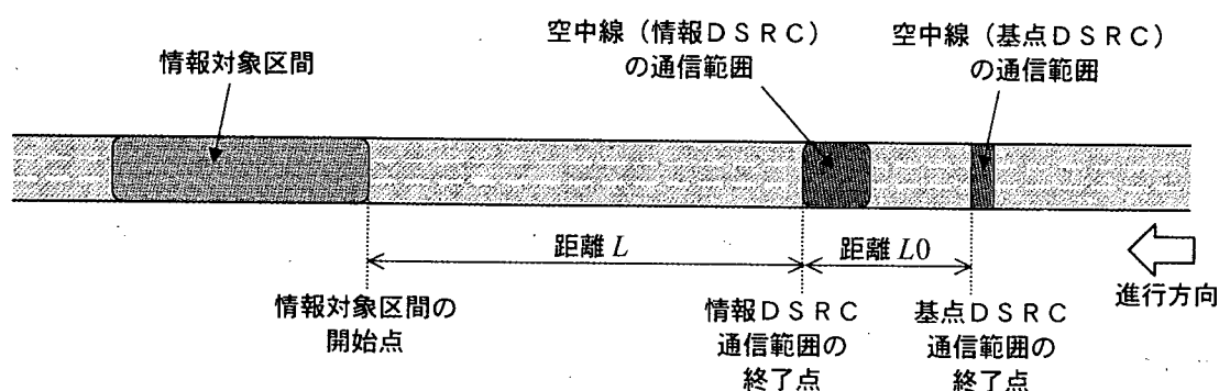
図 6.6-6 通信範囲
