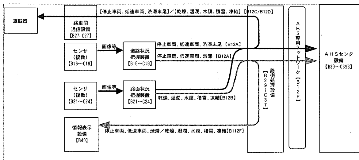
図 2.4-1 AHSインタフェース概念図
