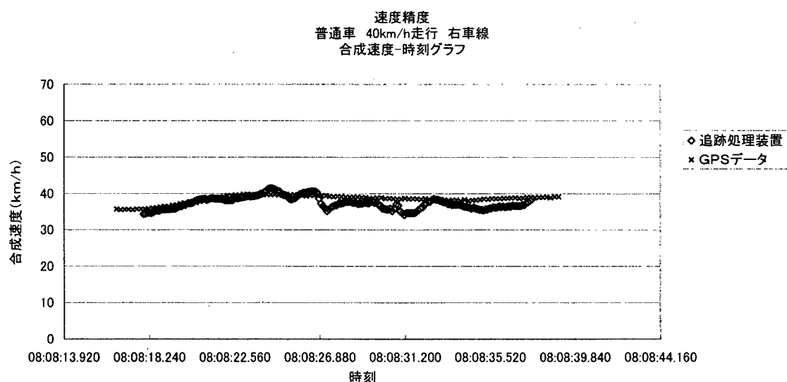
図 3. 2. 2-8 直進走行（40km/h）普通右車線 合成速度－時刻グラフ
