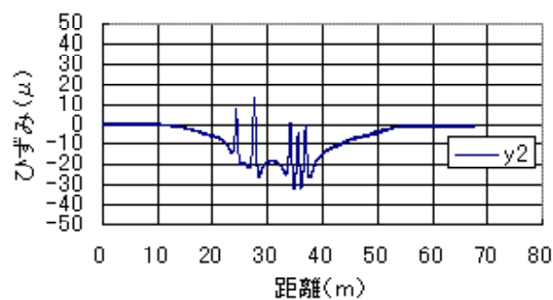
図-2.6.20 試験橋梁各部の応答（ケース L1-5）
